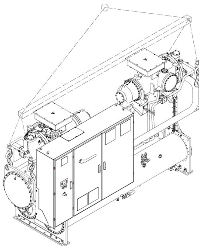
Enota z dvojnimi krogoma
