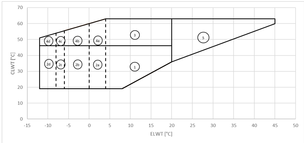
Slika 5 – Ovojnica EWWD_VZ_SS
