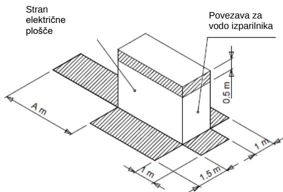
Slika 4 – Nameščanje enote
