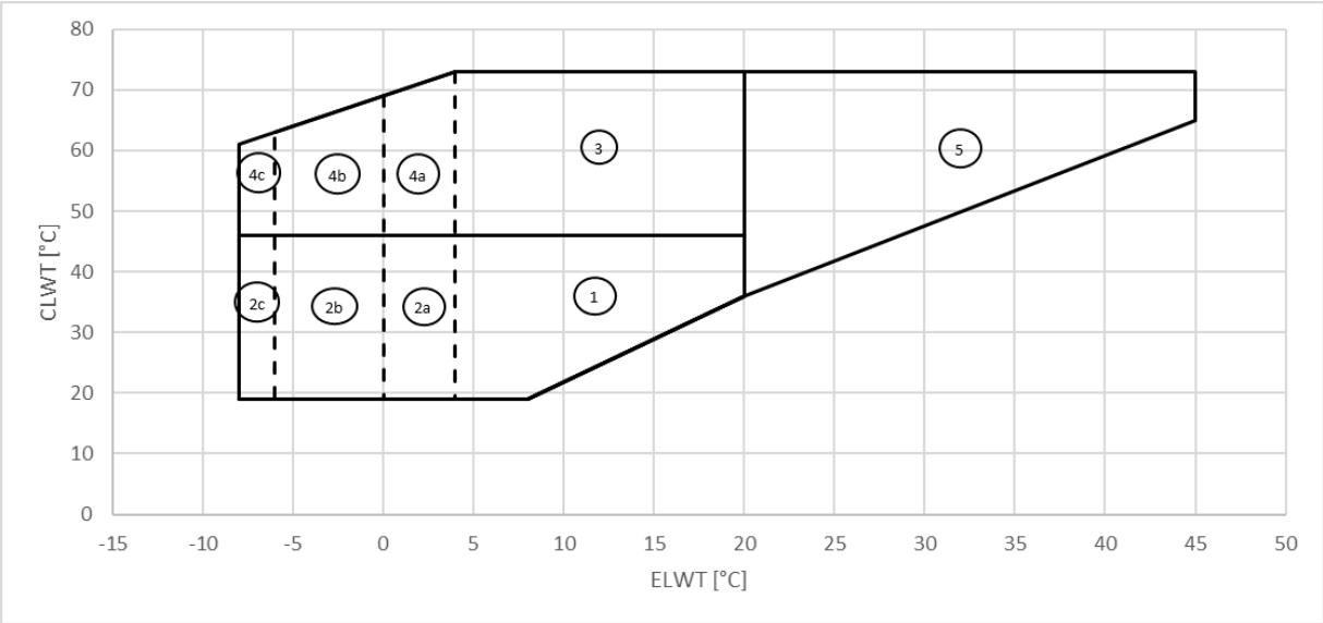
Figură 7 - EWWH_VZ_SS
