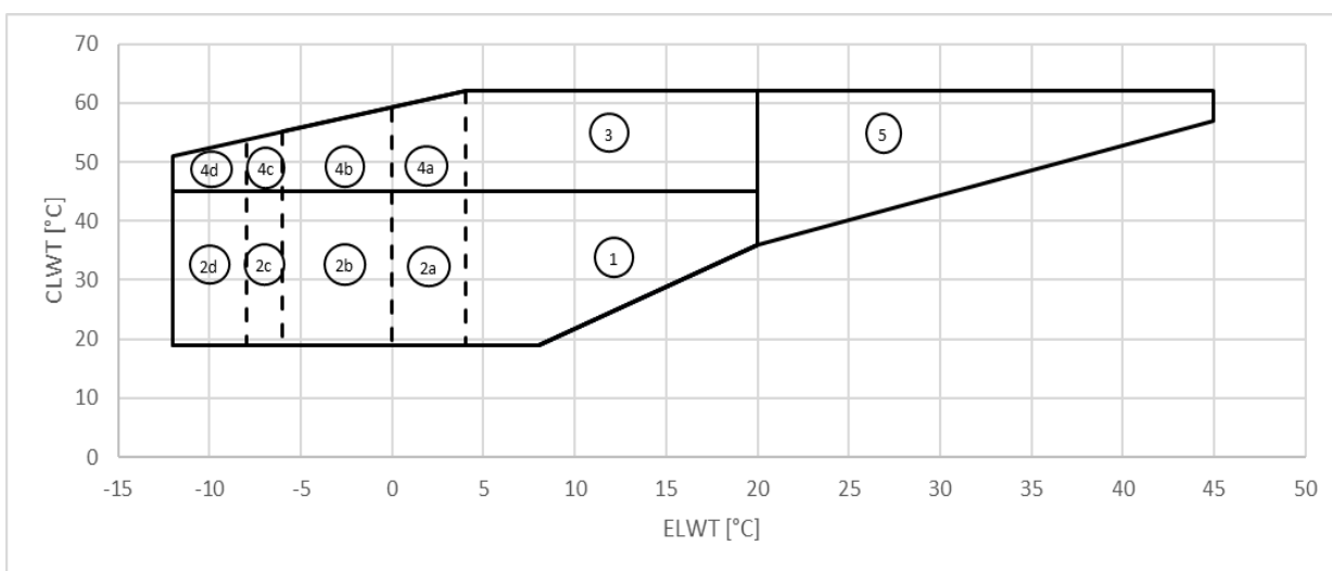
Figură 11 - EWWS_VZ_XS/PS
