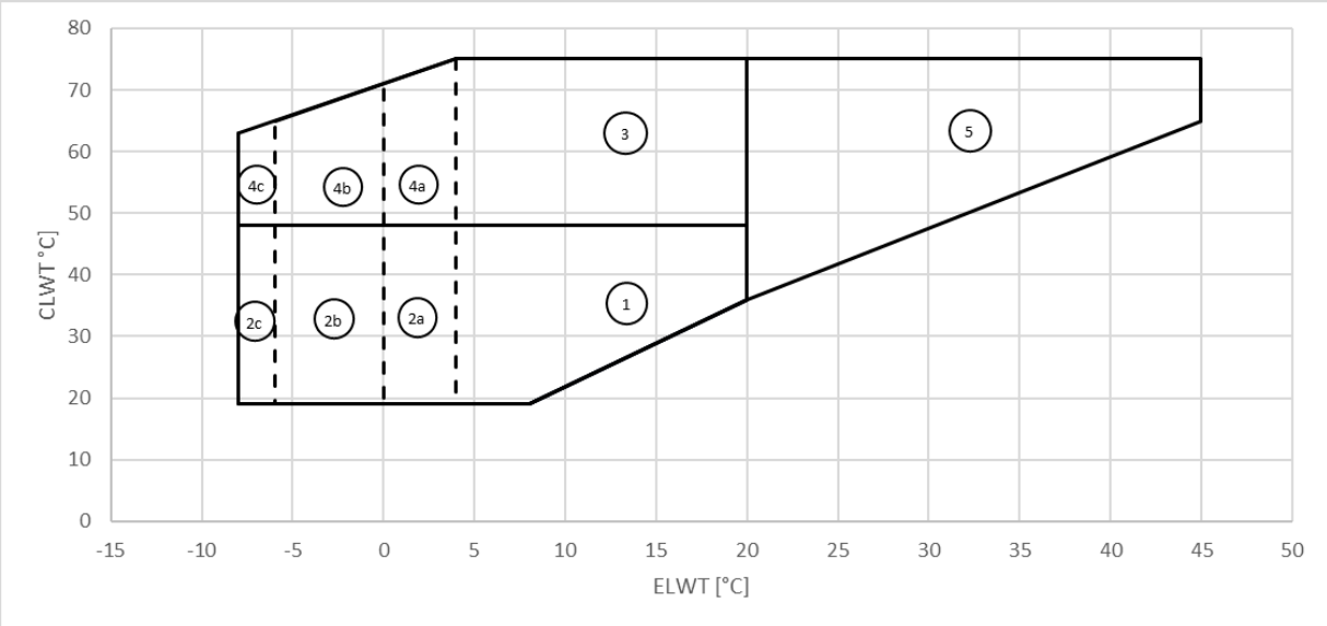
Figură 8 - EWWH_VZ_XS
