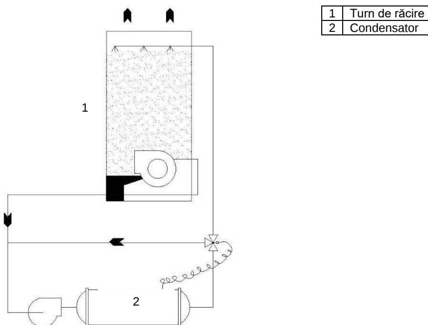
Figură 12 - Schema de control a condensatorului cu turn de răcire
