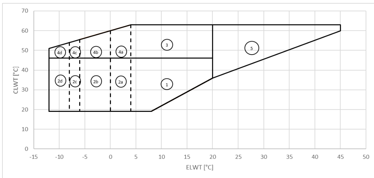
Figură 5 - Înveliș EWW-D-VZ_SS
