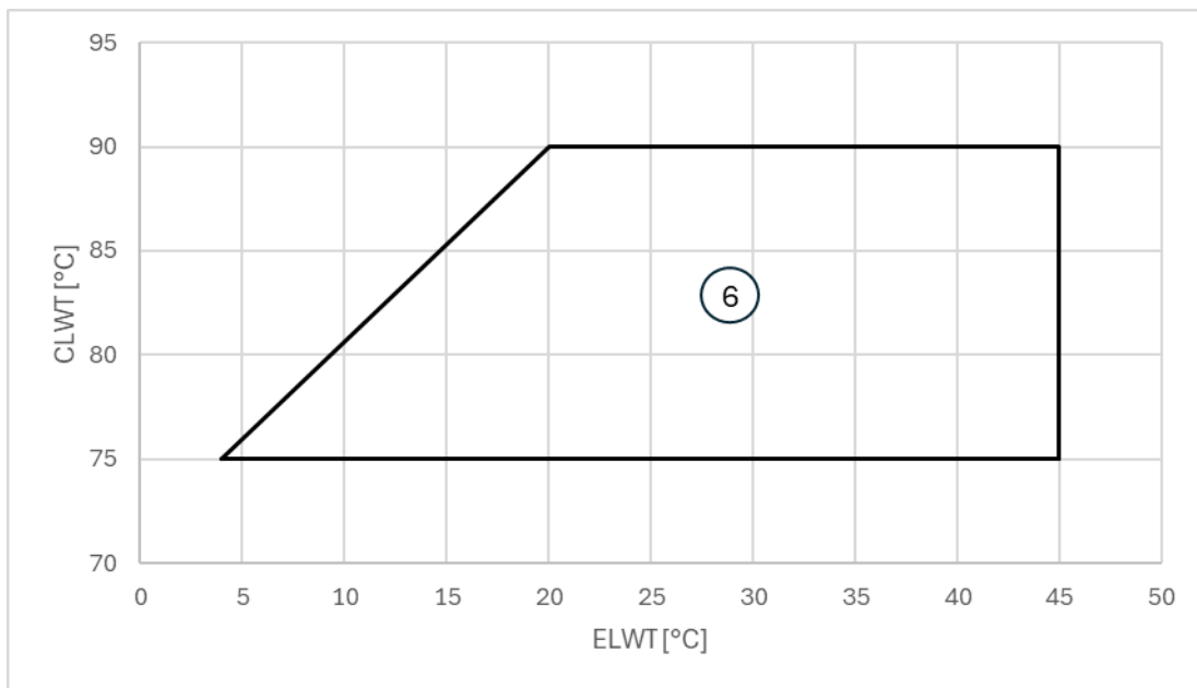
Afbeelding9 - EWWH_VZ_XS/PS Optie 251
