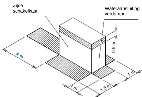
Afbeelding4 – Positionering eenheid
