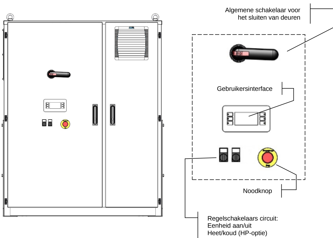
Afbeelding15 – Interface eenheid
