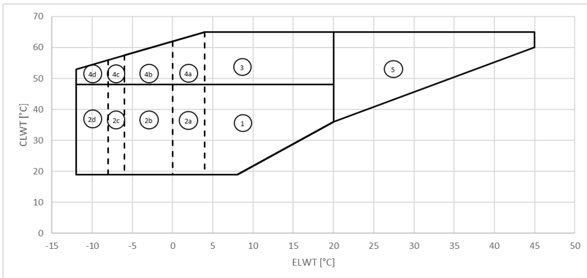
Afbeelding6 - EWWD-VZ-XS/PS
