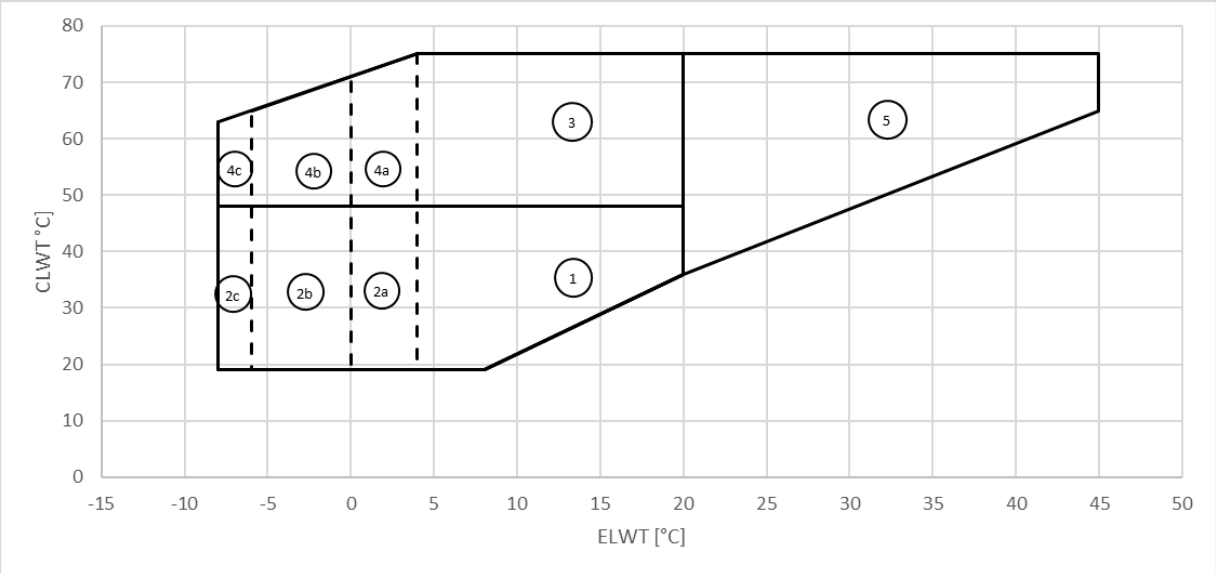
Afbeelding8 - EWWH_VZ_XS
