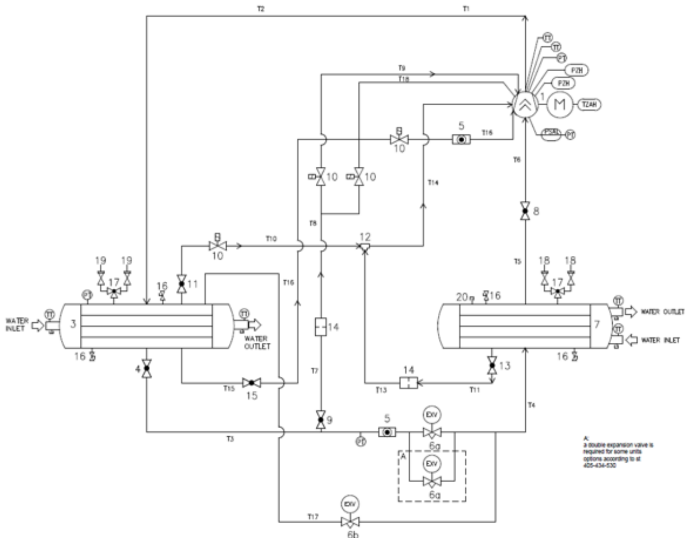
Afbeelding14 - P&ID optie251
