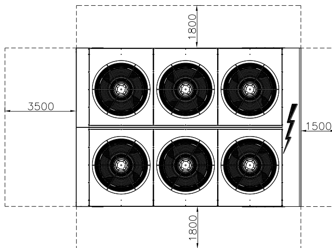
Fig. 5 - Cerințe minime de spațiu liber pentru întreținerea aparatului
