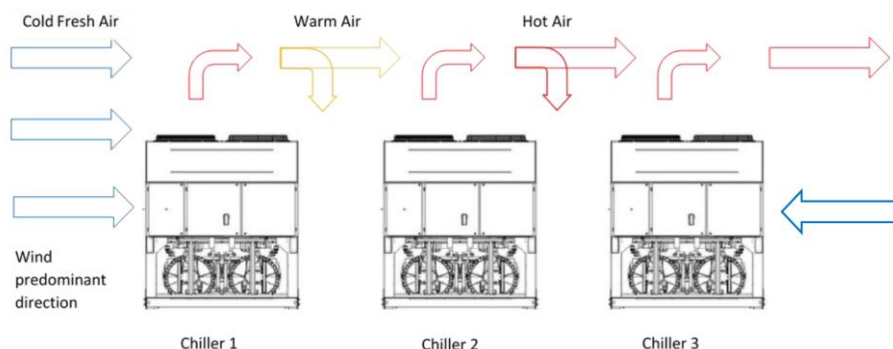
Fig. 6 - Instalarea mai multor răcitoare
