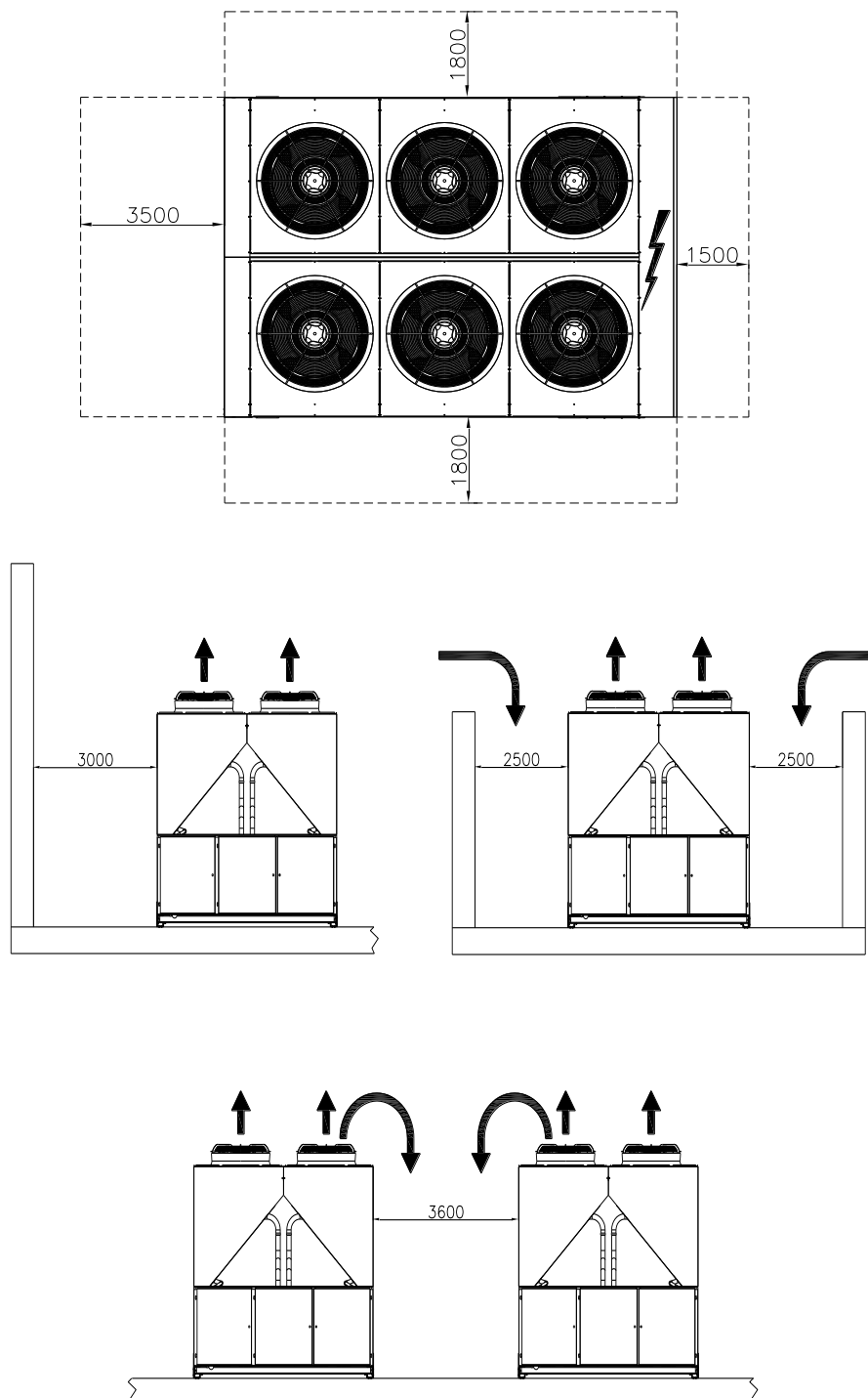
5 ábra - A gép karbantartásához szükséges minimális távolsági követelmények
