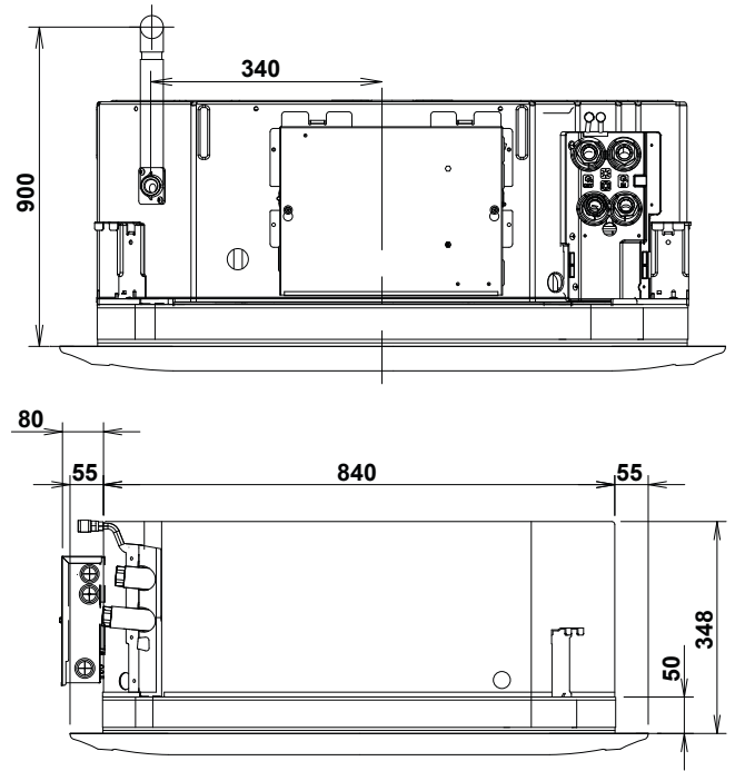
Seitenansichten mit Zierblende (mm)
