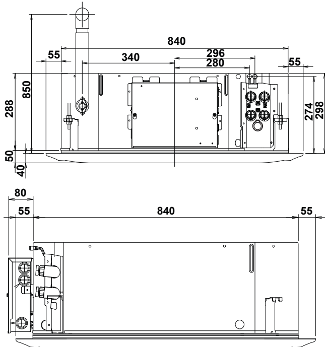
Seitenansichten mit Standardblende (mm)
