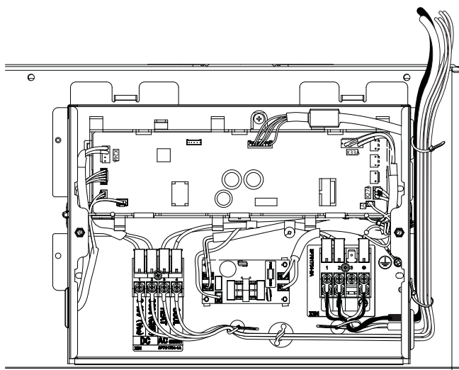
5 Die Stromversorgungskabel (L, N, Earth) am oberen Teil des X1M-Anschlusses anschließen.
