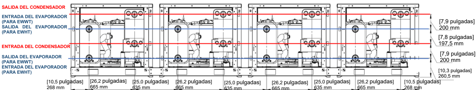
Fig. 28 - Configuración de las tuberías de agua
