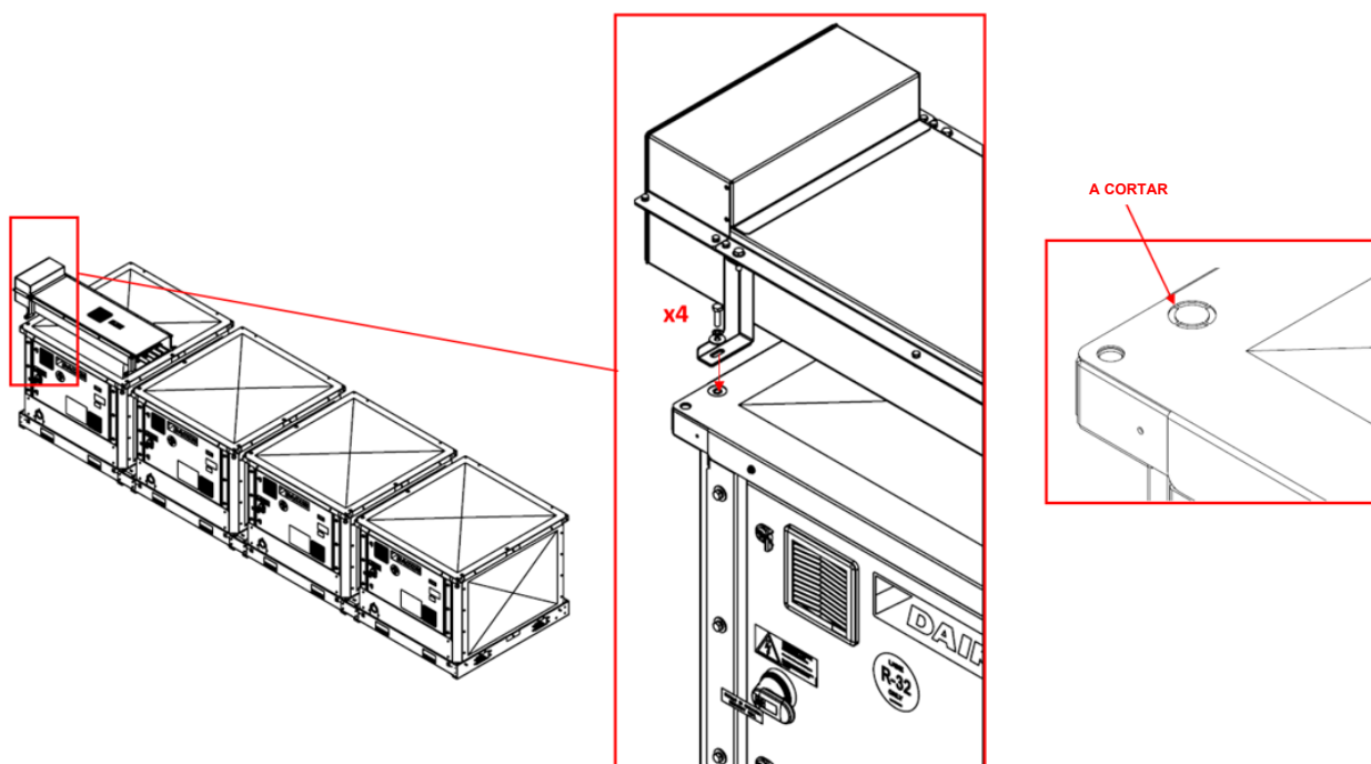
Fig. 55 - Fijación del sistema de barras de alimentación a la unidad
