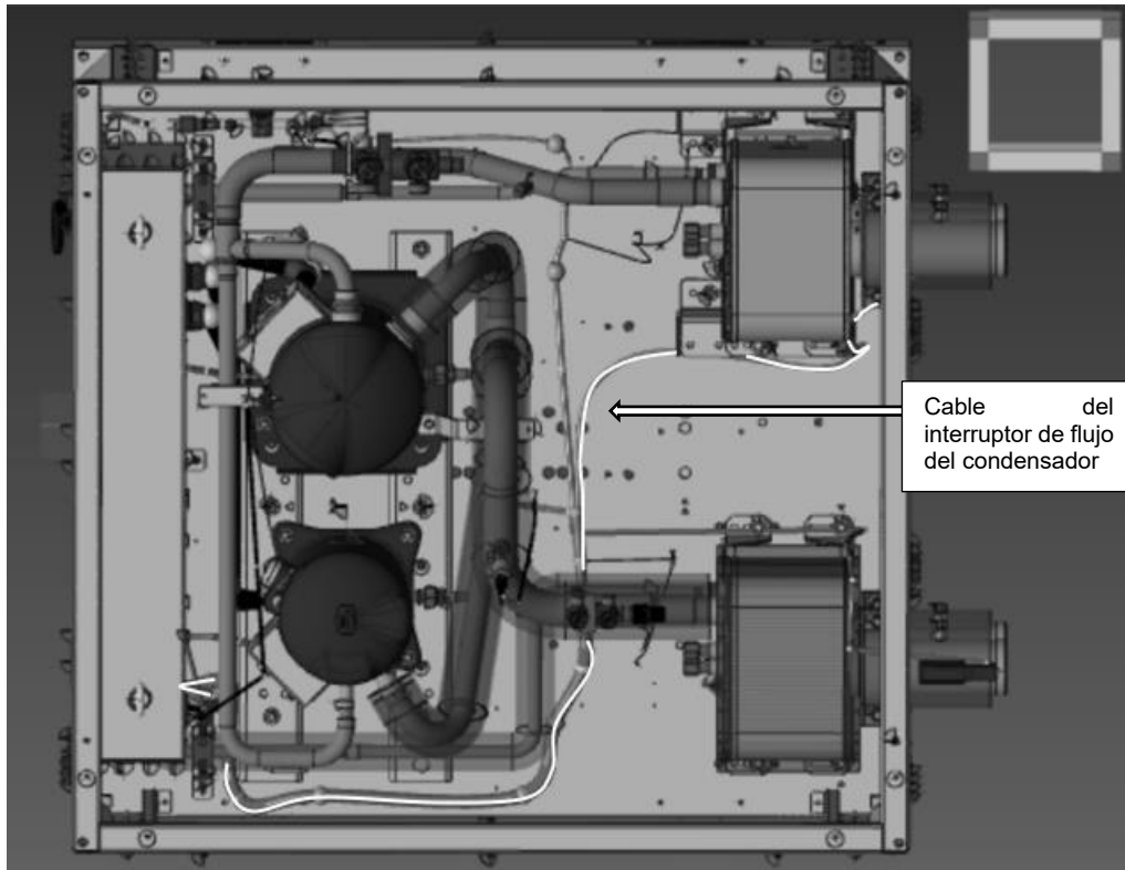
Fig. 18 - Punto de entrada del cuadro eléctrico para los cables del interruptor de flujo del evaporador y del condensador
