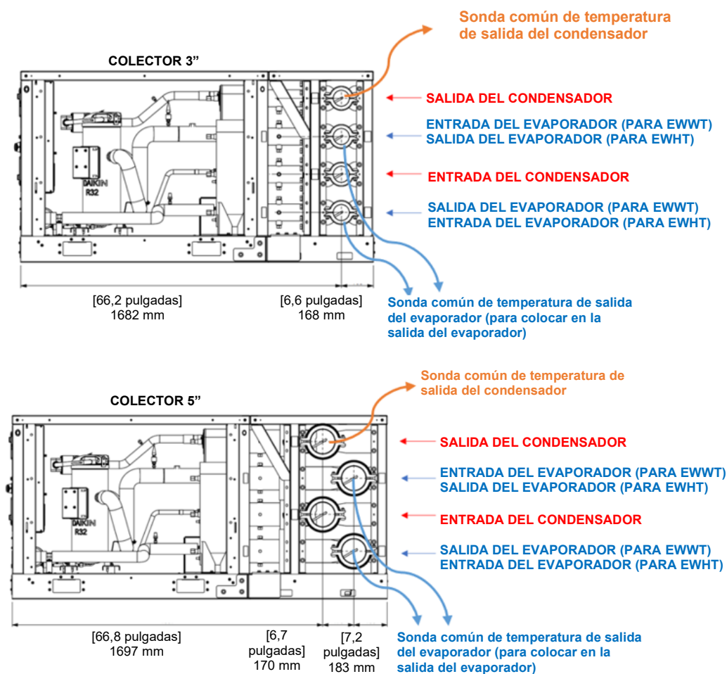
Fig. 62 - Posiciones de las sondas de temperatura para colectores de 3" y 5"
