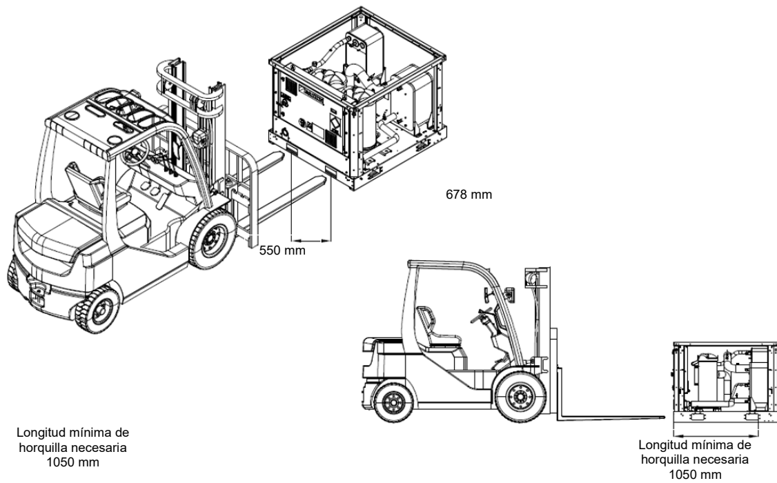
Fig. 12 - Método alternativo de manipulación con carretilla elevadora
