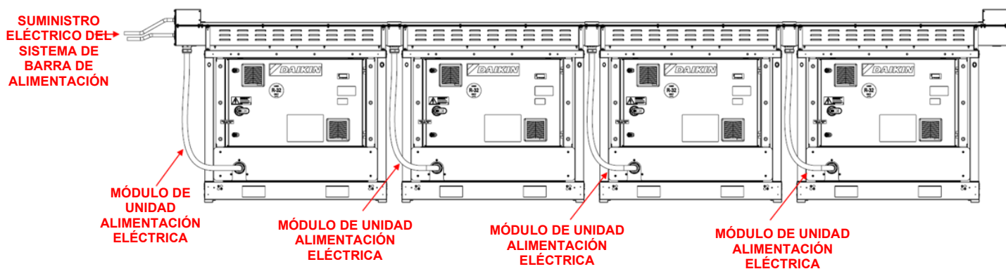
Fig. 54 - Detalles del cableado
