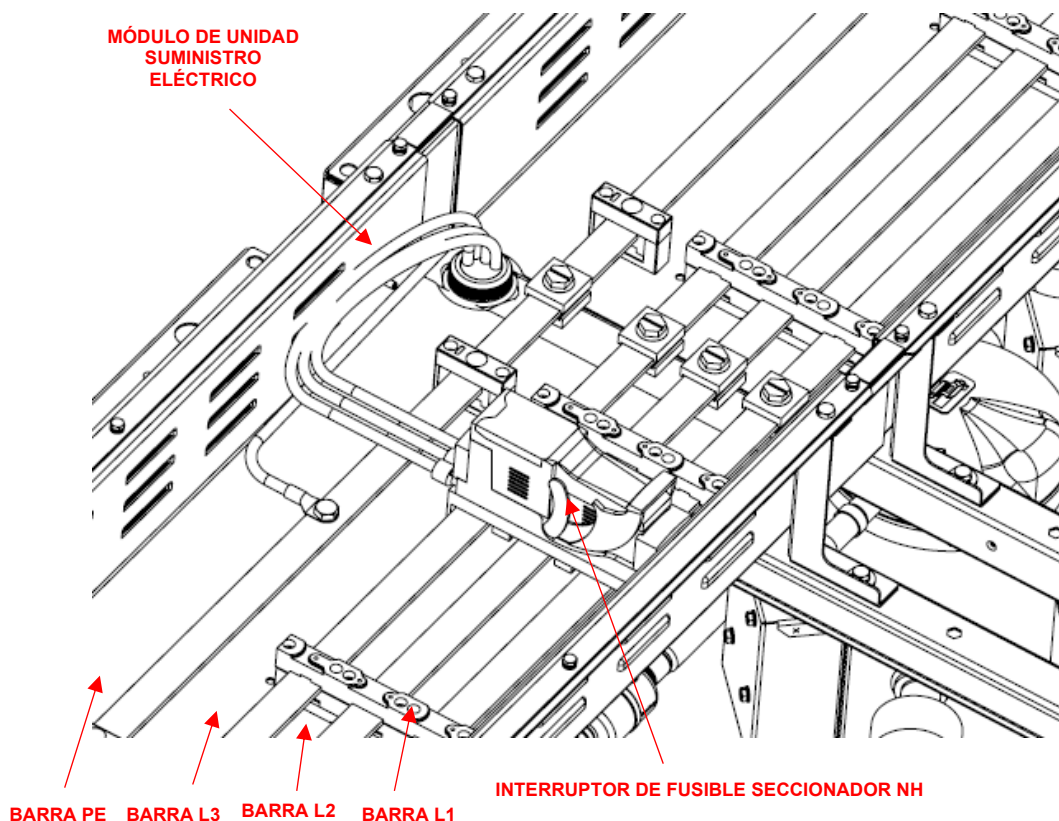
Fig. 60 - Detalle de la conexión eléctrica para cualquier otro módulo de la unidad
