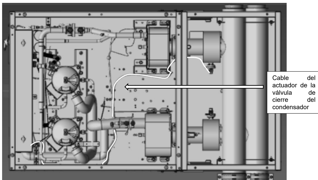
Fig. 40 - Cableado del actuador de la válvula de cierre del condensador
