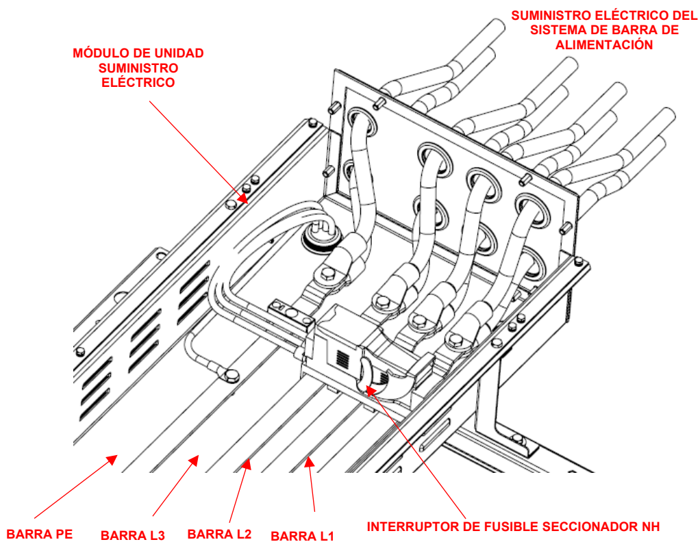
Fig. 59 - Detalle de la conexión eléctrica del módulo de la unidad inicial
