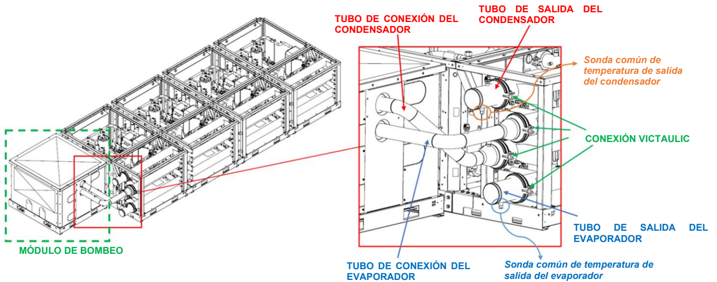
Fig. 63 - Detalles de la colocación de las sondas en los tubos
