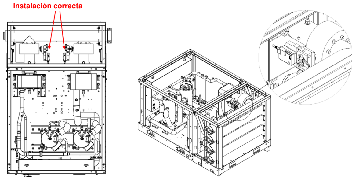
Fig. 34 - Indicaciones de montaje para el actuador de la válvula
