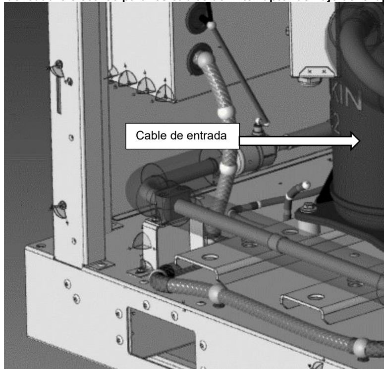
Fig. 18 - Punto de entrada del cuadro eléctrico para los cables del interruptor de flujo del evaporador y del condensador
