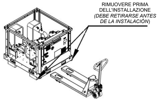
Fig. 13 - Método alternativo de manipulación con transpaleta
