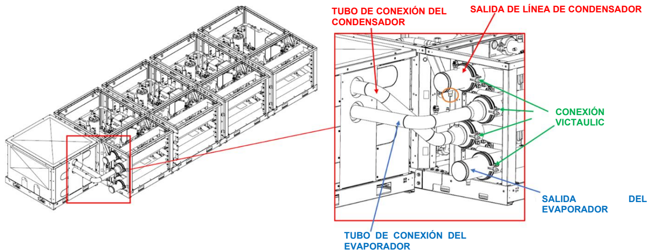
Fig. 46 - Instalación del módulo de bombeo - detalles de las tuberías
