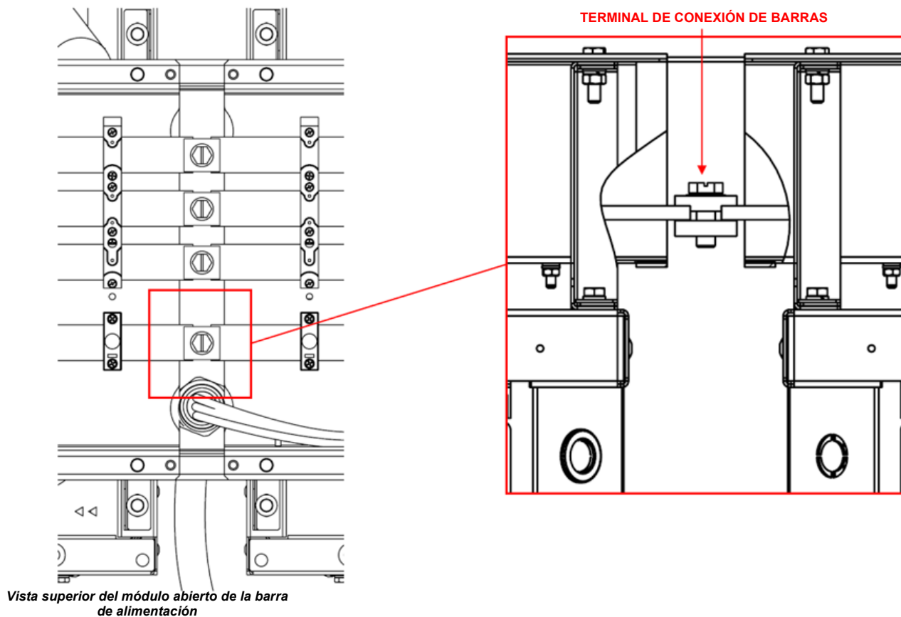
Fig. 57 - Detalles de la conexión de los módulos de la barra de alimentación
