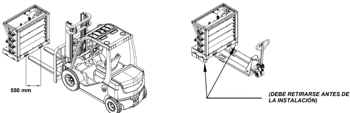
Fig. 47 - Manipulación del módulo distribuidor
