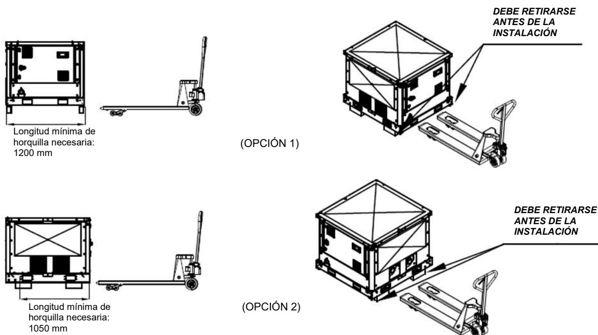
Fig. 51 - Manipulación del módulo de bomba con transpaleta
