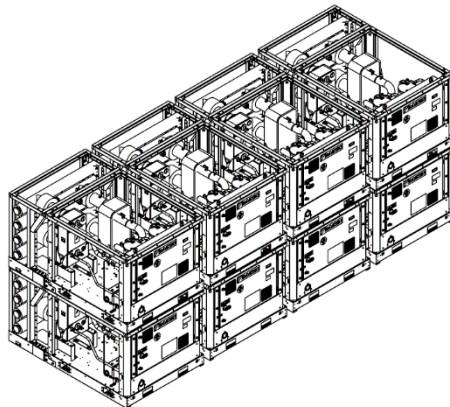
Fig. 44 - Instrucciones de montaje de sistemas de múltiples colectores de unidades entre sí
