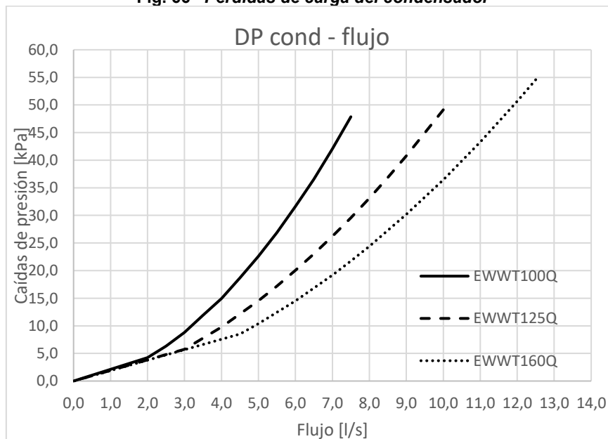
Fig. 66 - Pérdidas de carga del condensador
