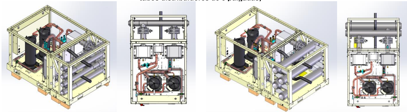
Fig. 27 - Tubos PHR con módulo distribuidor (a la izquierda para tubos distribuidores de 3 pulgadas - a la derecha para tubos distribuidores de 5 pulgadas)
