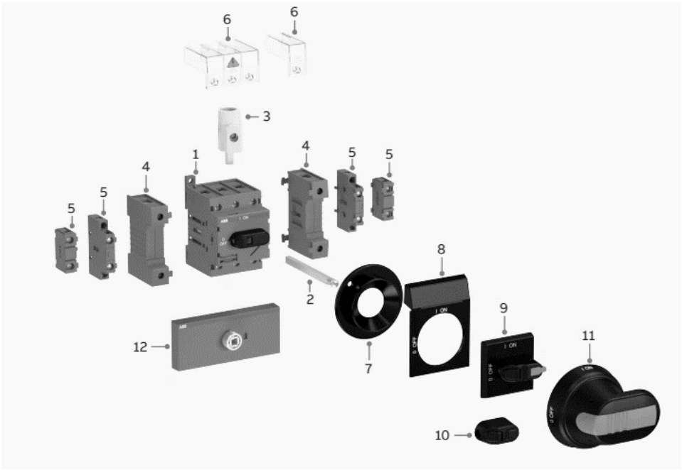
Fig. 23 - Instrucciones de montaje del mango
