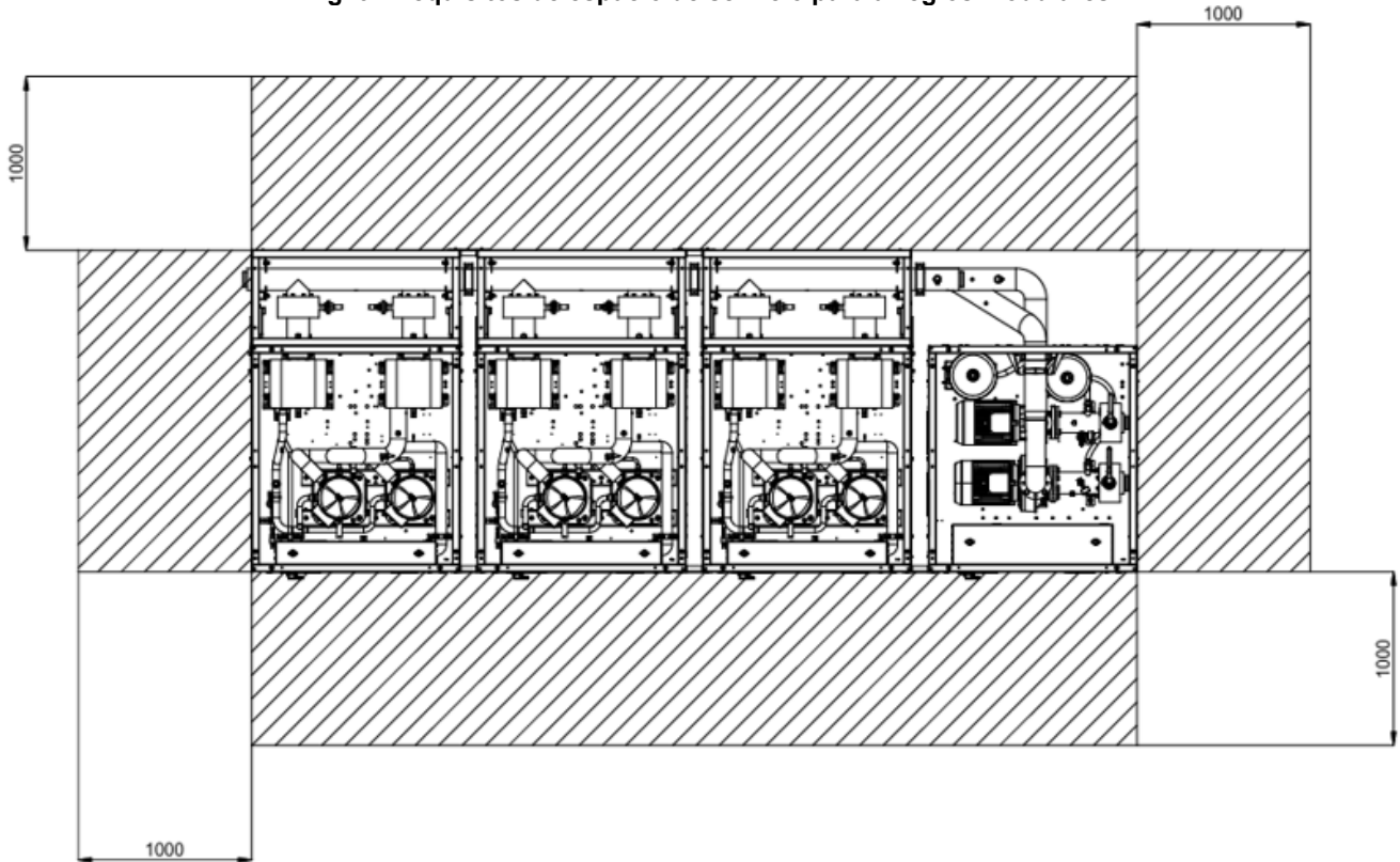
Fig. 9 –Requisitos de espacio de servicio para arreglos modulares
