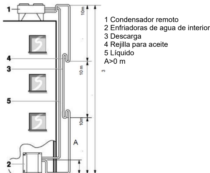
Fig. 20 - Conexión del circuito de refrigerante (1)
