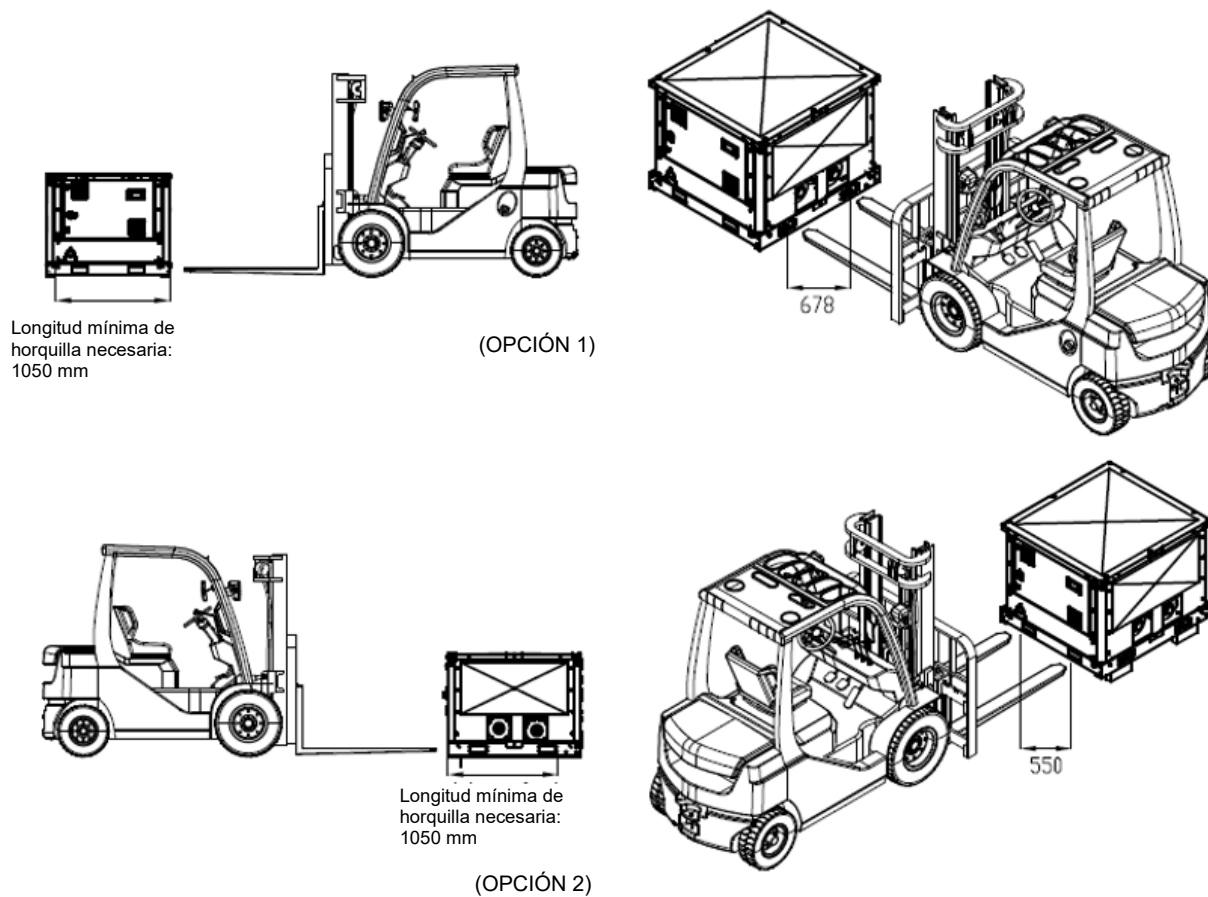
Fig. 50 - Manipulación del módulo de bombeo con carretilla elevadora
