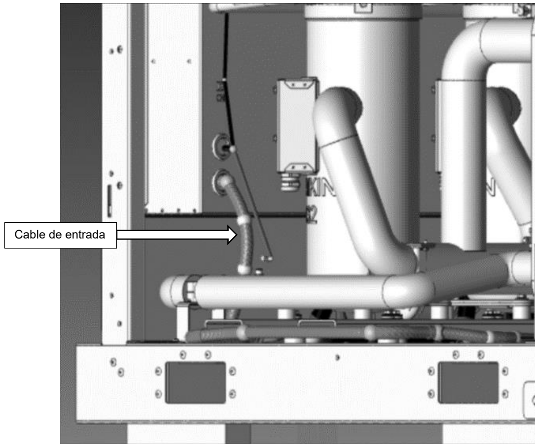
Fig. 41 - Entrada del panel eléctrico para los cables del actuador de las válvulas de cierre del evaporador y del condensador
