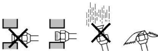
Fig. 21 - Conexión del circuito de refrigerante (4)
