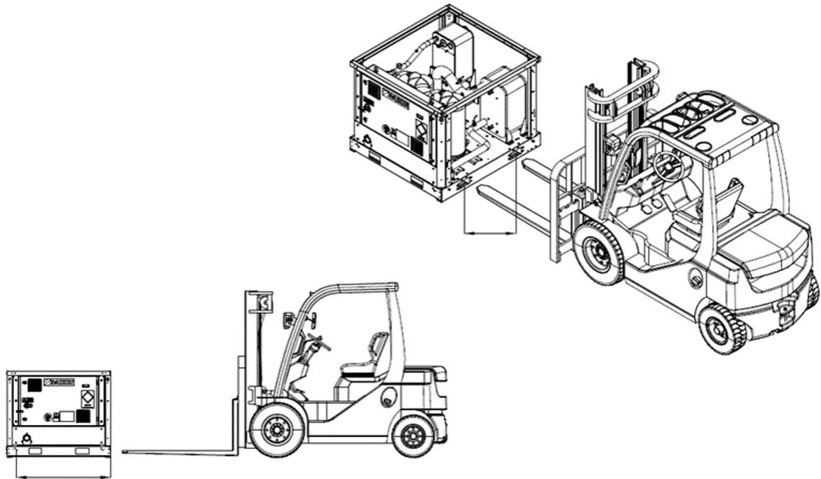
Fig. 11 - Manipulación de la unidad de circuito único
