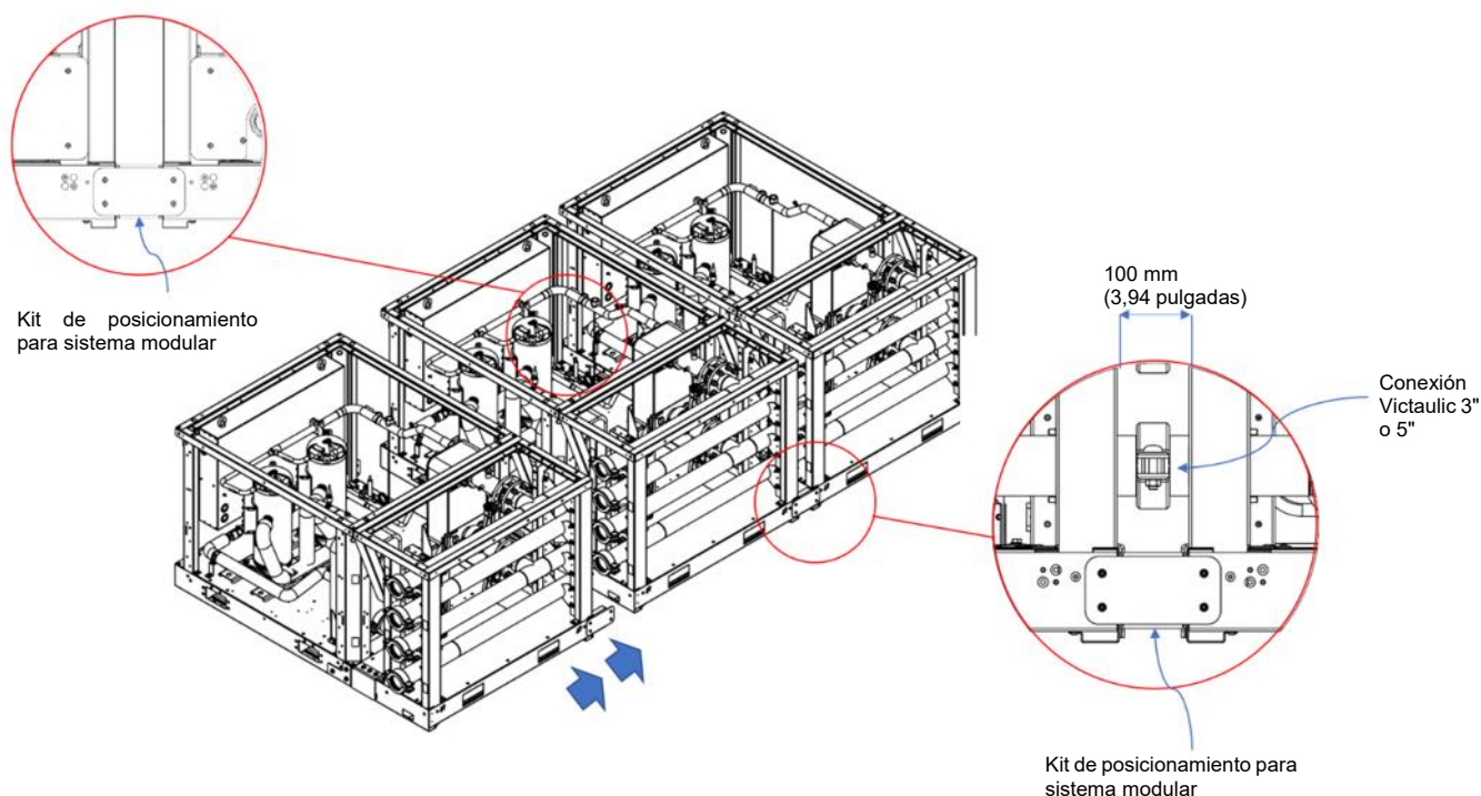
Fig. 29 - Conexión de sistemas modulares
