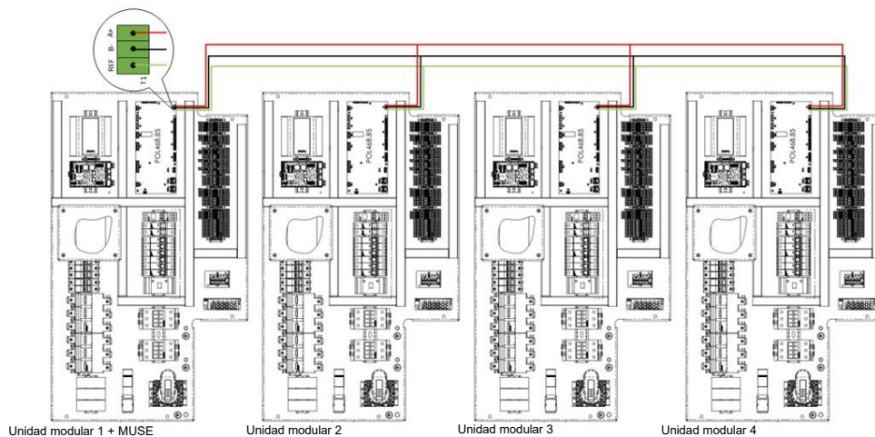
Fig. 64 - Conexión de 4 PLC en la misma red Modbus
