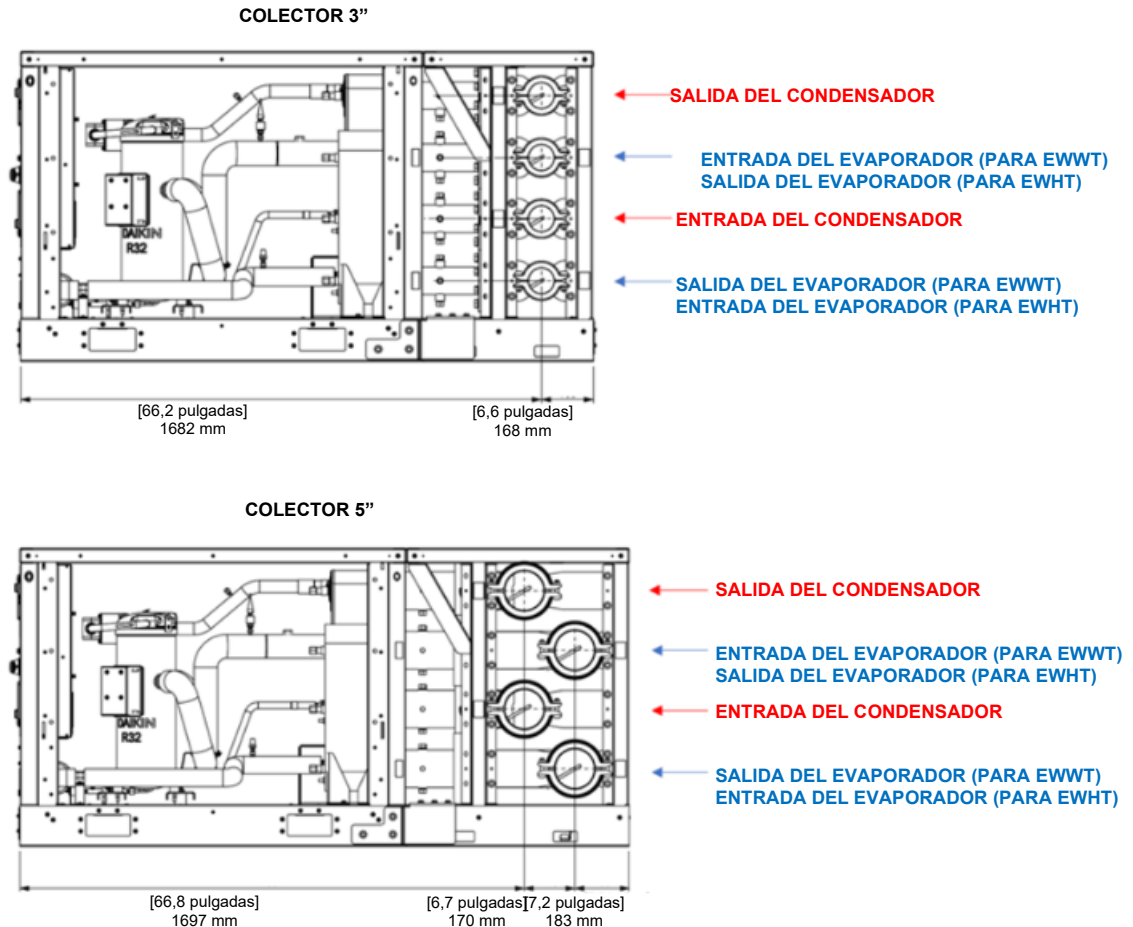
Fig. 30 - Tamaños de los colectores de agua
