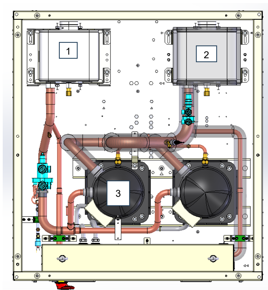
Fig. 14 - Plano de referencia para la identificación del evaporador y el condensador
