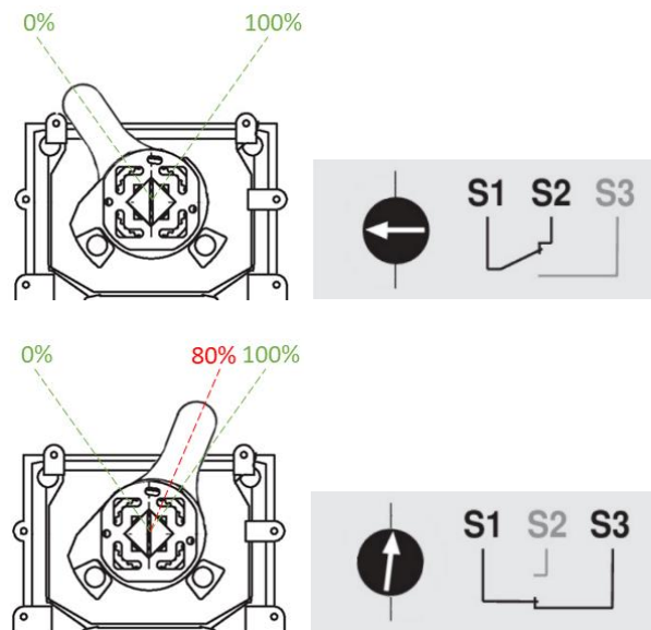
Fig. 42 - Configuración del disparador de interruptores de límite
