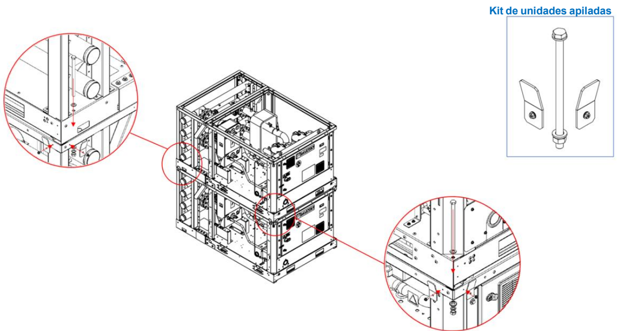
Fig. 43 - Instrucciones de montaje para unidades apiladas
