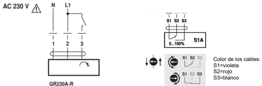
Fig. 35 - Esquema de conexión del motor (figura izquierda) y de los interruptores de límite (figura derecha)
