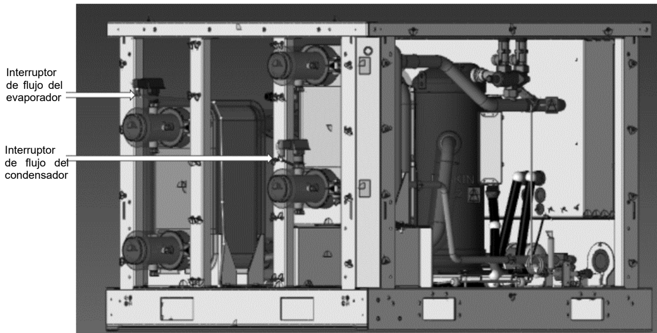
Fig. 16 - Trazado de los cables del interruptor de flujo del evaporador
