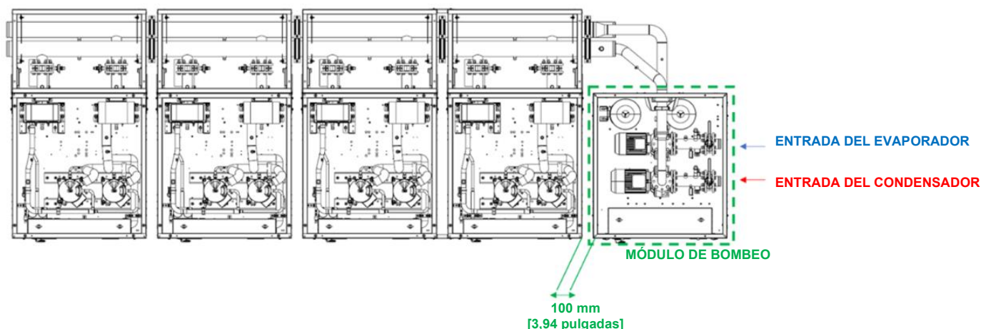
Fig. 46 - Instalación del módulo de bombeo - detalles de las tuberías
