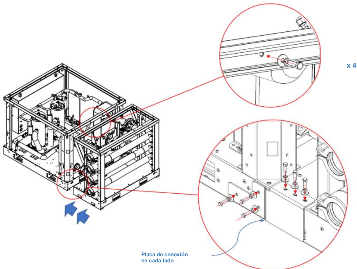
Fig. 26 - Instrucciones de conexión entre la enfriadora y los módulos colectores
