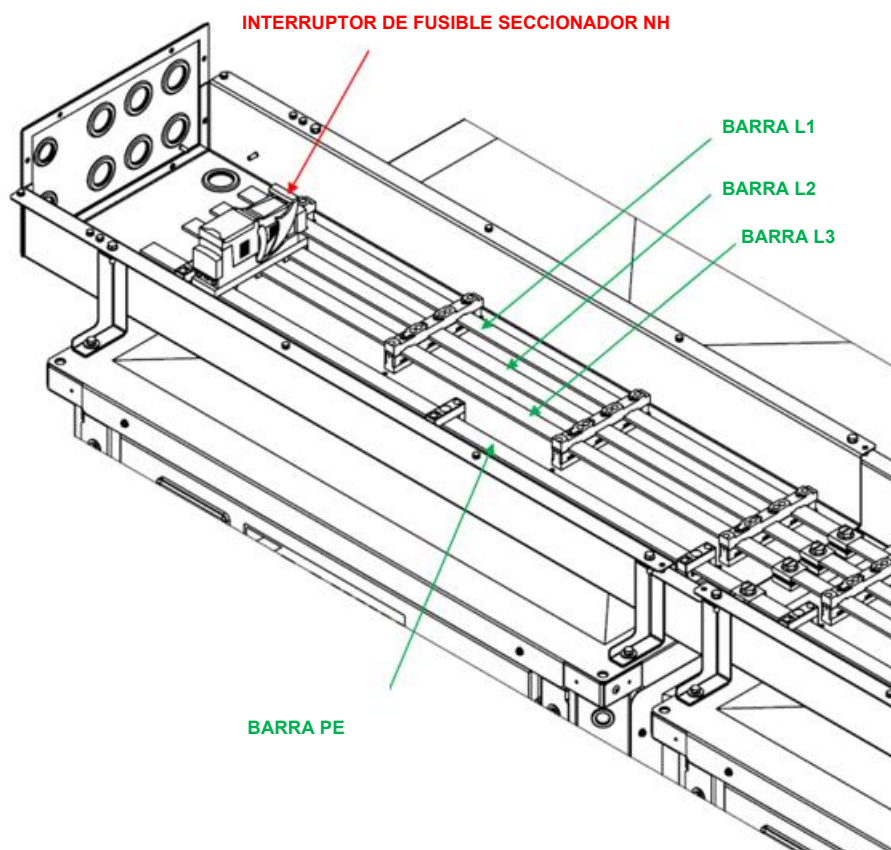
Fig. 58 - Detalle de los fusibles y de la caja de paso de cables del módulo de la barra de alimentación
