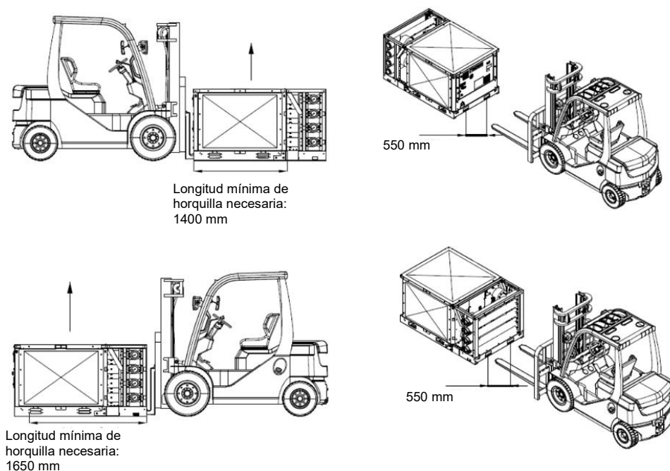
Fig. 48 - Manipulación de la unidad y los módulos colectores
