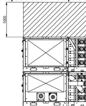
Fig. 10 - Requisitos de espacio de servicio para la configuración apilada
