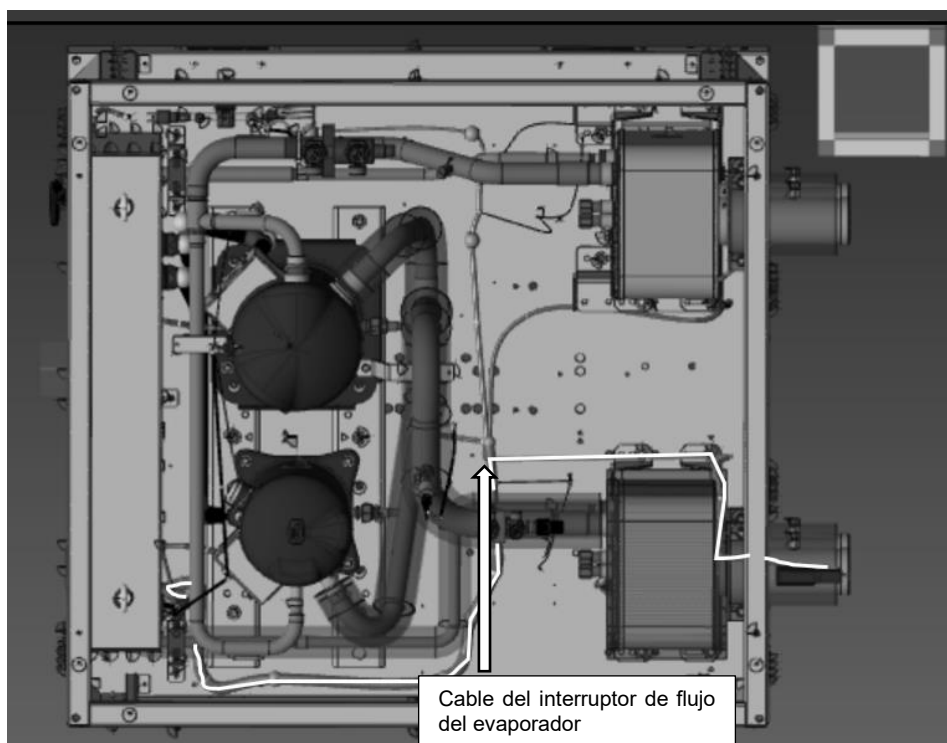
Fig. 16 - Trazado de los cables del interruptor de flujo del evaporador
