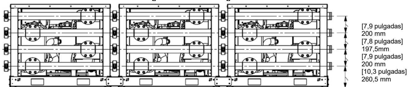
Fig. 31 - Conexión de agua a los módulos
