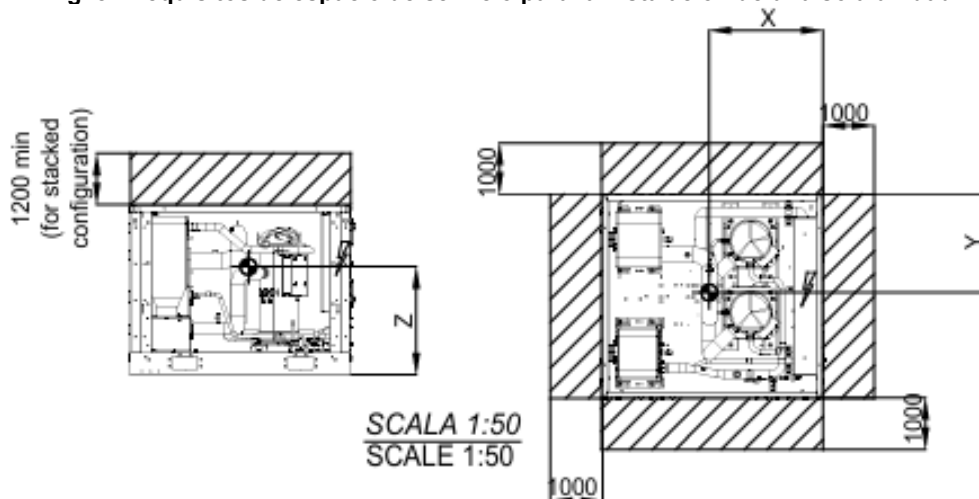
Fig. 8 –Requisitos de espacio de servicio para la instalación de una sola unidad
