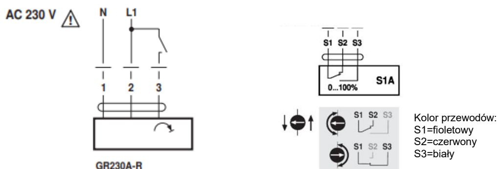
Rys. 35 – Schemat połączeń silnika (lewy rysunek) i wyłączników krańcowych (prawy rysunek)
