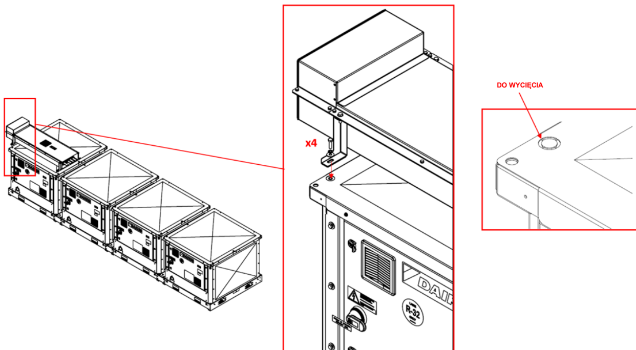
Rys. 55 – Mocowanie systemu listwy zasilającej do urządzenia
