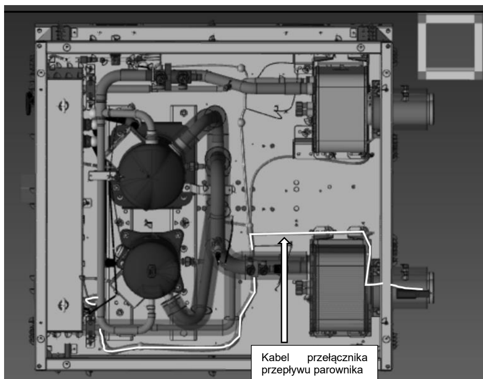
Rys. 16 – Prowadzenie kabli przełącznika przepływu parownika
