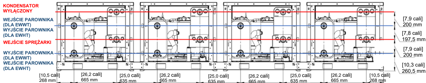
Rys. 28 – Konfiguracja przewodów wodnych
