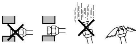
Rys. 21 – Podłączanie obwodu czynnika chłodniczego (4)
