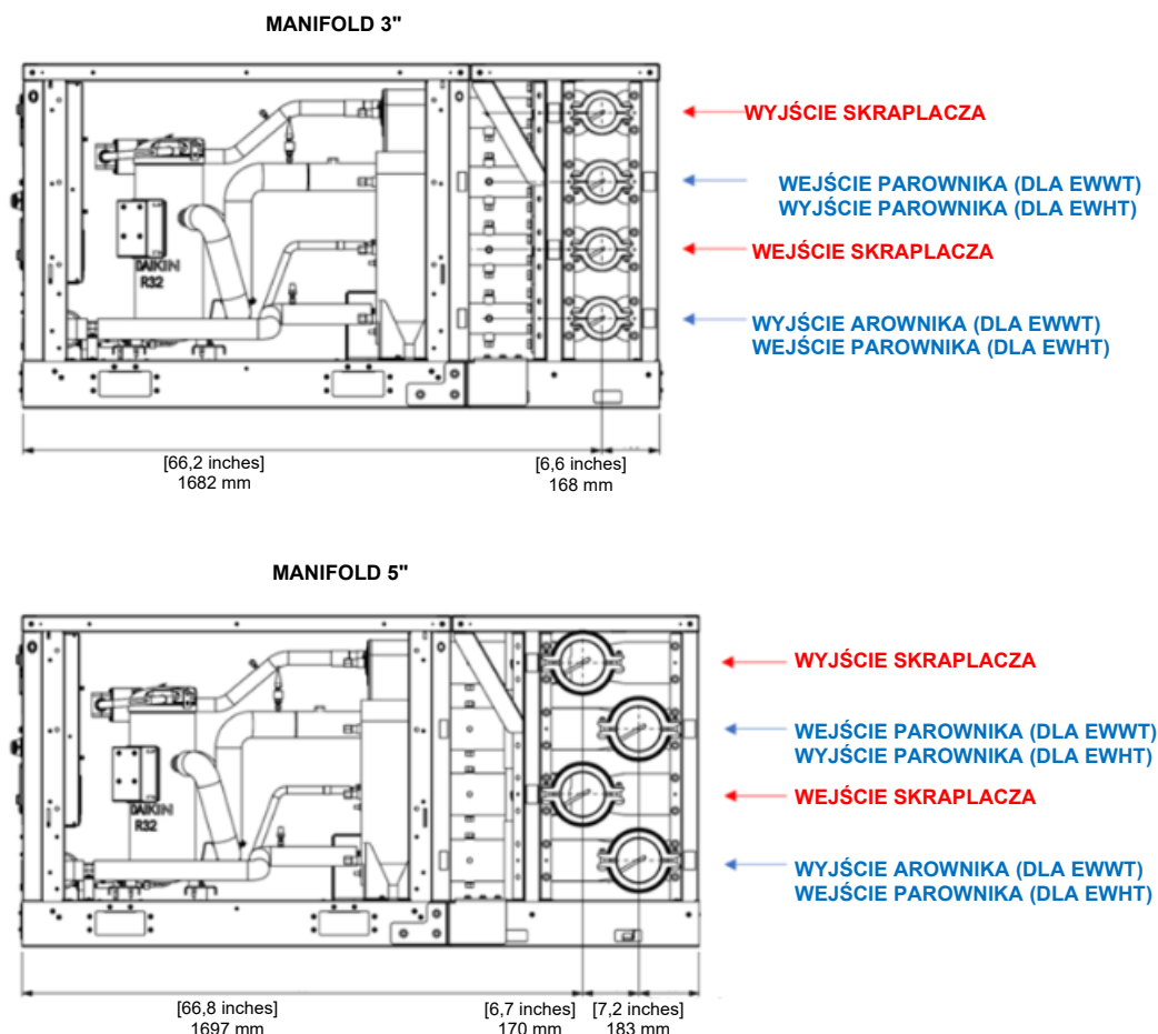
Rys. 30 – Rozmiary rozdzielaczy wody
