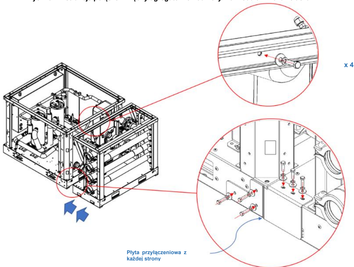
Rys. 26 – Instrukcje połączeń między agregatem chłodniczym a modułami rozdzielacza
