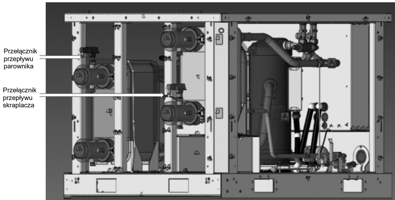
Rys. 16 – Prowadzenie kabli przełącznika przepływu parownika
