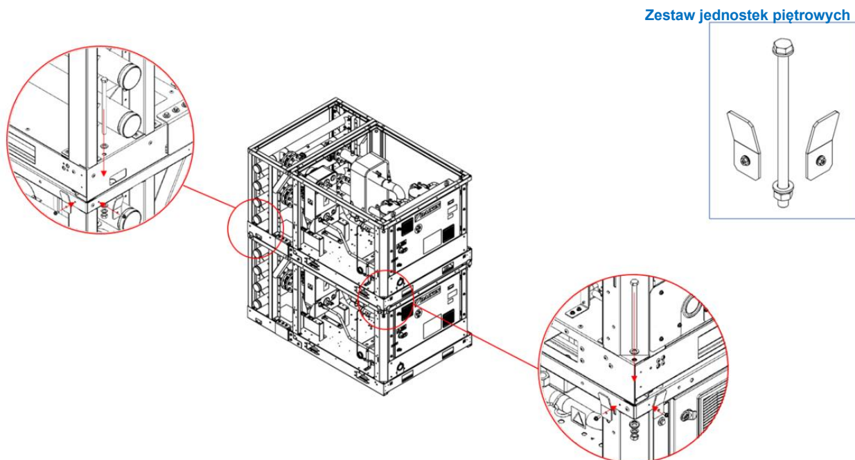
Rys. 43 – Instrukcje montażu jednostek piętrowych
