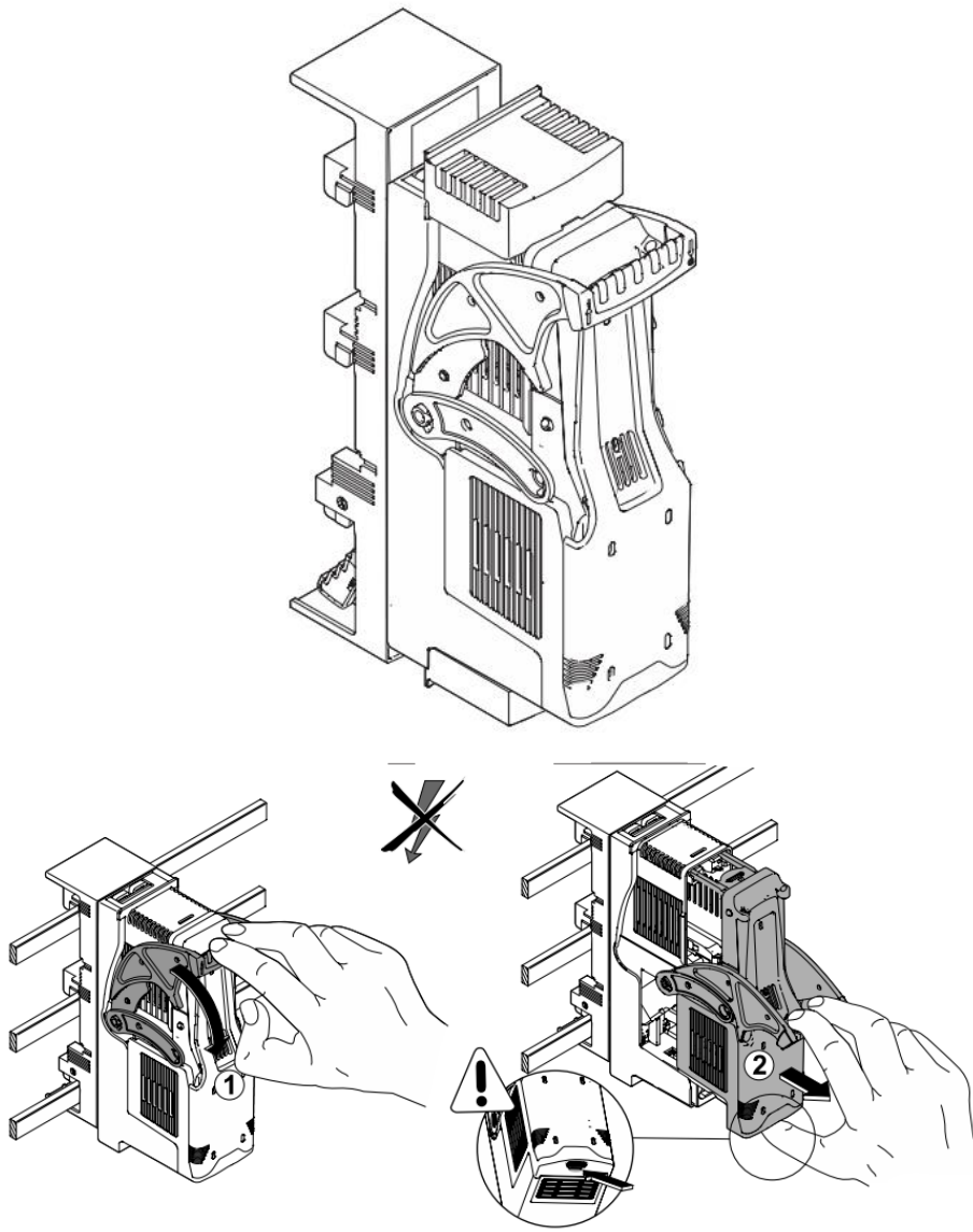
Rys. 61 – Rozłącznik bezpiecznikowy NH
