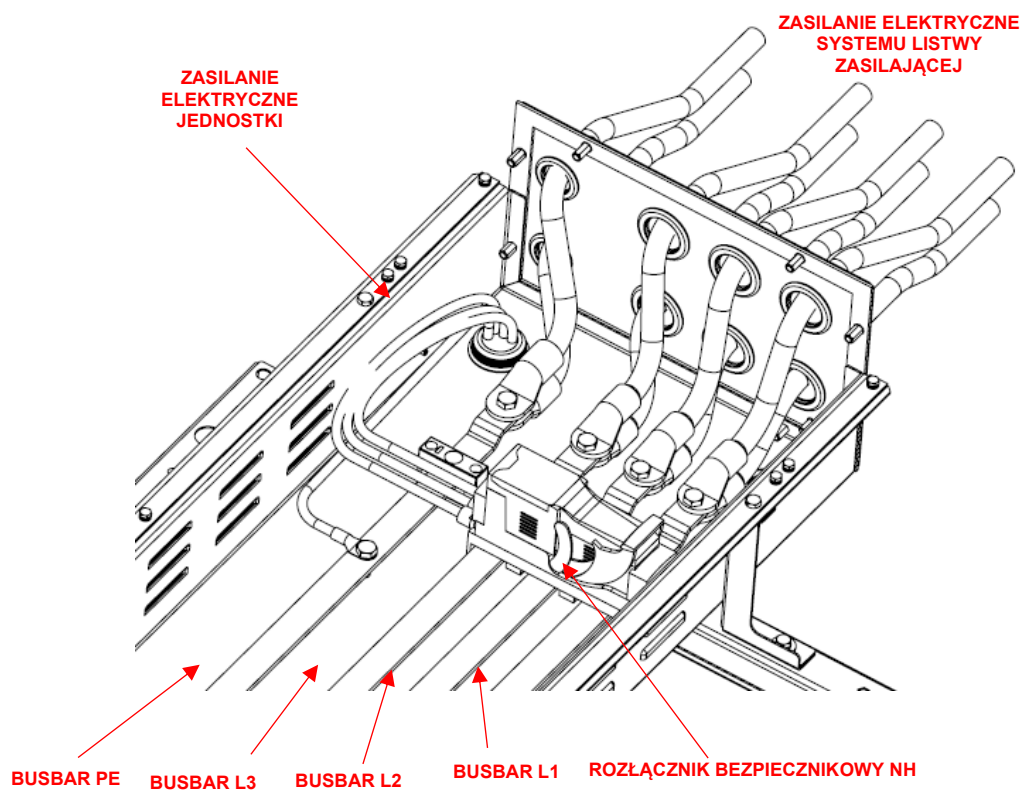
Rys. 59 – Szczegół połączenia elektrycznego dla modułu jednostki początkowej
