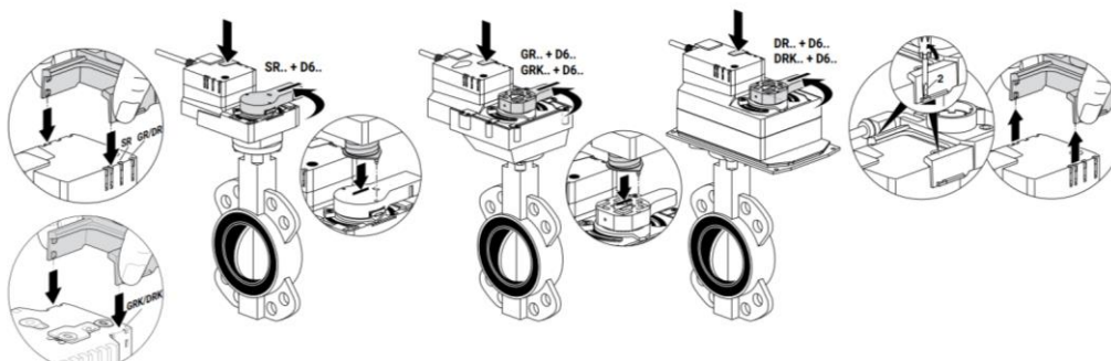
Rys. 33 – Instrukcje montażu wyłączników krańcowych silownika
