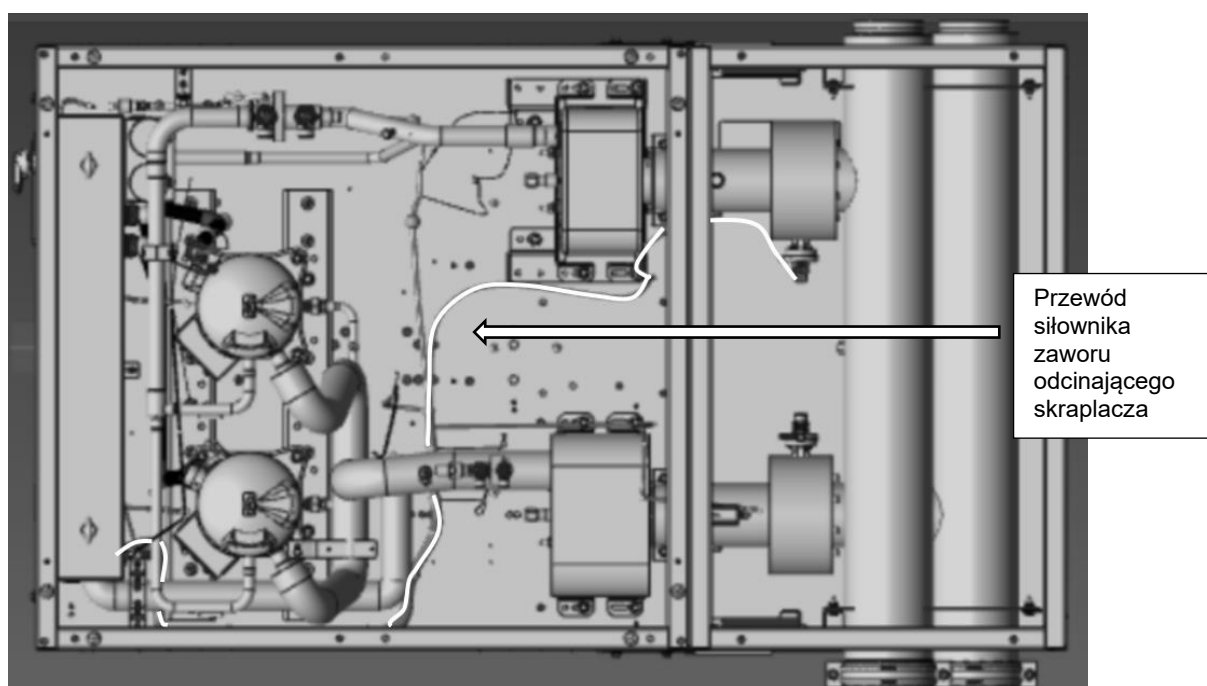
Rys. 40 – Prowadzenie kabla siłownika zaworu odcinającego skraplacza
