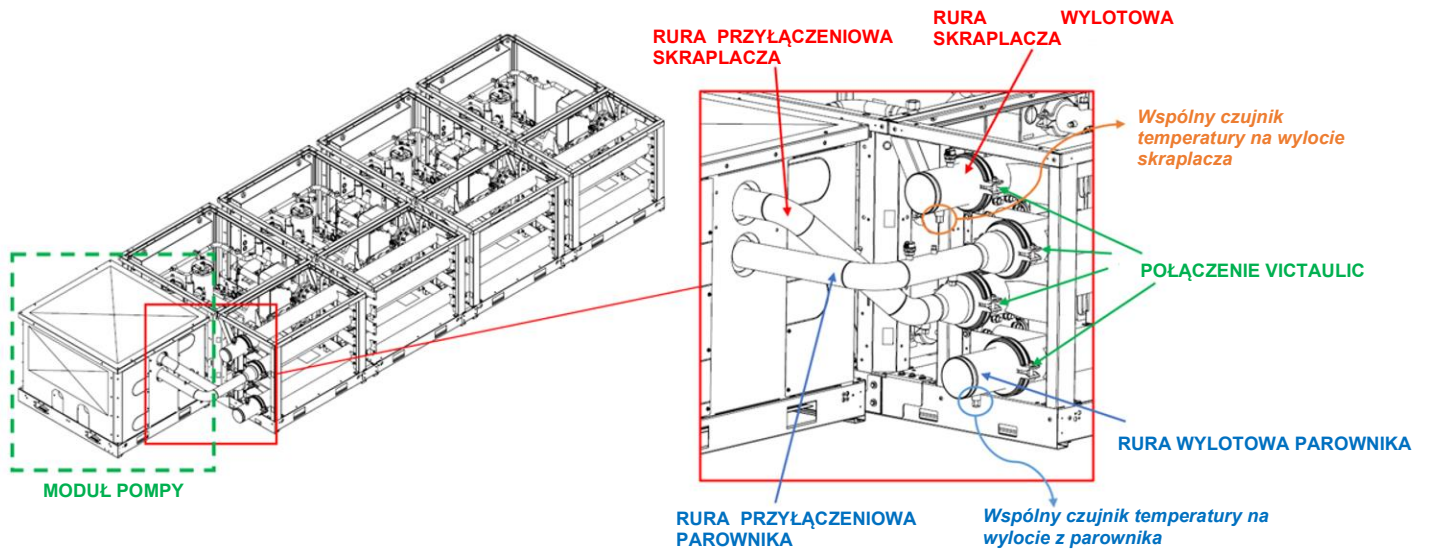
Rys. 63 – Szczegóły rozmieszczenia sond na rurach
