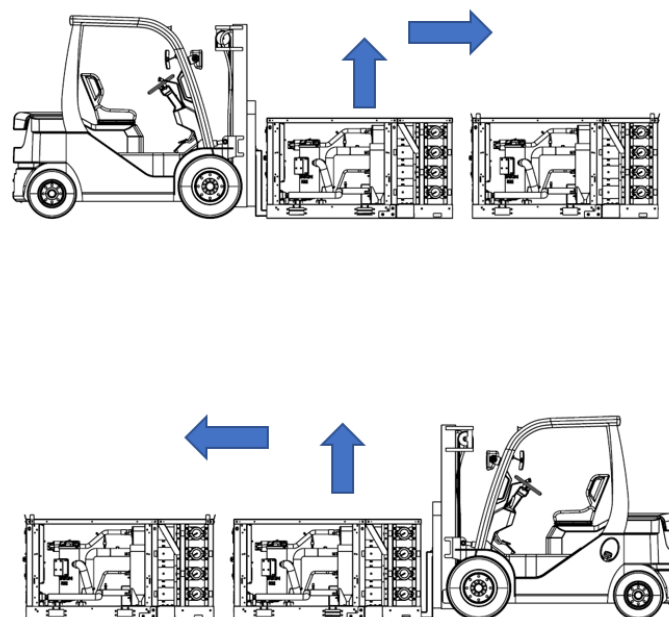
Rys. 50 – Obsługa modułu pompy za pomocą wózka widłowego
