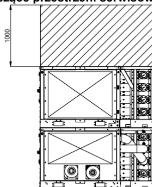
Rys. 10 - Wymagania dotyczące przestrzeni serwisowej dla konfiguracji piętrowej
