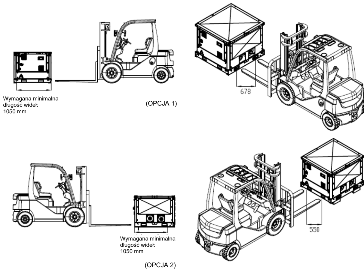
Rys. 50 – Obsługa modułu pompy za pomocą wózka widłowego
