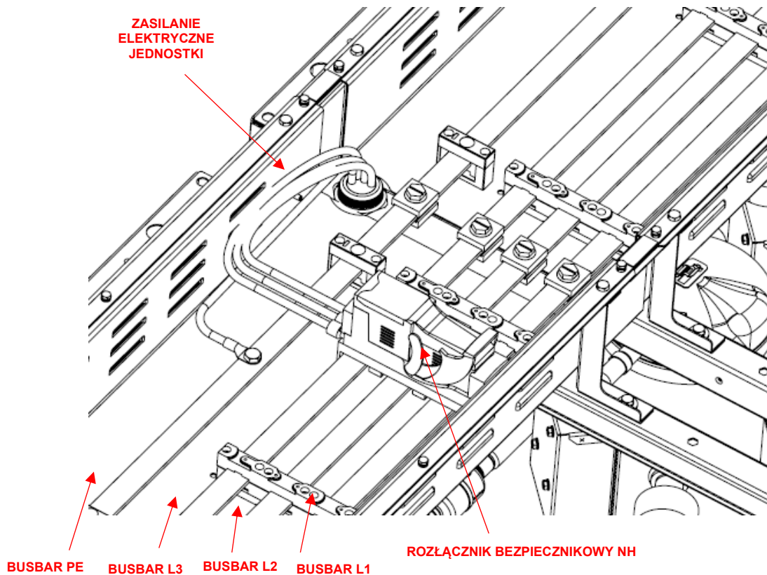
Rys. 60 – Szczegół połączenia elektrycznego dla dowolnego innego modułu urządzenia
