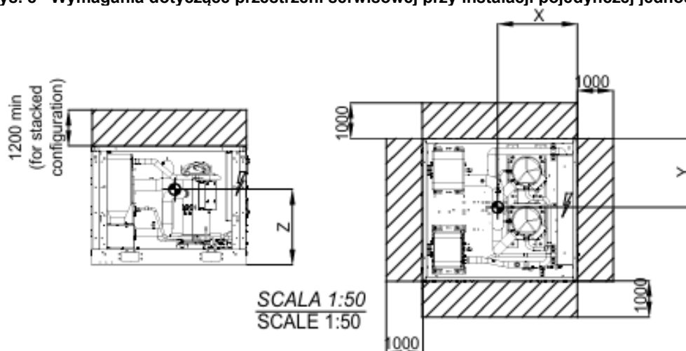
Rys. 8 –Wymagania dotyczące przestrzeni serwisowej przy instalacji pojedynczej jednostki
