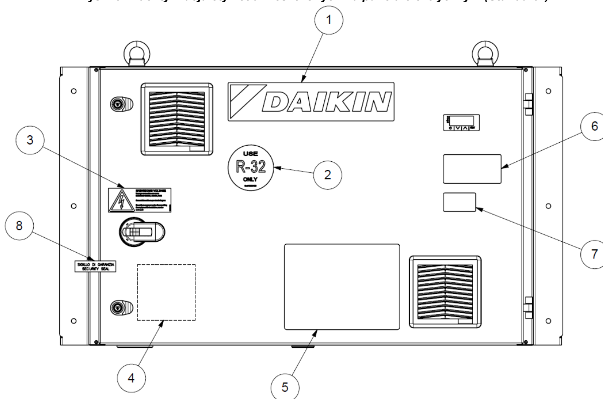
Rys. 25 – Identyfikacja etykiet umieszczonych na panelu elektrycznym (Standard*)
