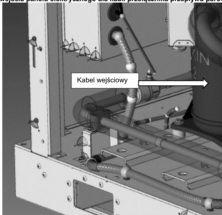
Rys. 18 – Punkt wejścia panelu elektrycznego dla kabli przełącznika przepływu parownika i skraplacza
