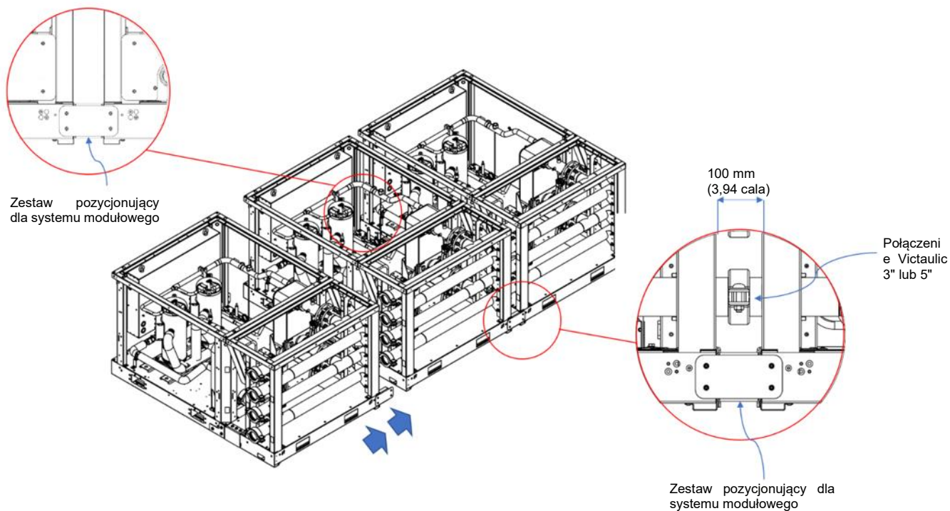
Rys. 29 – Połączenie systemów modułowych
