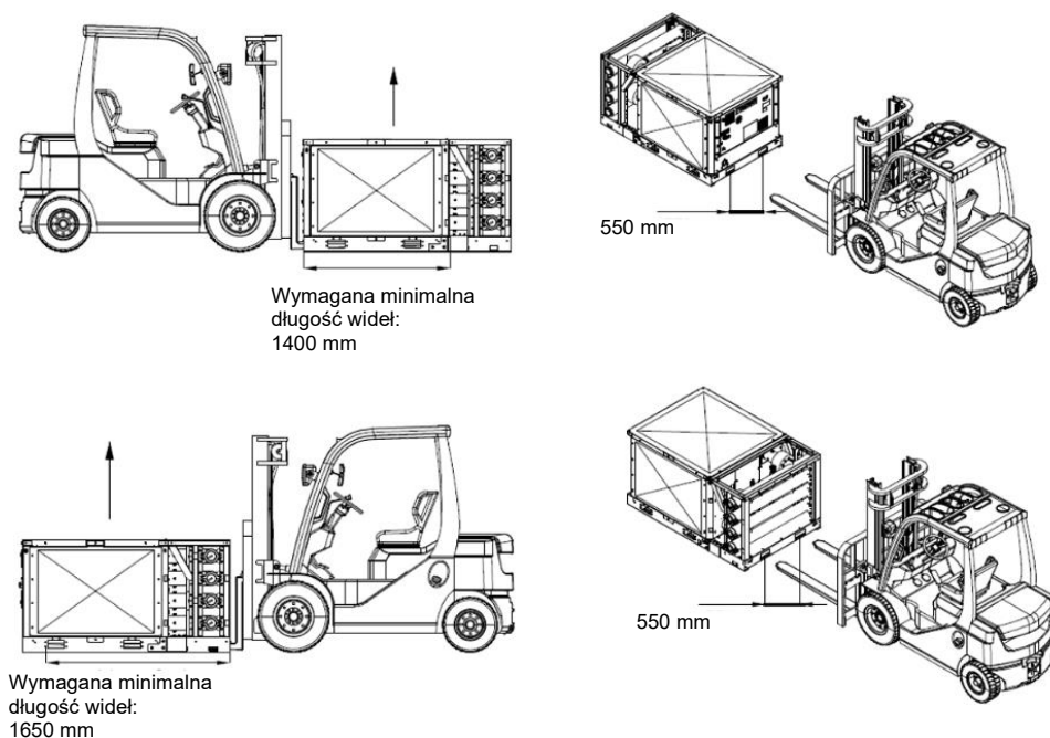
Rys. 48 – Obsługa modułów jednostki i rozdzielacza
