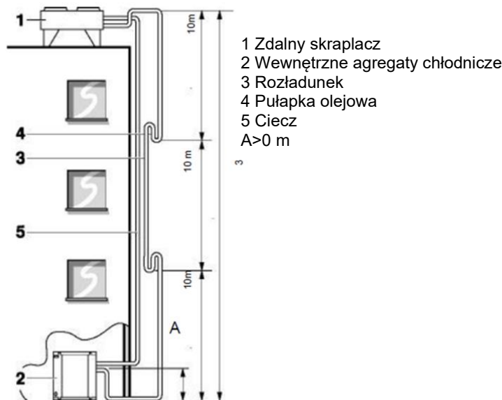
Rys. 20 – Podłączanie obiegu czynnika chłodniczego (1)
