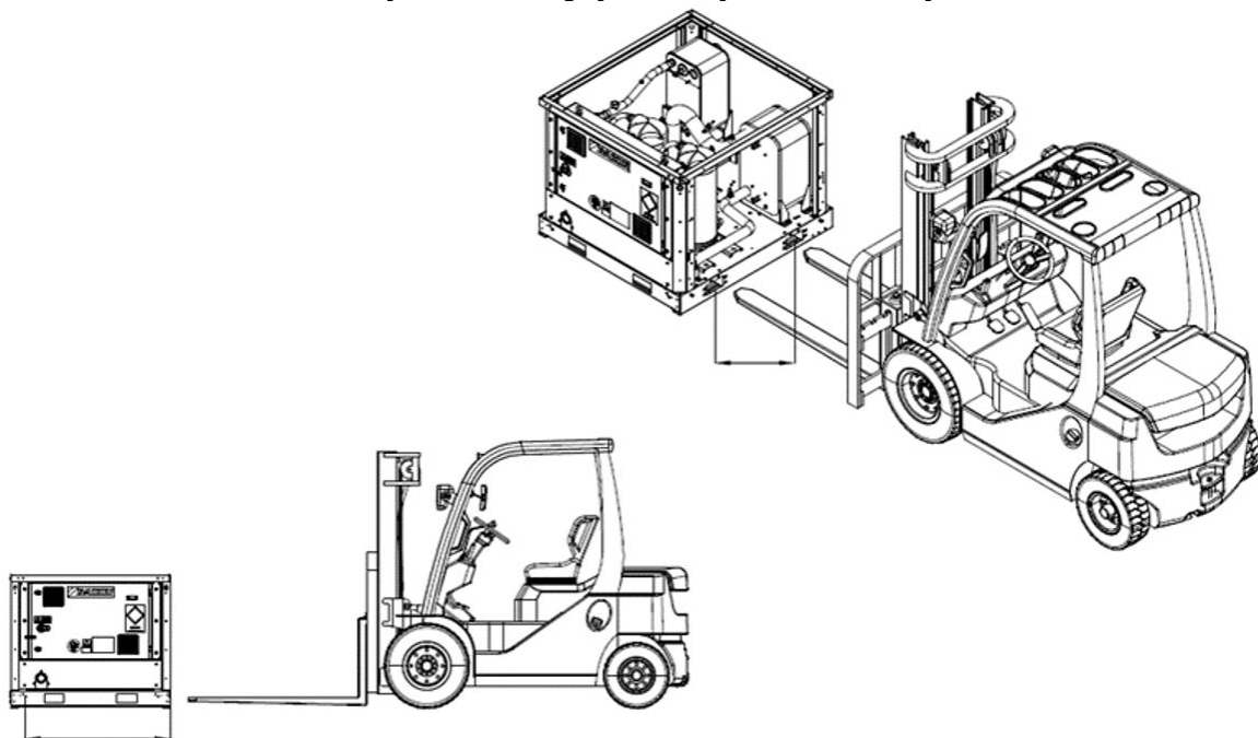
Rys. 11 – Obsługa jednostki jednoobwodowej
