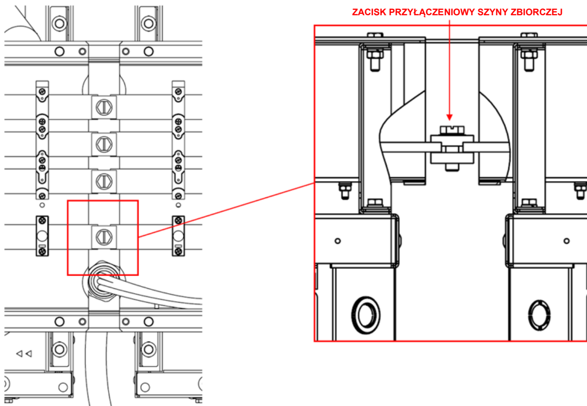
Rys. 57 – Szczegóły połączenia modułów listwy zasilającej
