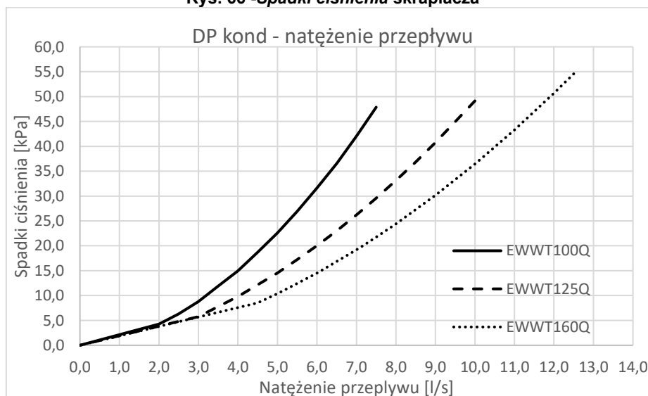
Rys. 66 - Spadki ciśnienia skraplacza
