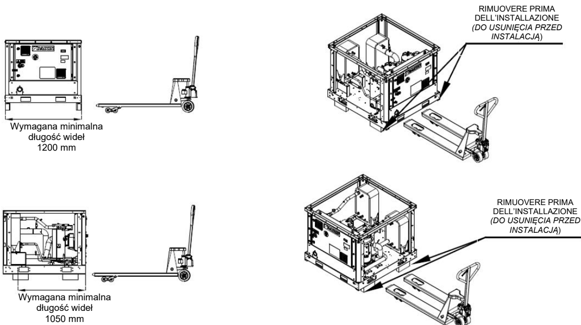
Rys. 13 – Alternatywna metoda obsługi za pomocą wózka paletowego
