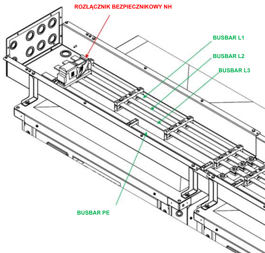
Rys. 58 – Szczegół bezpieczników i puszek do prowadzenia kabli modułu listwy zasilającej
