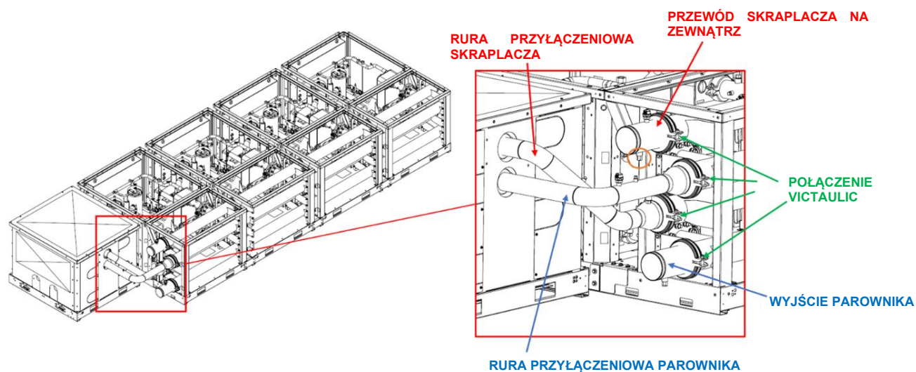
Rys. 46 – Instalacja modułu pompy – szczegóły orurowania
