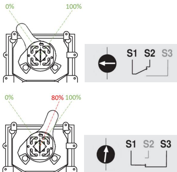
Rys. 42 – Ustawienie wyzwalacza wyłączników krańcowych
