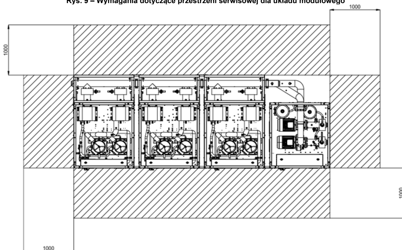
Rys. 9 – Wymagania dotyczące przestrzeni serwisowej dla układu modułowego
