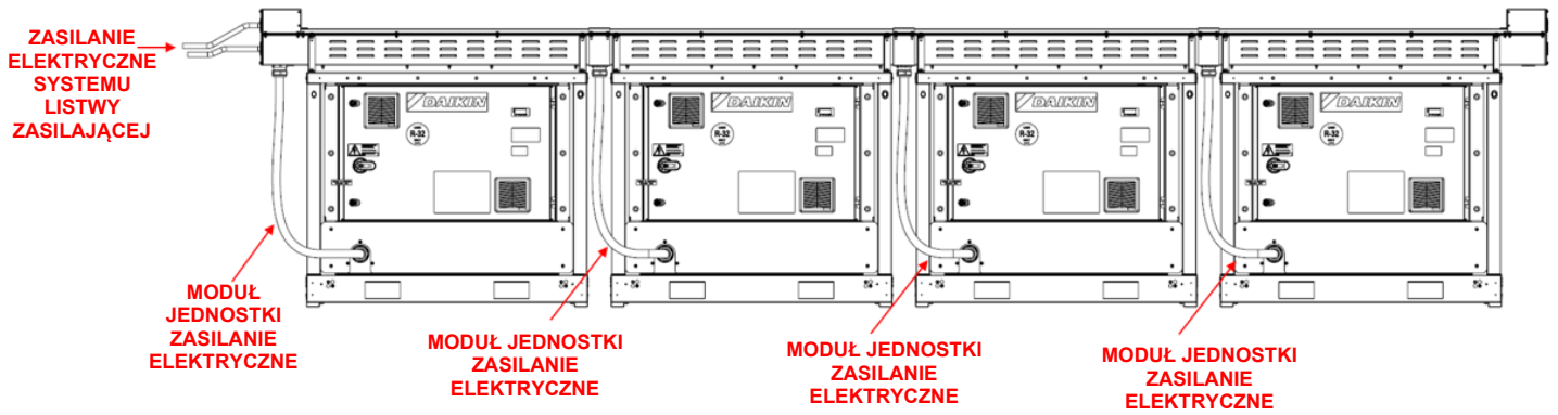
Rys. 54 – Szczegóły prowadzenia kabli
