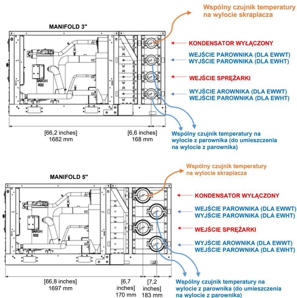
Rys. 62 – Położenie sond temperatury dla rozdzielacza 3" i 5"
