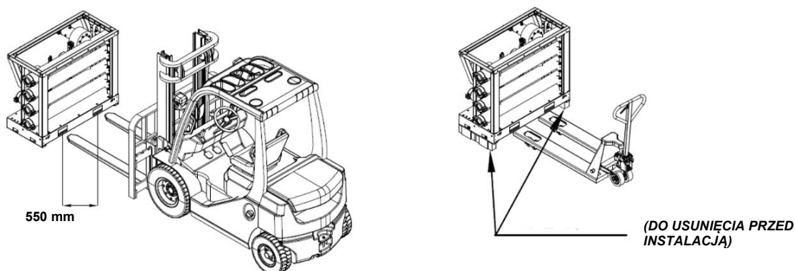
Rys. 47 – Obsługa modułu rozdzielacza
