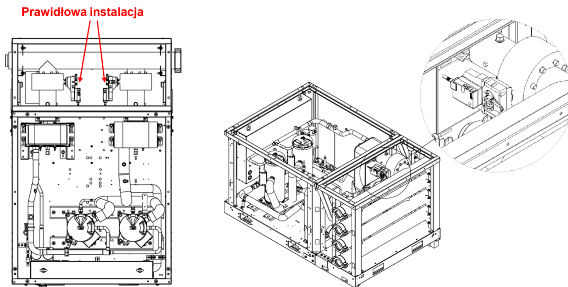
Rys. 34 – Wskazówki dotyczące montażu siłownika zaworu
