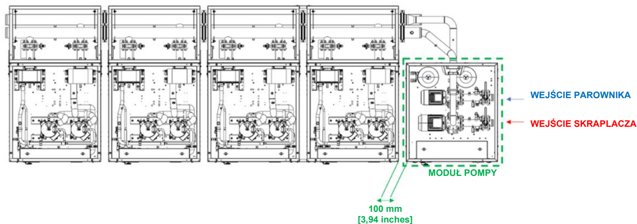
Rys. 46 – Instalacja modułu pompy – szczegóły orurowania
