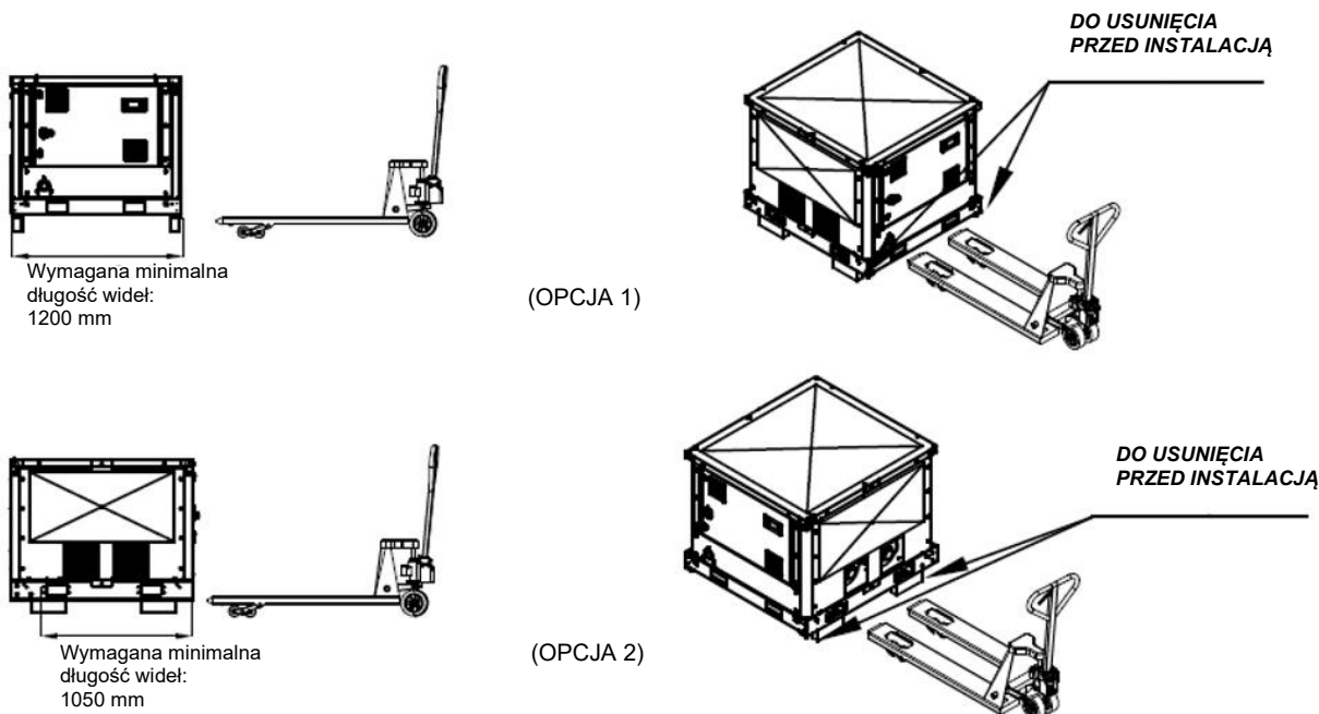
Rys. 51 – Obsługa modułu pompy za pomocą wózka paletowego
