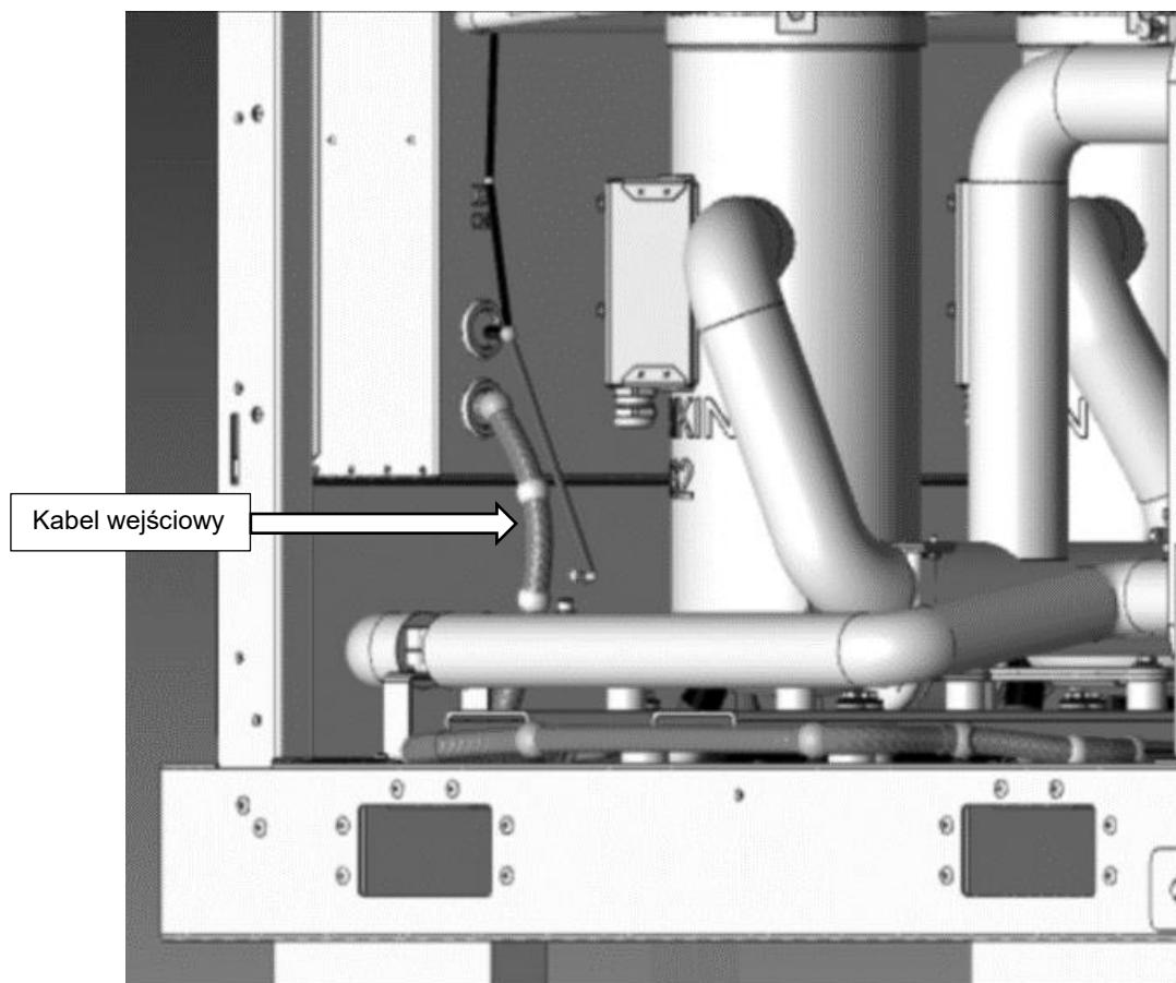
Rys. 41 – Wejście panelu elektrycznego dla przewodów siłownika zaworu odcinającego parownika i skraplacza
