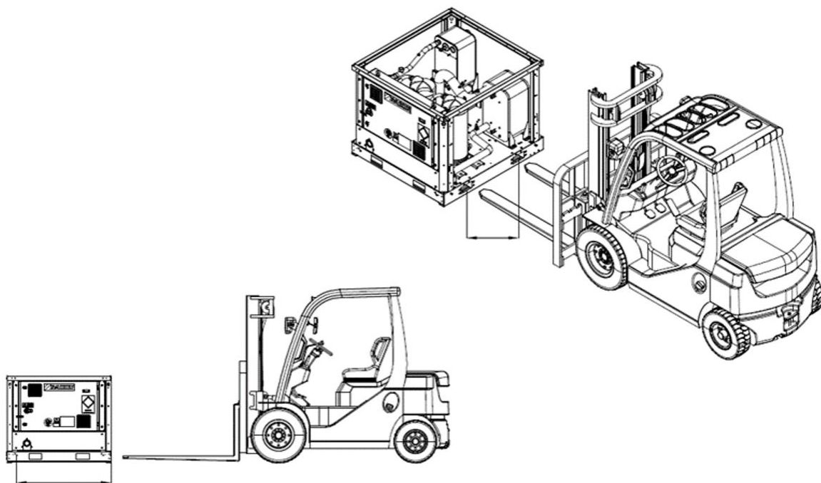
Fig. 11 - Manipolazione dell'unità a circuito singolo
