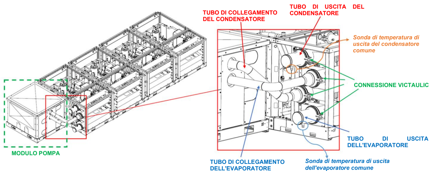
Fig. 63 - Dettagli del posizionamento delle sonde sui tubi
