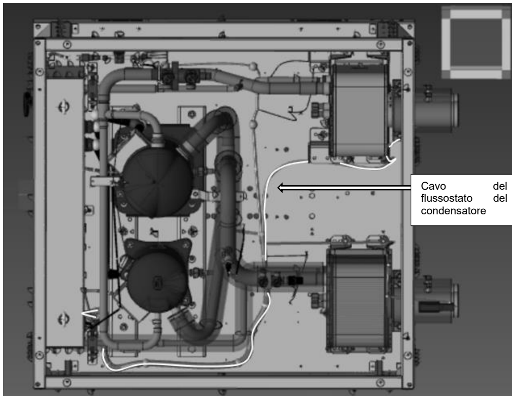
Fig. 18 - Punto di ingresso del pannello elettrico per i cavi del flussostato dell'evaporatore e del condensatore
