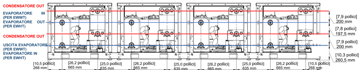
Fig. 28 - Configurazione delle tubazioni dell'acqua
