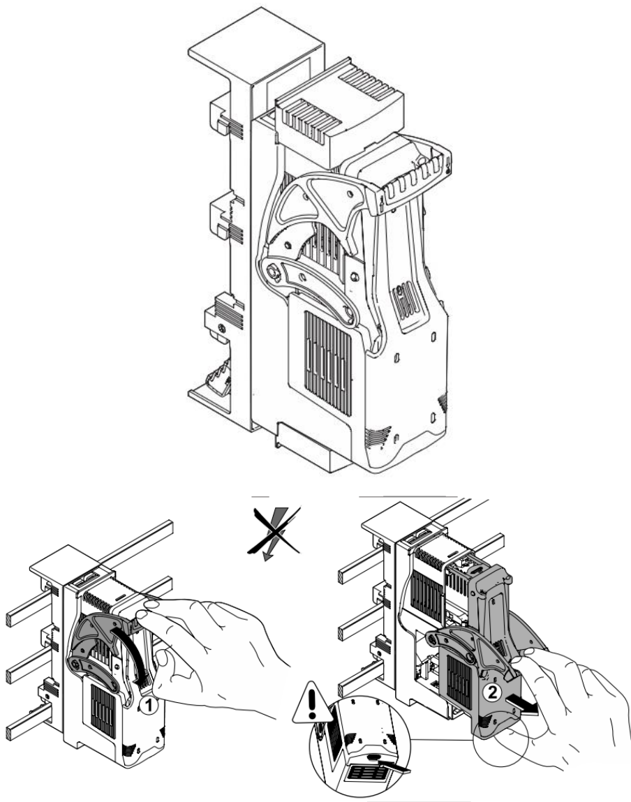
Fig. 61 - Sezionatore con fusibile NH
