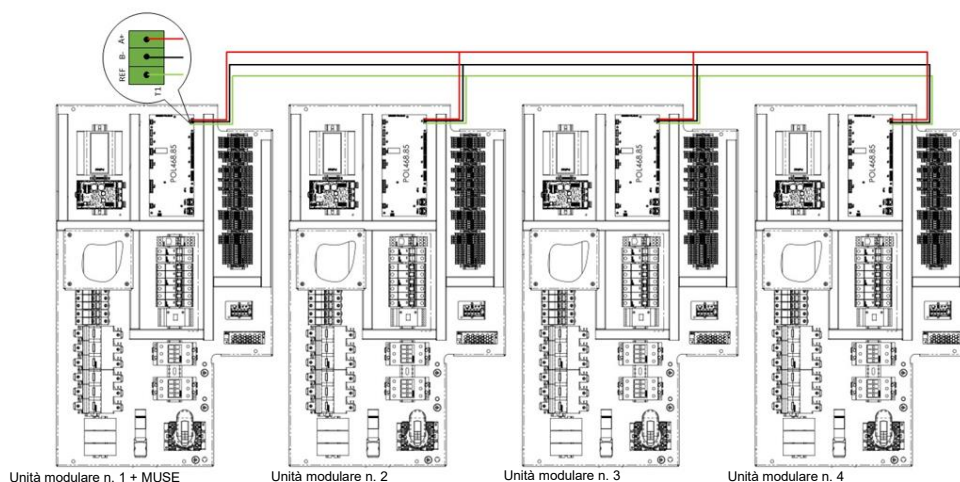
Fig. 64 - Collegamento di 4 PLC sulla stessa rete Modbus
