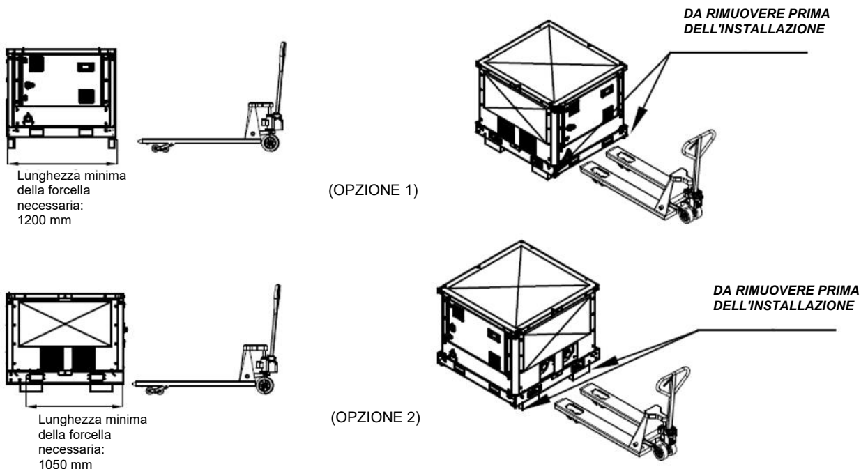
Fig. 51 - Movimentazione del modulo pompa con transpallet
