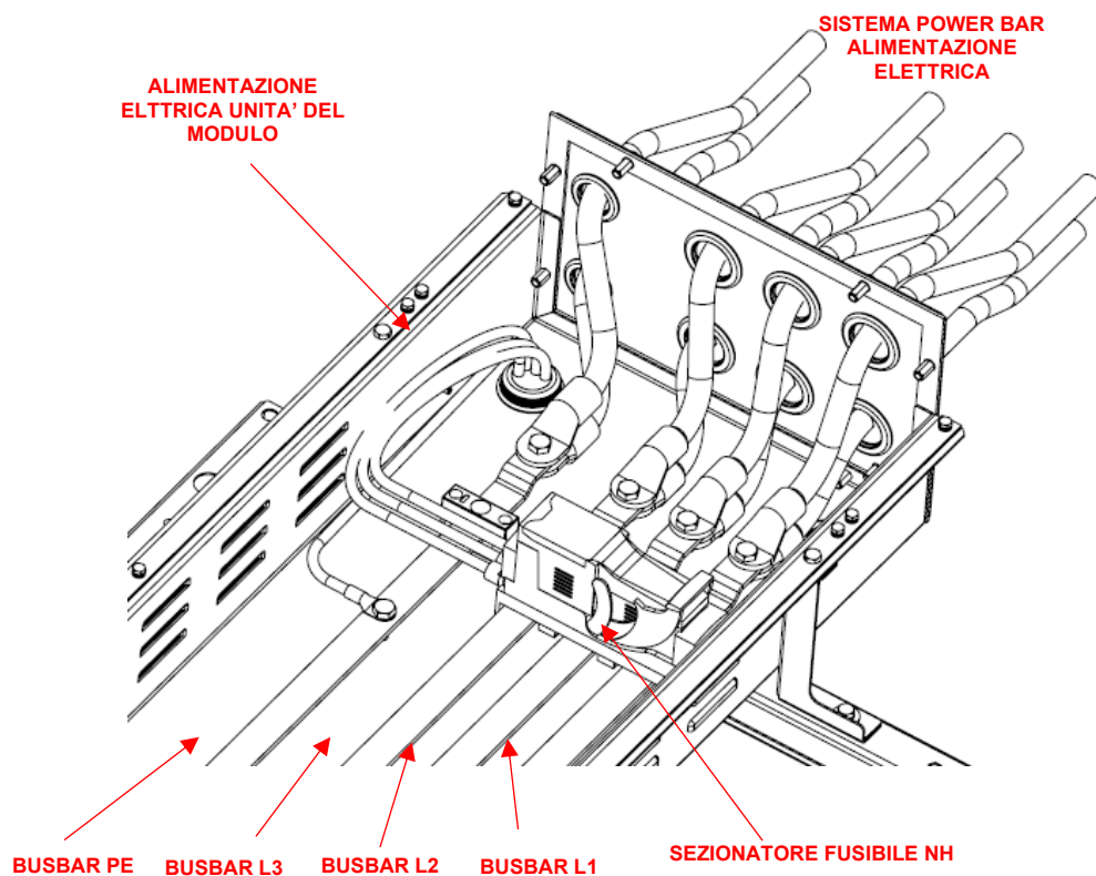
Fig. 59 - Dettaglio del collegamento elettrico del modulo iniziale dell'unità
