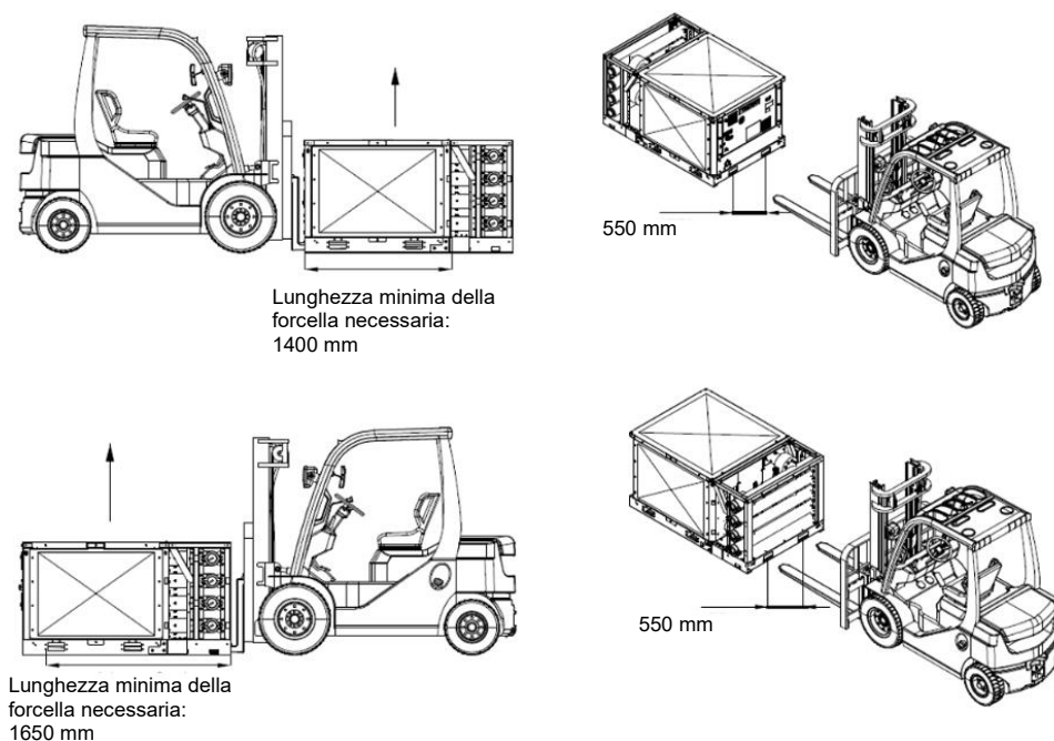
Fig. 48 - Movimentazione dei moduli dell'unità e del collettore
