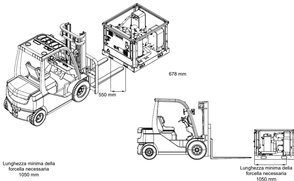
Fig. 12 - Metodo di movimentazione alternativo con carrello elevatore
