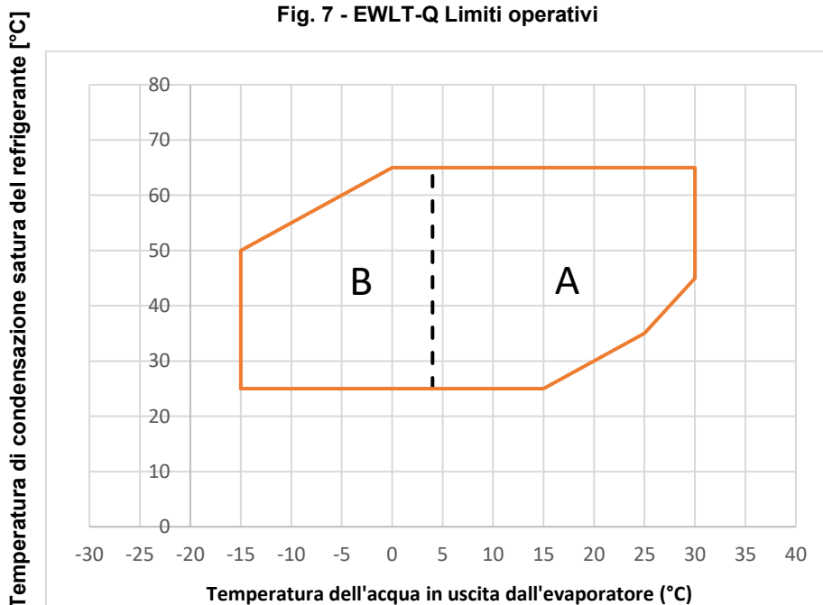
Fig. 7 - EWLT-Q Limiti operativi
