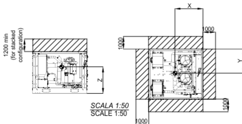
Fig. 9 – Requisiti di spazio per la manutenzione - installazione modulare-array
