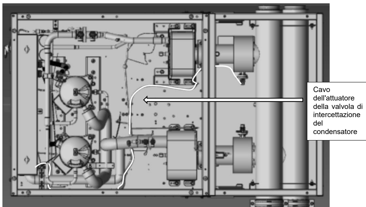
Fig. 40 - Passaggio del cavo dell'attuatore della valvola di intercettazione del condensatore
