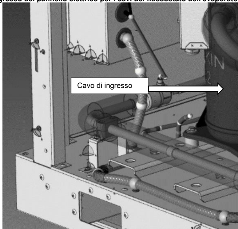
Fig. 18 - Punto di ingresso del pannello elettrico per i cavi del flussostato dell'evaporatore e del condensatore
