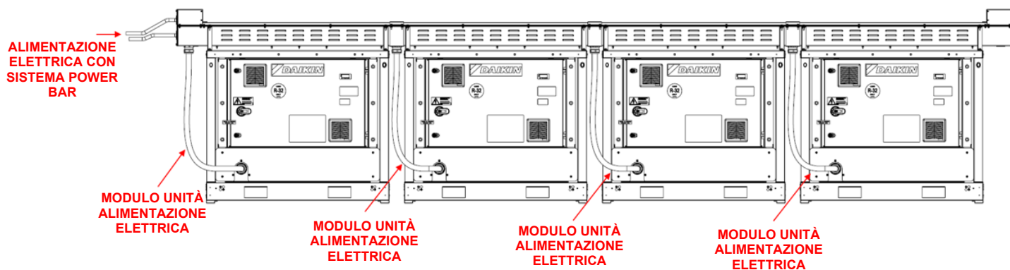
Fig. 54 - Dettagli della posa dei cavi
