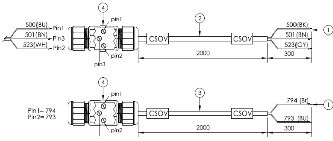
Fig. 38 - Schema di cablaggio dell'attuatore della valvola di intercettazione
