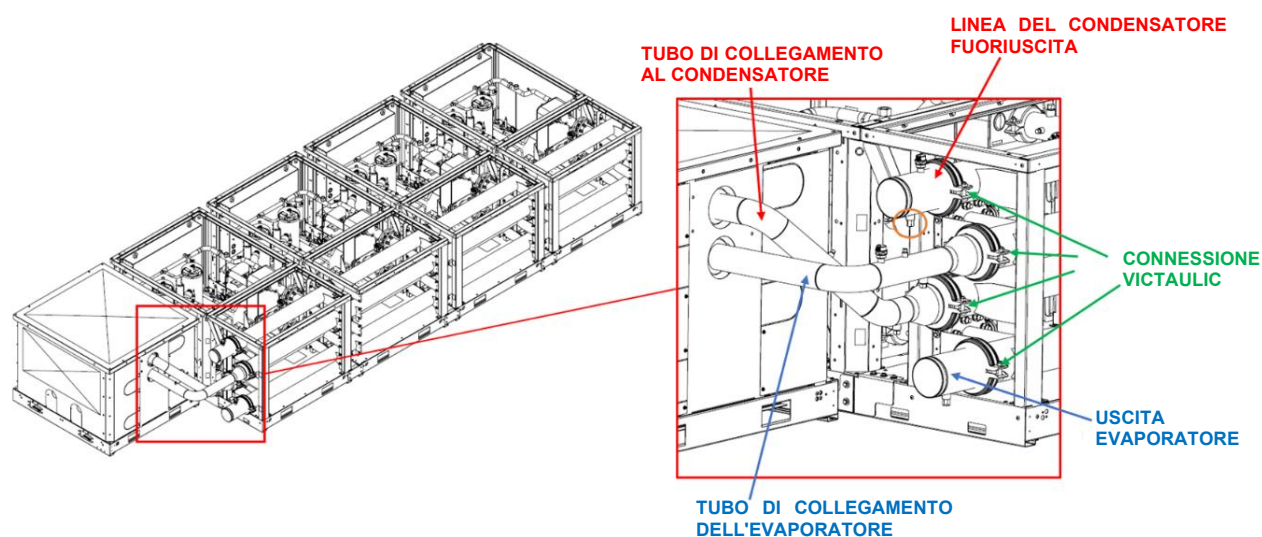
Fig. 46 - Installazione del modulo pompa - dettagli delle tubazioni
