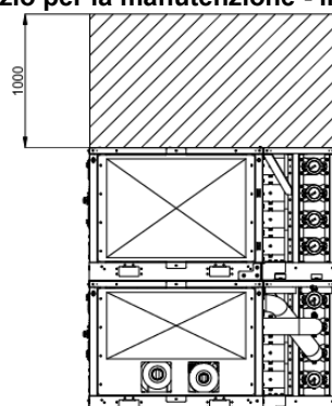
Fig. 10 - Requisiti di spazio per la manutenzione - installazione unità impilate
