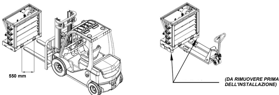
Fig. 47 - Manipolazione del modulo manifold
