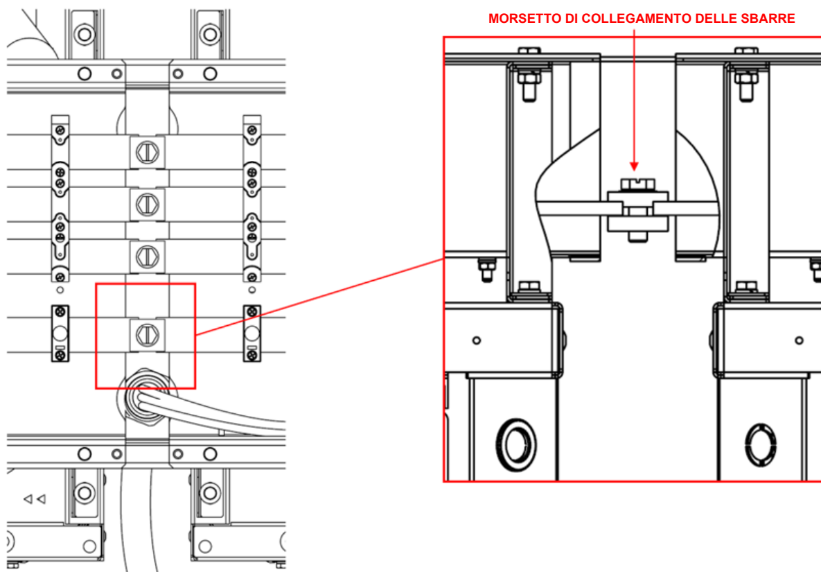
Fig. 57 - Dettagli del collegamento dei moduli della barra di potenza tra loro
