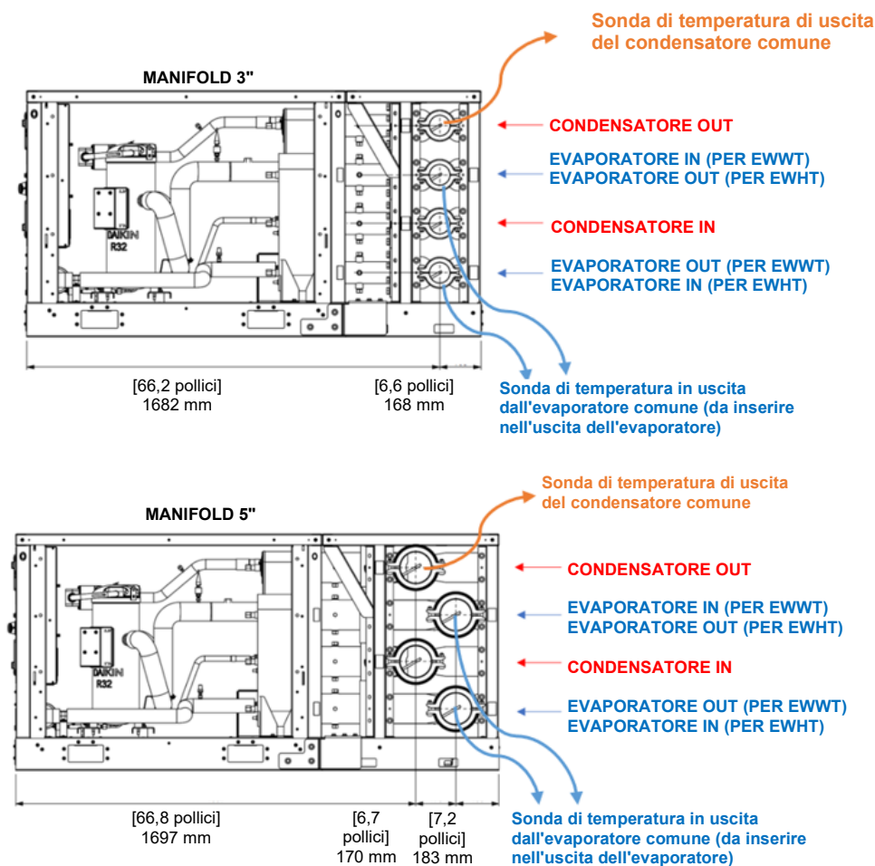
Fig. 62 - Posizioni delle sonde di temperatura per collettori da 3" e 5"
