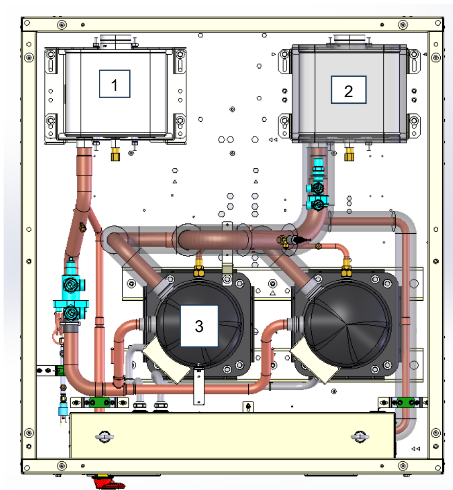
Fig. 14 - Disegno di riferimento per l'identificazione dell'evaporatore e del condensatore
