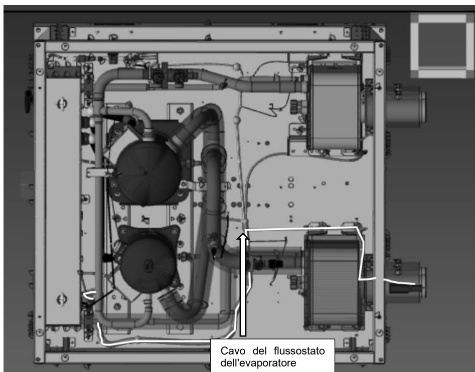
Fig. 16 - Percorso dei cavi del flussostato dell'evaporatore
