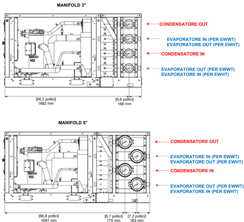
Fig. 30 - Dimensioni del collettore dell'acqua
