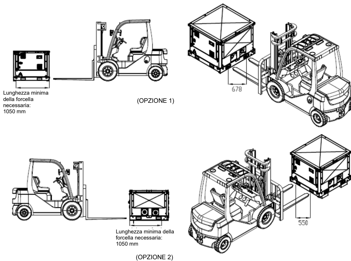
Fig. 50 - Movimentazione del modulo pompa con carrello elevatore
