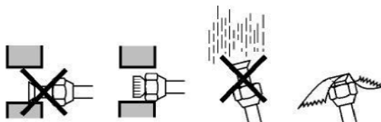
Fig. 21 - Collegamento del circuito del refrigerante (4)
