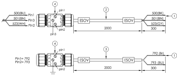
Fig. 37 - Adattatori per cavi per l'attuatore della valvola di intercettazione del condensatore e per i finecorsa
