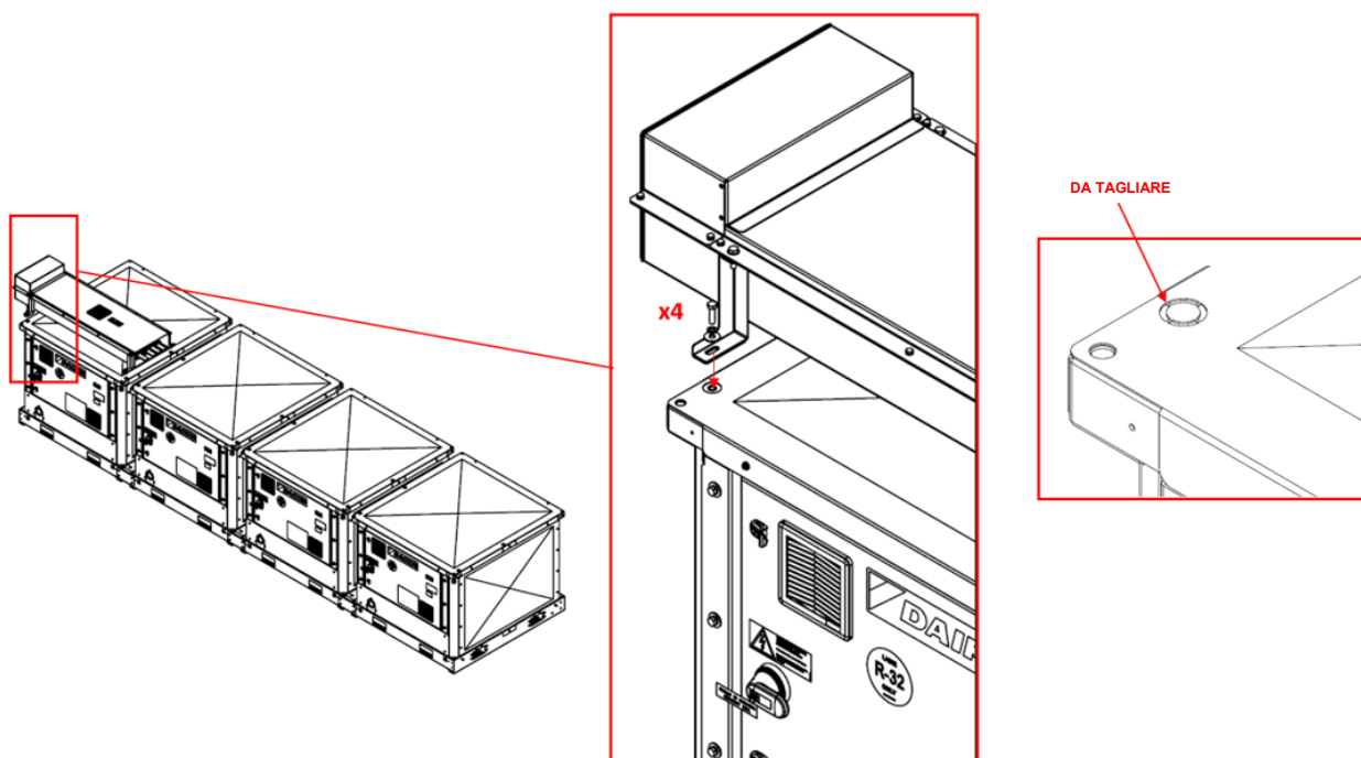
Fig. 55 - Fissaggio del sistema di barre di alimentazione all'unità
