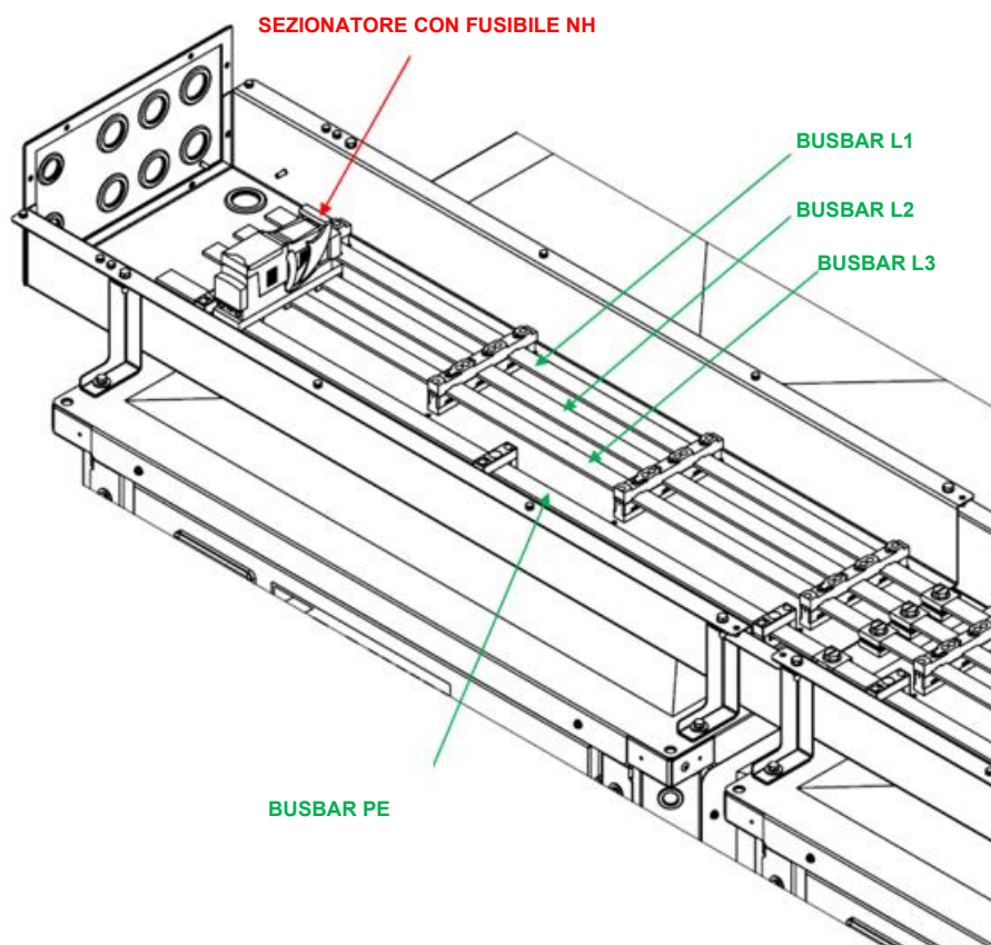
Fig. 58 - Dettaglio dei fusibili e della scatola per il passaggio dei cavi del modulo della barra di alimentazione
