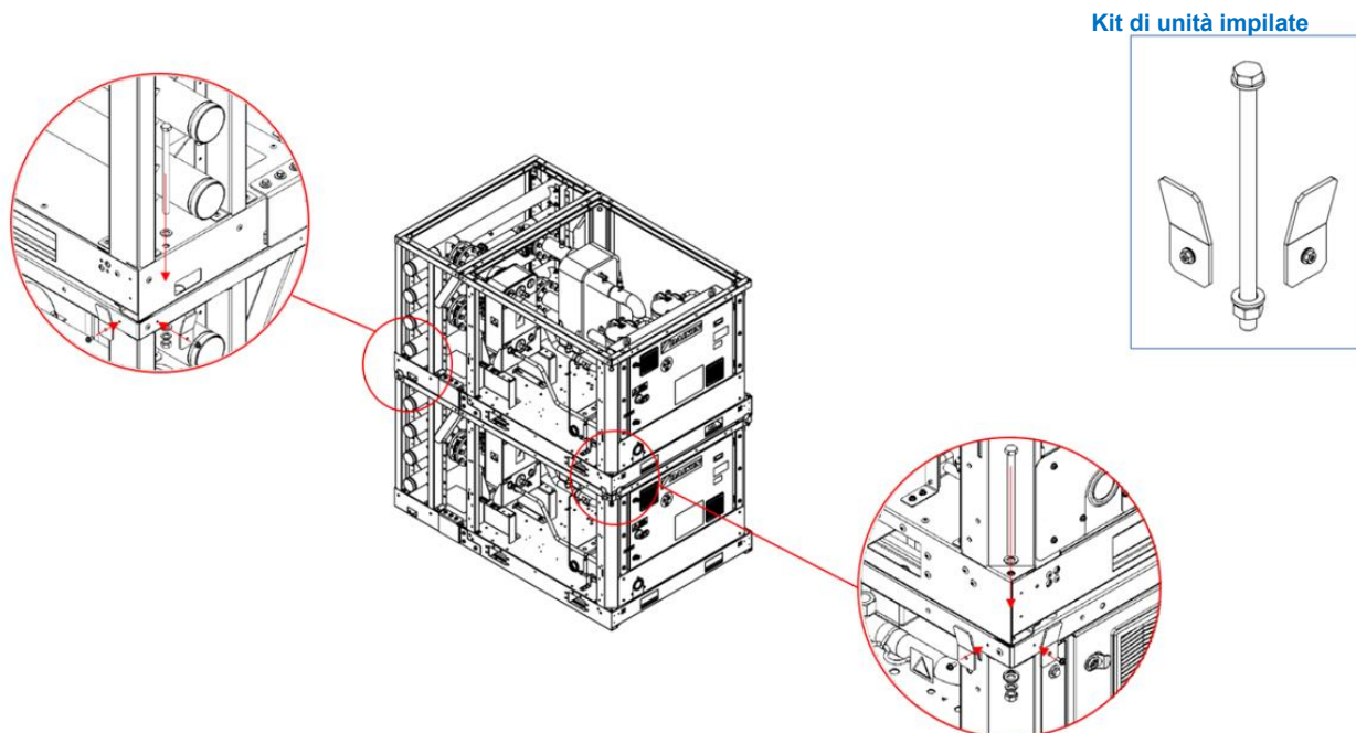
Fig. 43 - Istruzioni di montaggio per unità impilate
