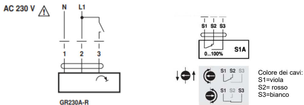
Fig. 35 - Schema di cablaggio del motore (figura a sinistra) e dei finecorsa (figura a destra)
