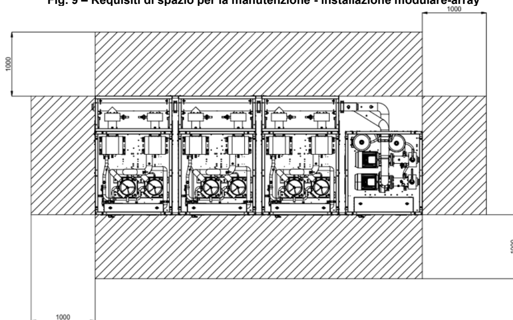
Fig. 9 – Requisiti di spazio per la manutenzione - installazione modulare-array
