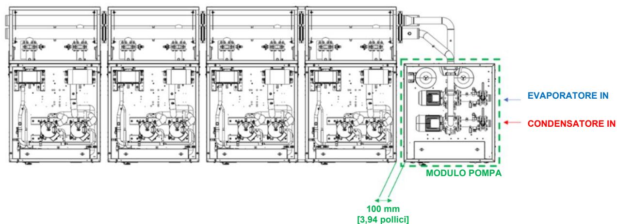
Fig. 46 - Installazione del modulo pompa - dettagli delle tubazioni
