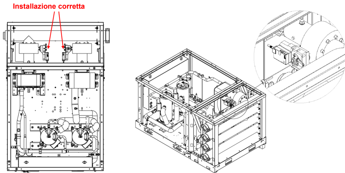
Fig. 34 - Indicazioni di montaggio per l'attuatore della valvola
