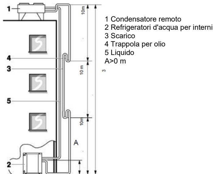
Fig. 20 - Collegamento del circuito frigorifero (1)
