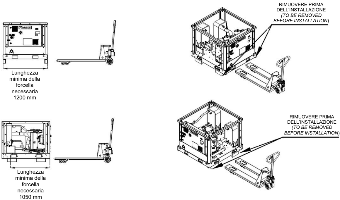
Fig. 13 - Metodo di movimentazione alternativo con transpallet
