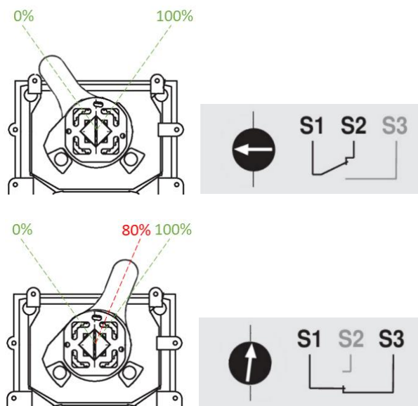
Fig. 42 - Impostazione dell'attivazione dei finecorsa
