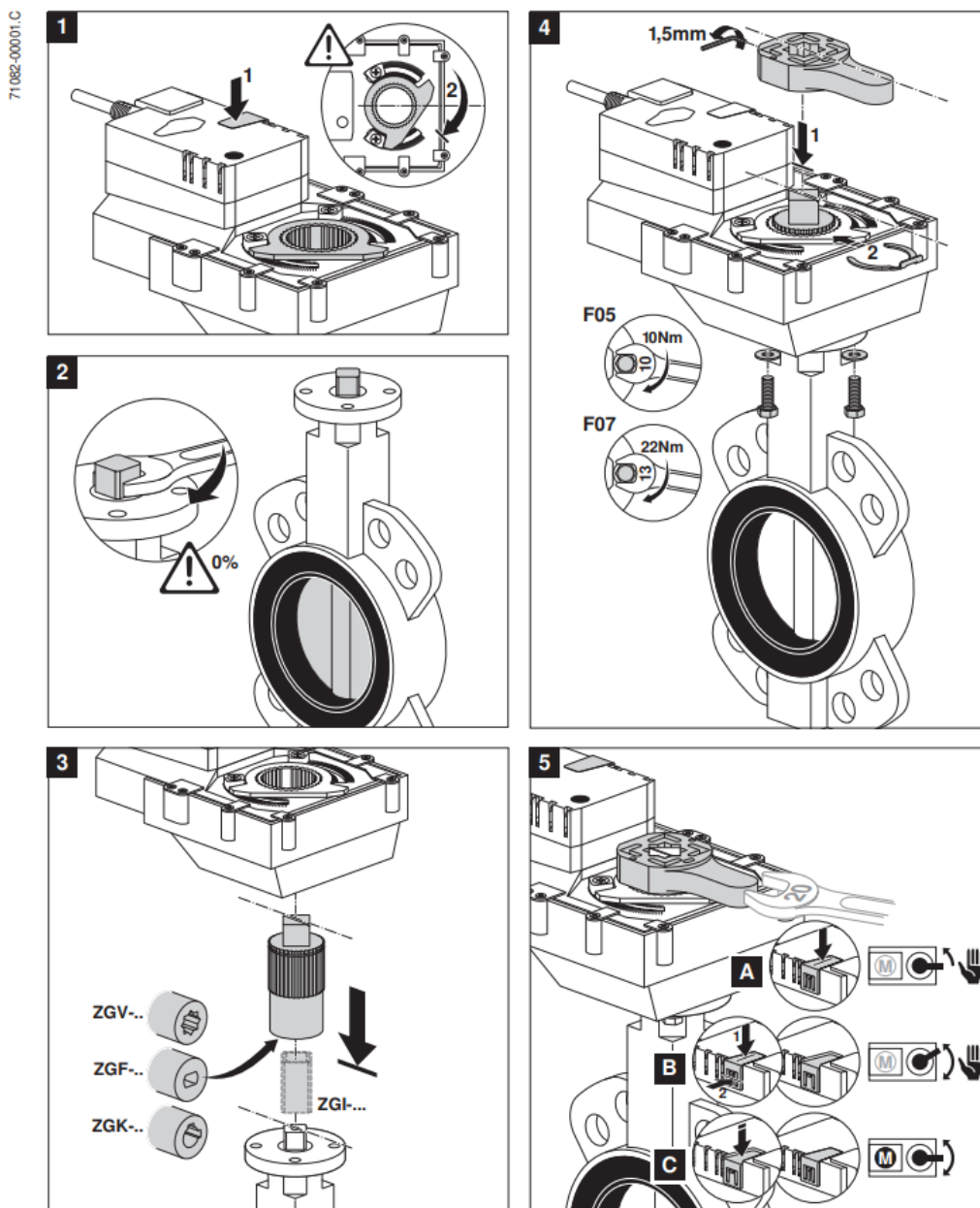
Fig. 32 - Istruzioni di montaggio per l'attuatore della valvola
