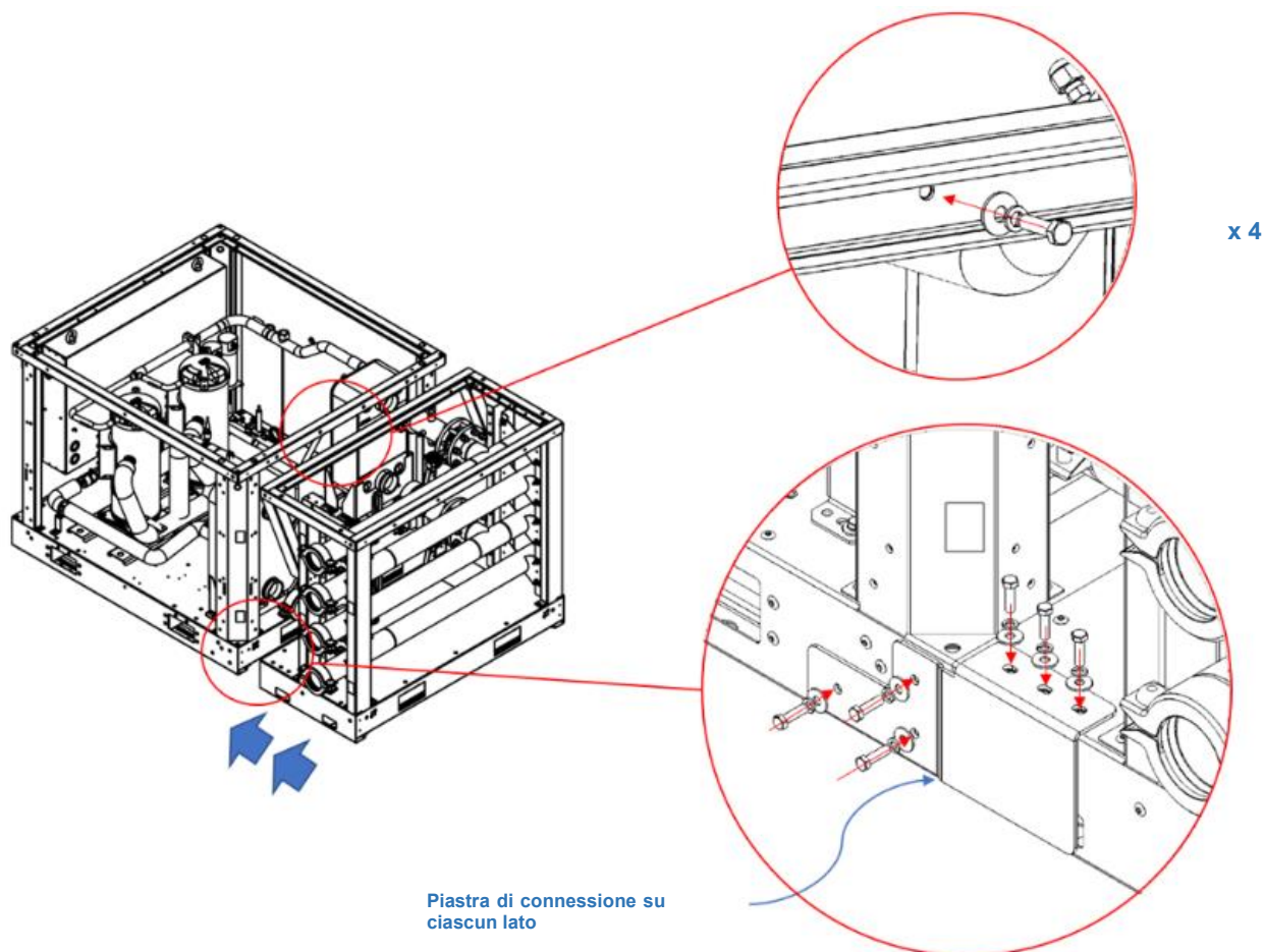
Fig. 26 - Istruzioni per il collegamento tra i moduli refrigeratori e manifold
