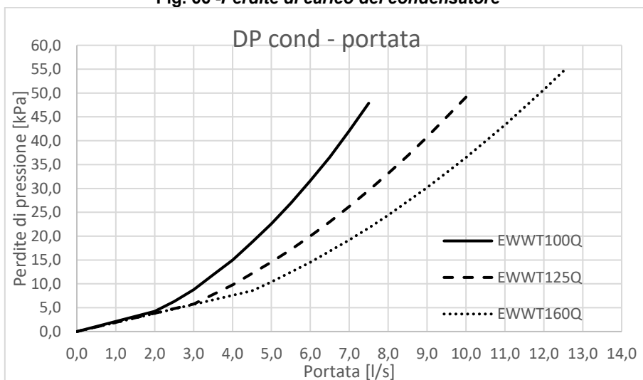
Fig. 66 - Perdite di carico del condensatore
