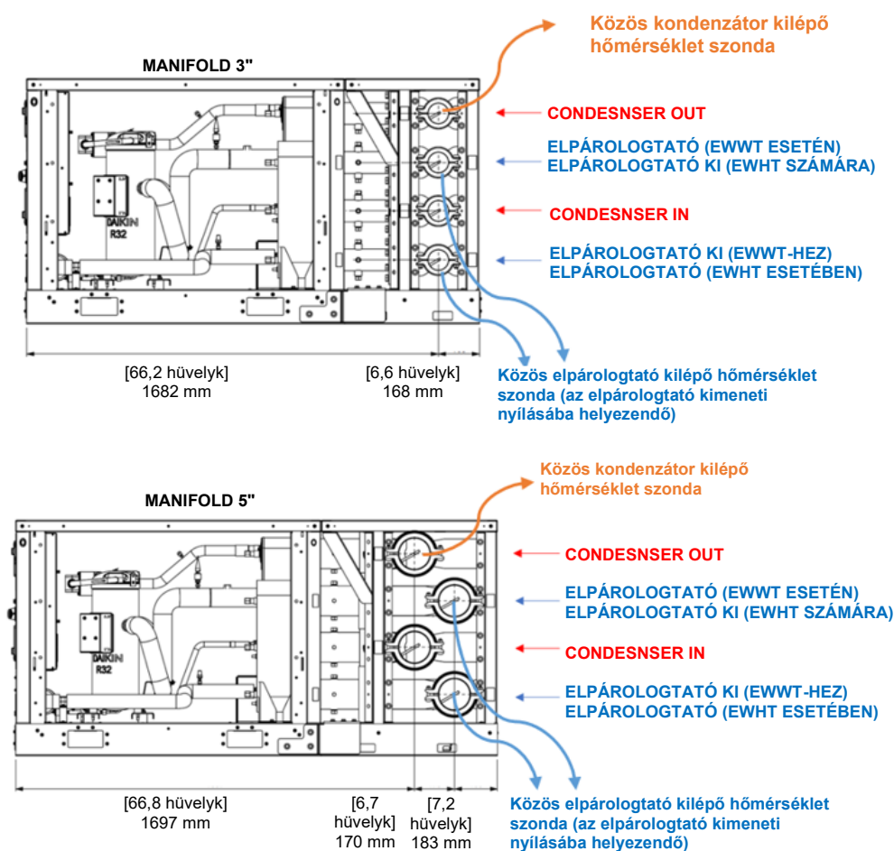
62. ábra - A hőmérséklet-szondák helyzete a 3" és 5" gyűjtőcsőhöz
