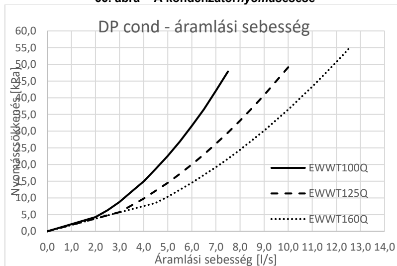
66. ábra - A kondenzátor nyomásesése
