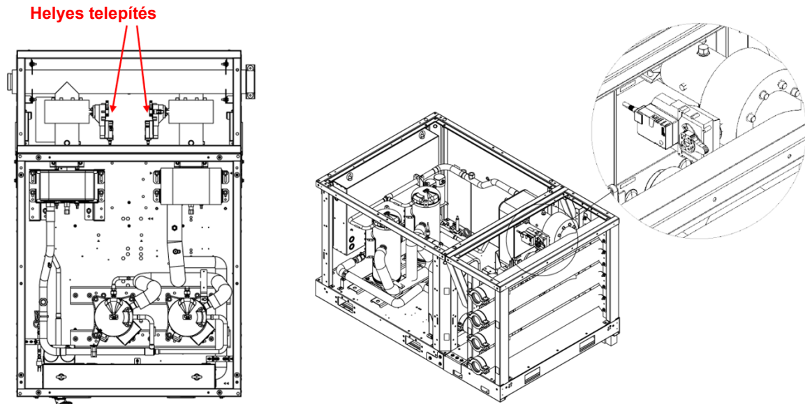
34. ábra - A szelepmeghajtás szerelési jelzései
