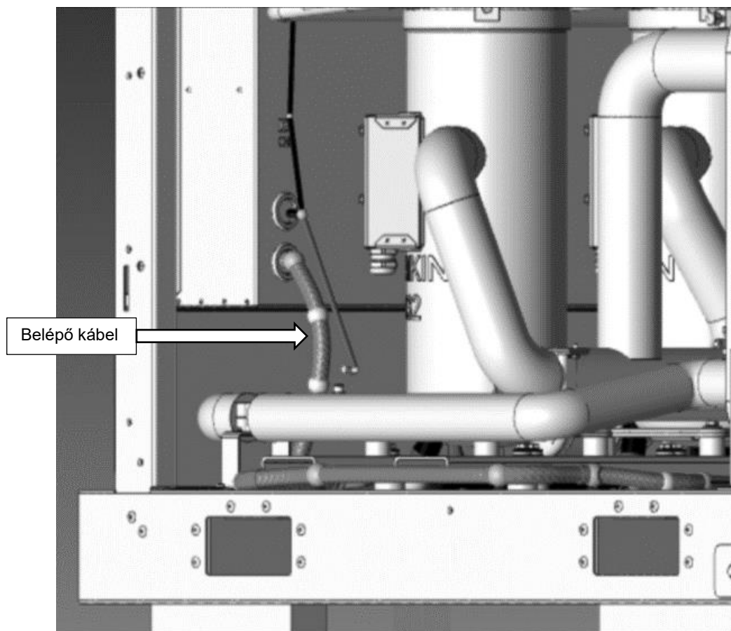
41. ábra - Az elpárologtató és a kondenzátor elzárószelep működtetőszelepének kábeleinek elektromos panelbejárata
