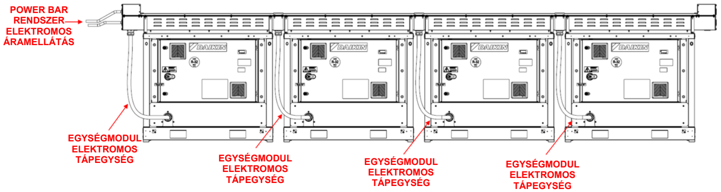
54. ábra - A kábelek elvezetésének részletei
