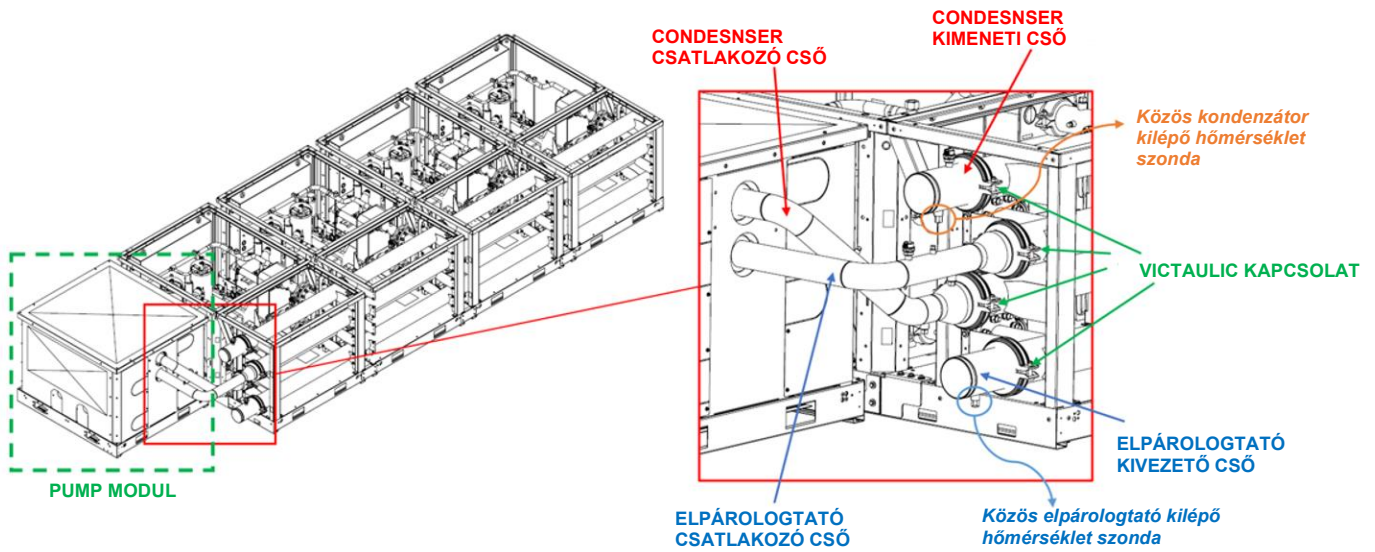
63. ábra - A szondák elhelyezésének részletei a csöveken
