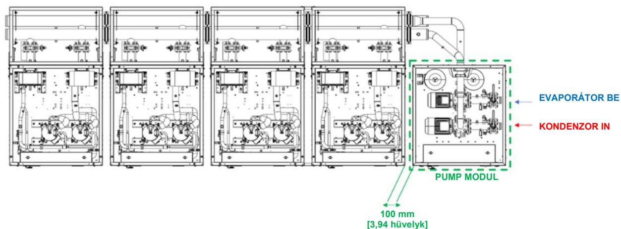
46. ábra - Szivattyúmodul telepítése - csővezetékek részletei
