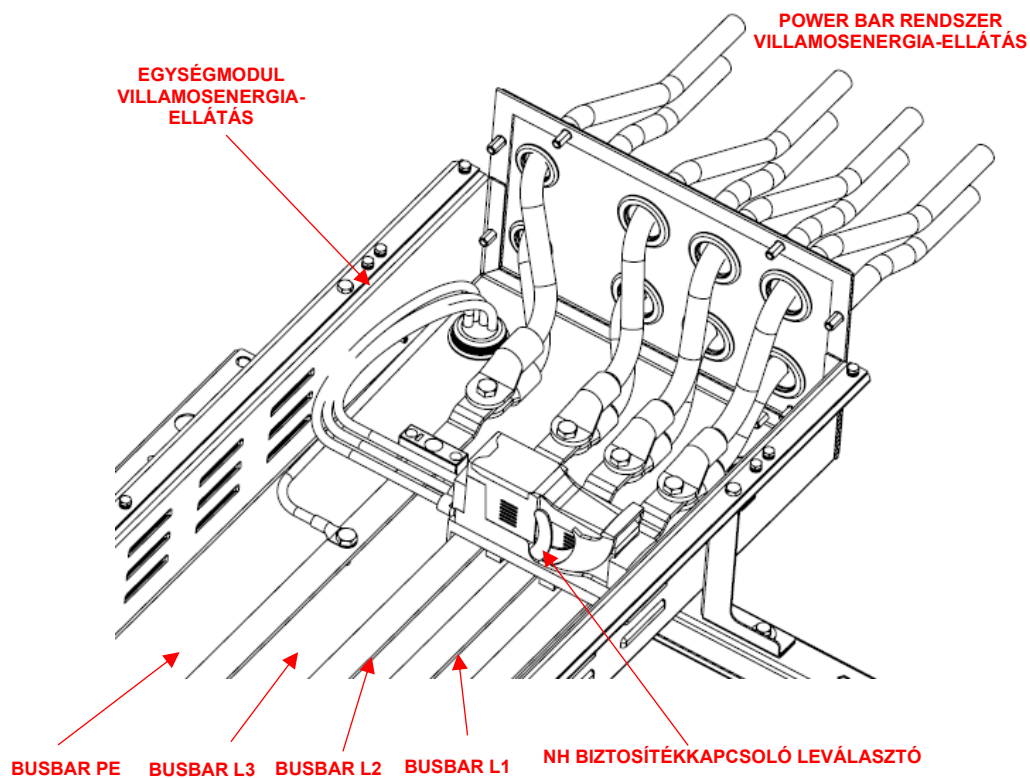
59. ábra - A kezdeti egységmodul elektromos csatlakozásának részletei
