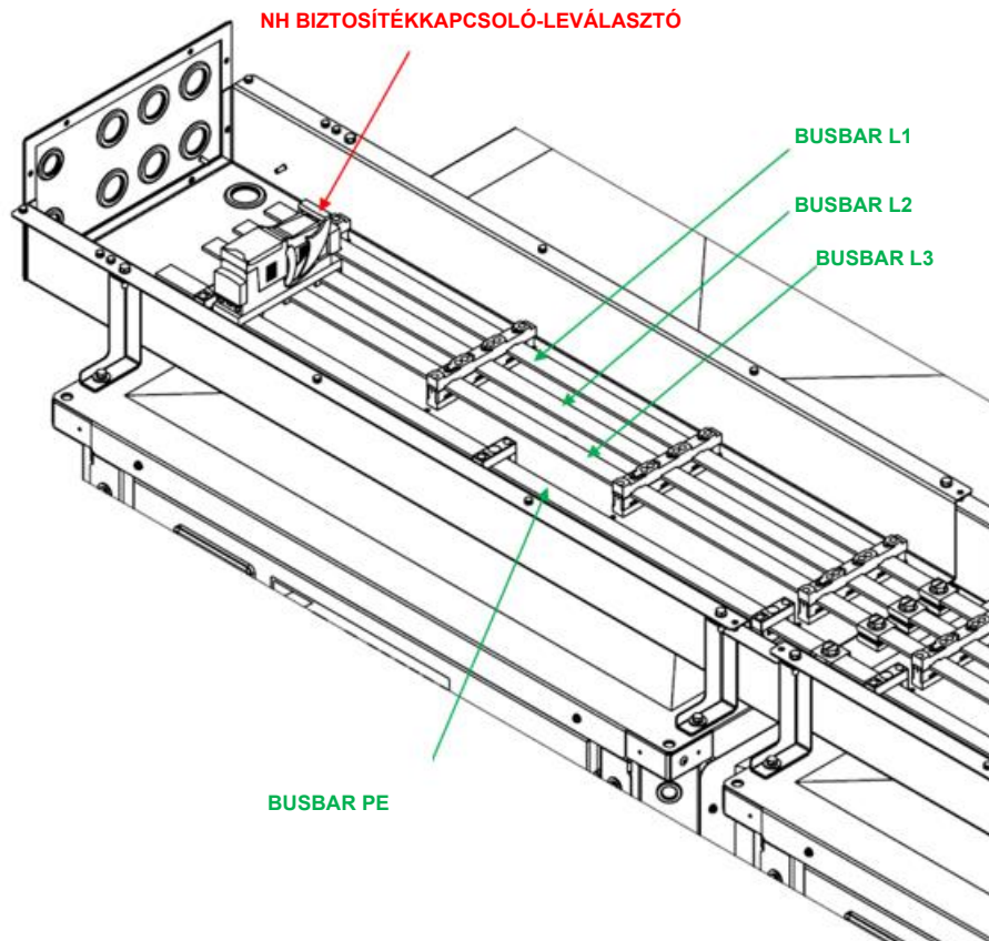
58. ábra - A biztosítékok és a tápkábel-modul kábelek elvezetésére szolgáló dobozának részletei
