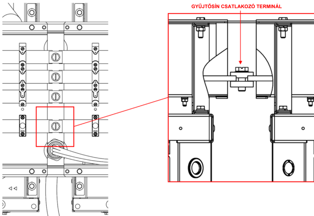
57. ábra - A teljesítménysáv-modulok összekapcsolásának részletei
