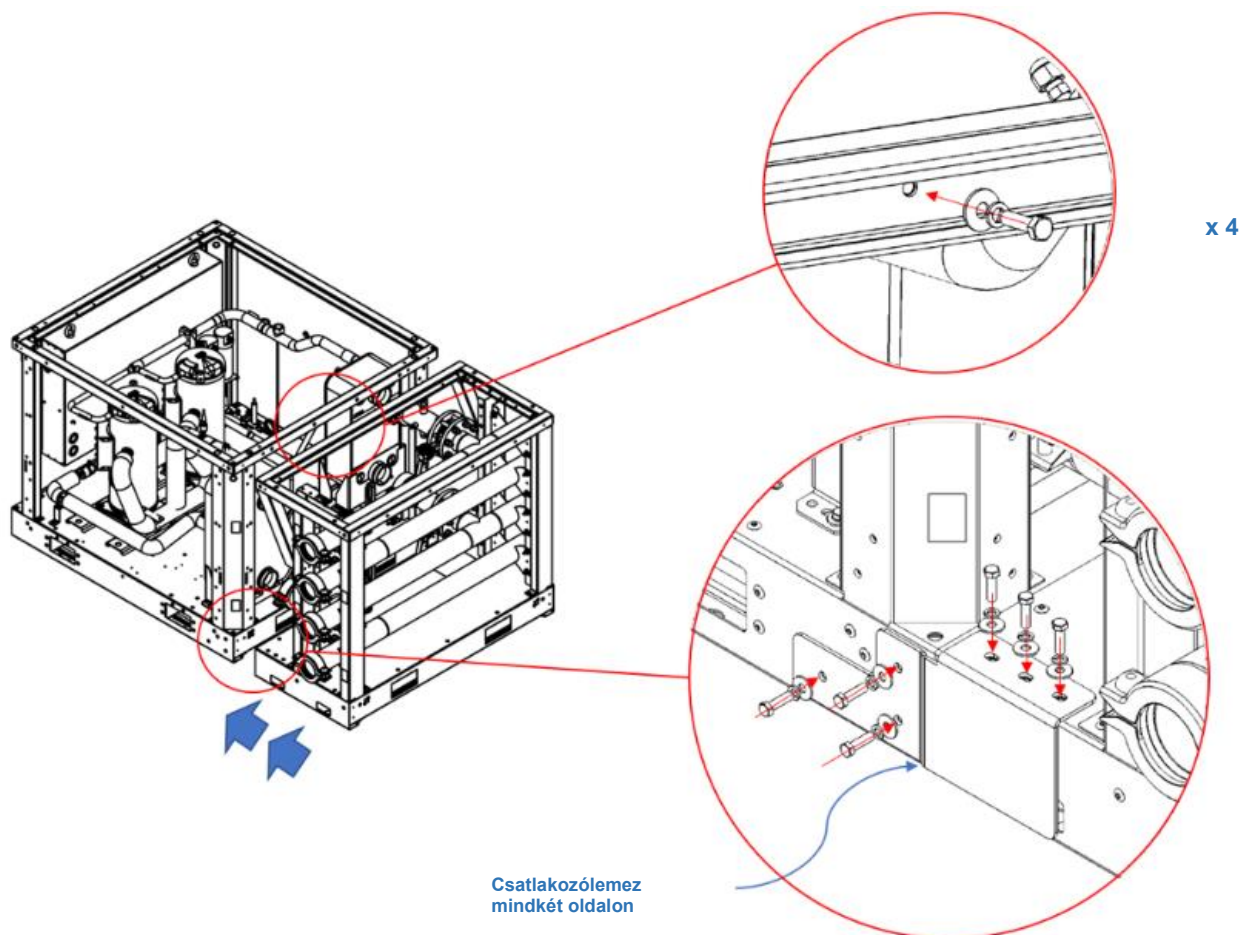
26. ábra - Csatlakozási utasítások a hűtő és a gyújtómodulok között
