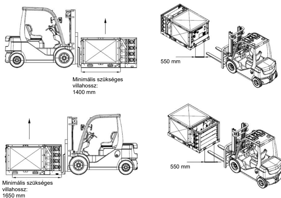
48. ábra - Az egység és a gyűjtőmodulok kezelése
