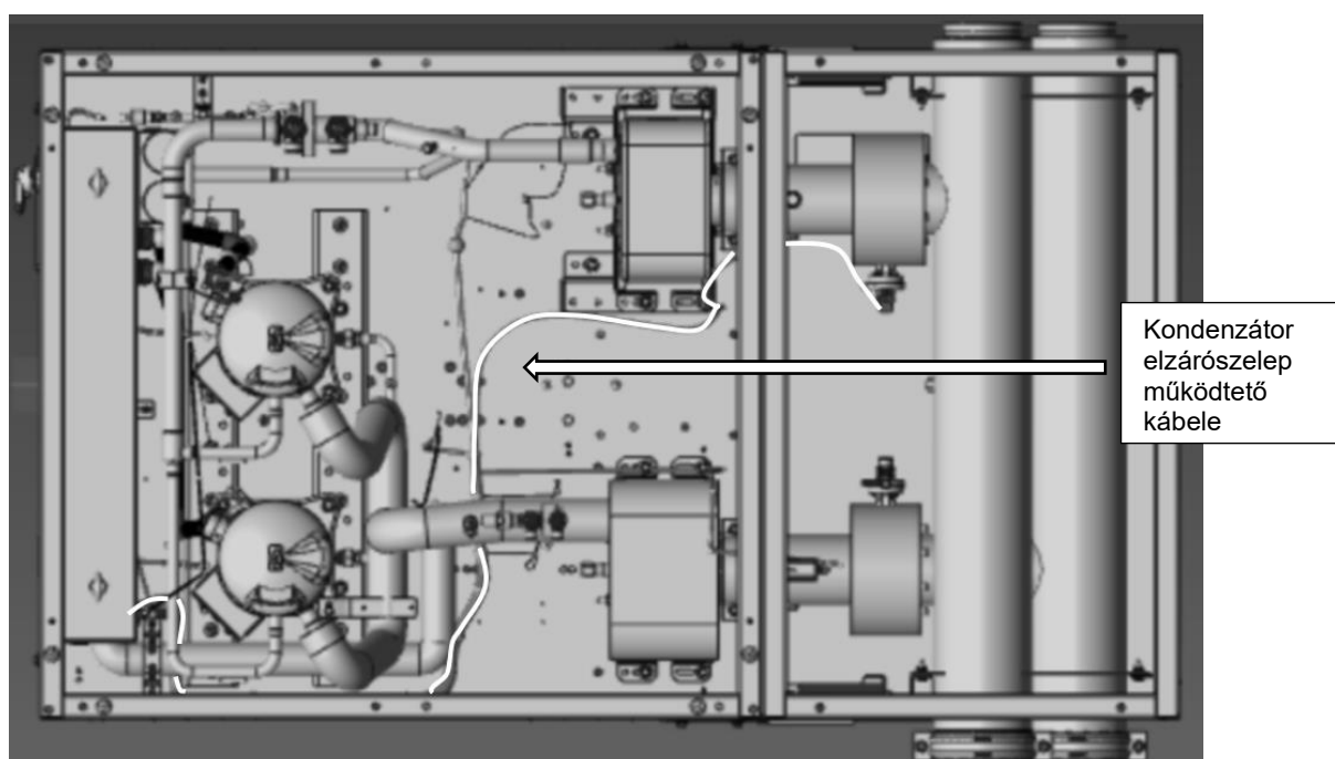
40. ábra - A kondenzátor elzárószelep működtetőjének kábelvezetése
