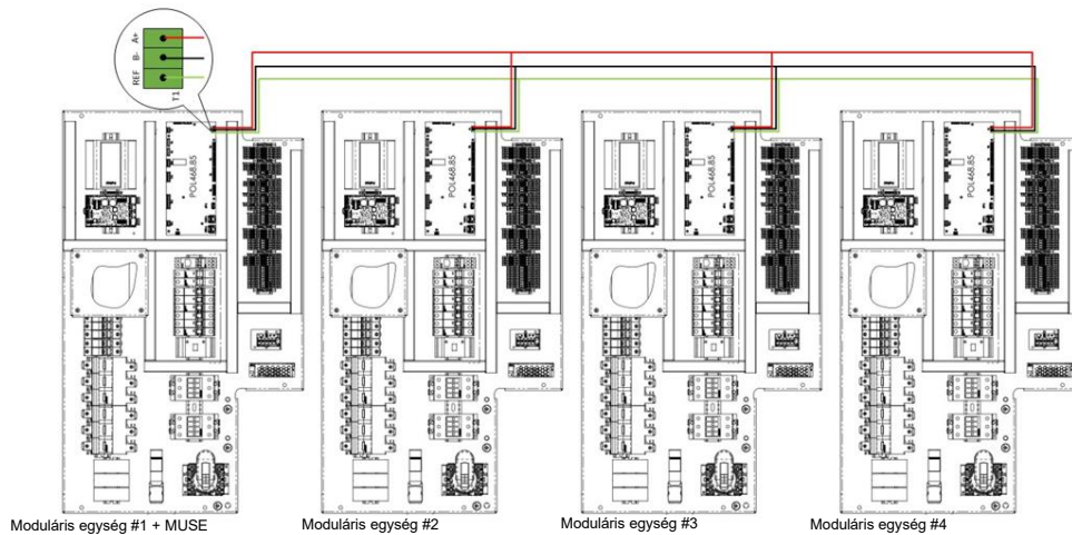
64. ábra - 4 PLC csatlakoztatása ugyanarra a Modbus hálózatra
