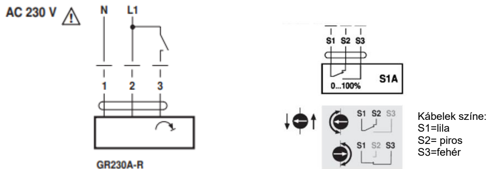
35. ábra - A motor (bal oldali ábra) és a végállaskapcsolók (jobb oldali ábra) kapcsolási rajzi
