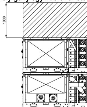
10. ábra - Szerviz helyigény egymásra rakott konfiguráció esetén
