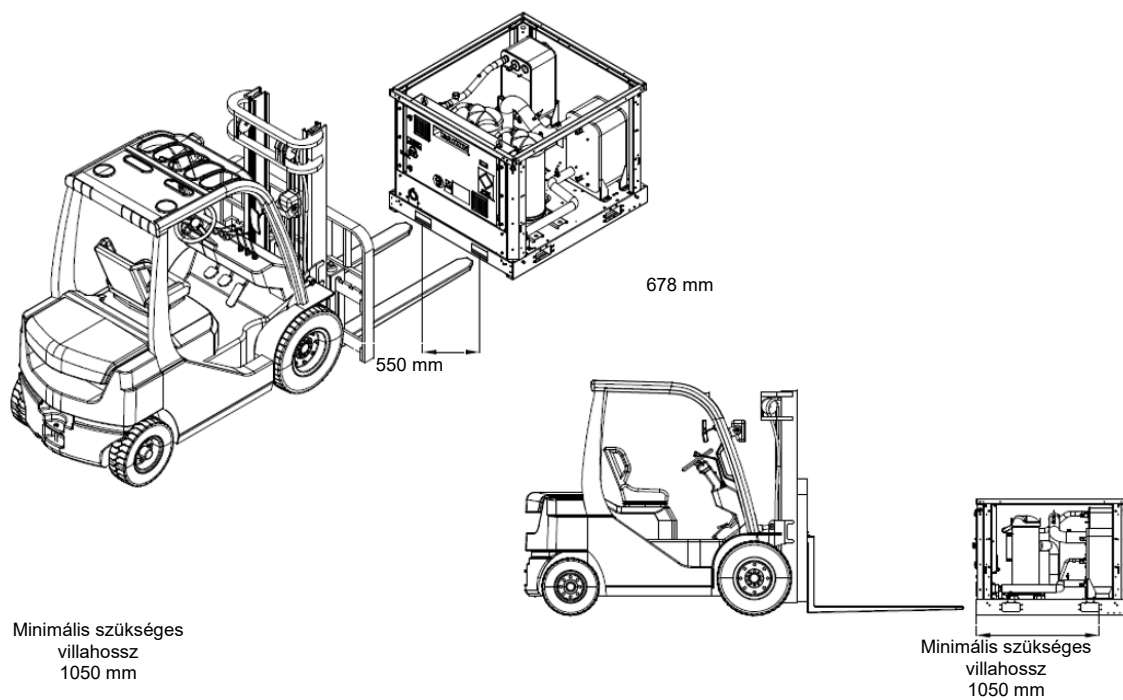
12. ábra - Alternatív kezelési módszer targoncával
