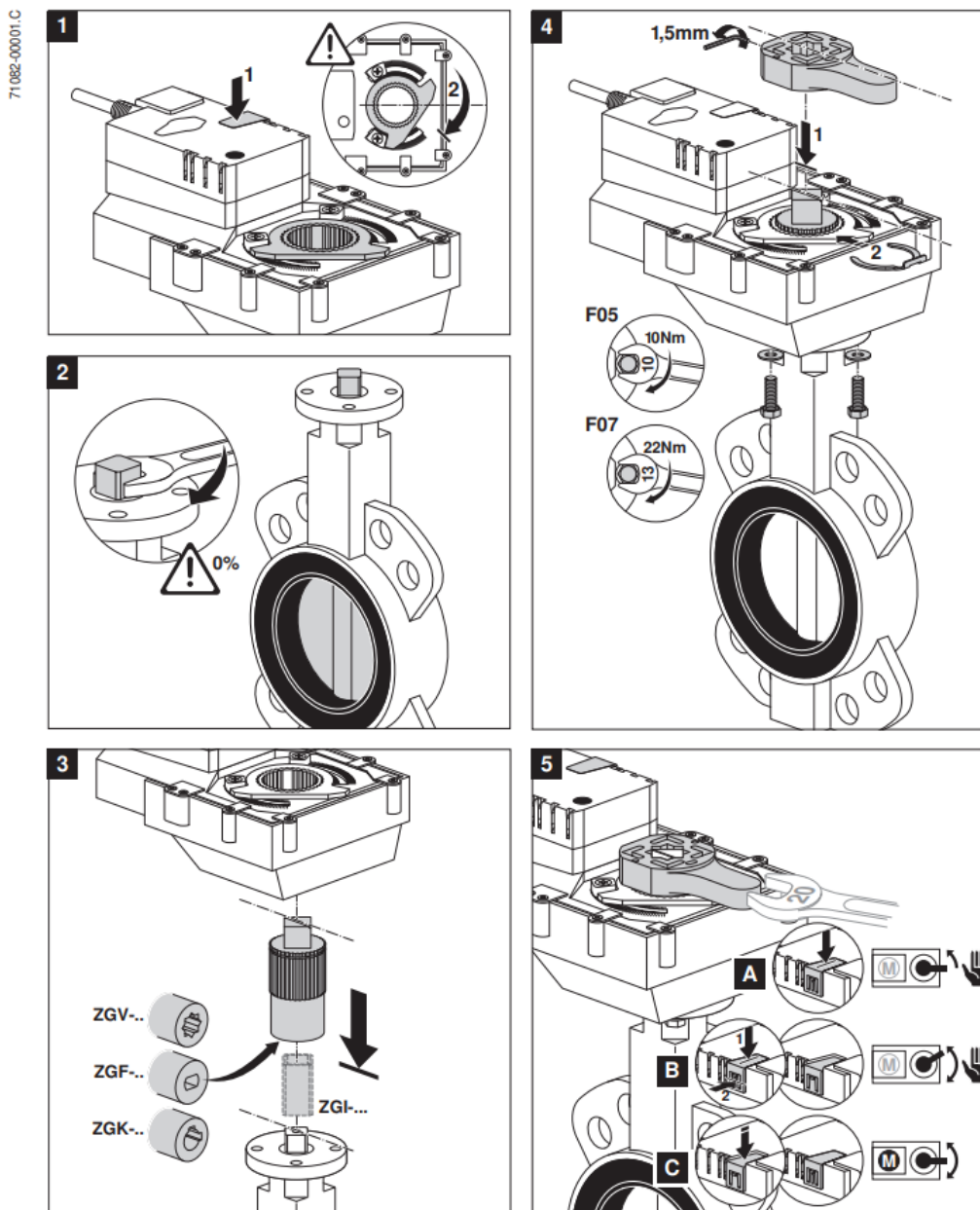
32. ábra - Szerelési utasítások a szelep működtetőjéhez
