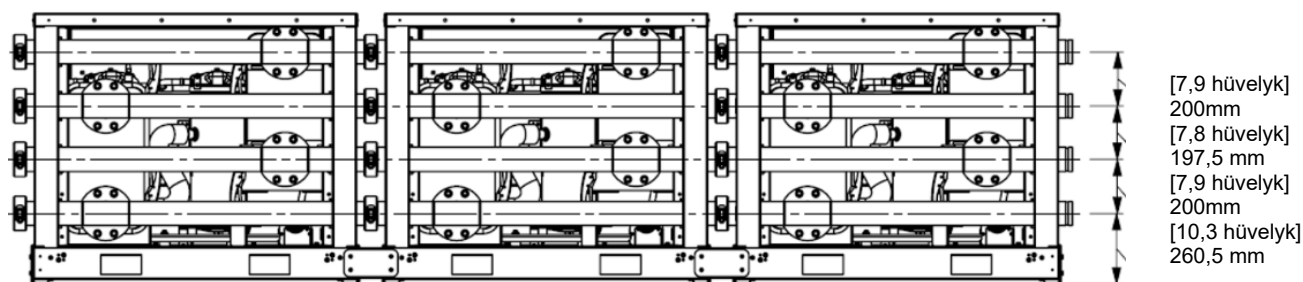
31. ábra - Vízcsatlakozás a modulokhoz
