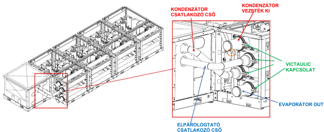
46. ábra - Szivattyúmodul telepítése - csővezetékek részletei
