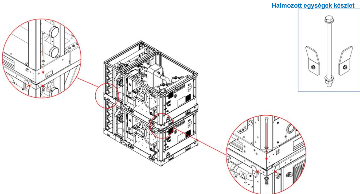
43. ábra - Szerelési utasítások egymásra helyezett egységekhez
