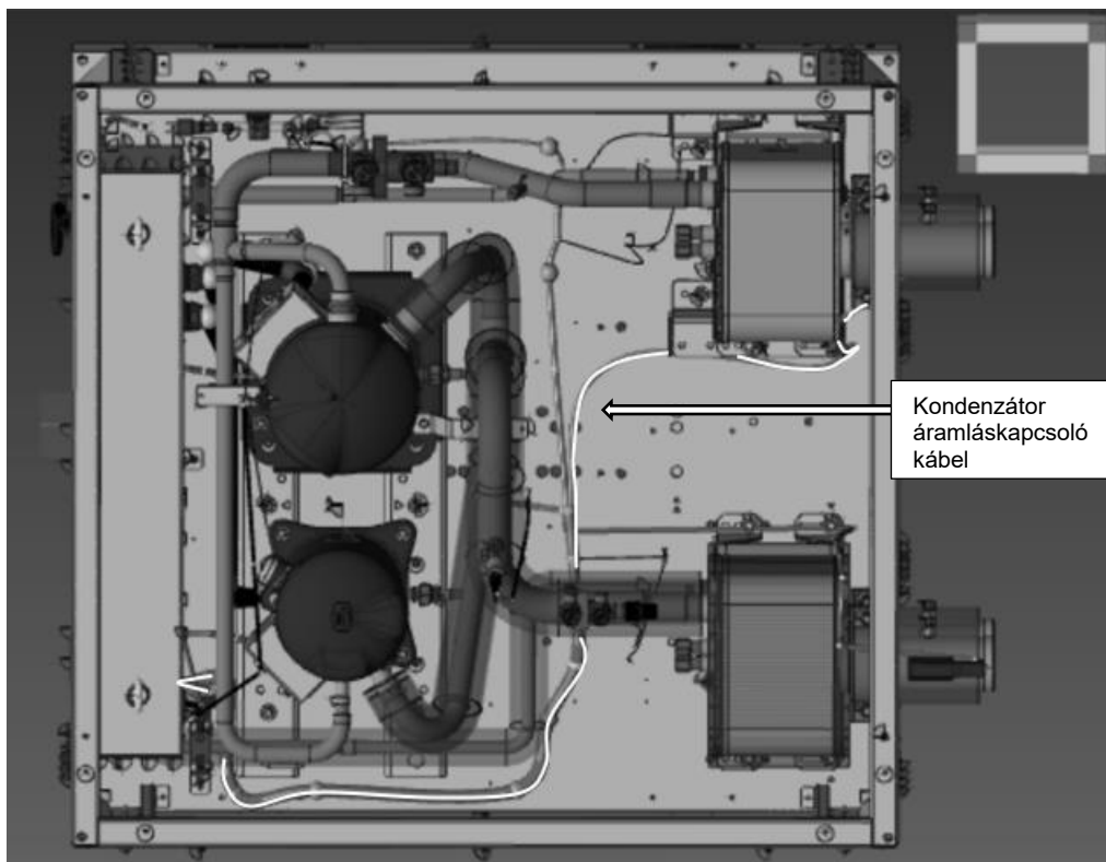
18. ábra - Az elpárolgató és a kondenzátor áramláskapcsoló kábeleinek elektromos panelen való bevezetési pontja
