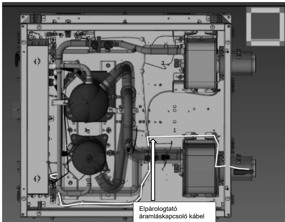
16. ábra - Az elpárologtató áramláskapcsoló kábeleinek elvezetése
