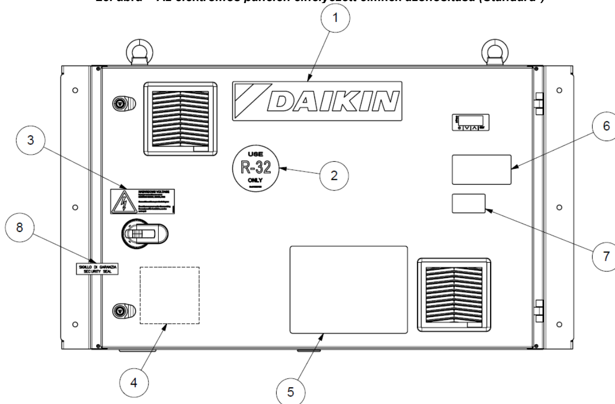
25. ábra - Az elektromos panelen elhelyezett címkek azonosítása (Standard*)
