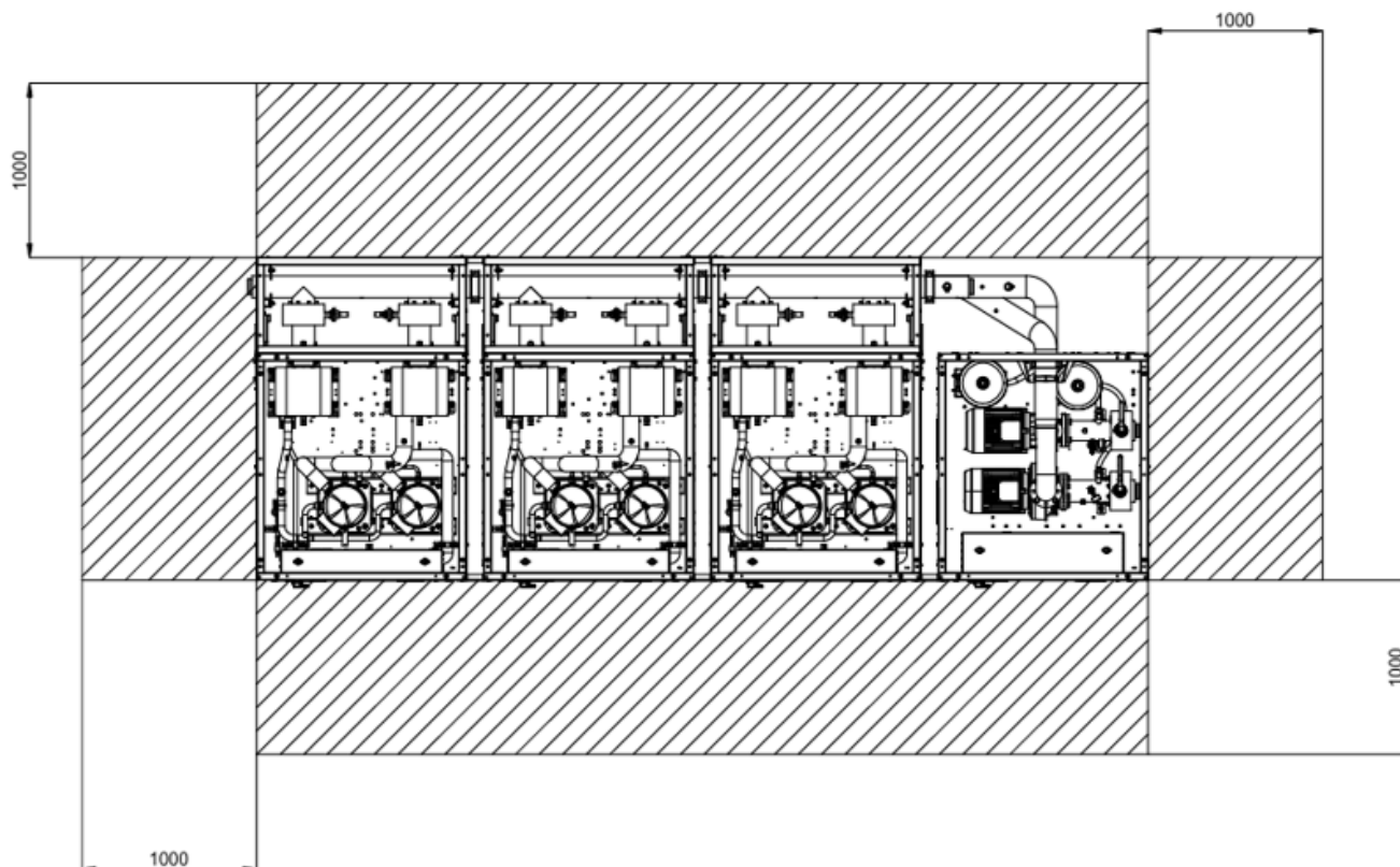
10. ábra - Szerviz helyigény egymásra rakott konfiguráció esetén
