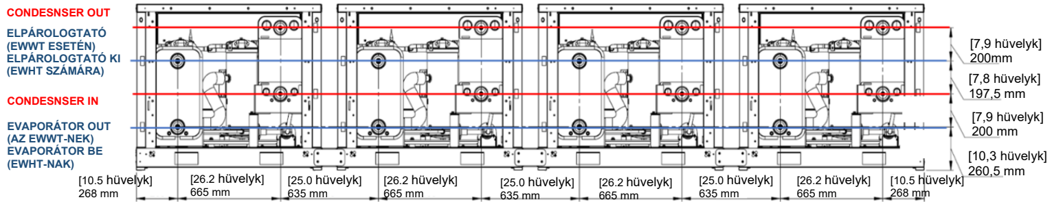
28. ábra - Vízvezeték-konfiguráció
