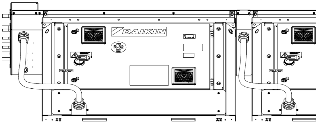
54. ábra - A kábelek elvezetésének részletei
