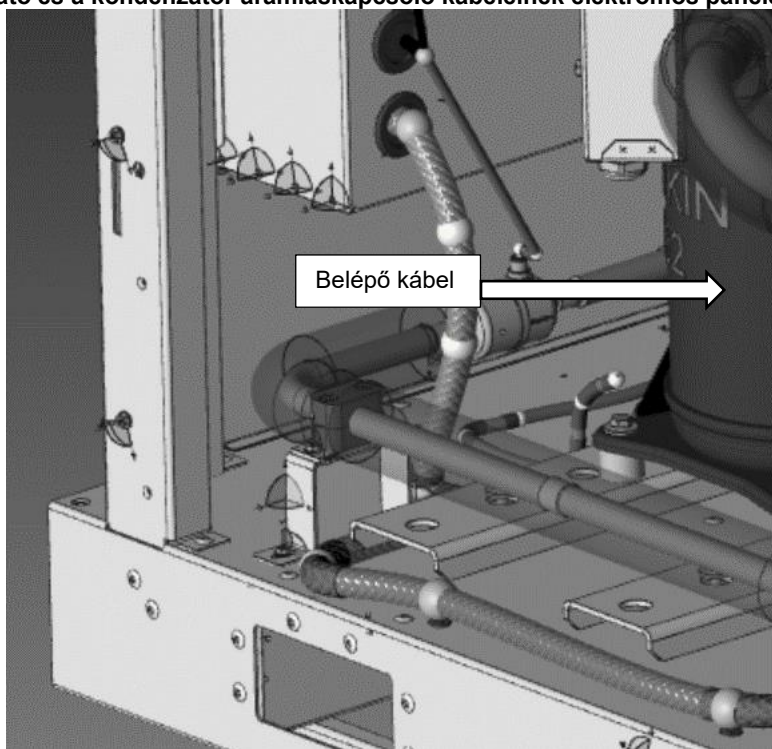
18. ábra - Az elpárolgató és a kondenzátor áramláskapcsoló kábeleinek elektromos panelen való bevezetési pontja
