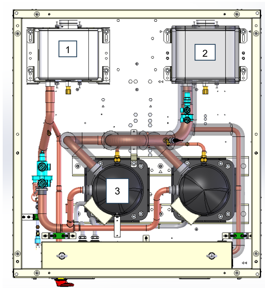
14. ábra - Referenciarajz az elpárolgató és a kondenzátor azonosításához
