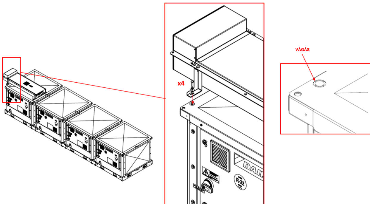
55. ábra - A tápegységhez való rögzítés a tápegységhez
