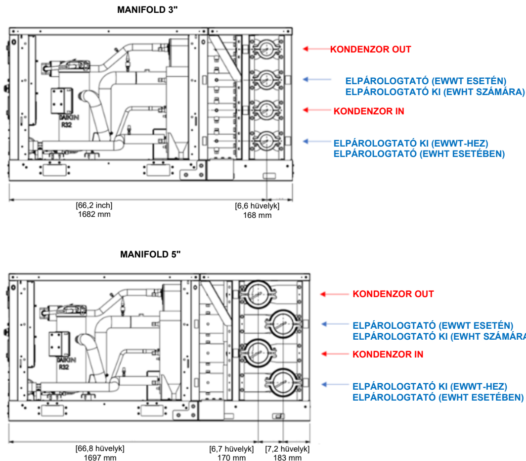
30. ábra - Vízugyjtőcső méretek
