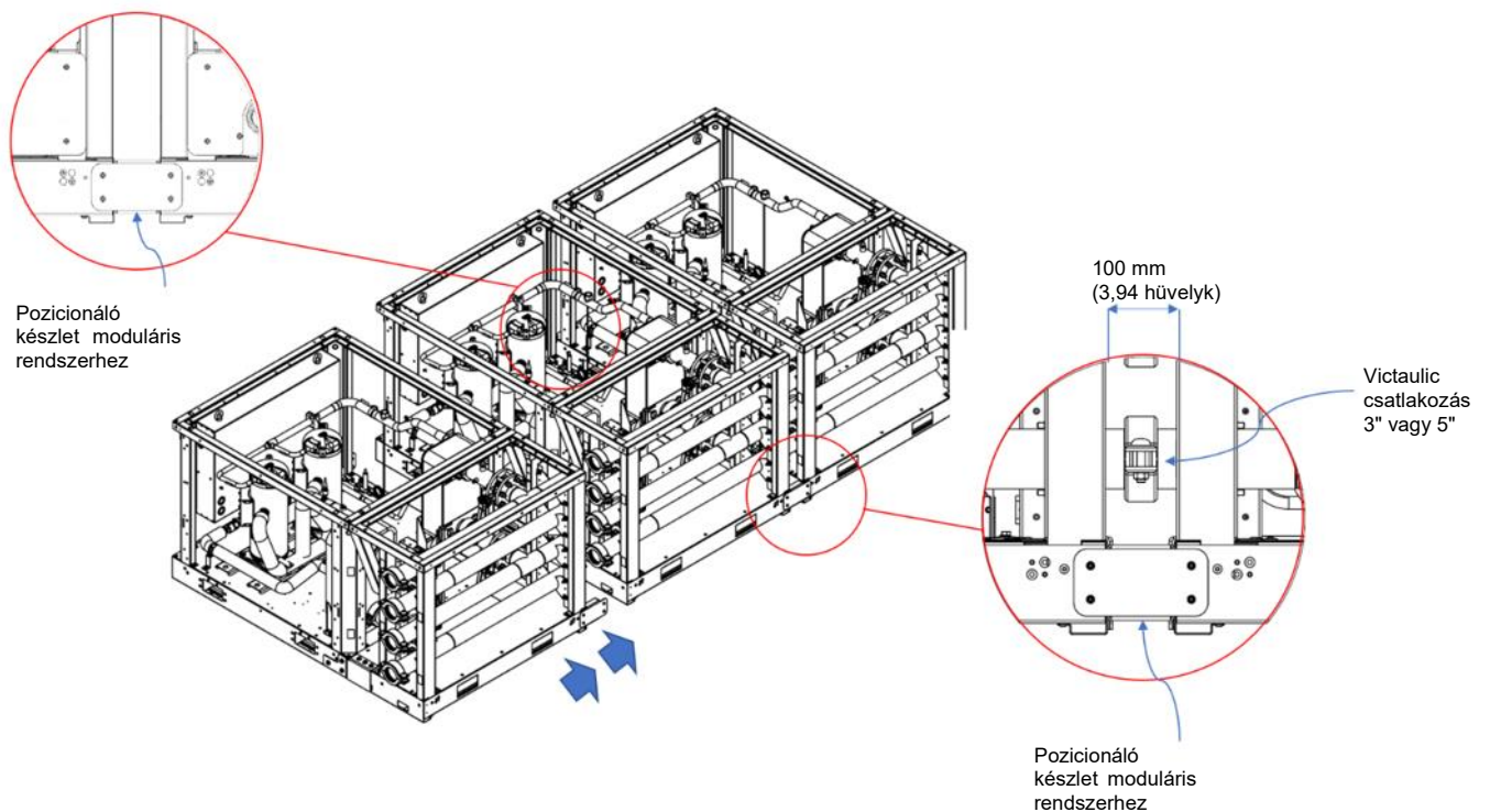
29. ábra - Moduláris rendszerek csatlakoztatása
