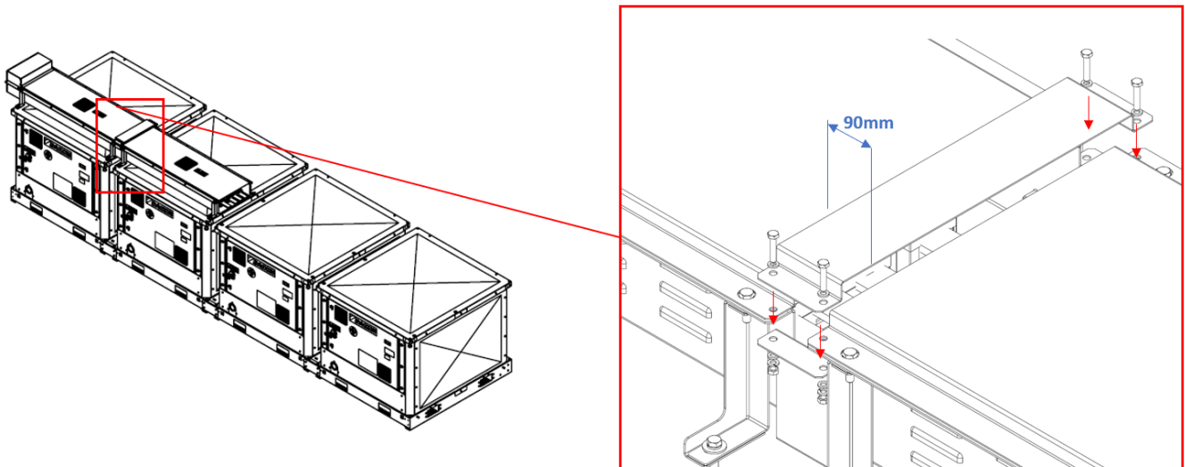
56. ábra - A teljesítménysáv-modulok összekapcsolása
