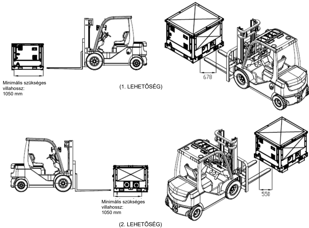
50. ábra - A szivattyúmodul kezelése targoncával
