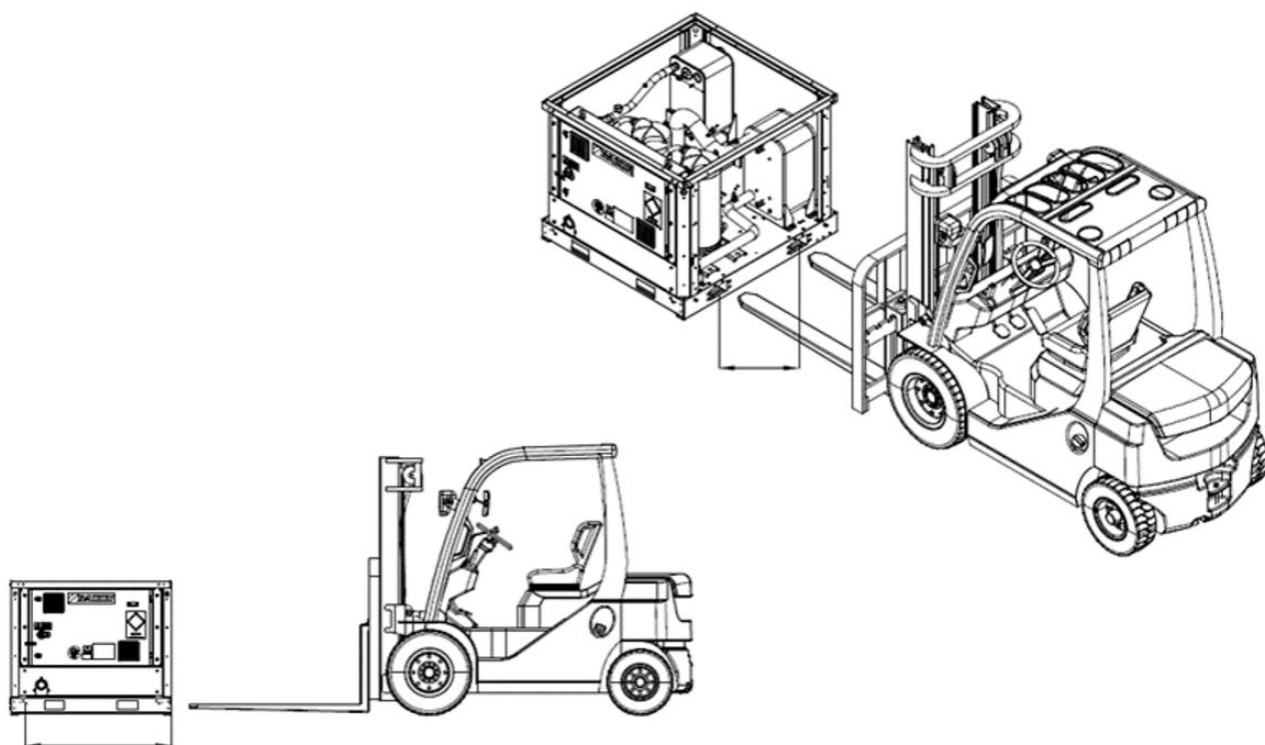
11. ábra - Az egykörös egység kezelése
