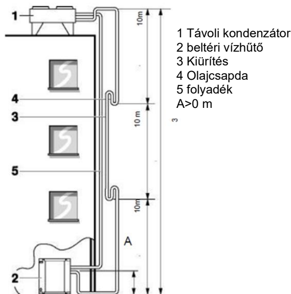
20. ábra - A hűtőközegkör csatlakoztatása (1)
