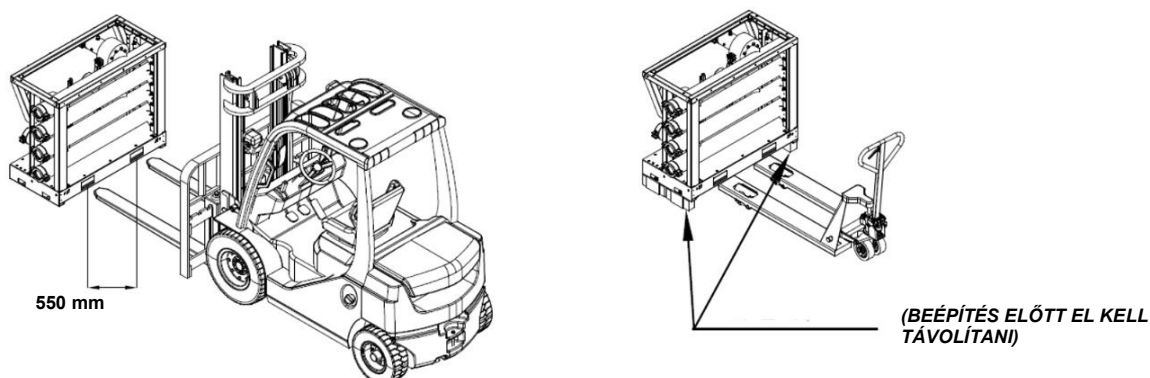
47. ábra - A gyűjtőmodul kezelése
