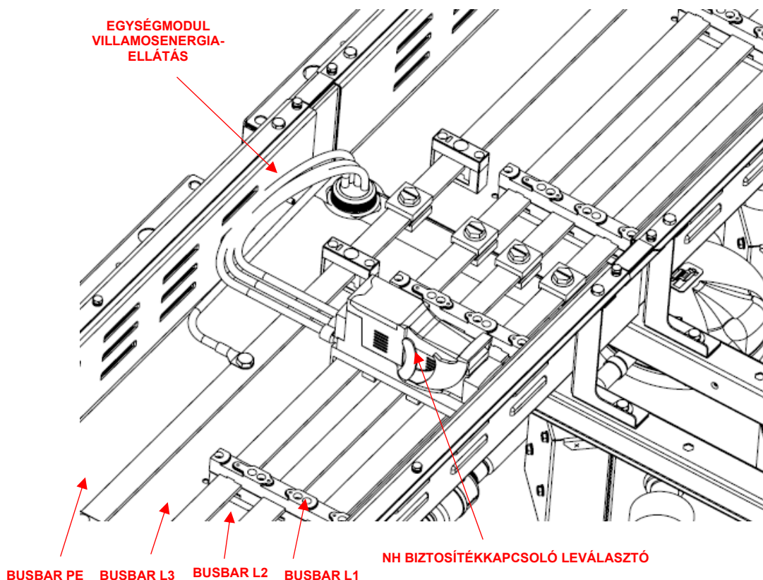
60. ábra - Az elektromos csatlakozás részletei bármely más egységmodulhoz
