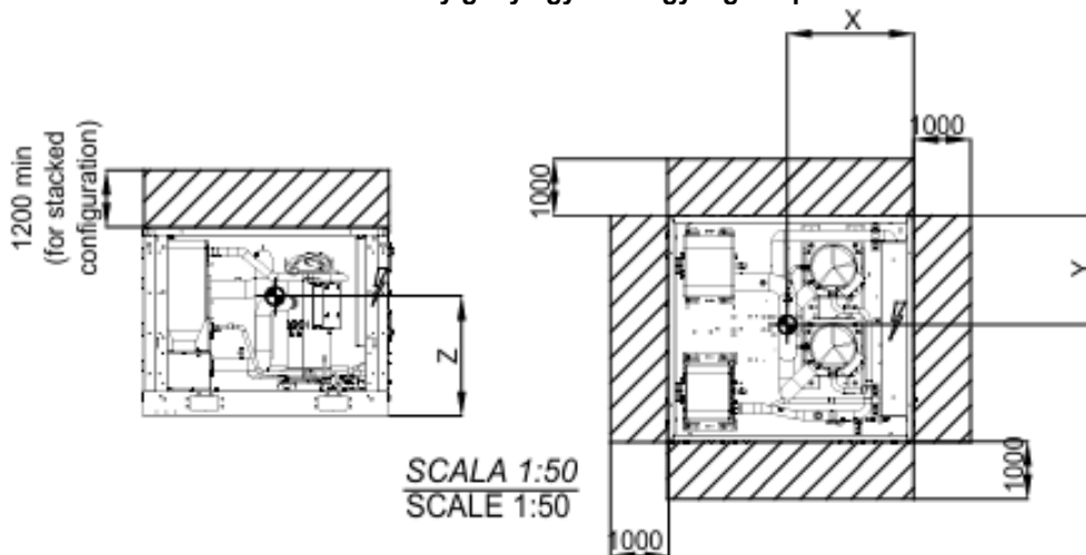
8. ábra – Szervizhelyigény egyetlen egység telepítéséhez
