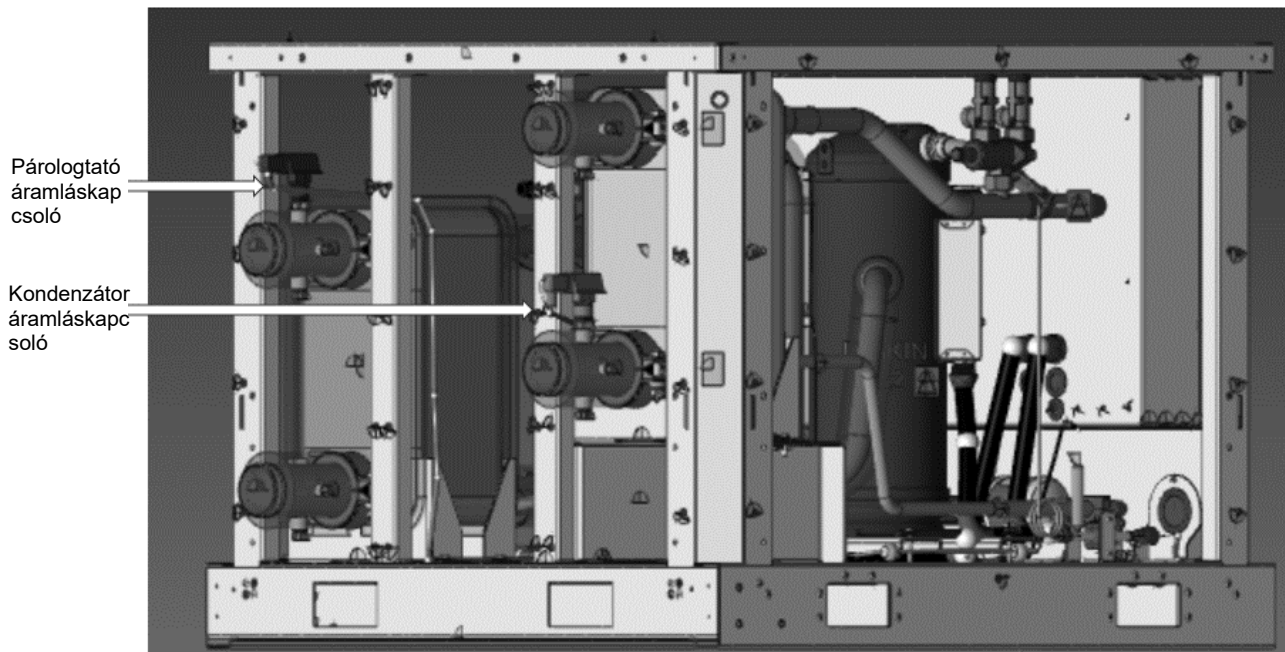
16. ábra - Az elpárologtató áramláskapcsoló kábeleinek elvezetése
