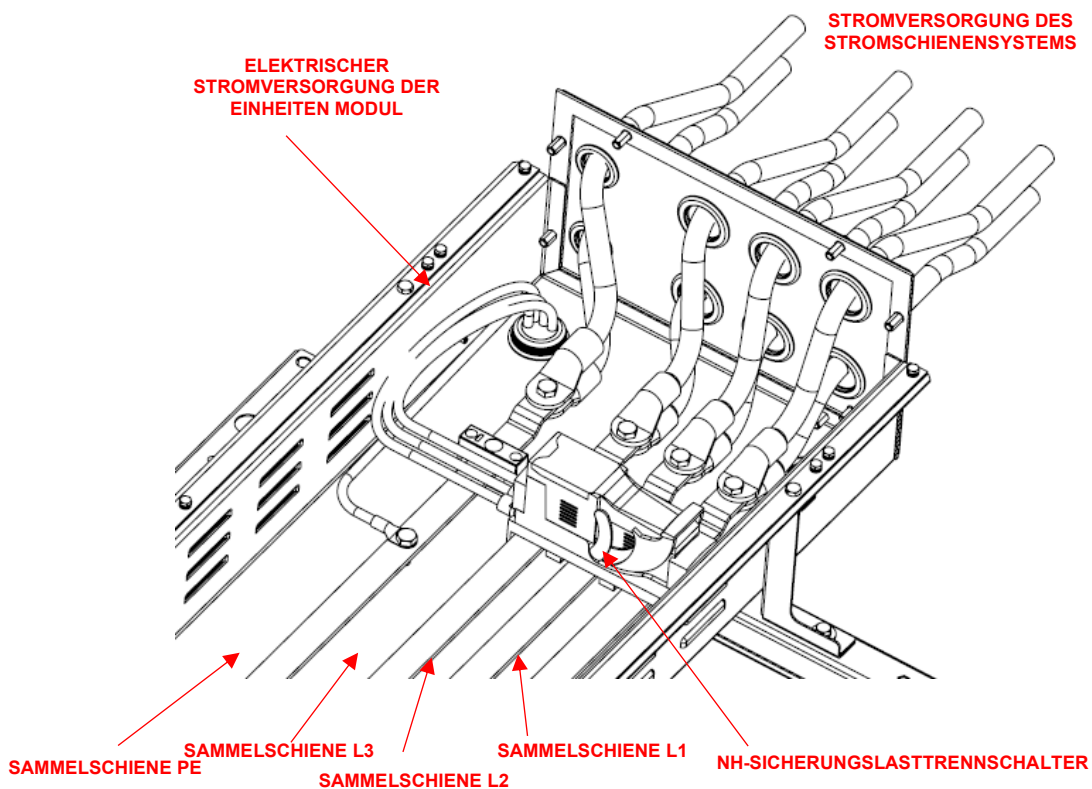
Abb. 59 - Detail des elektrischen Anschlusses des ersten Moduls der Einheit
