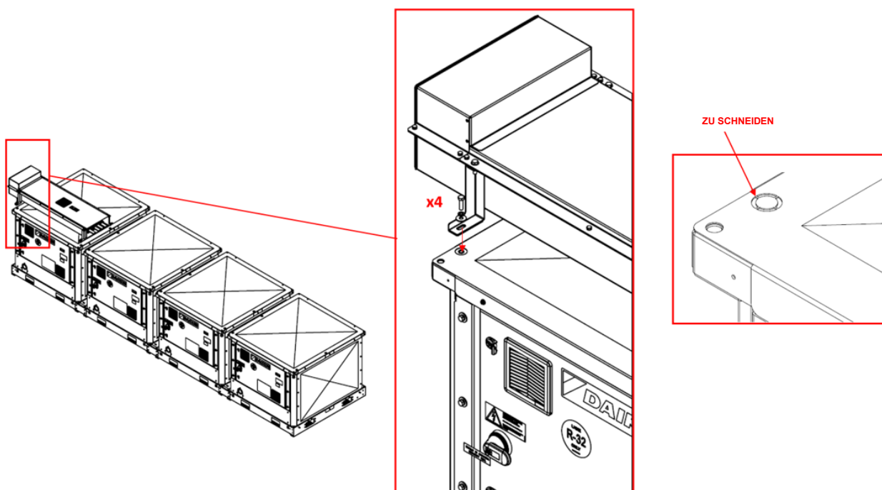
Abb. 55 - Befestigung des Stromschienensystems an der Einheit
