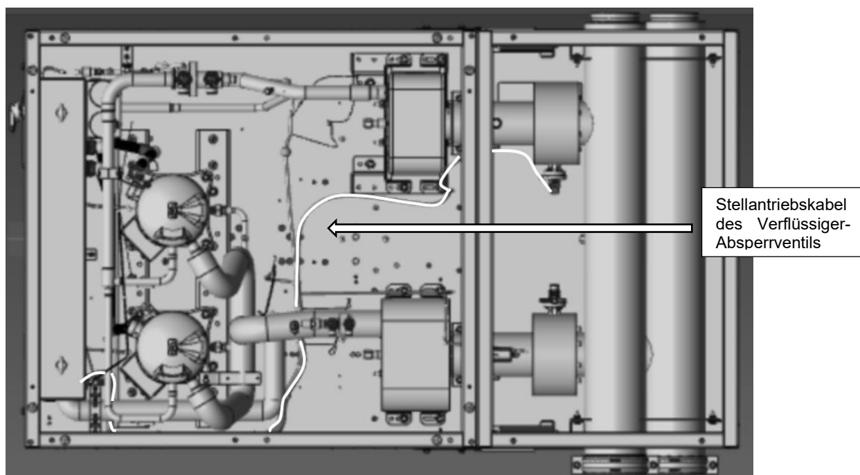
Abb. 40 - Kabelführung des Stellantriebs des Verflüssiger-Absperrventils
