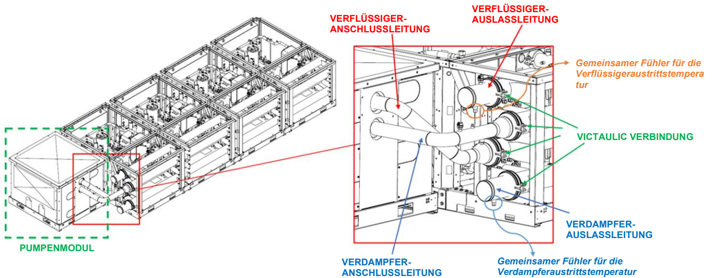
Abb. 63 - Einzelheiten zur Positionierung der Sonden an den Rohren
