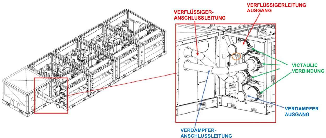
Abb. 46 - Installation des Pumpenmoduls - Details zur Verrohrung
