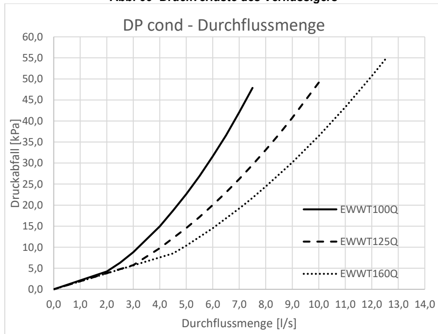
Abb. 66 - Druckverluste des Verflüssigers
