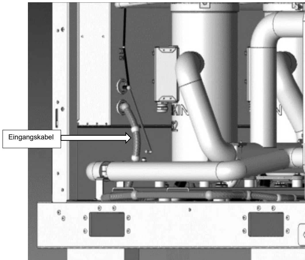
Abb. 41 - Schaltschrankeingang für Verdampfer- und Verflüssiger-Absperrventilstellerkabel
