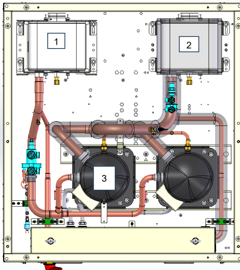
Abb. 14 - Referenzzeichnung zur Identifizierung von Verdampfer und Verflüssiger
