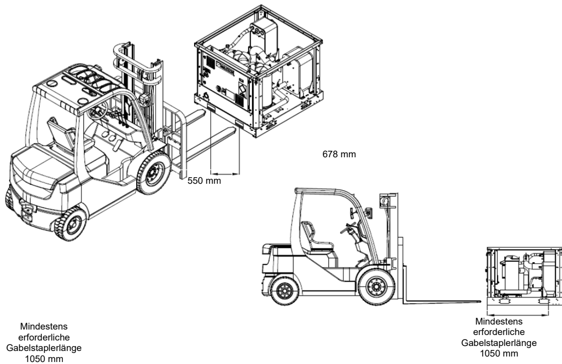
Abb. 12 - Alternative Handhabung mit Gabelstapler
