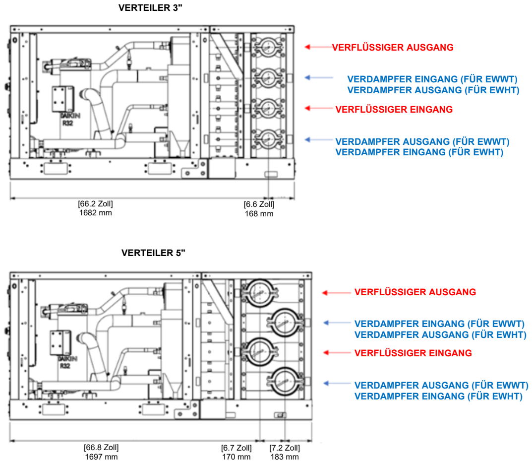
Abb. 30 - Größen des Wasserverteilers
