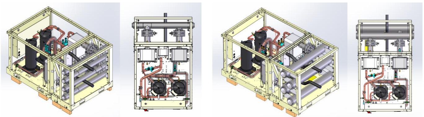
Abb. 27 - PHR-Rohre mit Verteilermodul (links für 3-Zoll - rechts für 5-Zoll-Verteilerrohre)
