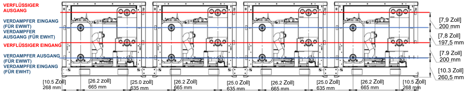
Abb. 28 - Konfiguration der Wasserleitungen
