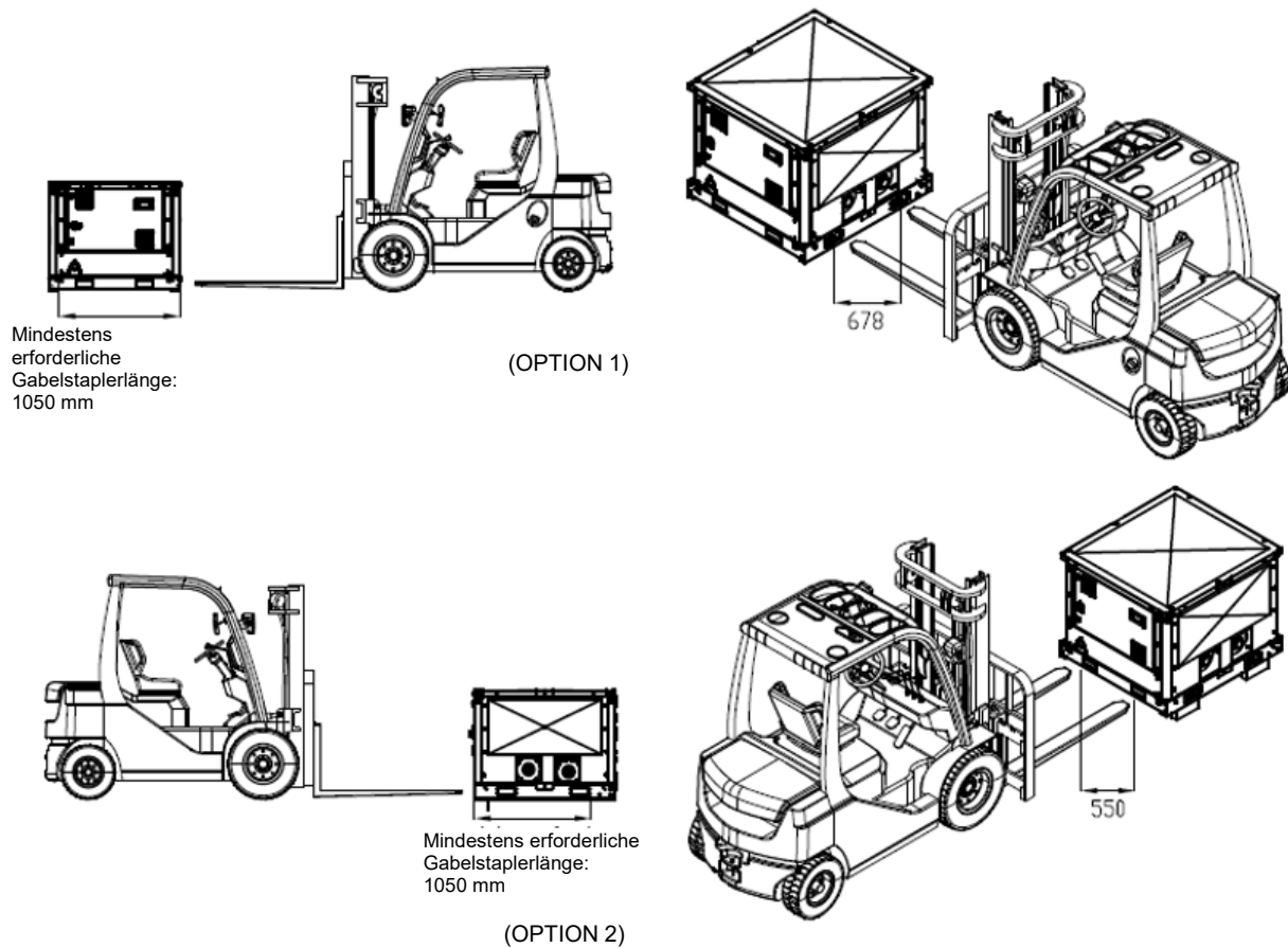
Abb. 50 - Handhabung des Pumpenmoduls mit einem Gabelstapler
