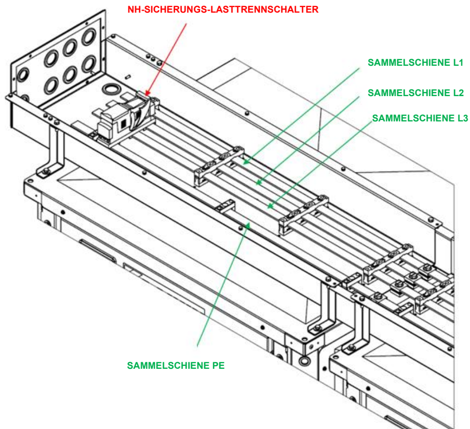
Abb. 58 - Detail der Sicherungen und des Kabeldurchführungsgehäuses des Stromschienenmoduls
