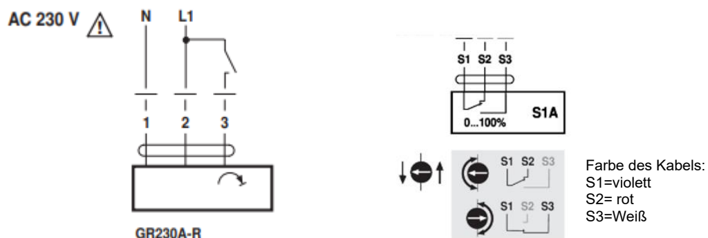
Abb. 35 - Schaltplan für Motor (linke Abbildung) und Endschalter (rechte Abbildung)
