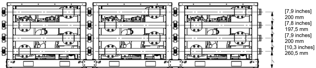
Abb. 31 - Wasseranschluss an die Module
