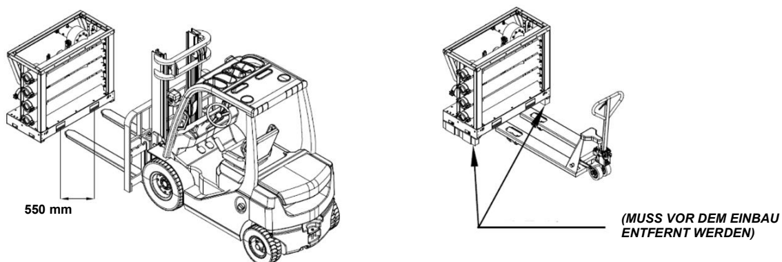
Abb. 47 - Handhabung des Verteilermoduls
