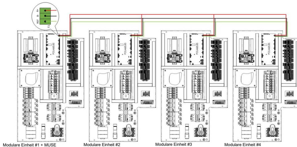
Abb. 64 - Anschluss von 4 PLCs an das gleiche Modbus-Netzwerk
