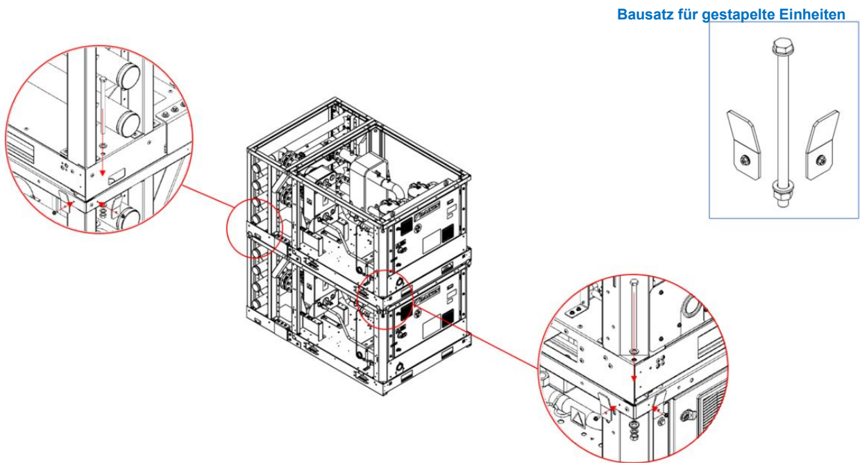
Abb. 43 - Montageanleitung für gestapelte Einheiten
