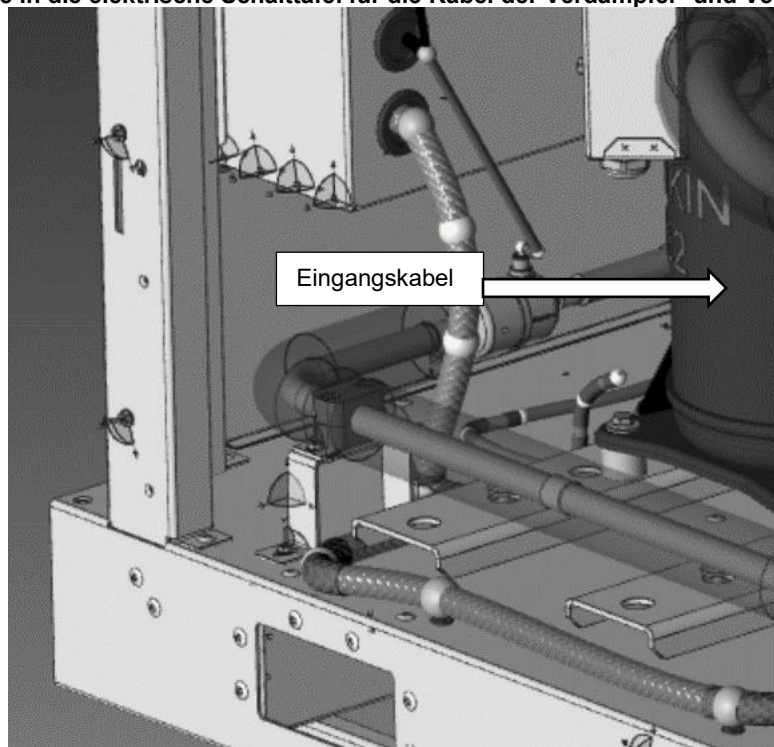
Abb. 18 - Eintrittsstelle in die elektrische Schalttafel für die Kabel der Verdampfer- und Verflüssigerstromschalter
