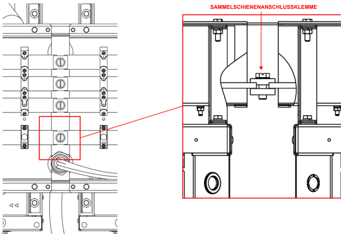
Abb. 57 - Details zur Verbindung der Stromschienenmodule untereinander
