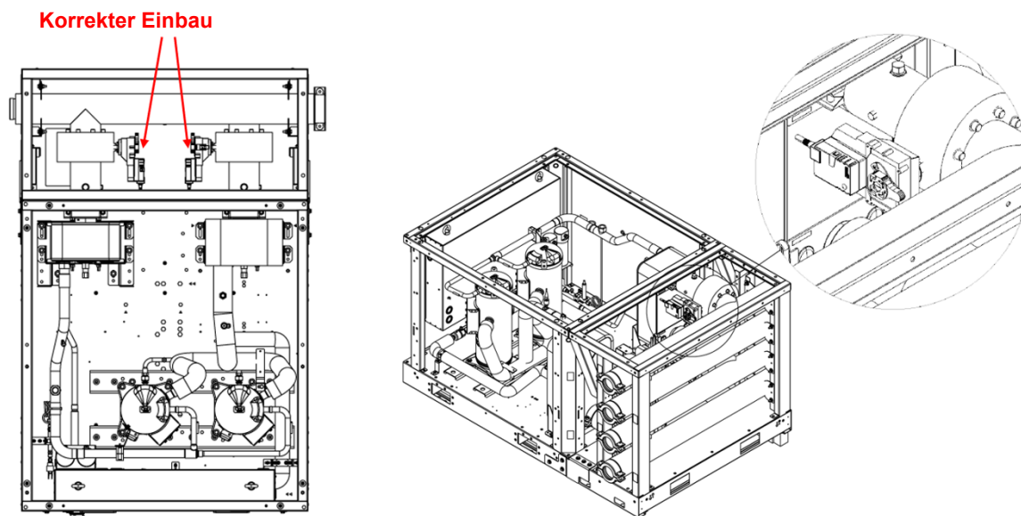
Abb. 34 - Montagehinweise für den Ventiltrieb
