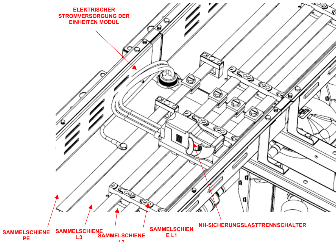
Abb. 60 - Detail des elektrischen Anschlusses für jedes andere Modul der Einheit
