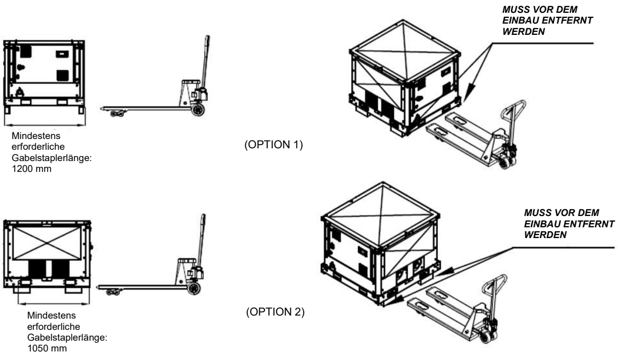
Abb. 51 - Handhabung des Pumpenmoduls mit einem Gabelhubwagen
