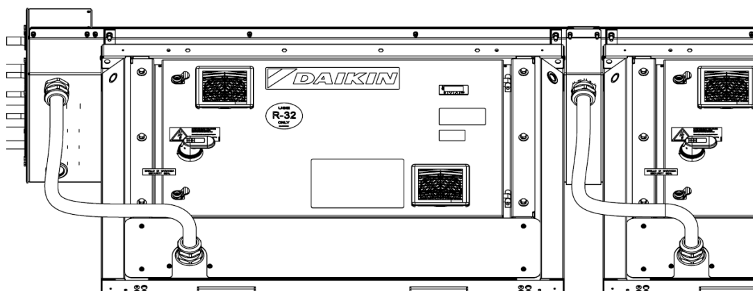
Abb. 54 - Details der Kabelverlegung
