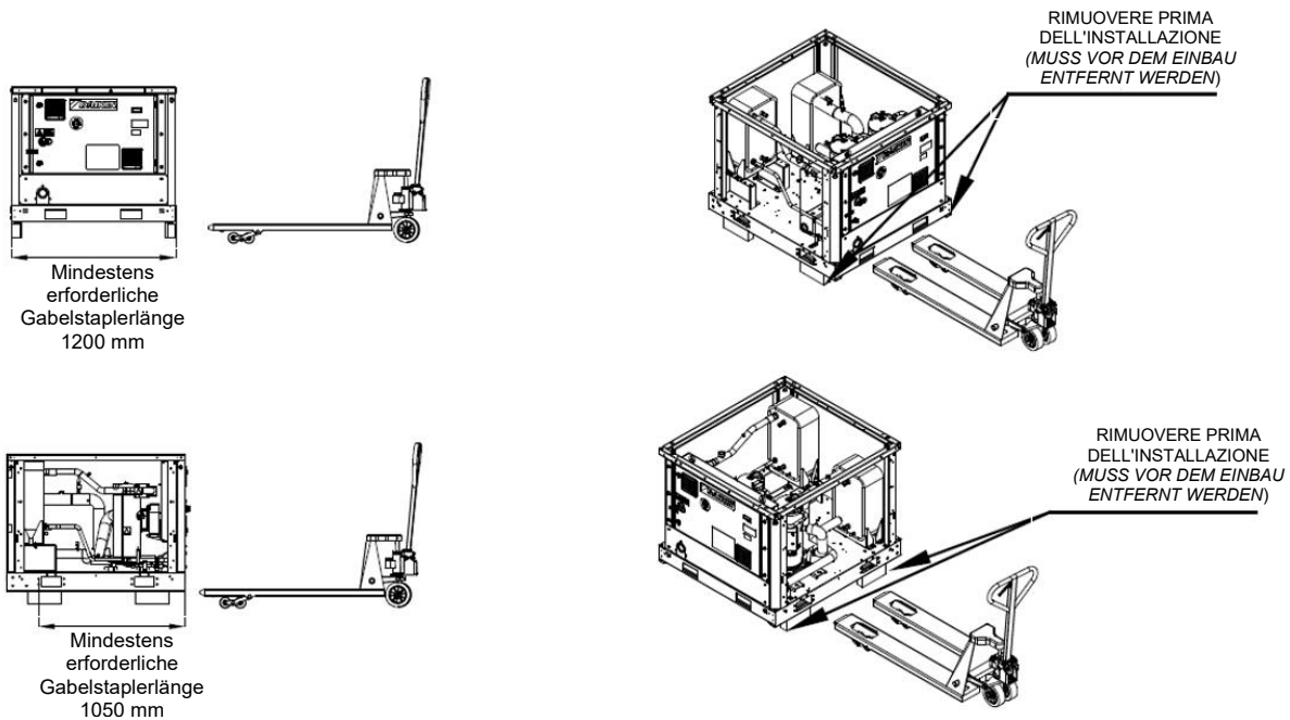
Abb. 13 - Alternative Handhabung mit Gabelhubwagen
