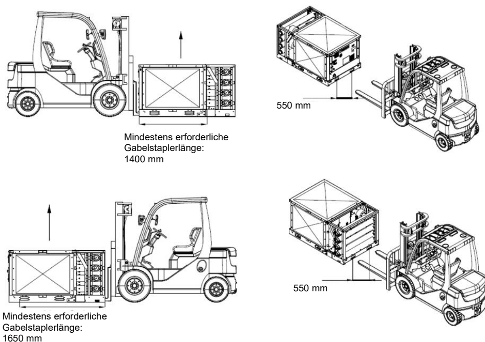
Abb. 48 - Handhabung der Geräte- und Verteilermodule
