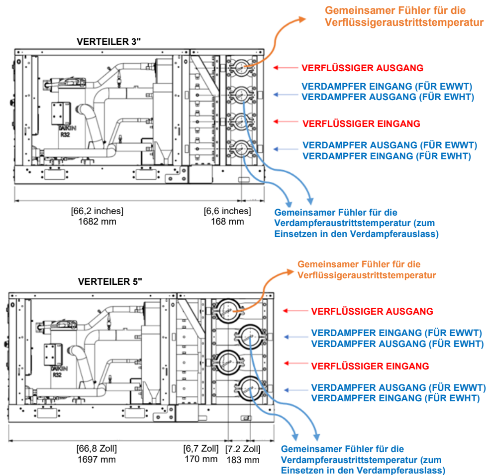
Abb. 62 - Positionen der Temperaturfühler für 3" und 5" Verteiler
