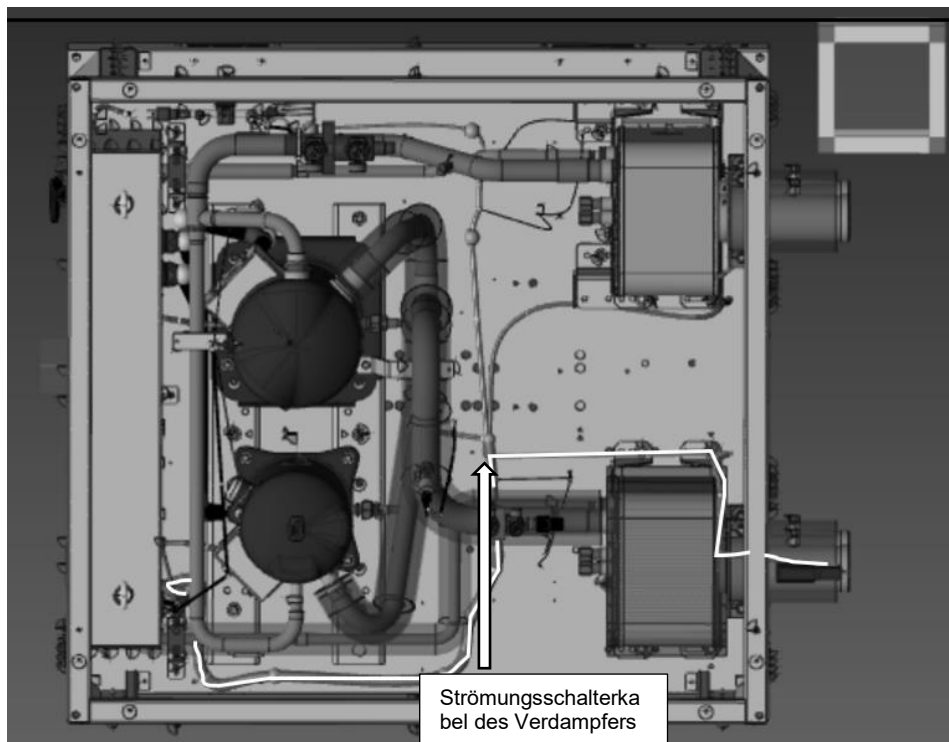
Abb. 16 - Kabelverlegung des Verdampfer-Strömungswächters
