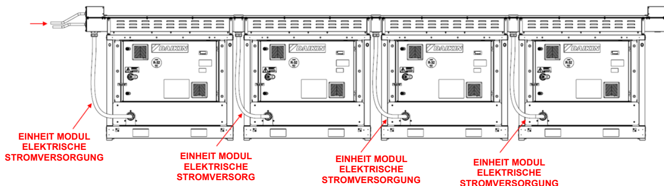
Abb. 54 - Details der Kabelverlegung
