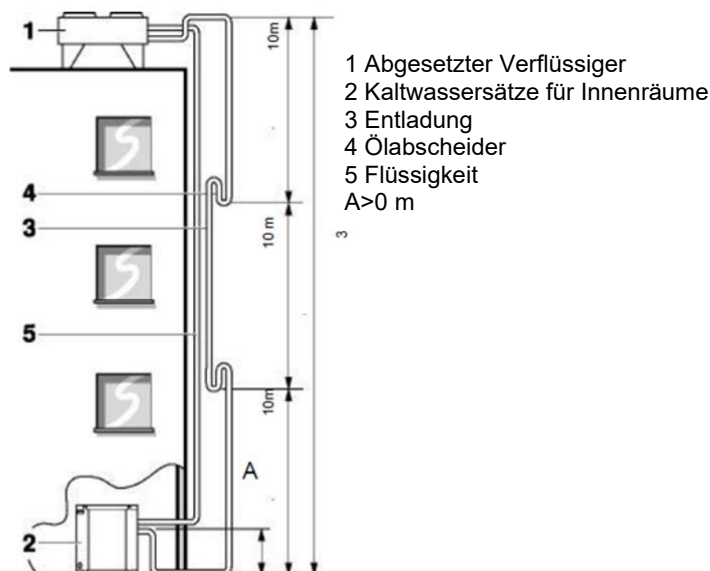
Abb. 20 - Anschluss des Kältemittelkreislaufs (1)
