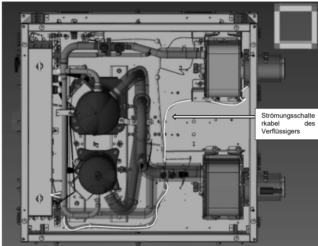
Abb. 18 - Eintrittsstelle in die elektrische Schalttafel für die Kabel der Verdampfer- und Verflüssigerstromschalter
