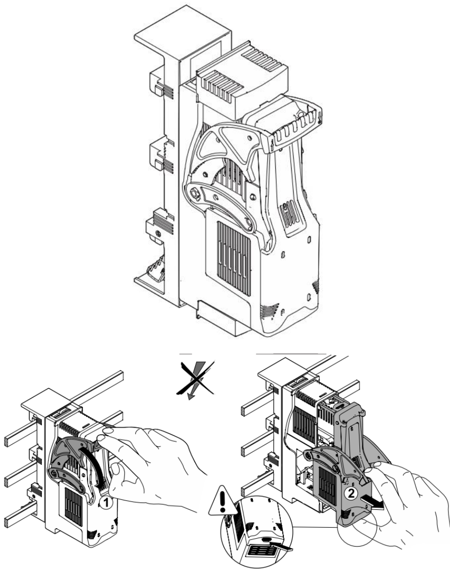
Abb. 61 - NH-Sicherungs-Lasttrennschalter
