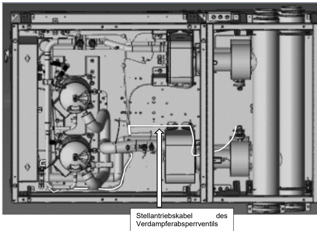
Abb. 39 - Kabelführung des Stellantriebs des Verdampferabsperrentils
