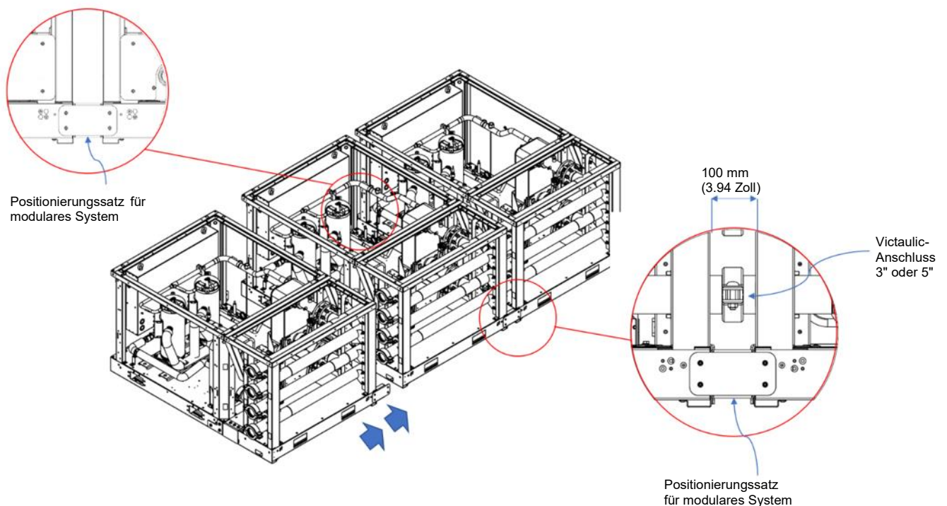
Abb. 29 - Verbindung der modularen Systeme
