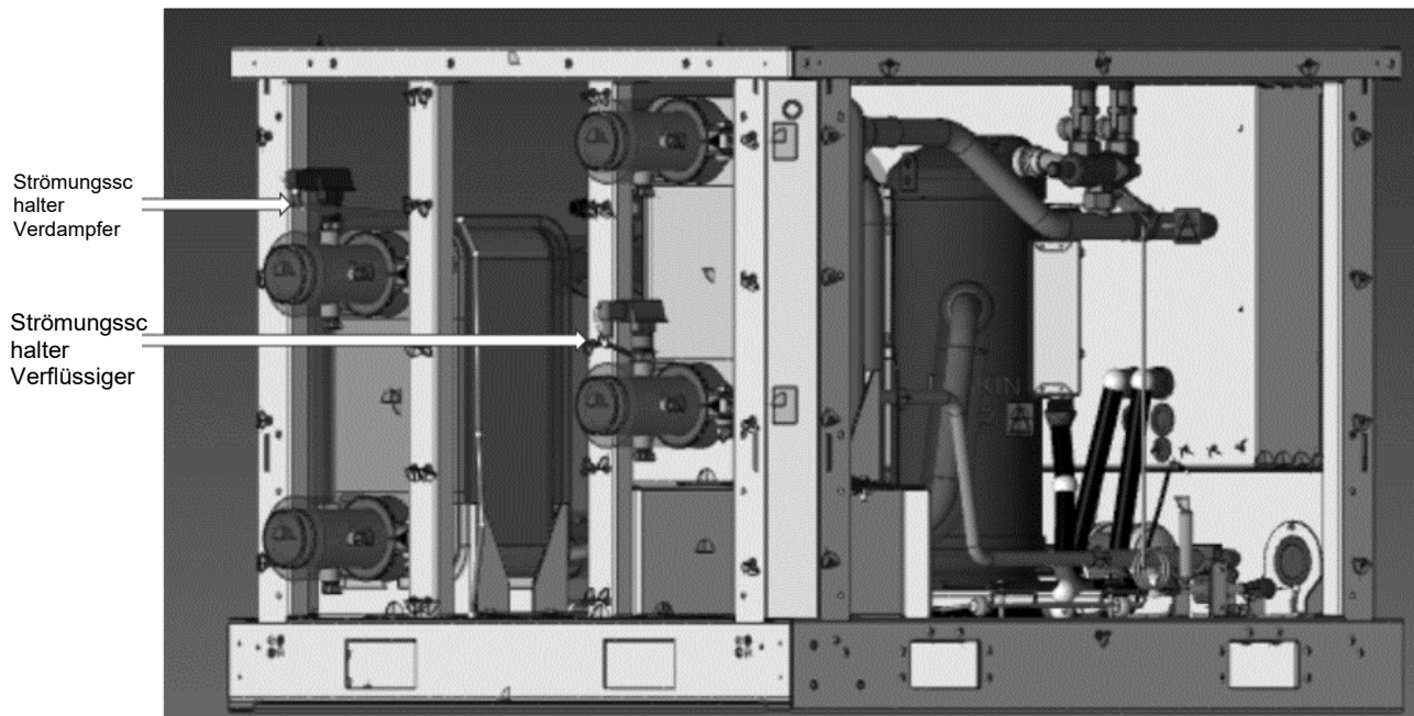
Abb. 16 - Kabelverlegung des Verdampfer-Strömungswächters
