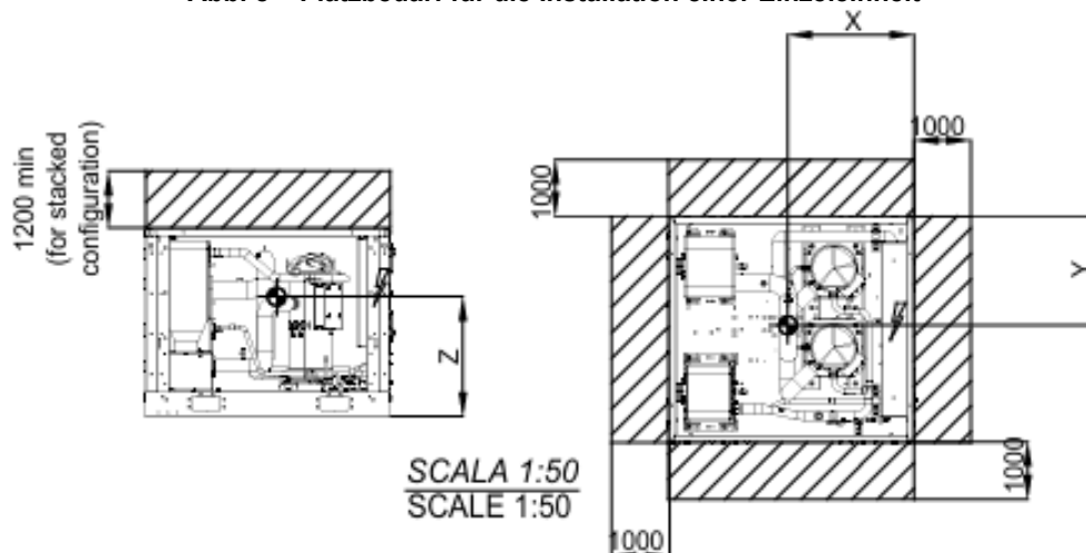
Abb. 8 – Platzbedarf für die Installation einer Einzeleinheit
