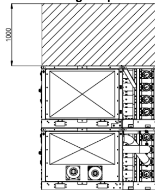
Abb. 10 - Platzbedarf für gestapelte Konfigurationen
