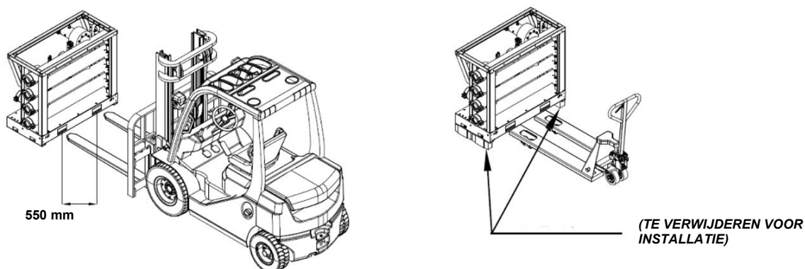
Fig. 47 - Behandeling van verdeelstukmodule
