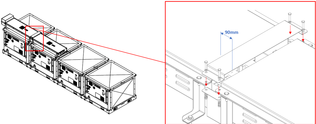
Fig. 56 - De Powerbar-modules met elkaar verbinden
