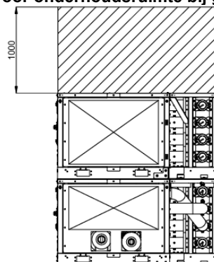
Fig. 10 - Vereisten voor onderhoudsruimte bij gestapelde opstelling
