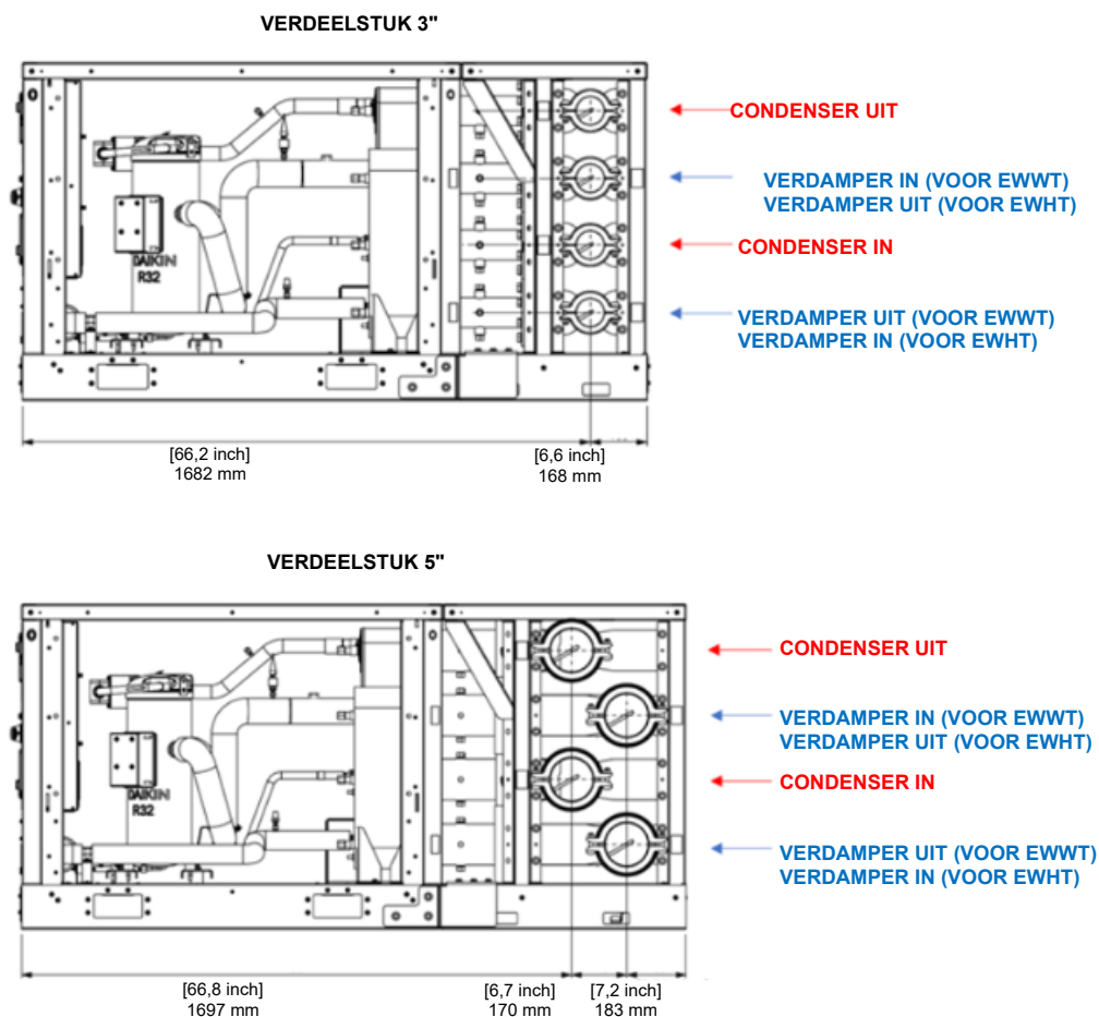
Fig. 30 - Afmetingen waterverdeler
