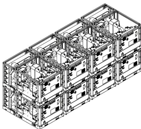
Fig. 44 - Montage-instructies voor meer unit-verdelersystemen samen
