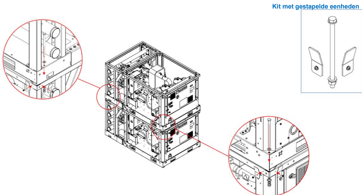
Fig. 43 - Montage-instructies voor gestapelde eenheden
