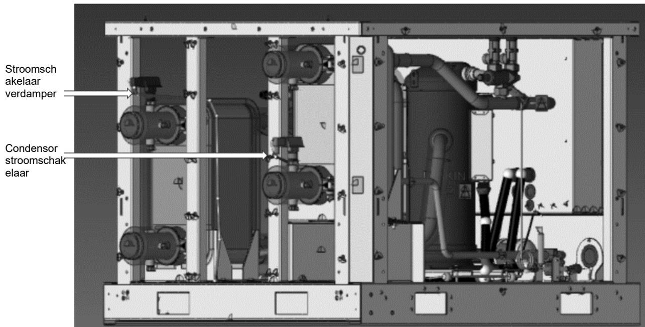
Fig. 16 - Kabels van de stroomschakelaar van de verdamper
