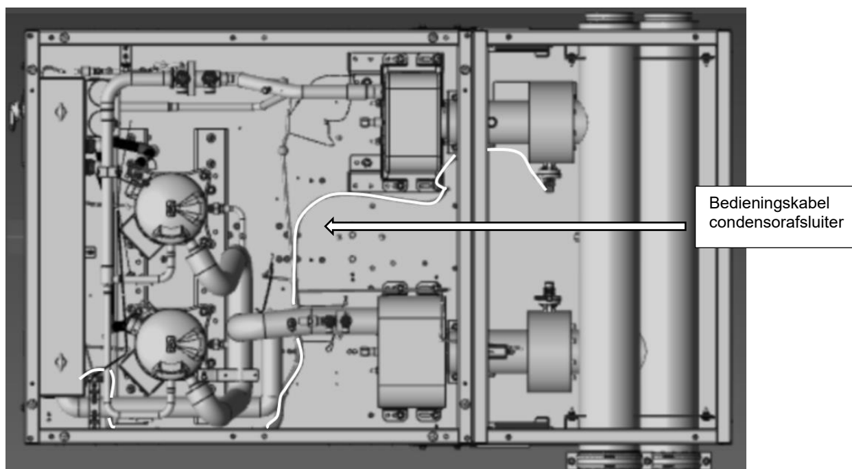
Fig. 40 - Kabelgeleiding van de condensatorafsluiter
