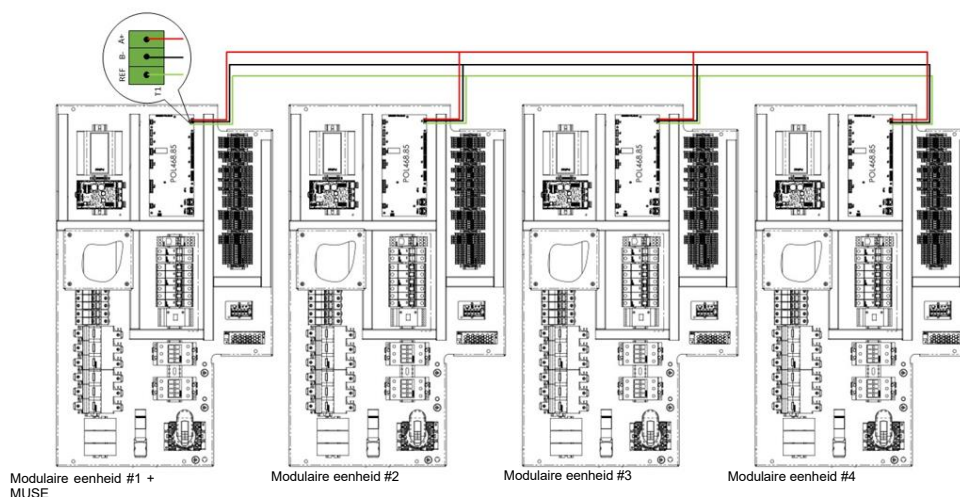
Fig. 64 - Aansluiting van 4 PLC's op hetzelfde Modbus-netwerk
