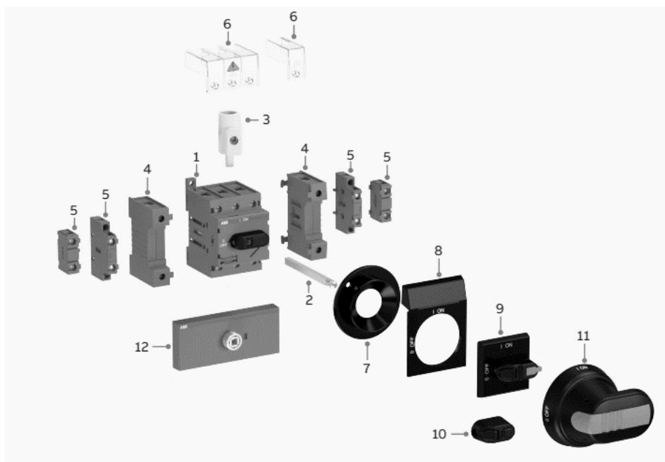
Fig. 23 - Montagehandleiding handgreep
