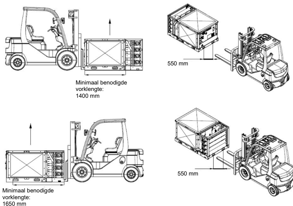
Fig. 48 - Behandeling van unit- en verdeelmodules
