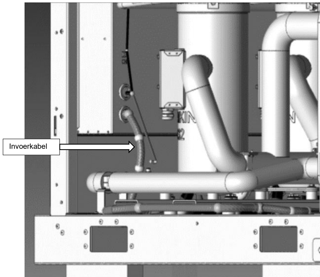
Fig. 41 - Elektrische paneelingang voor bedieningskabels voor verdamper- en condensorafsluitkleppen
