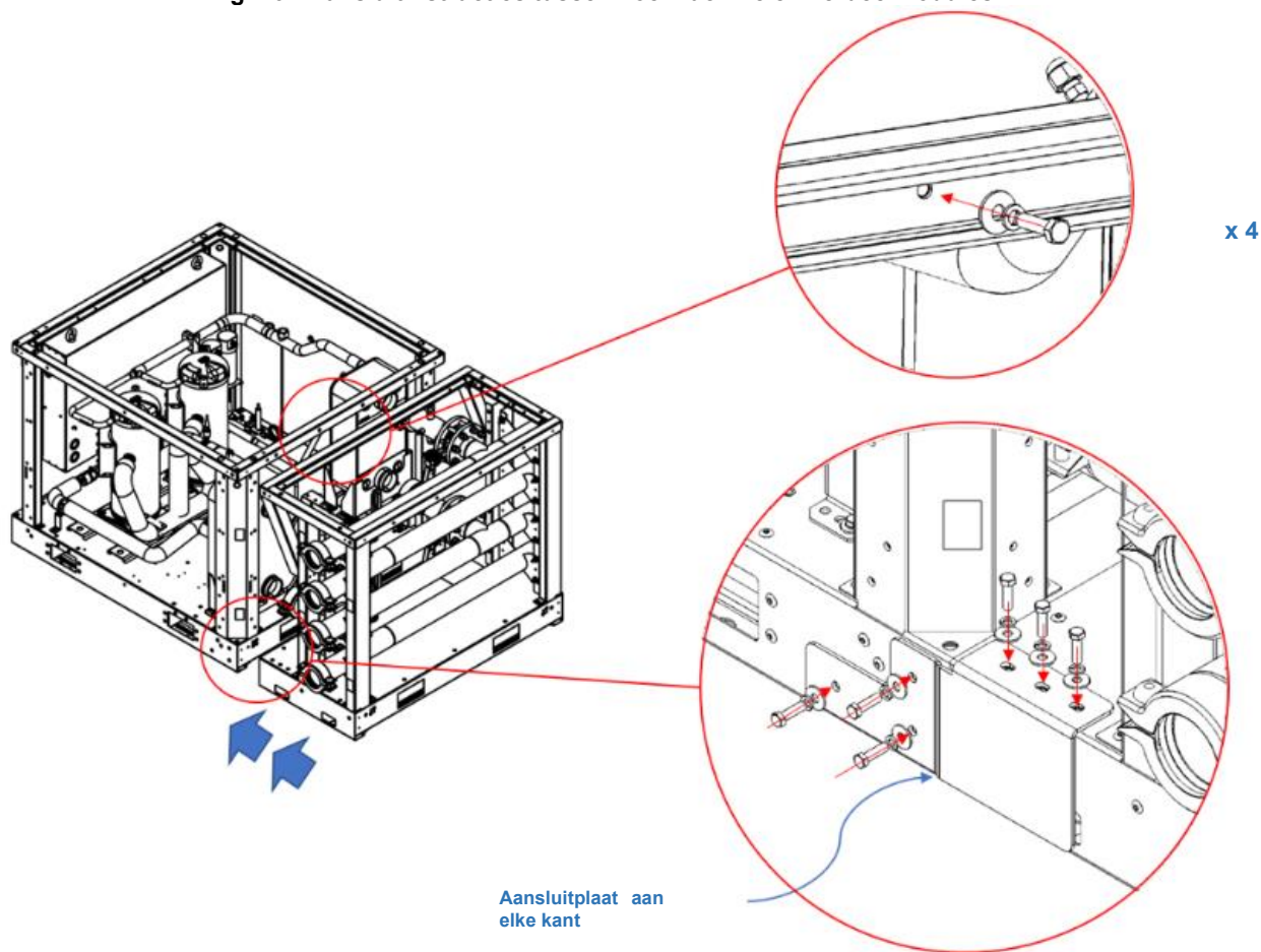
Fig. 26 - Aansluitinstructies tussen koelmachine en verdeelmodules
