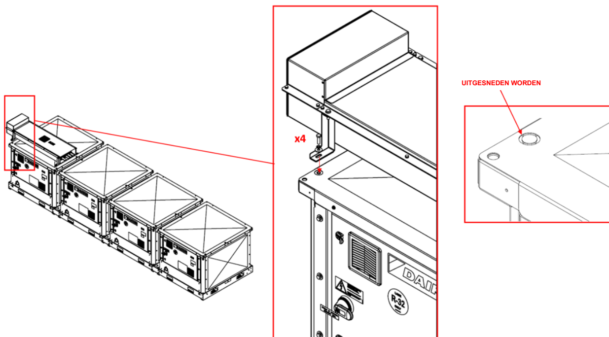
Fig. 55 - Bevestiging van het stroomrailsysteem aan de eenheid
