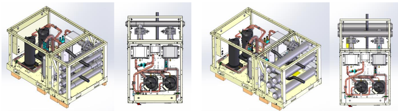
Fig. 27 - PHR-buizen met verdeelmodule (links voor 3inch - rechts voor 5inch-verdeelbuizen)
