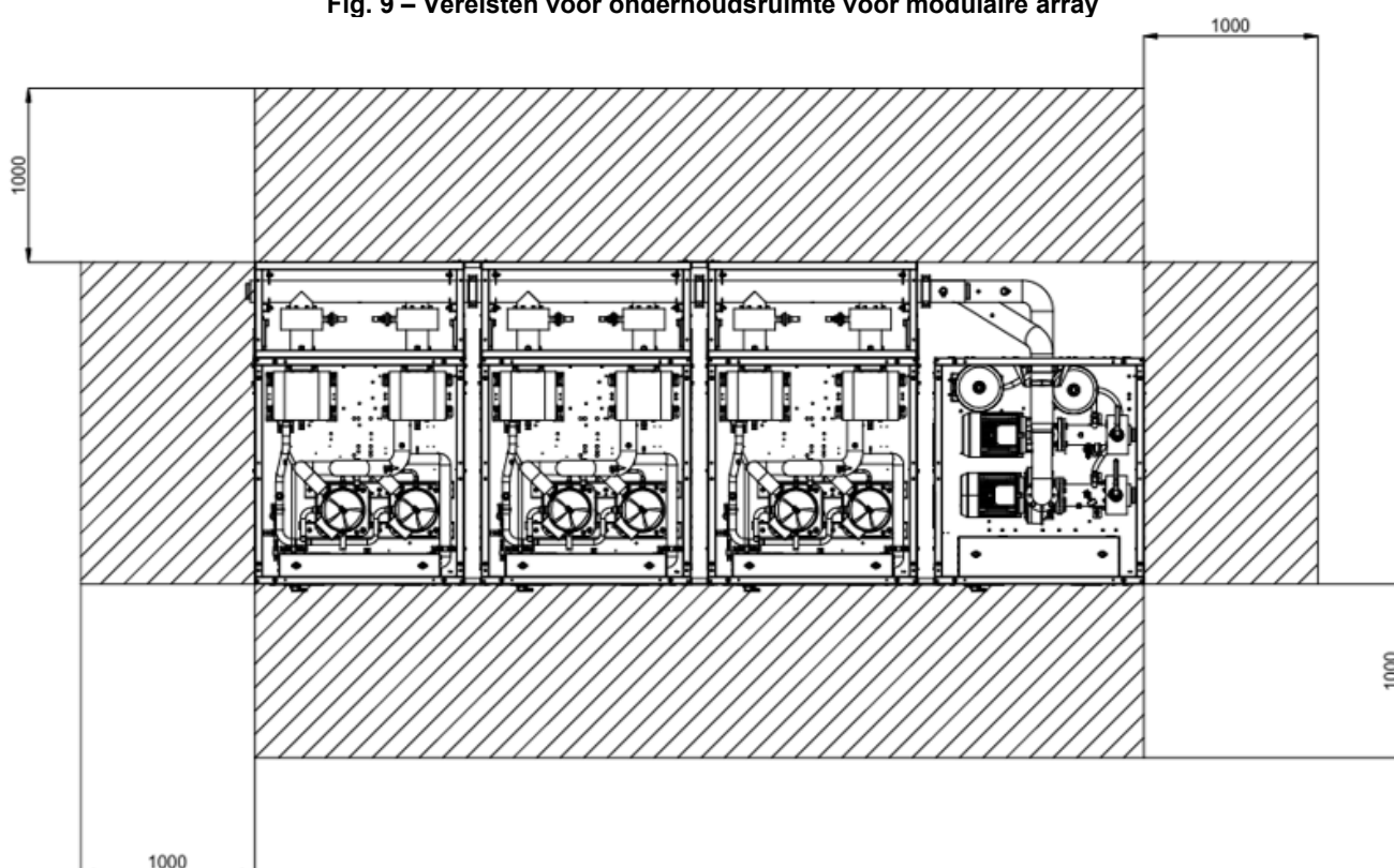
Fig. 9 – Vereisten voor onderhoudsruimte voor modulaire array
