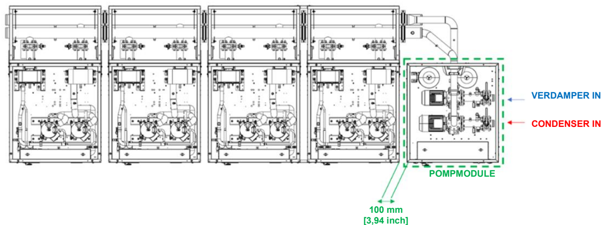
Fig. 46 - Installatie pompmodule - leidingdetails
