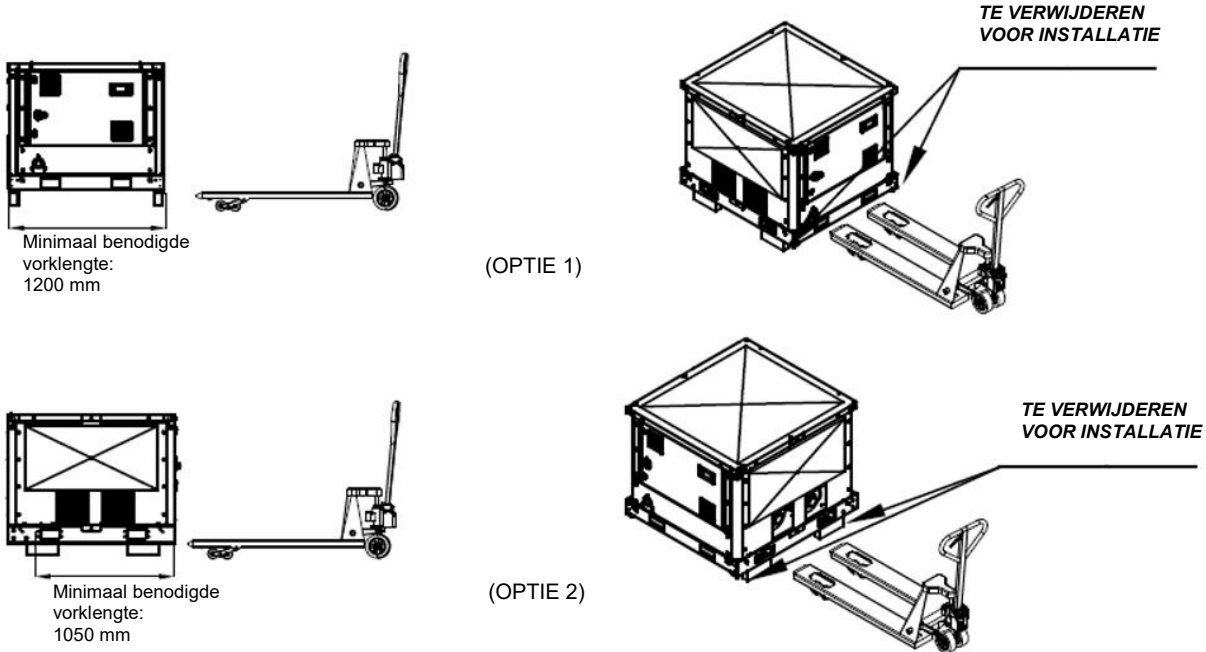
Fig. 51 - Behandeling van pompmodule met behulp van pallettruck
