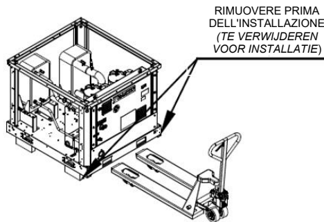
Fig. 13 - Alternatieve transportmethode met pallettruck
