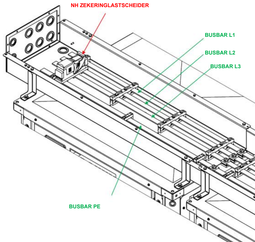
Fig. 58 - Detail van de zekeringen en van de doos voor kabeldoorvoer van de voedingsbalkmodule
