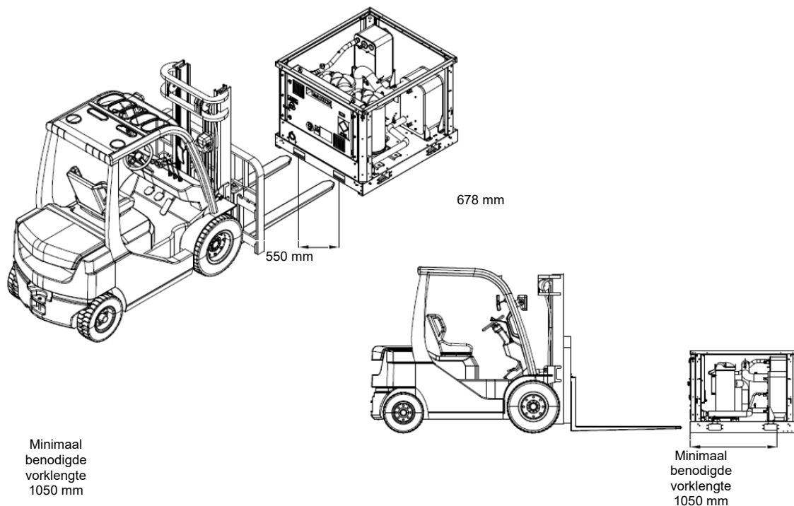
Fig. 12 - Alternatieve transportmethode met vorkheftruck
