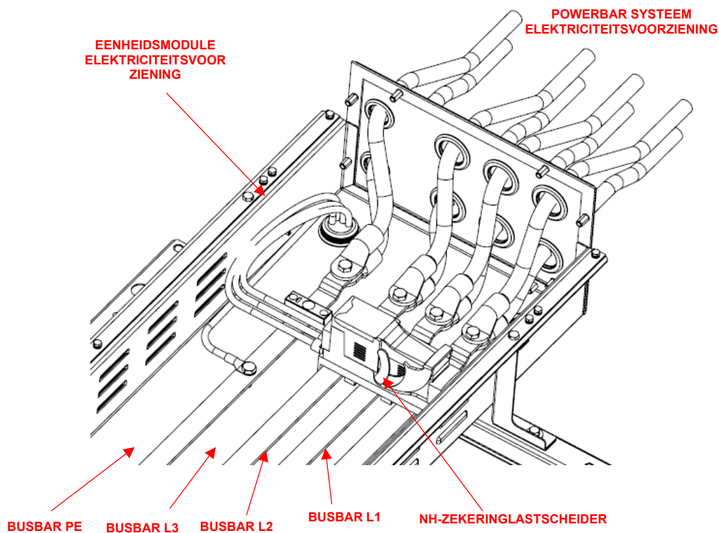
Fig. 59 - Detail van de elektrische aansluiting voor de module van de eerste eenheid
