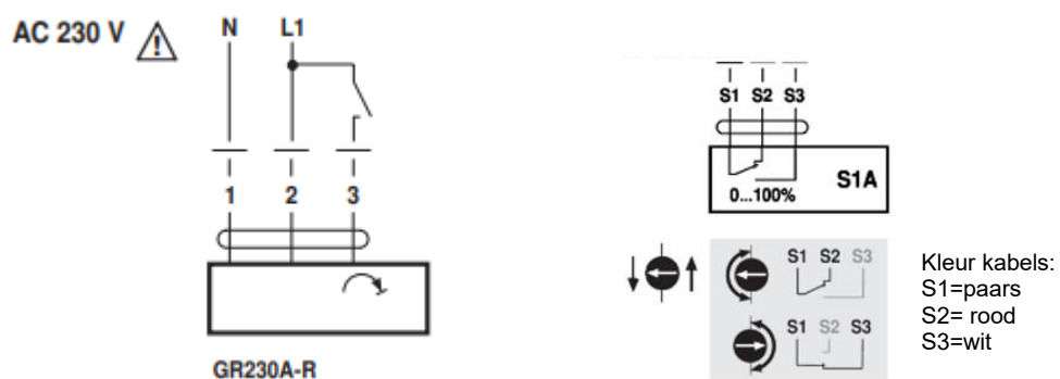
Fig. 35 - Aansluitschema voor motor (linker figuur) en eindschakelaars (rechter figuur)
