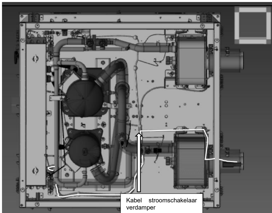
Fig. 16 - Kabels van de stroomschakelaar van de verdamper
