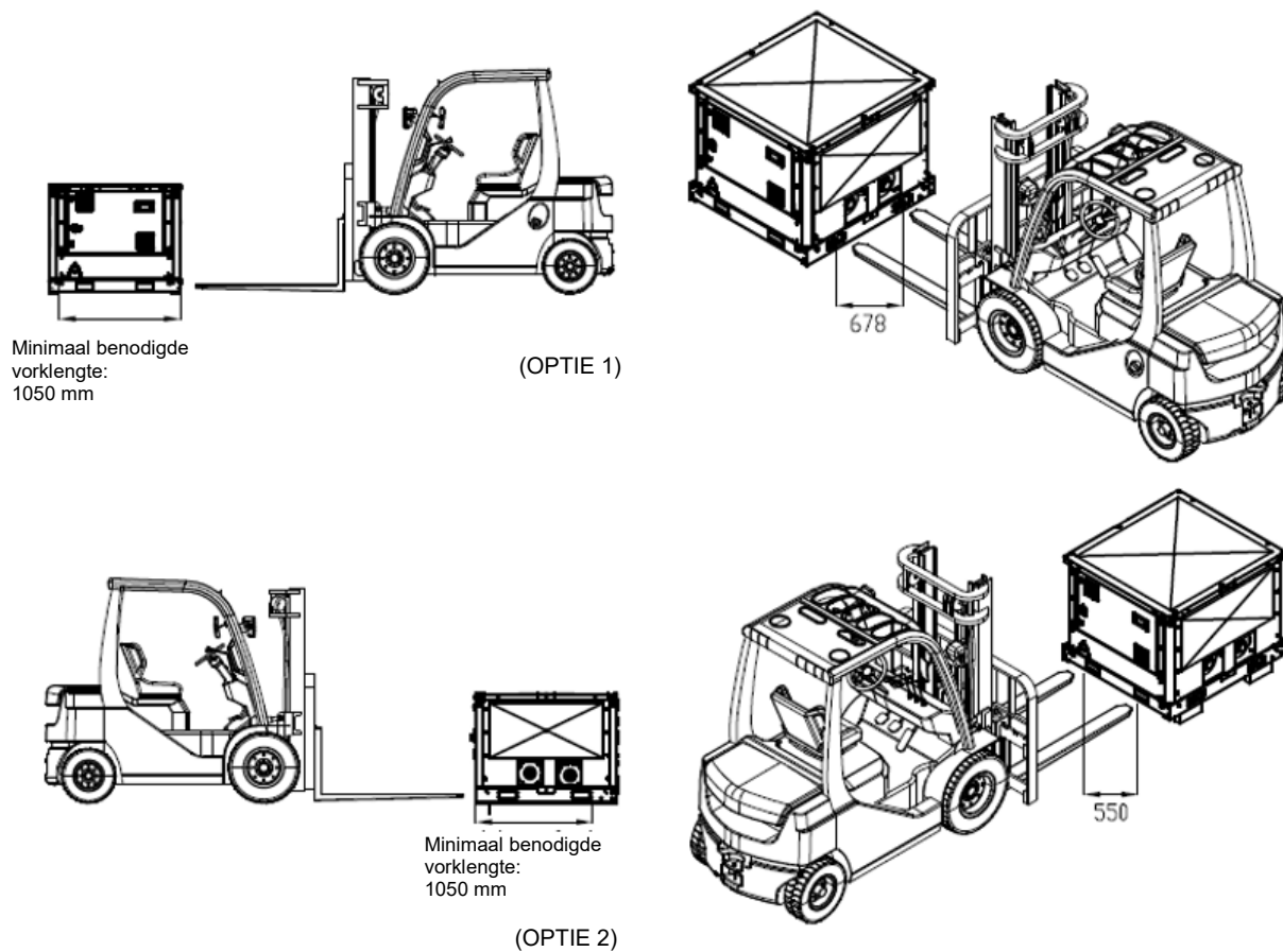
Fig. 50 - Hantering van pompmodule met vorkheftruck
