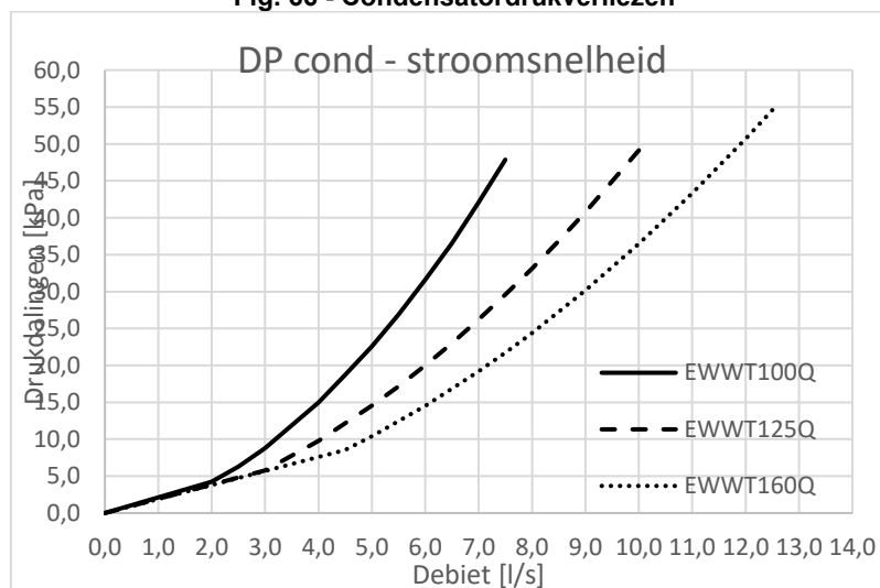
Fig. 66 - Condensatordrukverliezen
