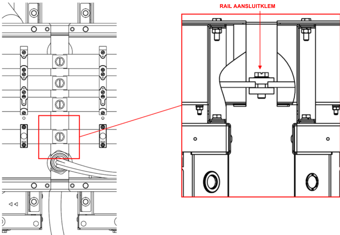
Fig. 57 - Details van de aansluiting van de voedingsbalkmodules
