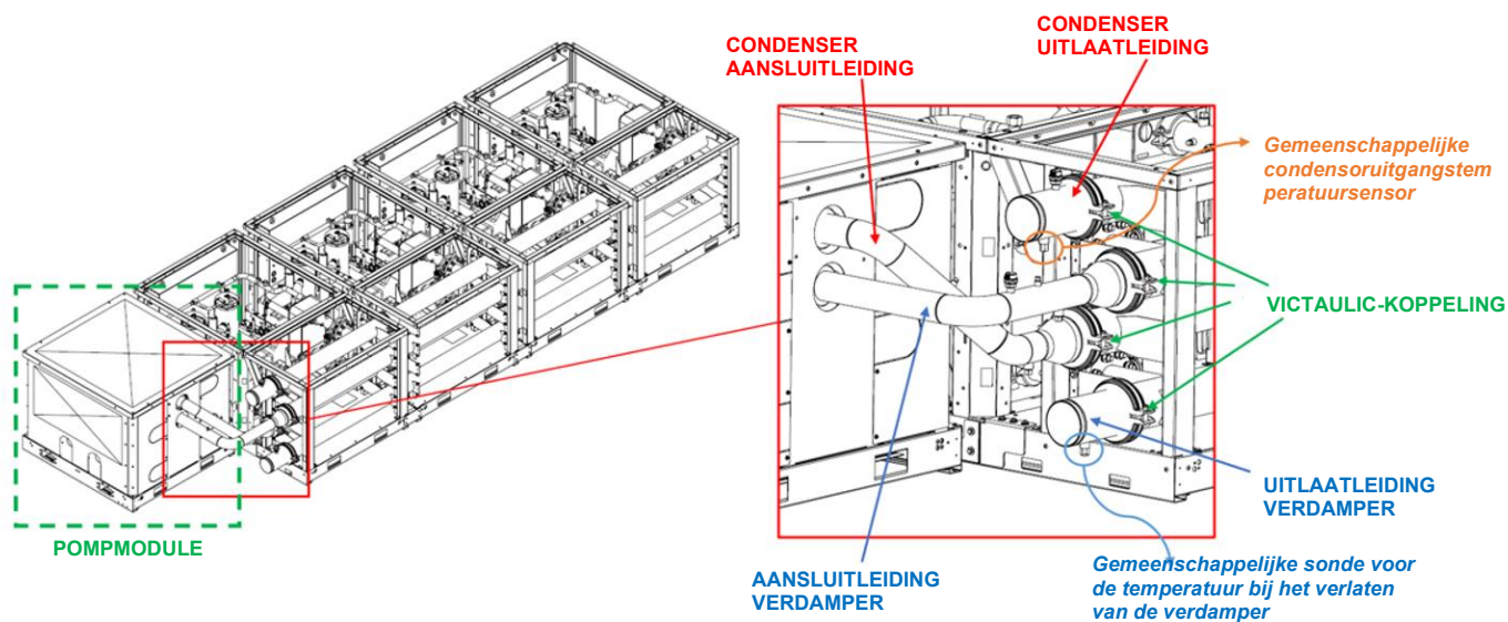
Fig. 63 - Details van de plaatsing van de sondes op de pijpen
