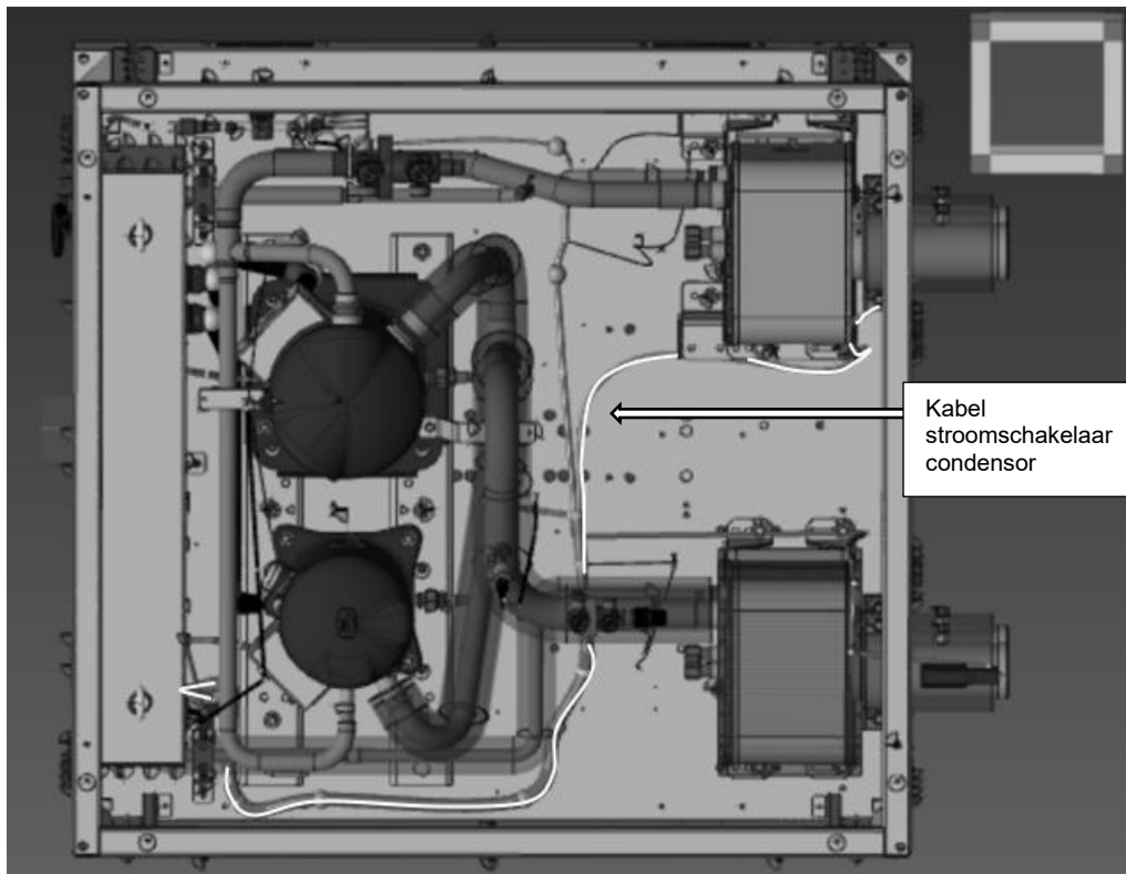
Fig. 18 - Invoerpunt in het elektrische paneel voor stroomschakelaarkabels voor verdamper en condensor
