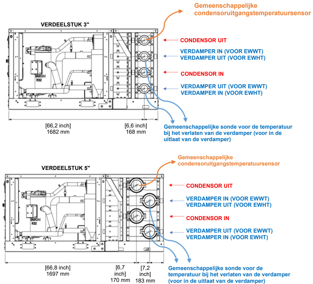
Fig. 62 - Posities van de temperatuursensoren voor 3" en 5" verdeler
