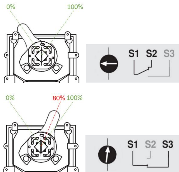
Fig. 42 - Instelling van de trekker van de eindschakelaars
