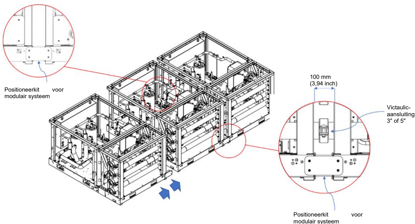
Fig. 29 - Aansluiting modulaire systemen
