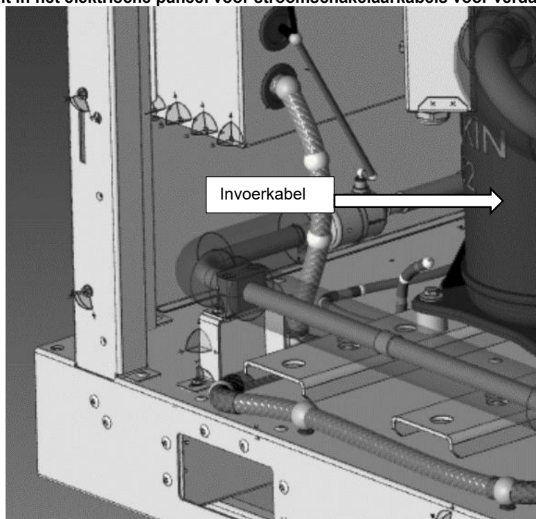
Fig. 18 - Invoerpunt in het elektrische paneel voor stroomschakelaarkabels voor verdamper en condensor
