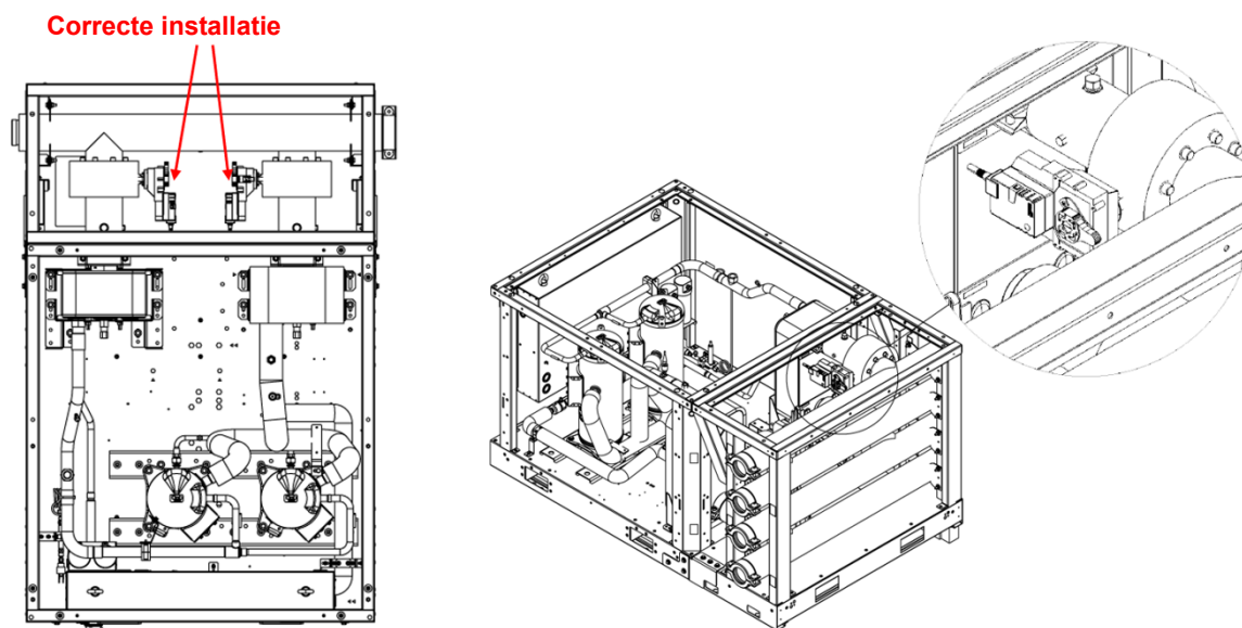
Fig. 34 - Montage-indicaties voor klepaandrijving
