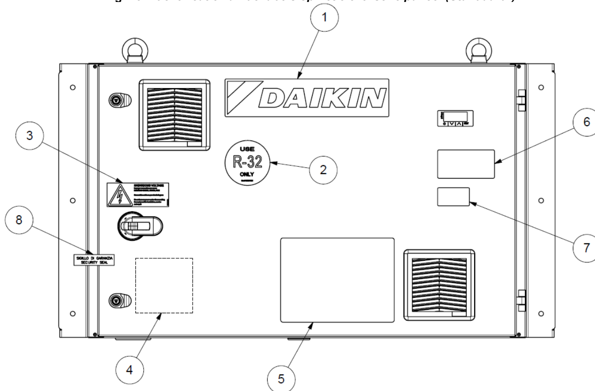
Fig. 25 - Identificatie van de labels op het elektrische paneel (Standaard*)
