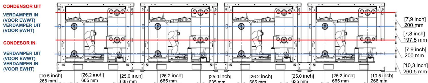
Fig. 28 - Waterleidingconfiguratie
