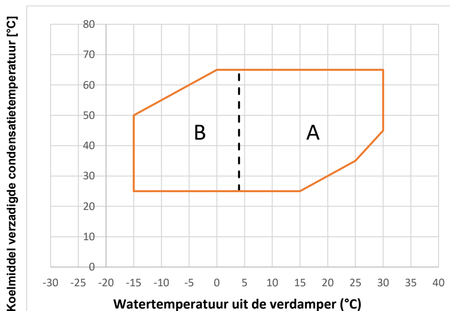
Fig. 7 - EWLT-Q Bedrijfslimieten
