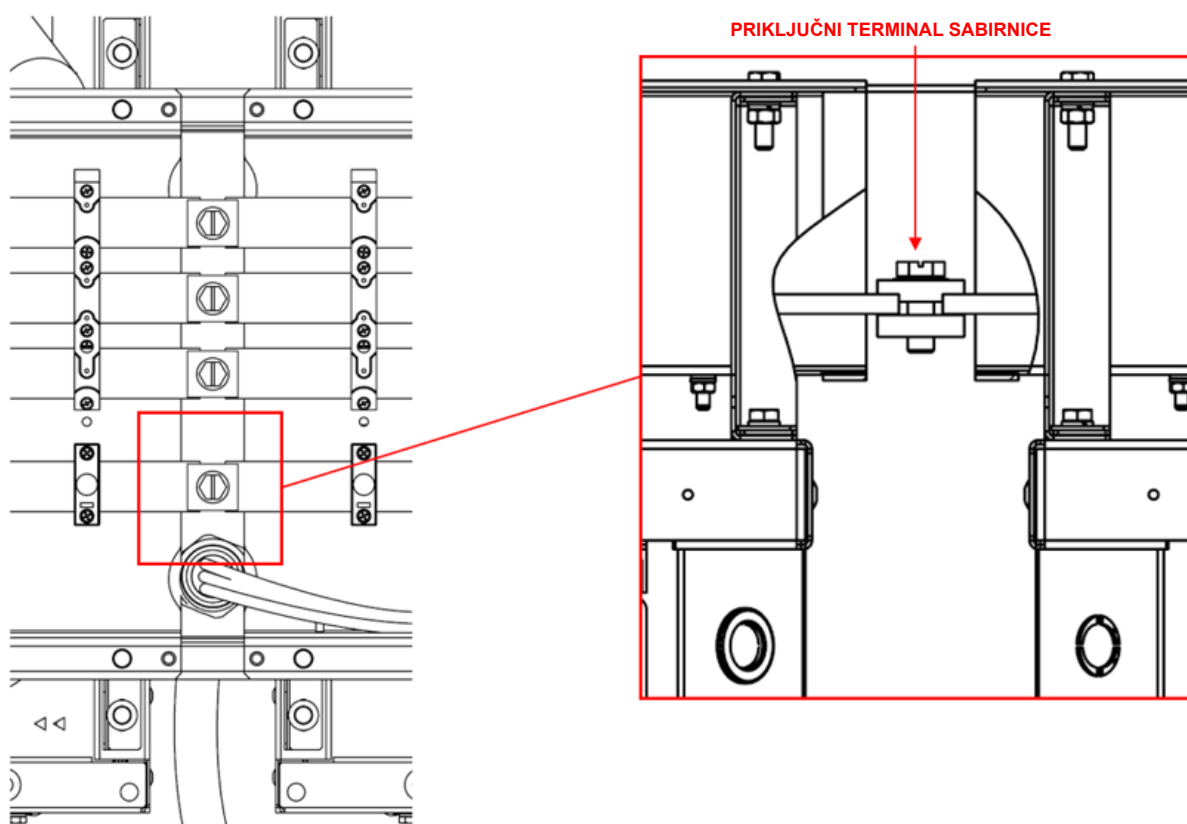
Slika 57 – Pojediniosti o međusobnom povezivanju modula šipki za napajanje
