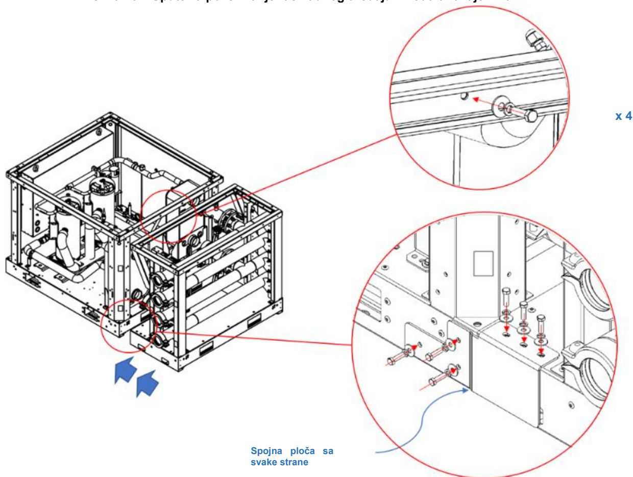
Slika 26 – Upute za povezivanje rashladnog uređaja i modula razdjelnika
