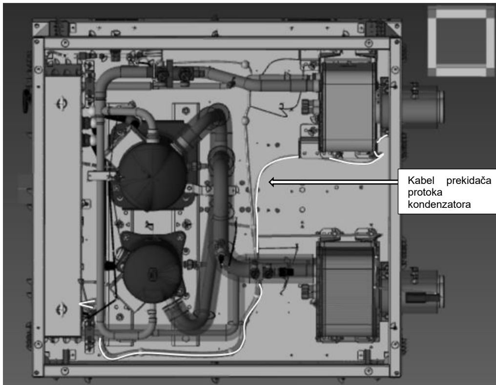
Slika 18 – Ulazna točka na električnoj ploči za kabele prekidača protoka isparivača i kondenzatora
