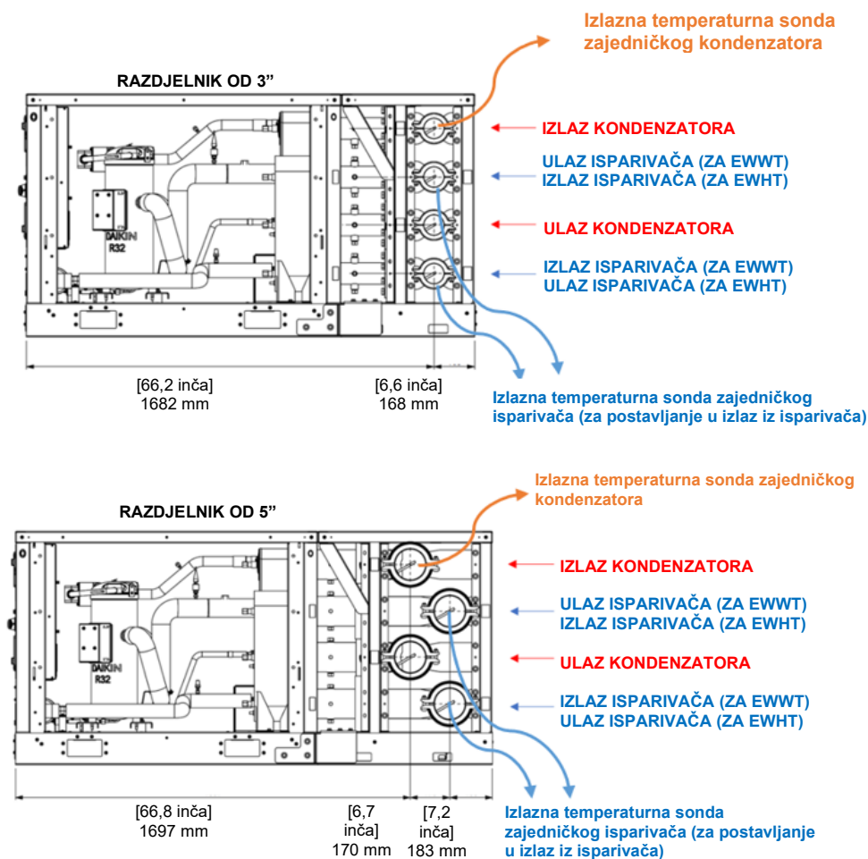
Slika 62 – Položaji temperaturnih sonde za razdjelnik od 3" i 5"
