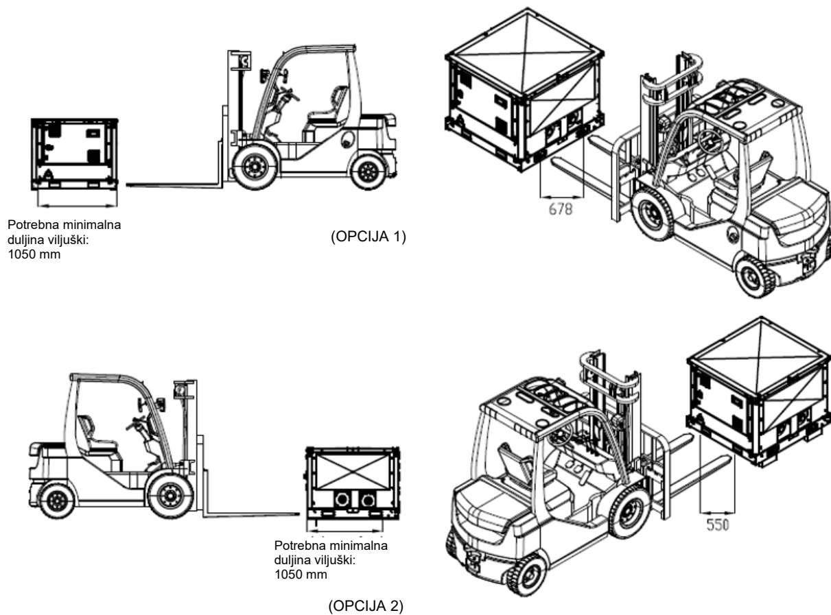
Slika 50 – Rukovanje modulom pumpe pomoću viličara
