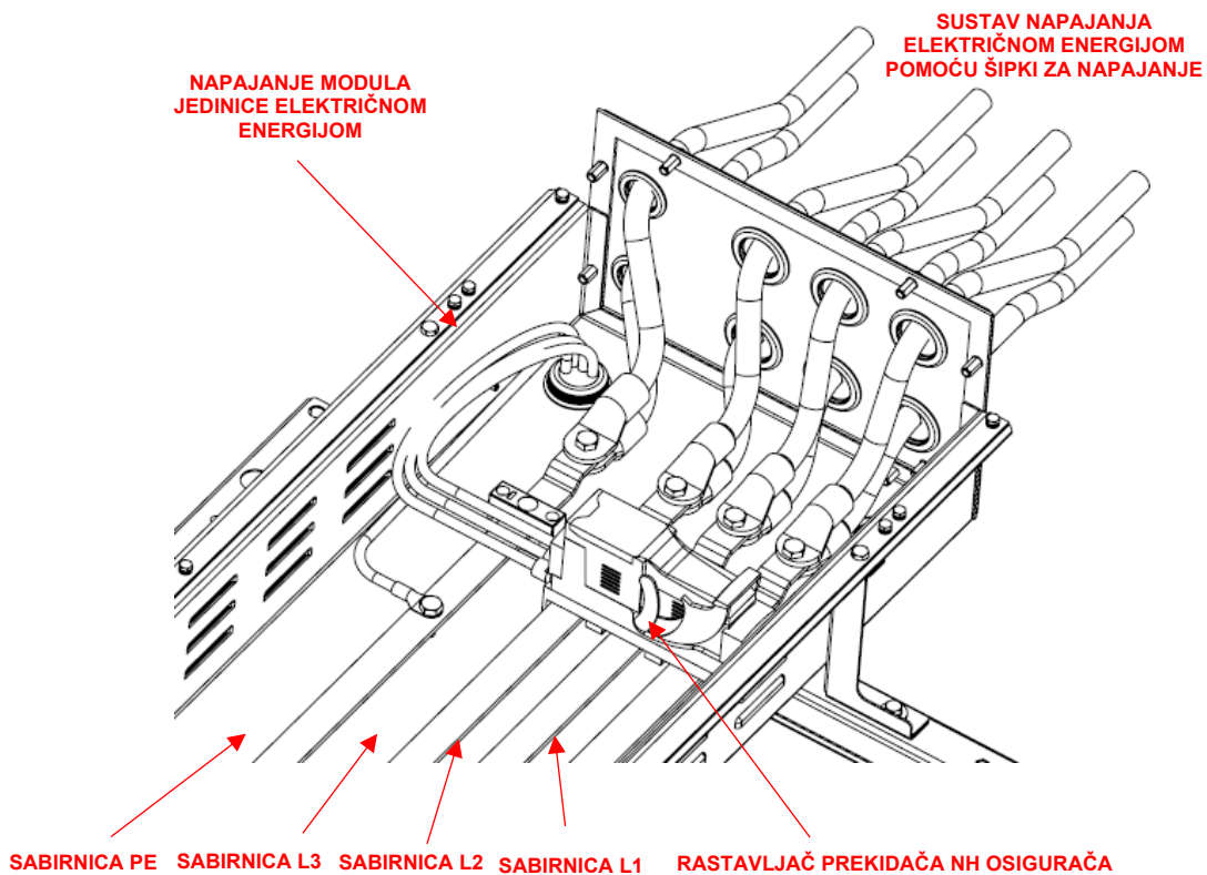
Slika 59 – Pojediniosti o električnom priključku za modul početne jedinice
