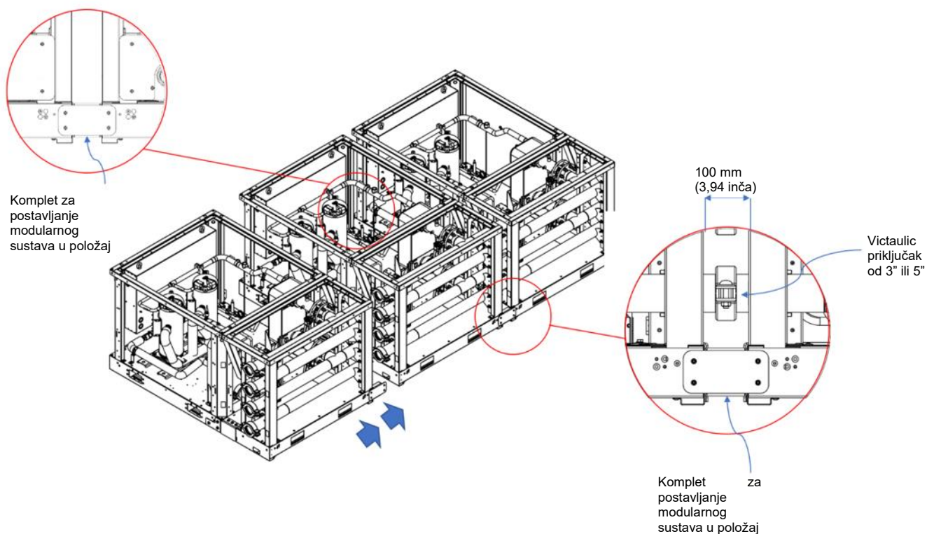
Slika 29 – Povezivanje modularnih sustava
