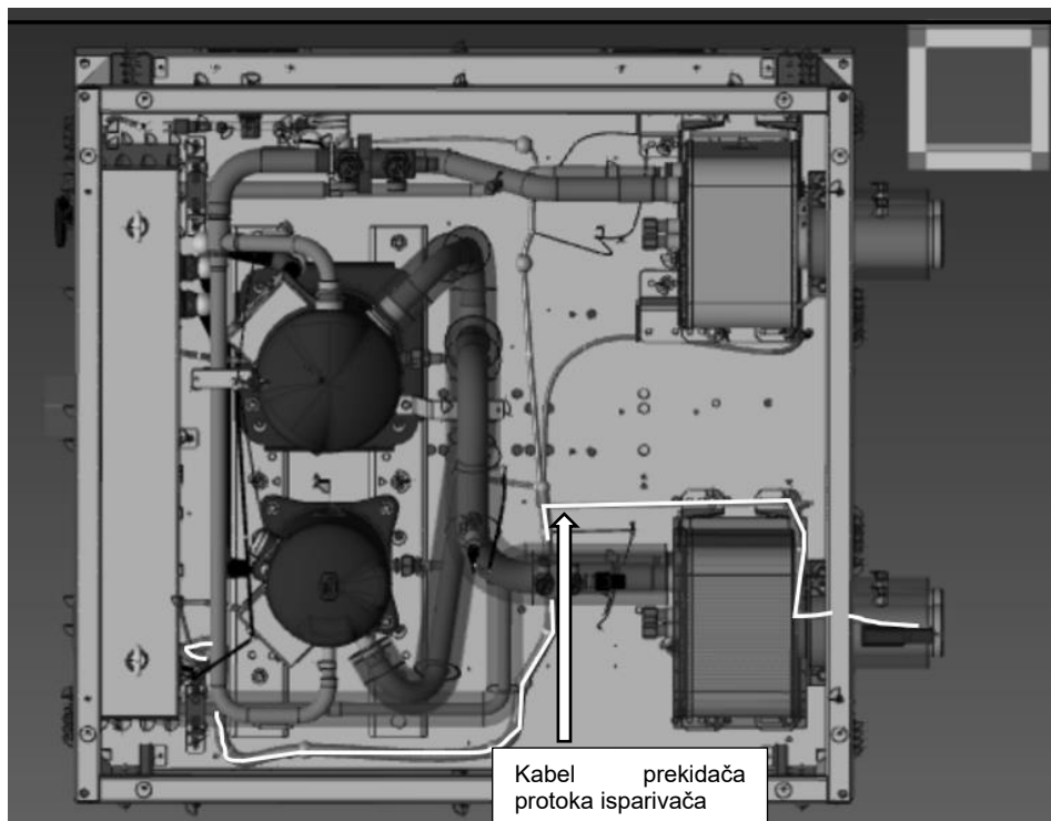
Slika 16 – Trase prekidača protoka kabela isparivača
