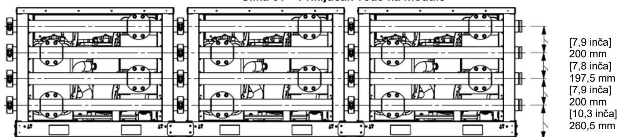
Slika 31 – Priključak vode na module
