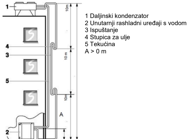
Slika 20 – Spajanje rashladnog kruga (1)
