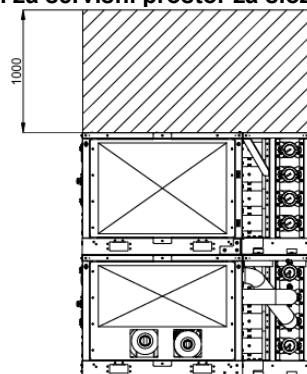
Slika 10- Zahtjevi za servisni prostor za složenu konfiguraciju
