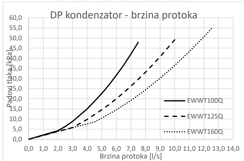
Slika 66 – Padovi tlaka kondenzatora
