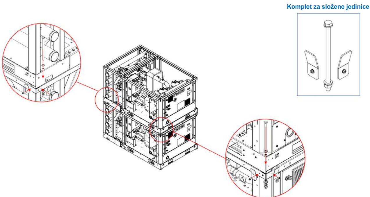
Slika 43 – Upute za montažu složenih jedinica
