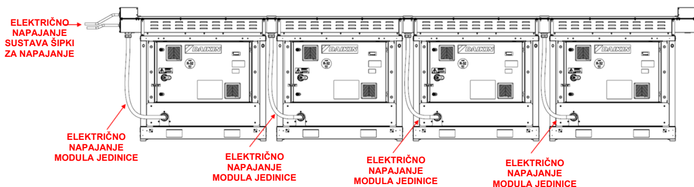
Slika 54 – Pojediniosti o trasiranju kabela
