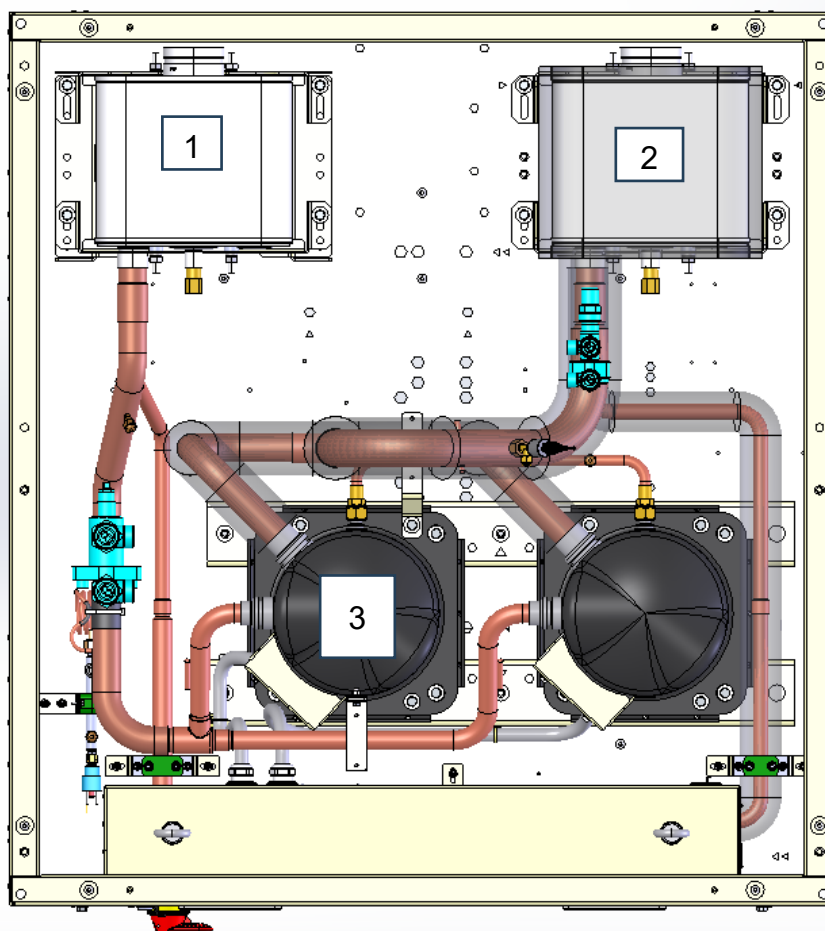
Slika 14 – Referentni nacrt za identifikaciju isparivača i kondenzatora
