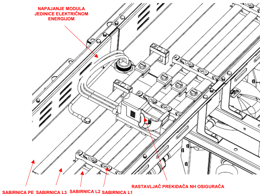
Slika 60 – Pojediniosti o električnom priključku za bilo koji drugi modul jedinice
