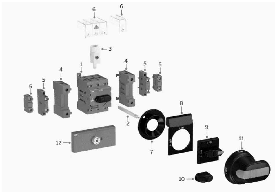
Slika 23 – Upute za sastavljanje ručke
