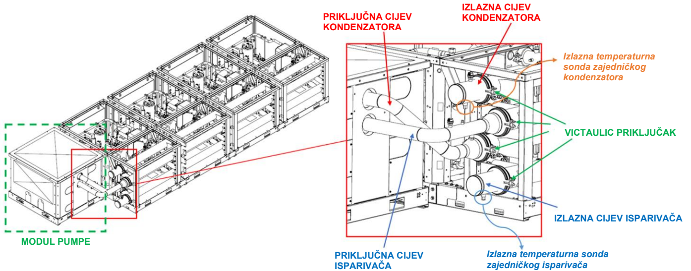
Slika 63 – Pojediniosti postavljanja sonde u položaj na cijevima
