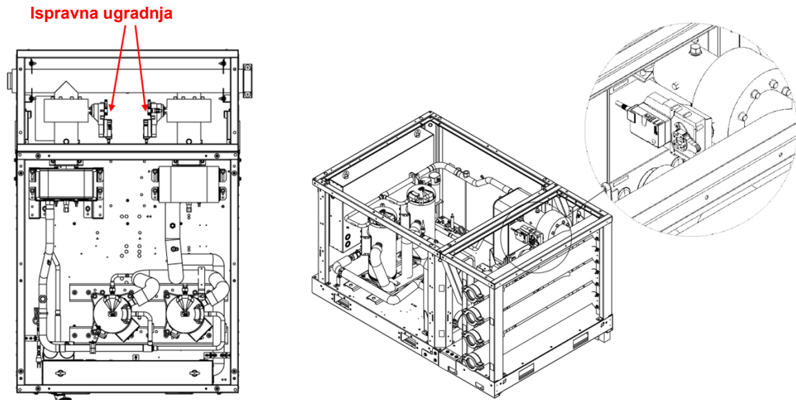
Slika 34 – Indikacije za montažu aktuatora ventila
