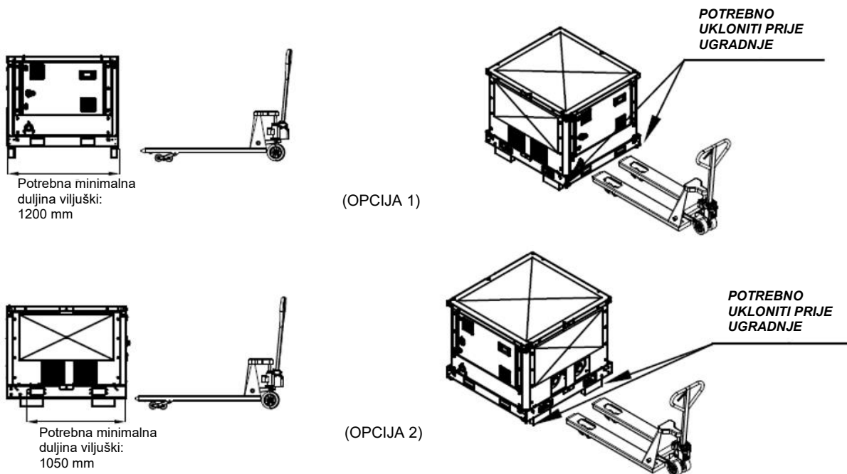
Slika 51 – Rukovanje modulom pumpe pomoću paletnog viličara
