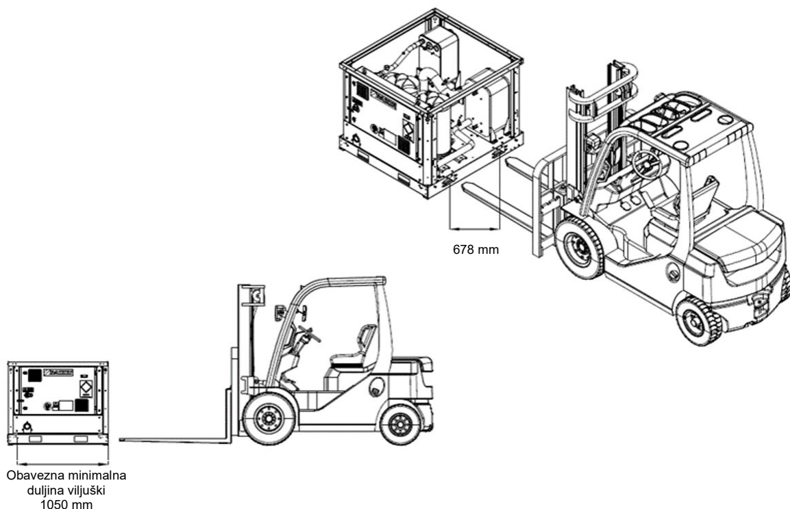
Slika 12 – Alternativni način rukovanja pomoću viličara
