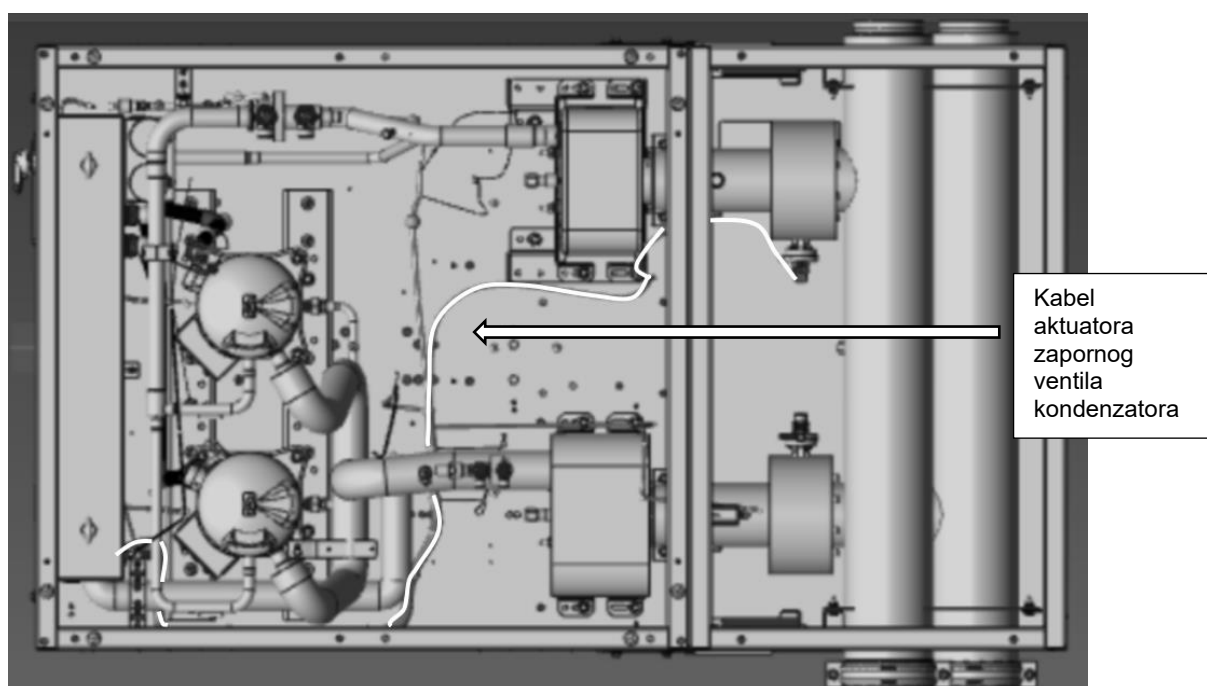
Slika 40 – Trase kabla aktuatora zapornog ventila kondenzatora
