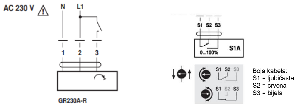
Slika 35 – Shema ožičenja motora (lijeva slika) i graničnih prekidača (desna slika)
