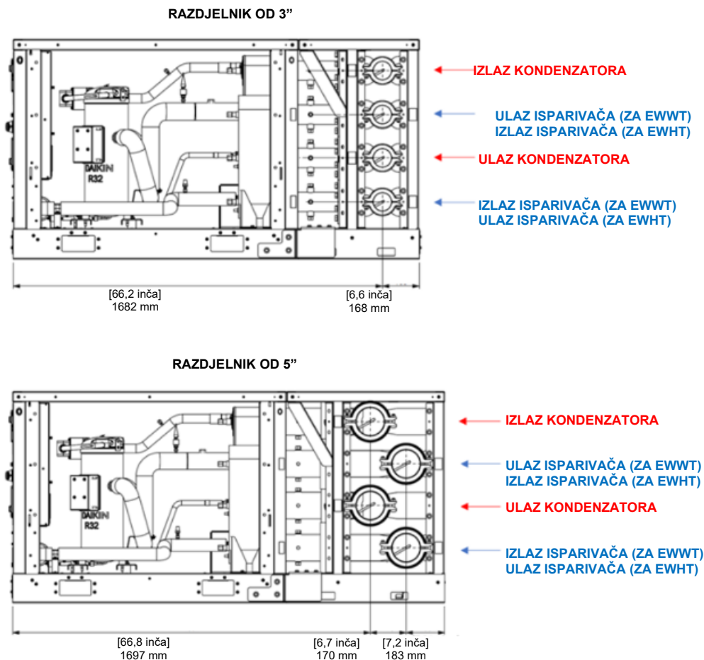
Slika 30 – Veličine razdjelnika za vodu
