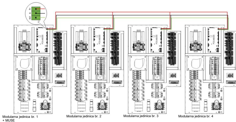
Slika 64 – Spajanje 4 PLC-a na istu Modbus mrežu
