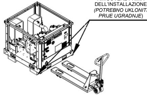
Slika 13 – Alternativni način rukovanja pomoću paletnog viličara
