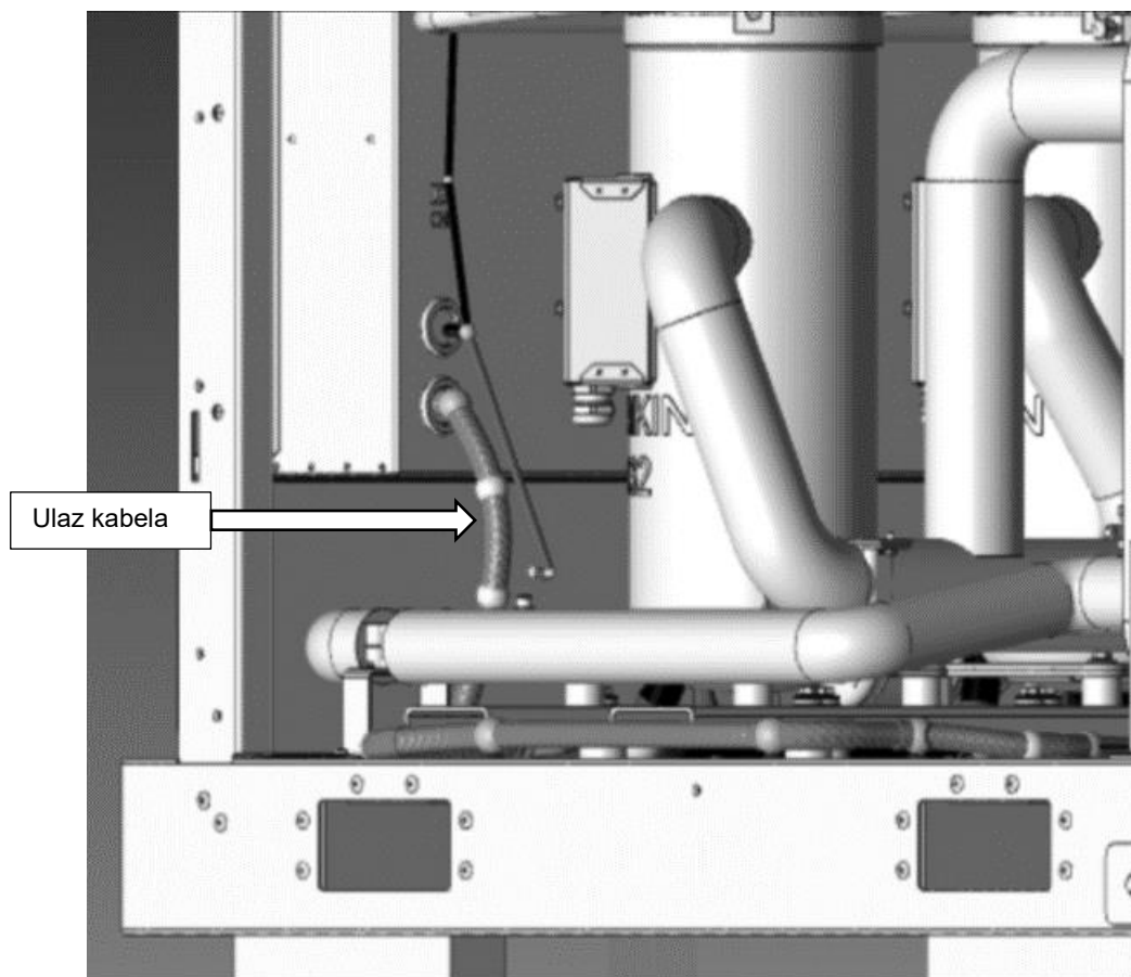
Slika 41 – Ulaz na električnoj ploči za kabele aktuatora zapornog ventila isparivača i kondenzatora
