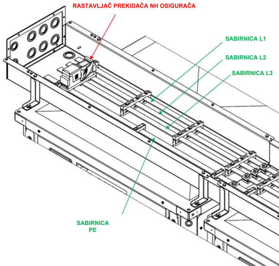
Slika 58 – Pojediniosti o osiguračima i kutiji za trasiranje kabela modula šipke za napajanje
