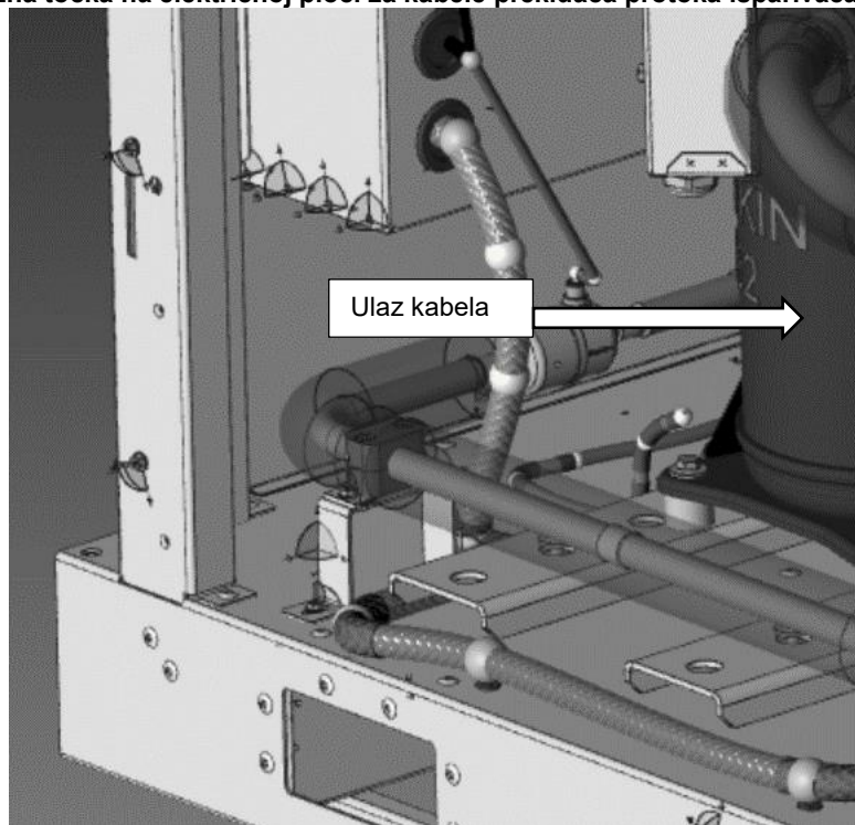
Slika 18 – Ulazna točka na električnoj ploči za kabele prekidača protoka isparivača i kondenzatora
