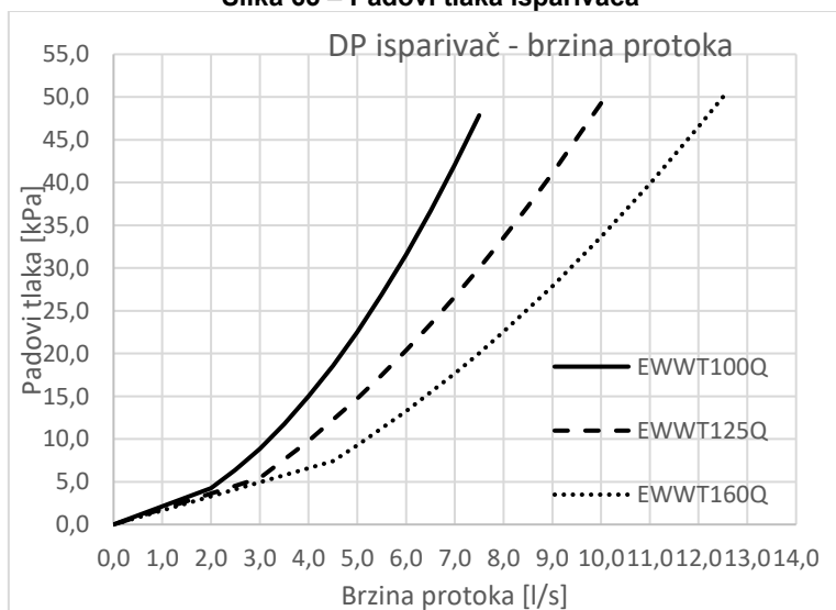
Slika 65 – Padovi tlaka isparivača
