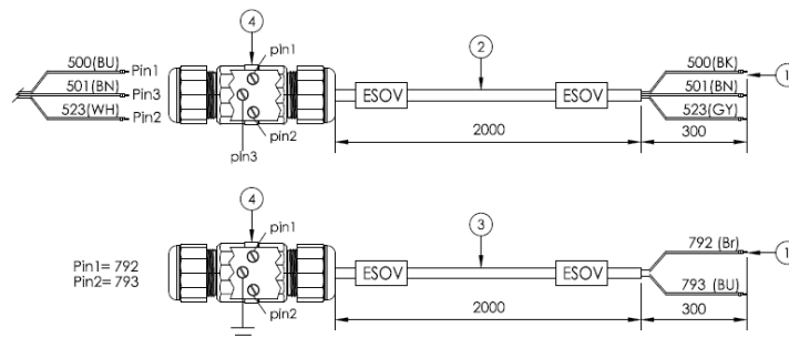
Slika 37 – Adapteri za kabele za aktuator zapornog ventila kondenzatora i granične prekidače
