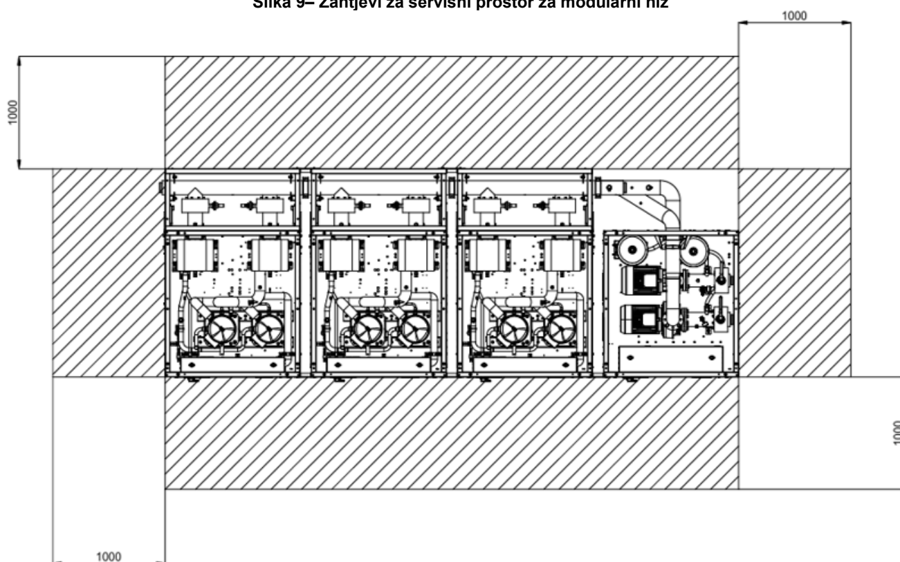
Slika 9– Zahtjevi za servisni prostor za modularni niz
