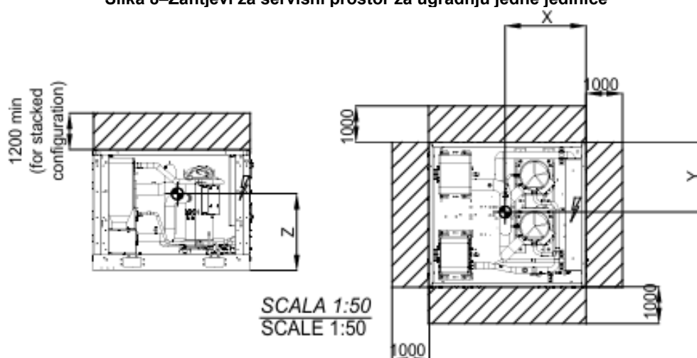
Slika 8–Zahtjevi za servisni prostor za ugradnju jedne jedinice
