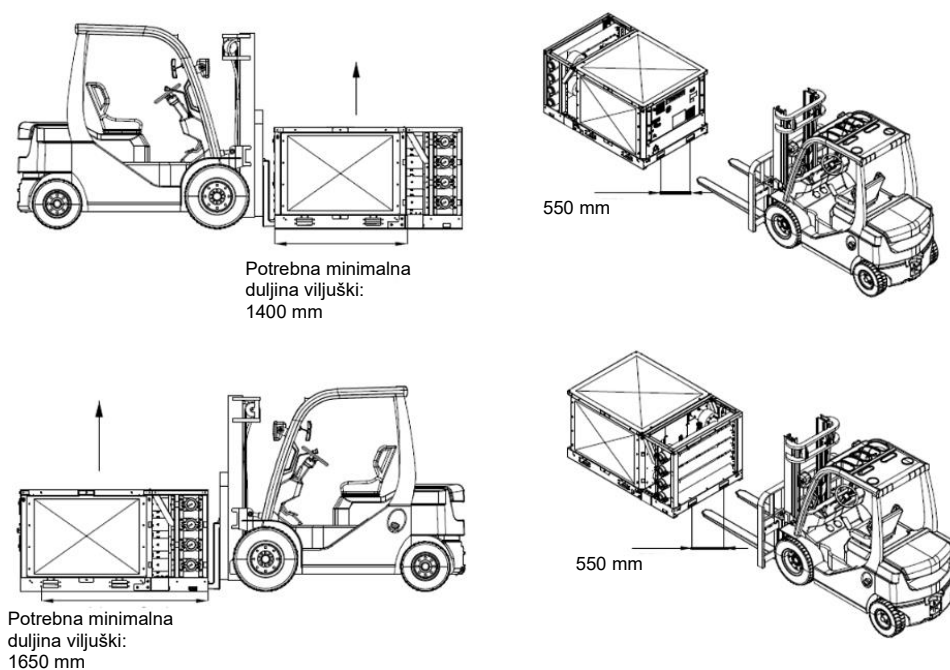
Slika 48 – Rukovanje jedinicom i modulima razdjelnika
