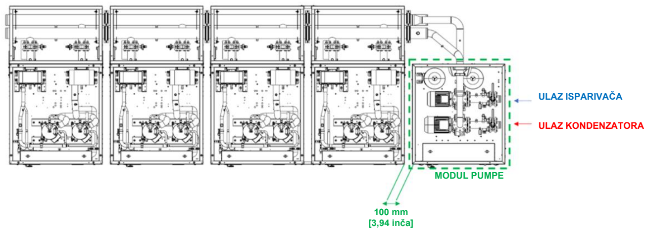
Slika 45 – Ugradnja modula pumpe
