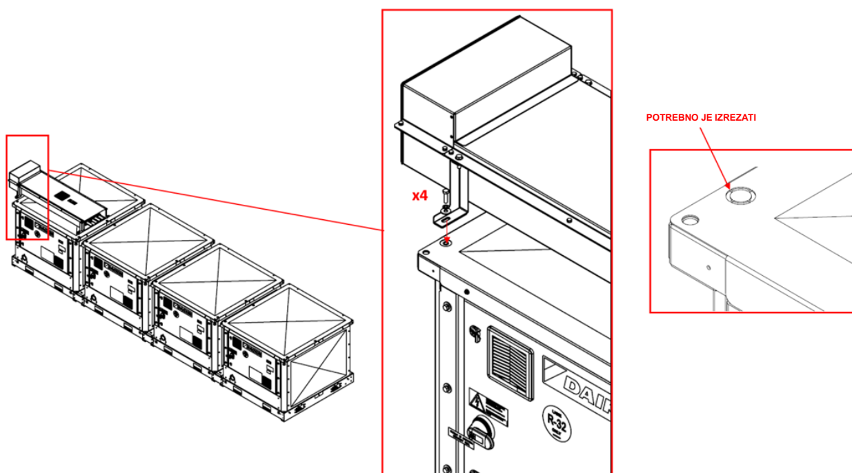
Slika 55 – Pričvršćivanje sustava šipki za napajanje na jedinicu
