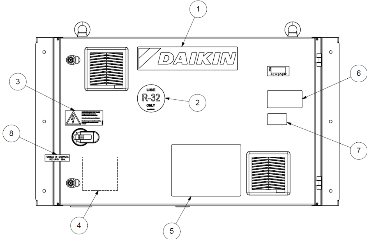
24. ábra - Az elektromos panelen elhelyezett címkek azonosítása (Standard*)
