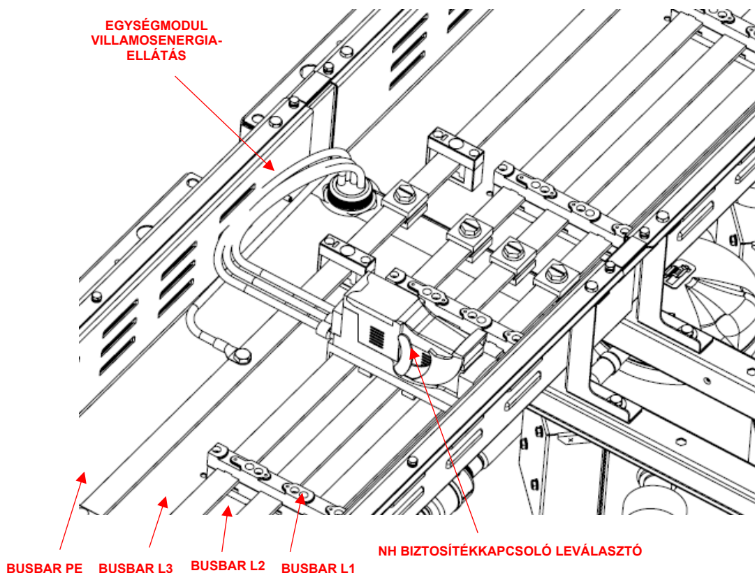
59. ábra - Az elektromos csatlakozás részletei bármely más egységmodulhoz
