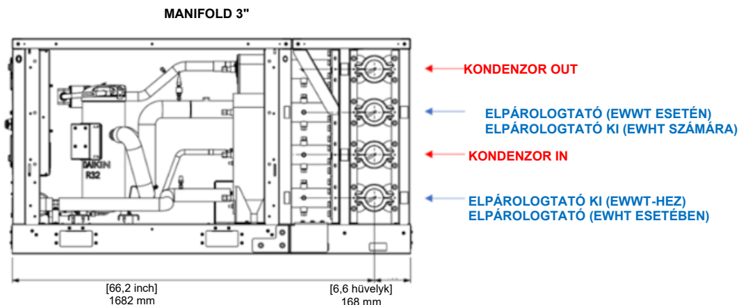
29. ábra - Vízugyjtőcső méretek
