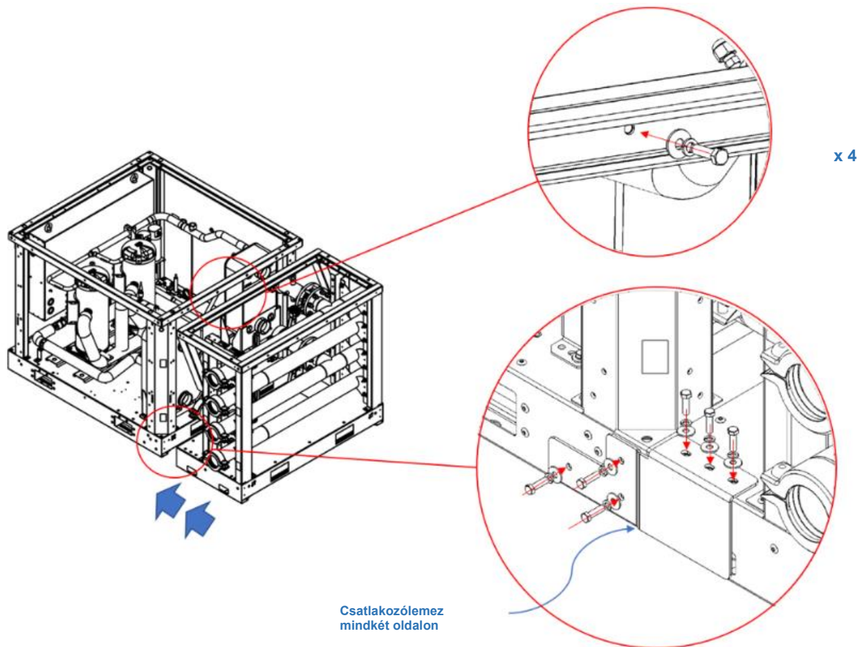
25. ábra - Csatlakozási utasítások a hűtő és a gyűjtőmodulok között
