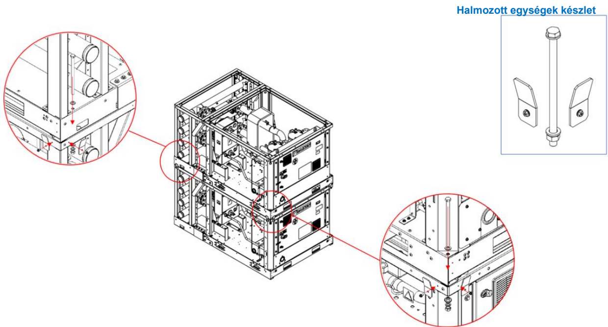
42. ábra - Szerelési utasítások egymásra helyezett egységekhez
