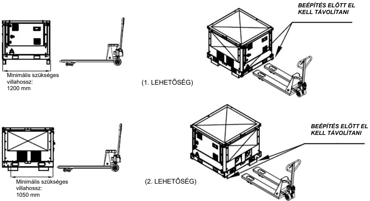
50. ábra - A szivattyúmodul kezelése raklapos targonccal
