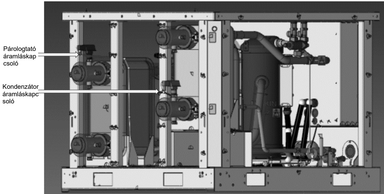
15. ábra - Az elpárologtató áramláskapcsoló kábeleinek elvezetése
