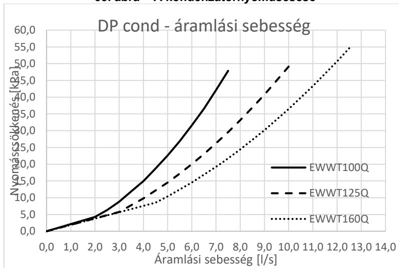
65. ábra - A kondenzátor nyomásesése
