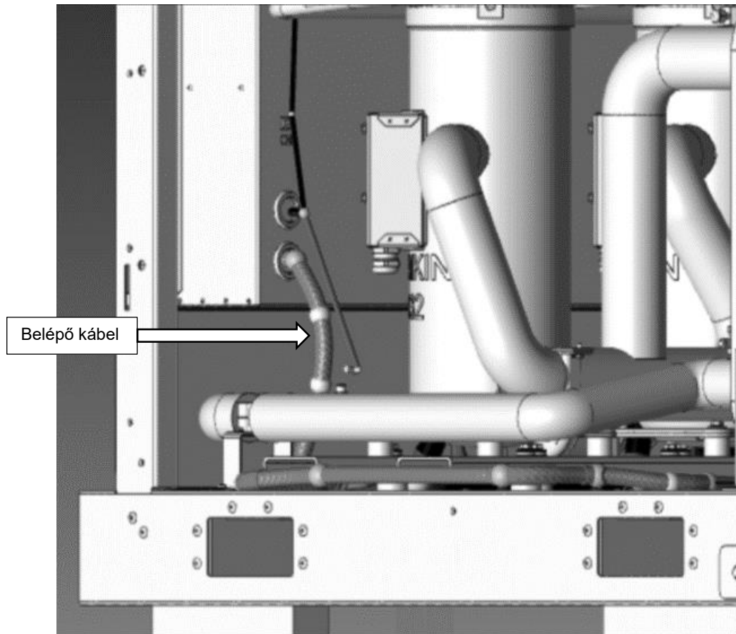
40. ábra - Az elpárolgató és a kondenzátor elzárószelep működtetőszelvényének kábeleinek elektromos panelbejárata
