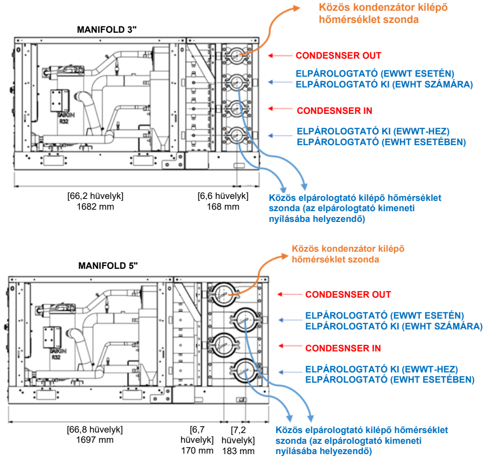
61. ábra - A hőmérséklet-szondák helyzete a 3" és 5" gyűjtőcsőhöz
