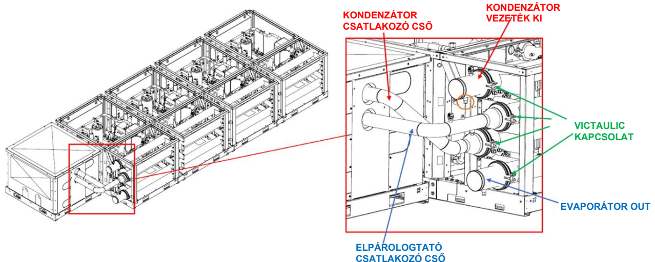
45. ábra - Szivattyúmodul telepítése - csővezetékek részletei
