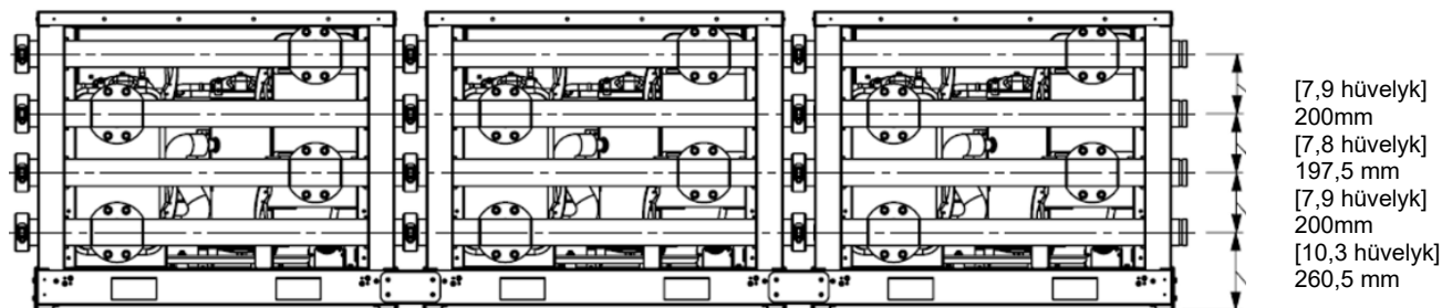
30. ábra - Vízcsatlakozás a modulokhoz
