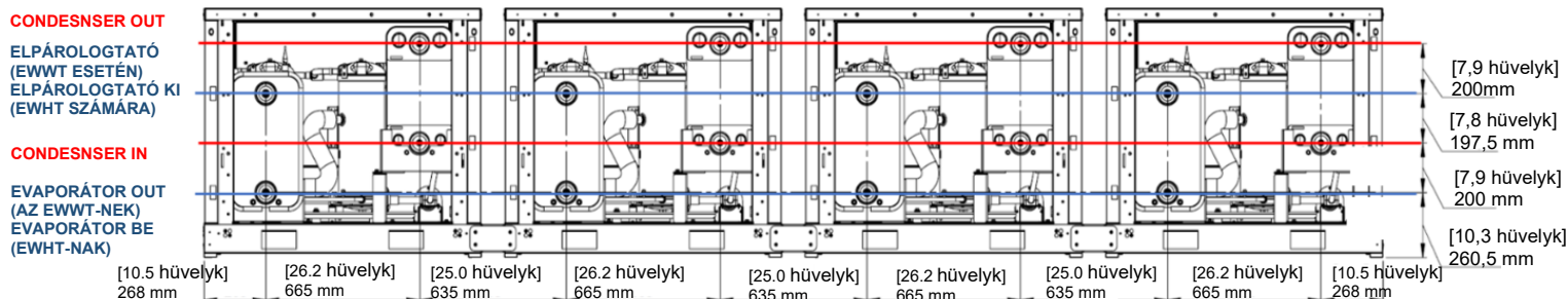
27. ábra - Vízvezeték-konfiguráció
