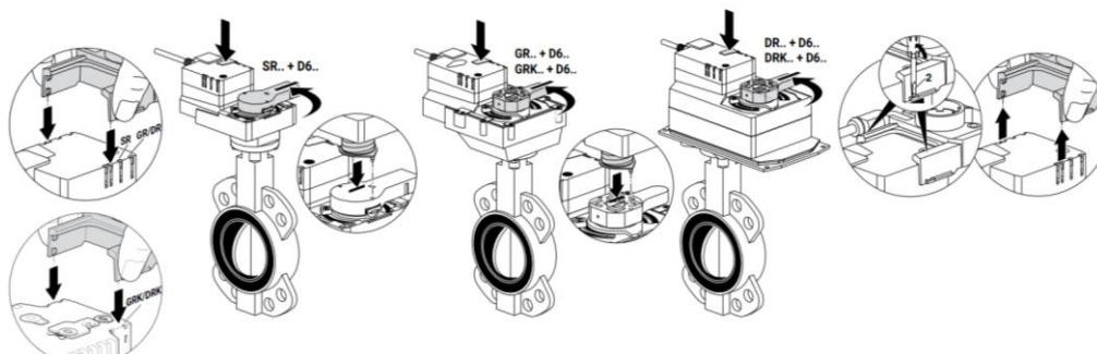
32. ábra - Szerelési utasítások a működtető végálláskapcsolóhoz
