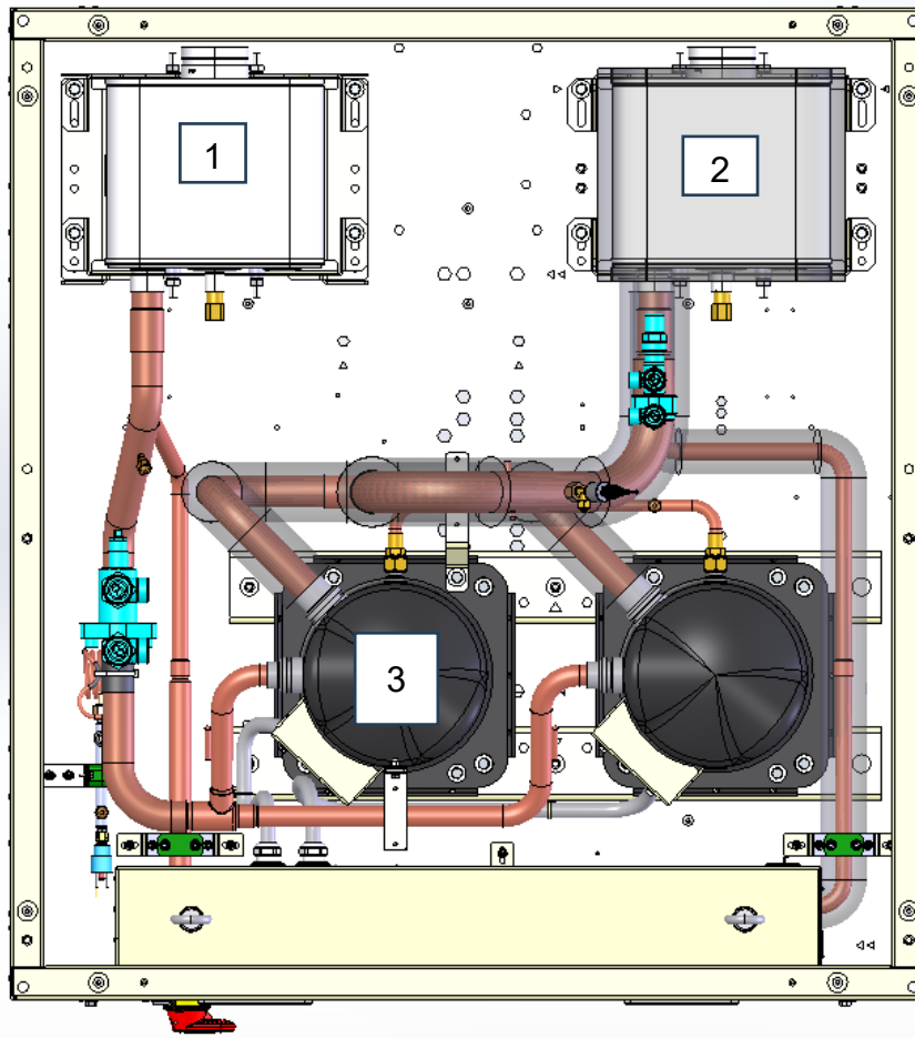
13. ábra - Referenciarajz az elpárolgató és a kondenzátor azonosításához
