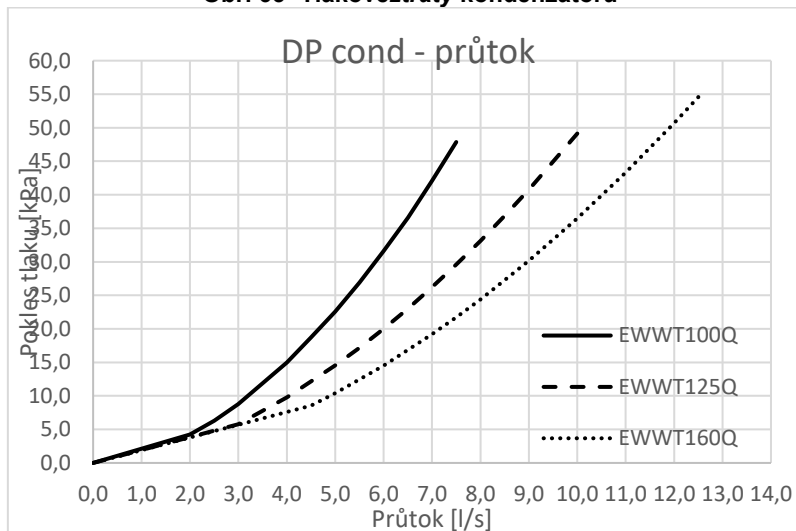
Obr. 65 - Tlakové ztráty kondenzátoru
