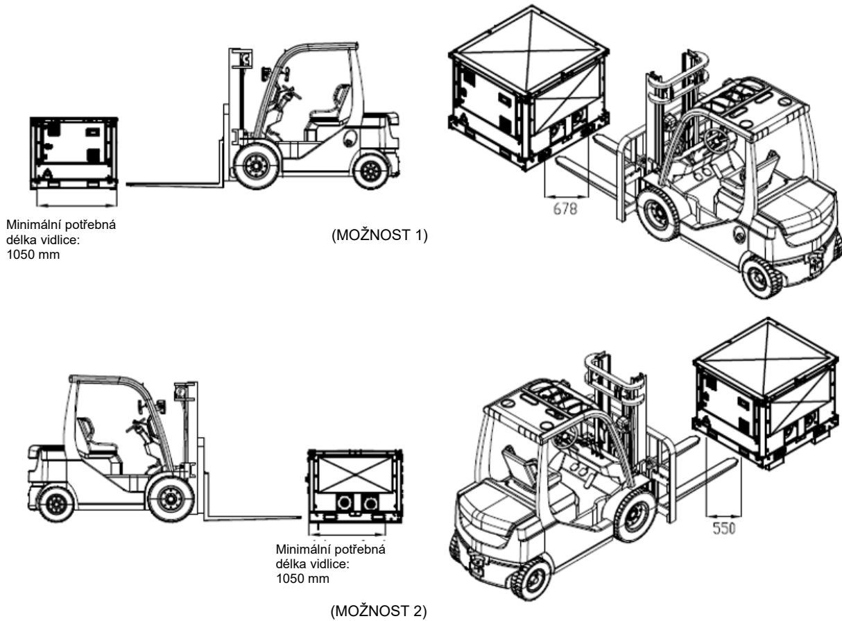
Obr. 49 - Manipulace s modulem čerpadla pomocí vysokozdvizného vozíku
