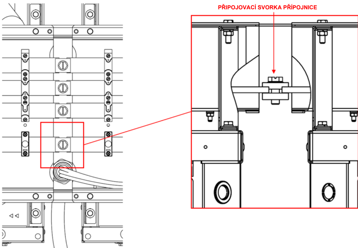
Pohled na otevřený modul napájecího panelu shora
