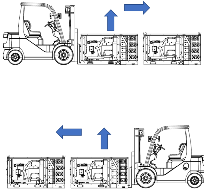
Obr. 49 - Manipulace s modulem čerpadla pomocí vysokozdvizného vozíku
