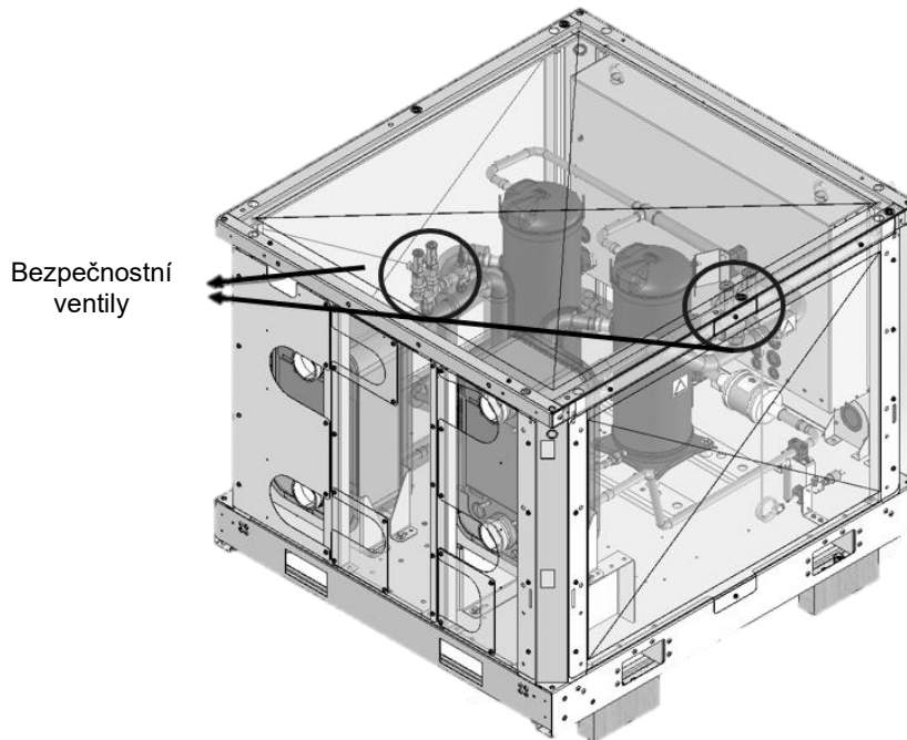
Obr. 12 - Poloha bezpečnostních ventilů jednotky
