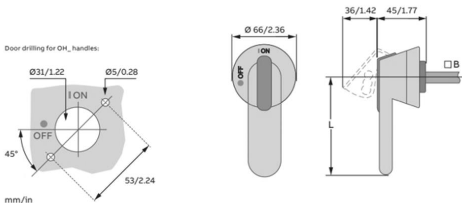
Obr. 23 - Detaily rukojeti pistole
