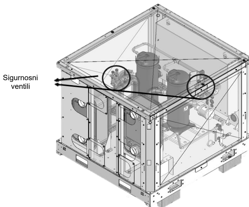
Slika 11 – Položaj sigurnosnih ventila jedinice
