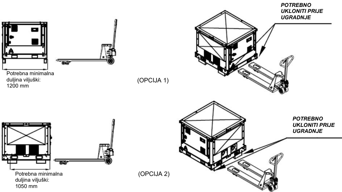
Slika 50 – Rukovanje modulom pumpe pomoću paletnog viličara
