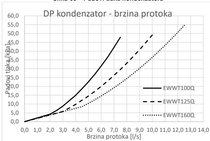
Slika 65 – Padovi tlaka kondenzatora
