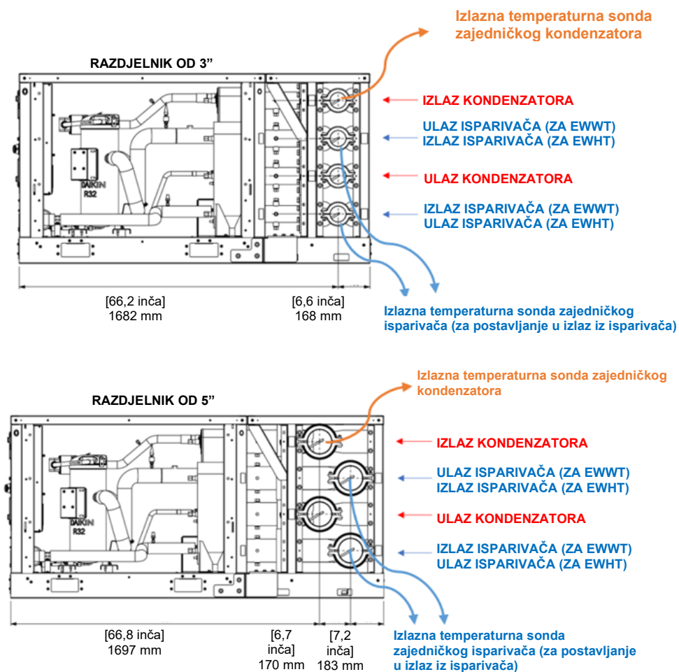
Slika 61 – Položaji temperaturnih sonde za razdjelnik od 3" i 5"
