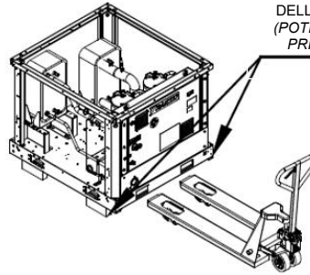
Slika 10 – Alternativni način rukovanja pomoću paletnog viličara
