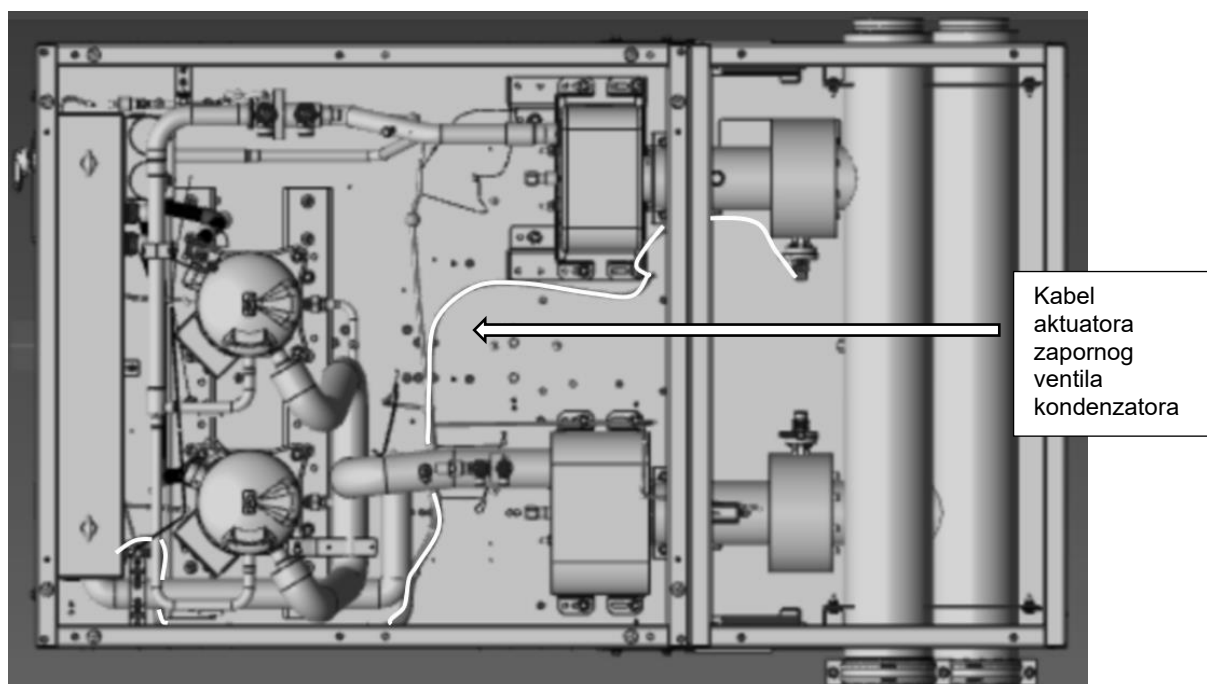
Slika 39 – Trase kabela aktuatora zapornog ventila kondenzatora
