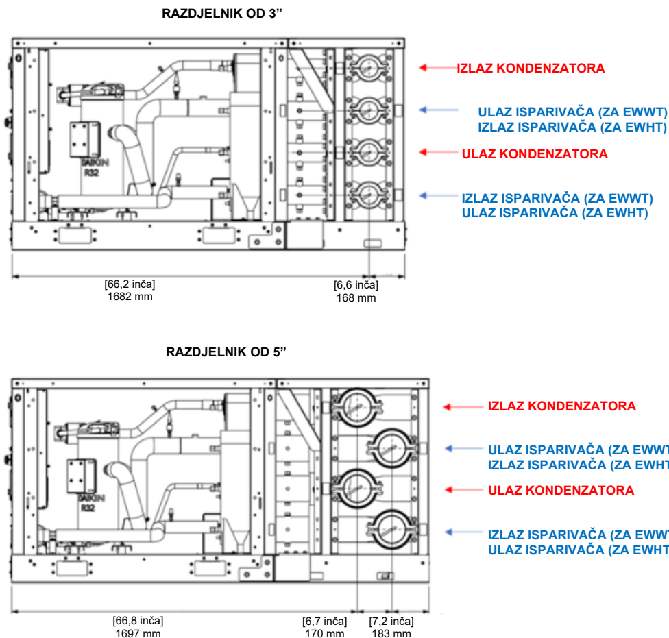
Slika 29 – Veličine razdjelnika za vodu
