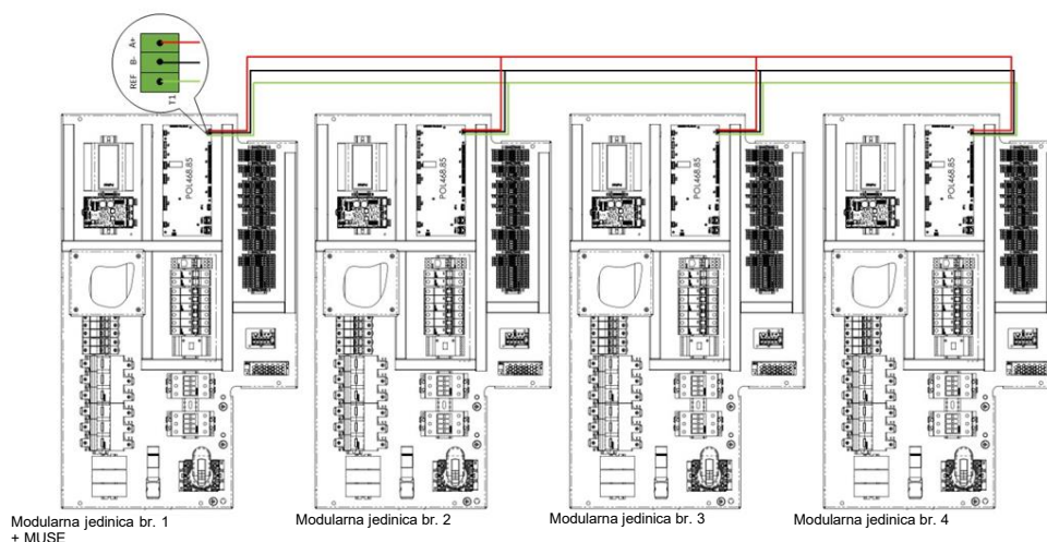
Slika 63 – Spajanje 4 PLC-a na istu Modbus mrežu
