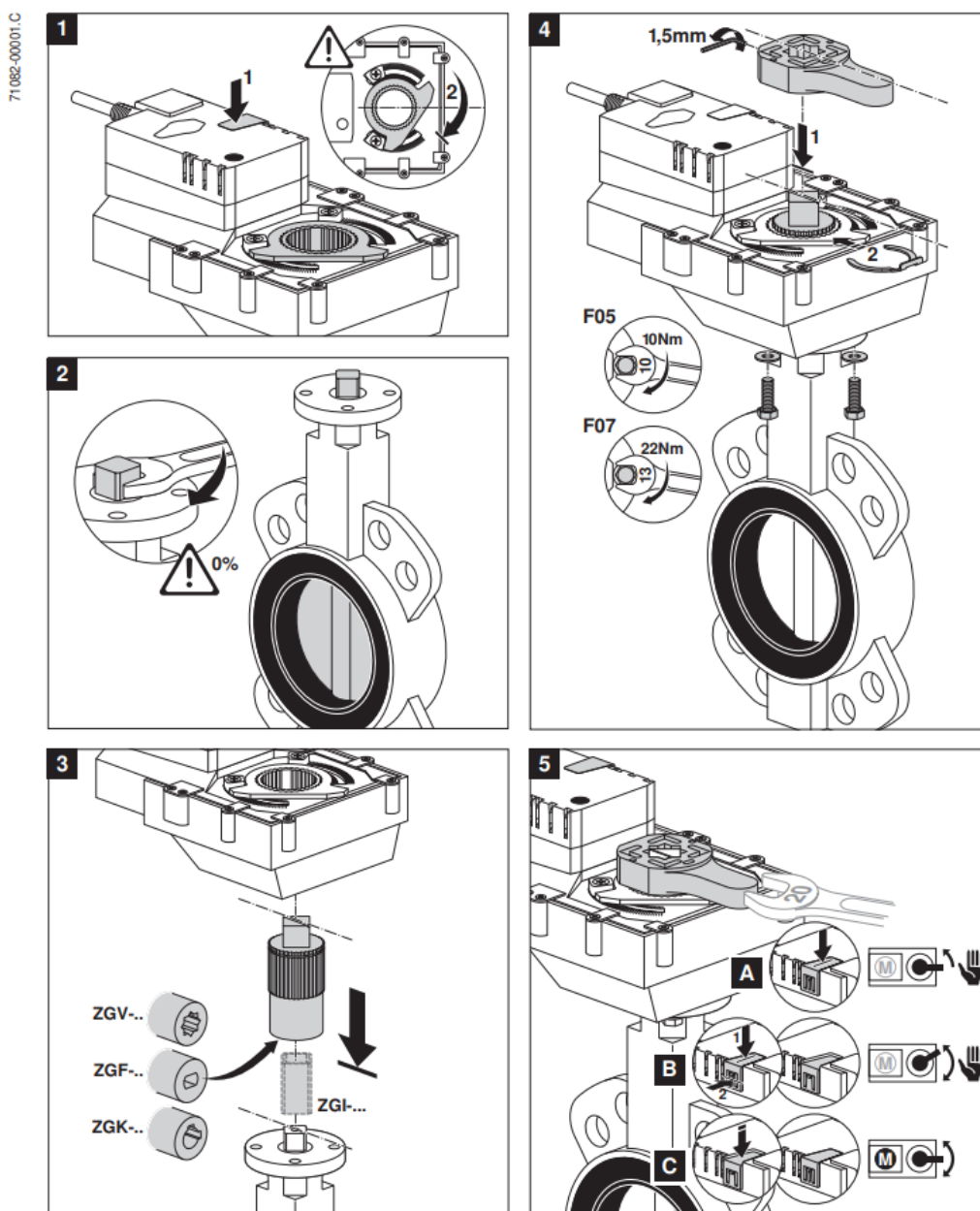
Figur 31– Monteringsinstruktioner för ventilens ställdon
