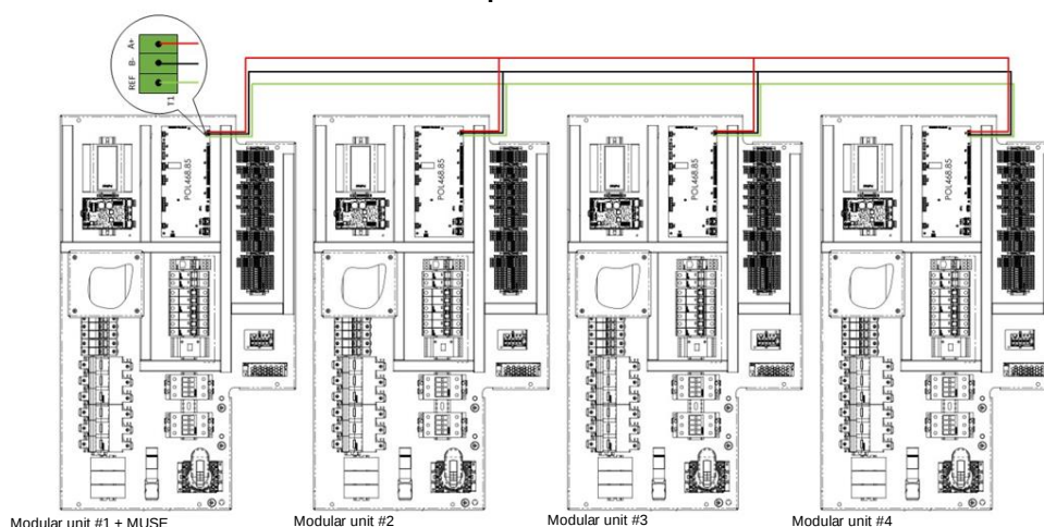
Εικόνα 61 – Σύνδεση 4 PLC στο ίδιο δίκτυο Modbus
