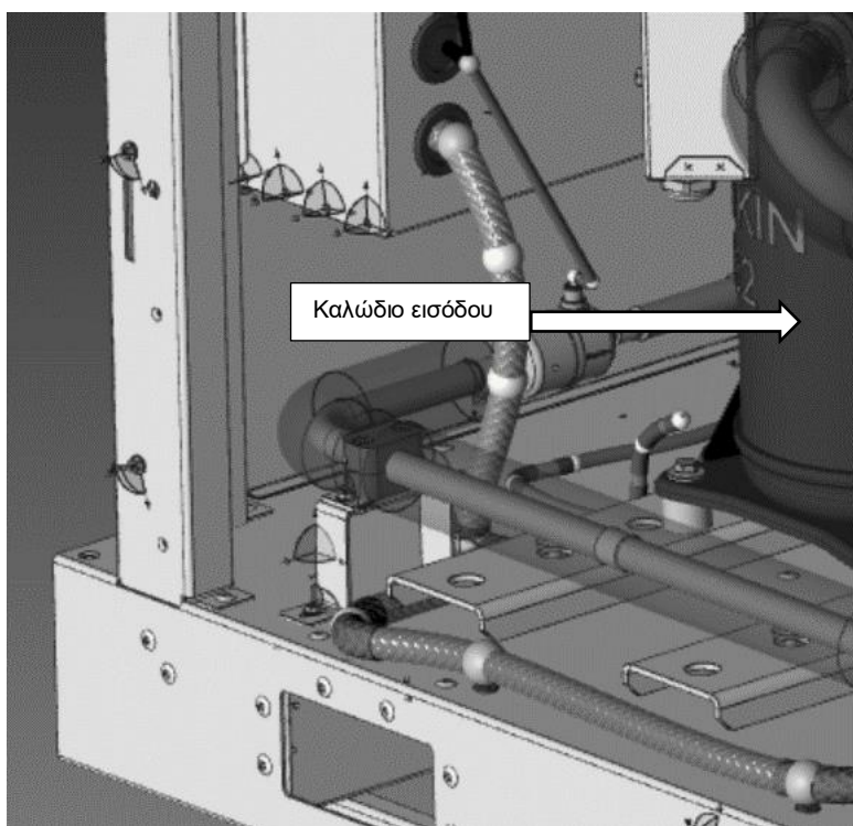
Εικόνα 15 – Σημείο εισόδου ηλεκτρικού πίνακα για καλώδια διακόπτη ροής εξατμιστή και συμπυκνωτή
