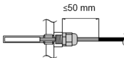
Εικόνα 16 – Αισθητήρας θερμοκρασίας νερού
