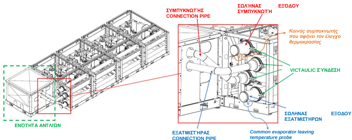
Εικόνα 60 – Λεπτομέρειες τοποθέτησης ανιχνευτών στους σωλήνες
