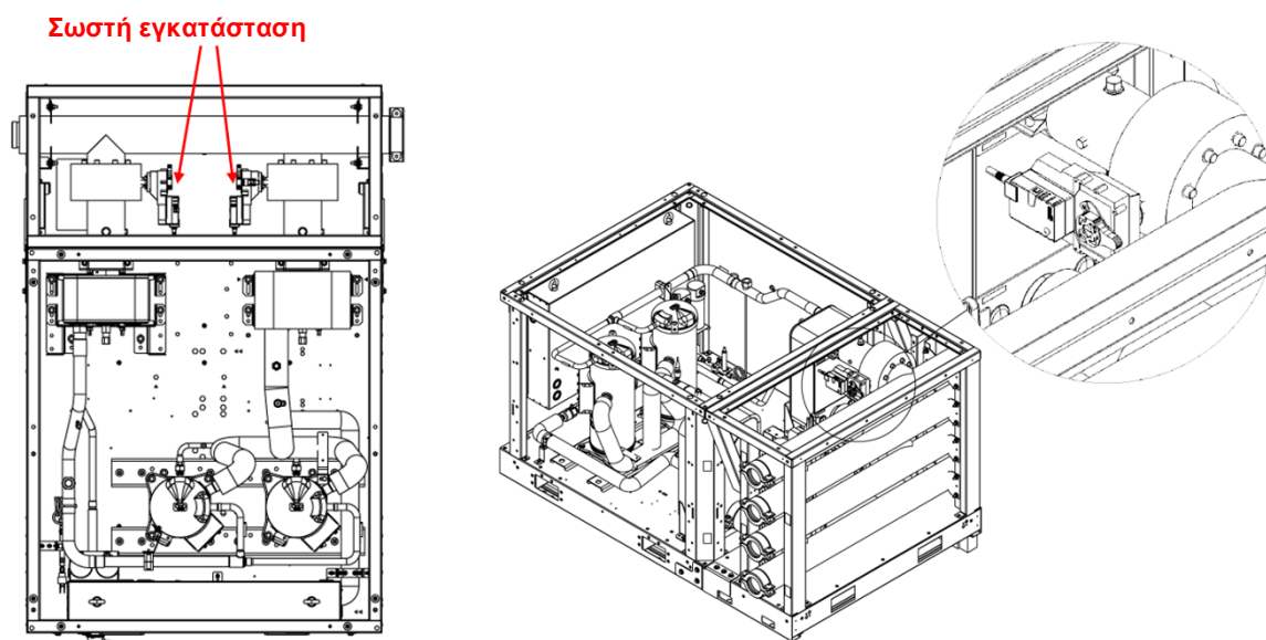
Εικόνα 31 – Ενδείξεις τοποθέτησης ενεργοποιητή βαλβίδας
