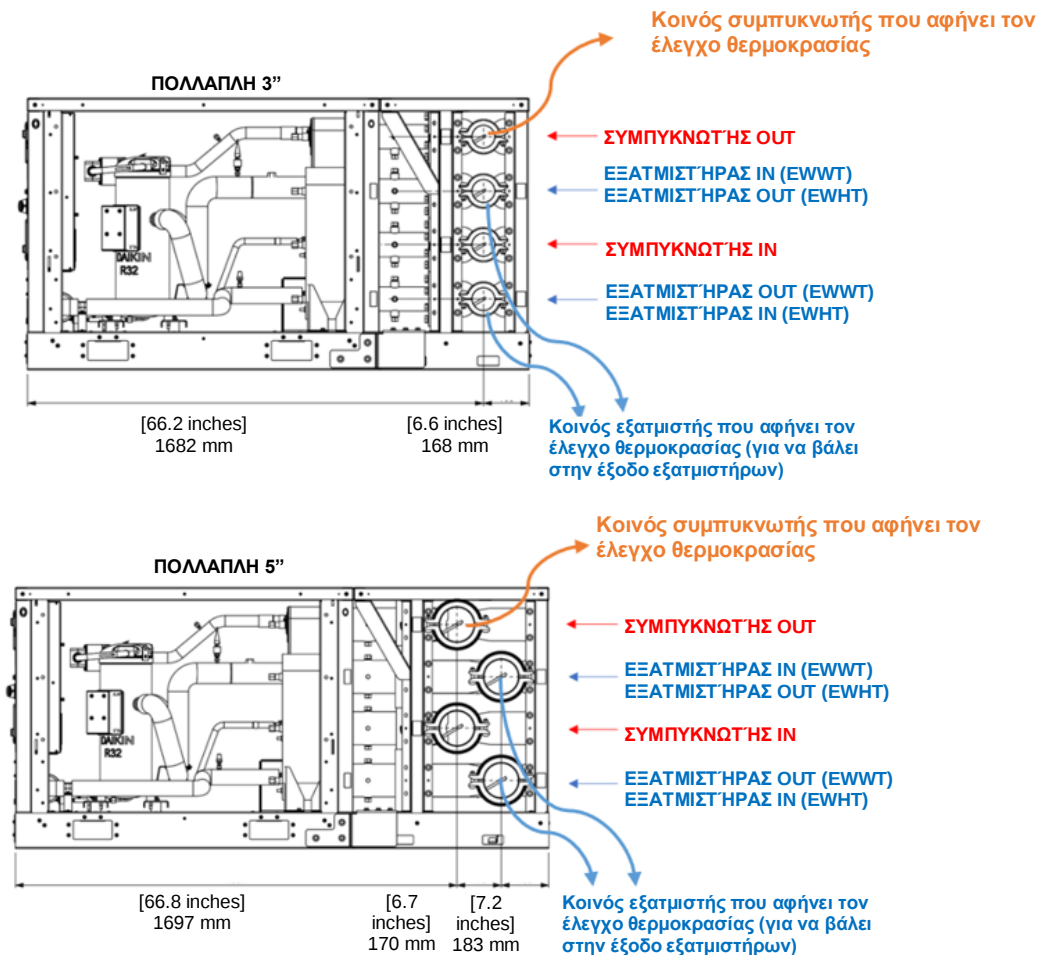
Εικόνα 59 – Θέσεις των αισθητήρων θερμοκρασίας για πολλαπλή μονάδα 3" και 5"
