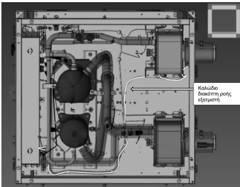
Εικόνα 15 – Σημείο εισόδου ηλεκτρικού πίνακα για καλώδια διακόπτη ροής εξατμιστή και συμπυκνωτή
