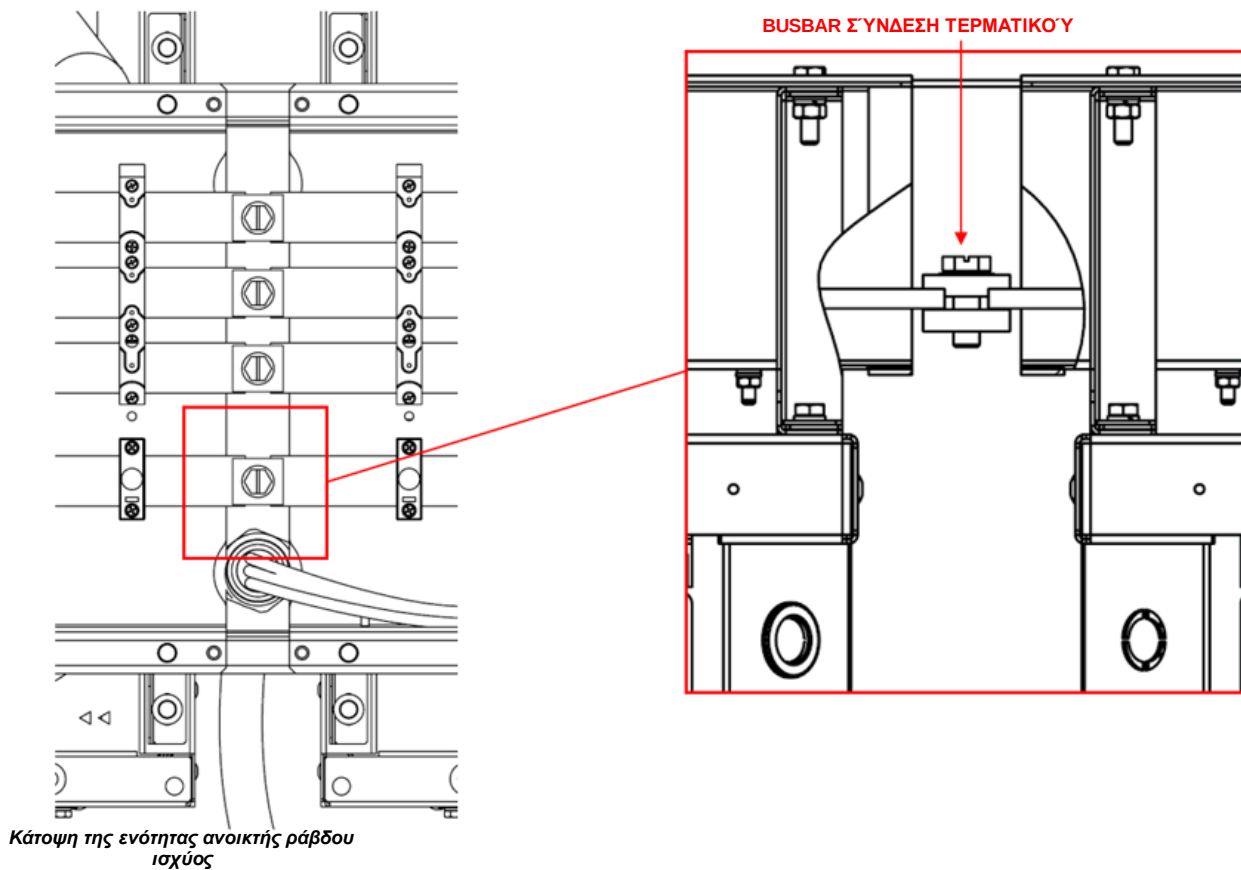
Εικόνα 54 – Λεπτομέρειες σύνδεσης των μονάδων της ράβδου ισχύος μεταξύ τους
