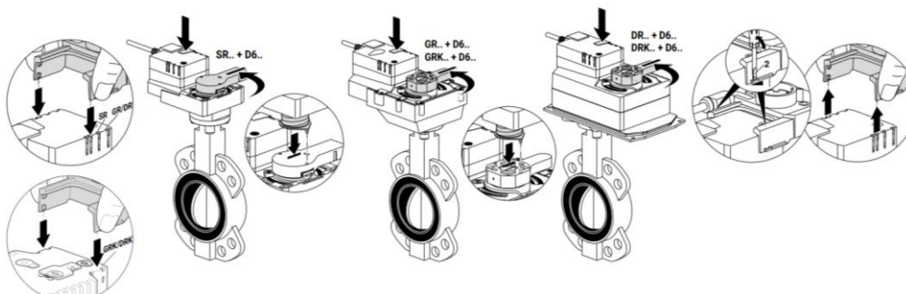
Εικόνα 30 – Οδηγίες τοποθέτησης για διακόπτες ορίου ενεργοποιητή
