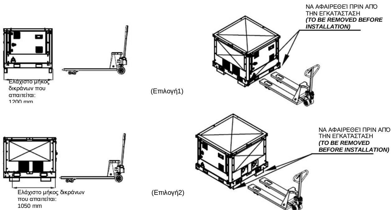
Εικόνα 48 – Χειρισμός μονάδας αντλίας με χρήση για παλετοφόρο
