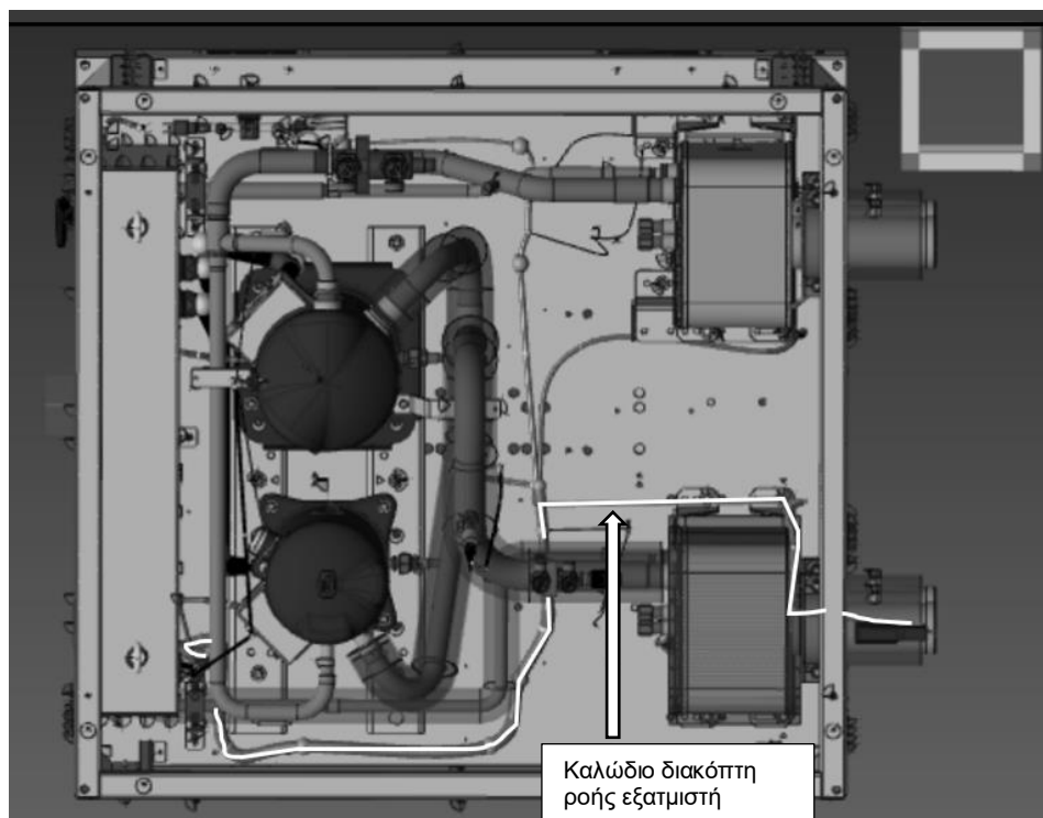
Εικόνα 14 – Δρομολόγηση καλωδίων του διακόπτη ροής εξατμιστή
