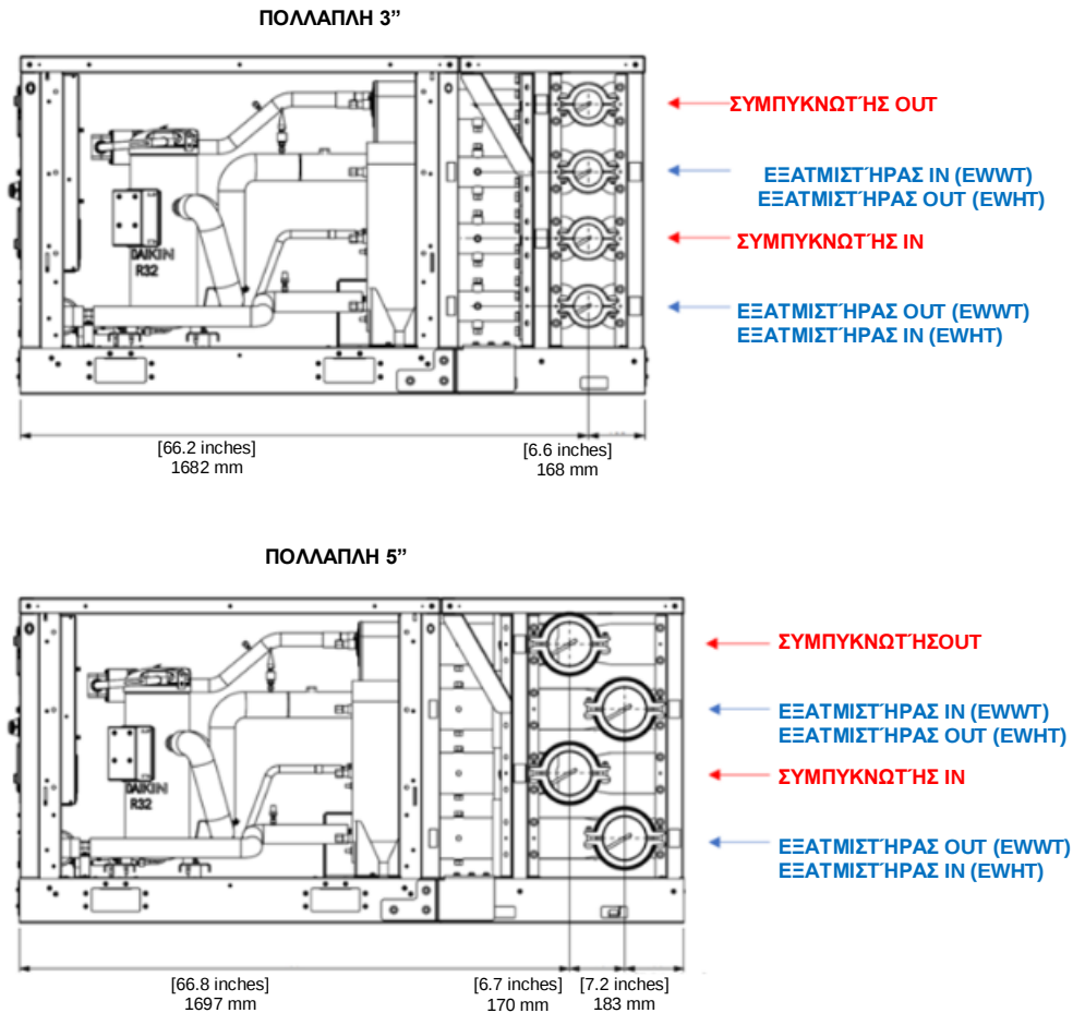
Εικόνα 27 – Μεγέθη πολλαπλής μονάδας νερού
