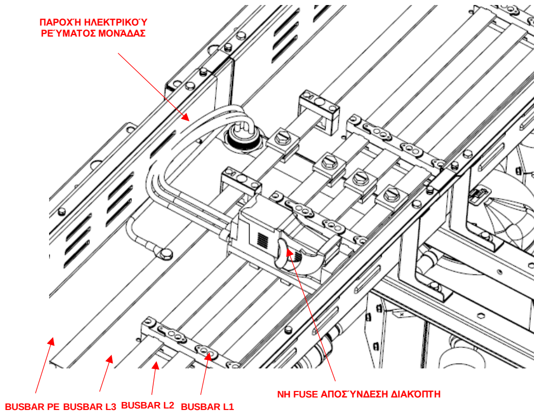
Εικόνα 57 – Λεπτομέρεια ηλεκτρικής σύνδεσης για κάθε άλλη μονάδα
