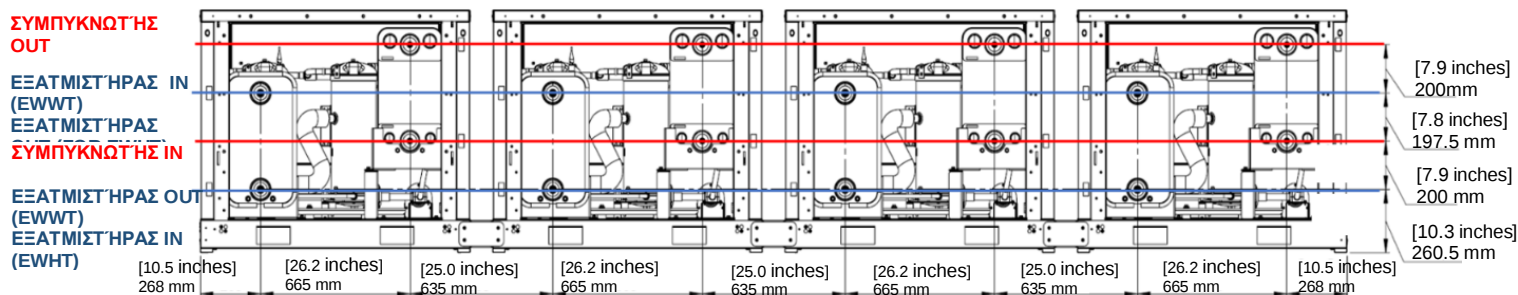
Εικόνα 25 – Διαμόρφωση σωληνώσεων νερού
