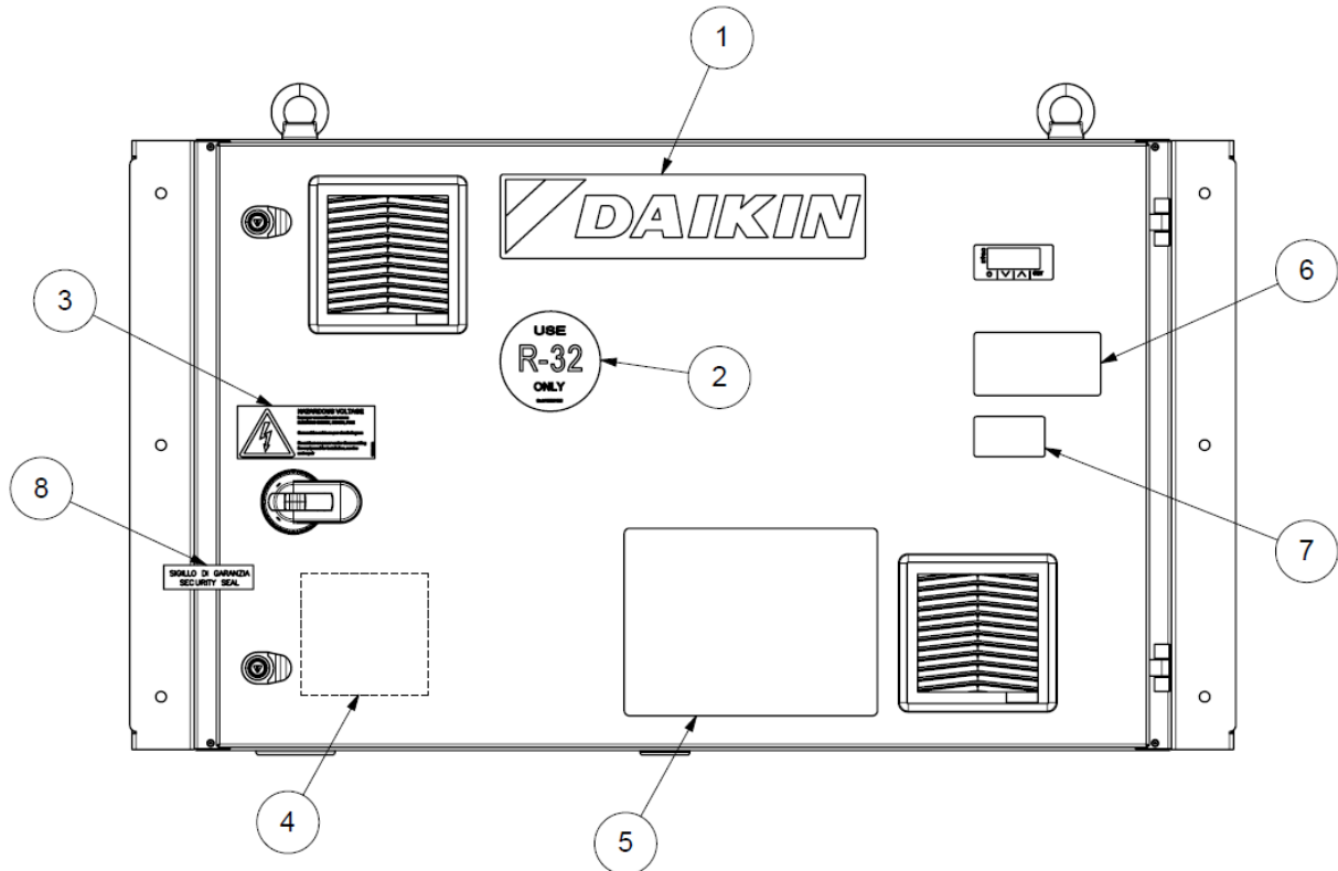
Εικόνα 22 – Περιγραφή των ετικετών που υπάρχουν στον ηλεκτρικό πίνακα (Τυπική*)
