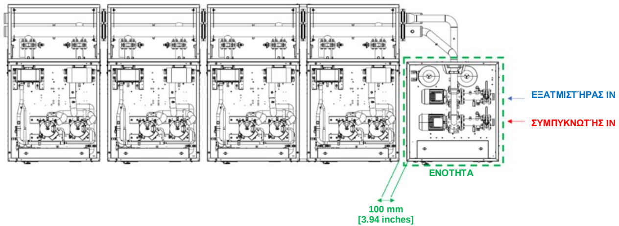
Εικόνα 43 – Εγκατάσταση μονάδας αντλίας – λεπτομέρειες σωληνώσεων
