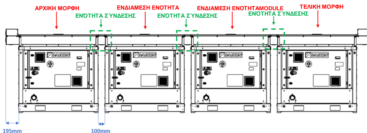
Εικόνα 50 – Δρομολόγηση καλωδίων μεταξύ συστήματος ράβδου και μονάδας
