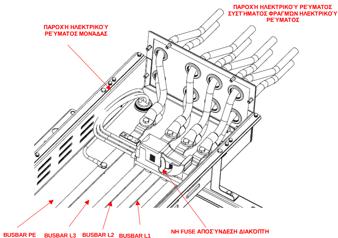
Εικόνα 56 – Λεπτομέρεια ηλεκτρικής σύνδεσης για την αρχική μονάδα
