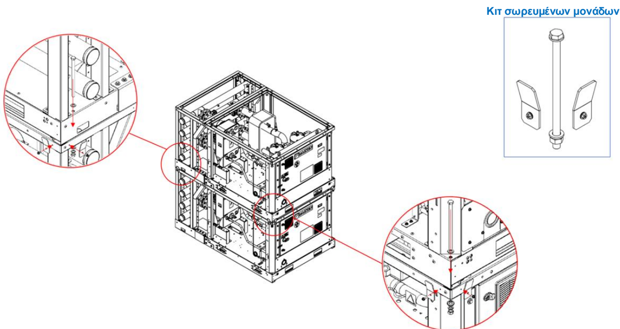
Εικόνα 40 – Οδηγίες τοποθέτησης για στοιβαγμένες μονάδες
