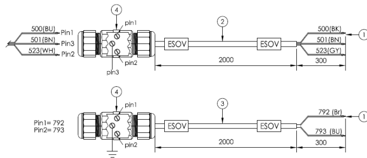
Εικόνα 33 – Προσαρμογείς καλωδίων για ενεργοποιητή βαλβίδας διακοπής λειτουργίας εξατμιστή και διακόπτες ορίου
