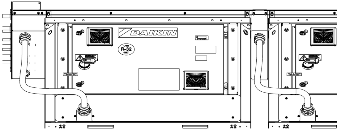
Εικόνα 51 – Λεπτομέρειες δρομολόγησης καλωδίων
