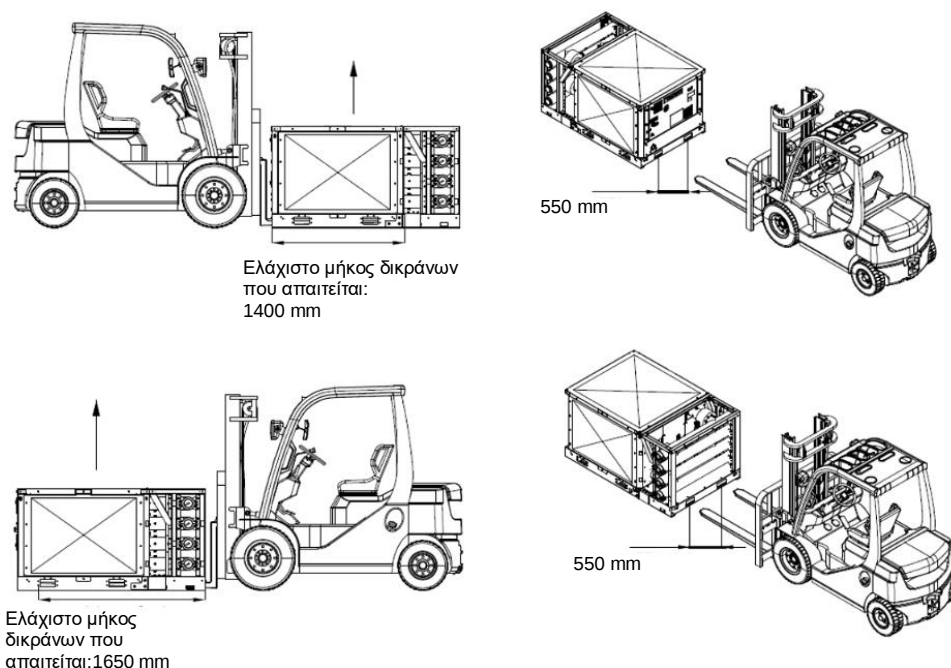
Εικόνα 45 – Χειρισμός μονάδας και πολλαπλών μονάδων
