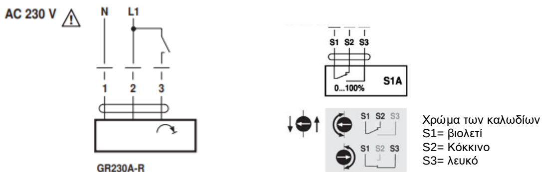
Εικόνα 32 – Διάγραμμα καλωδίωσης για κινητήρα (αριστερό σχήμα) και διακόπτες ορίου (δεξιό σχήμα)
