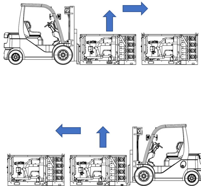
Εικόνα 46 – Ενδείξεις για εγκατάσταση στοιβαγμένων μονάδων
