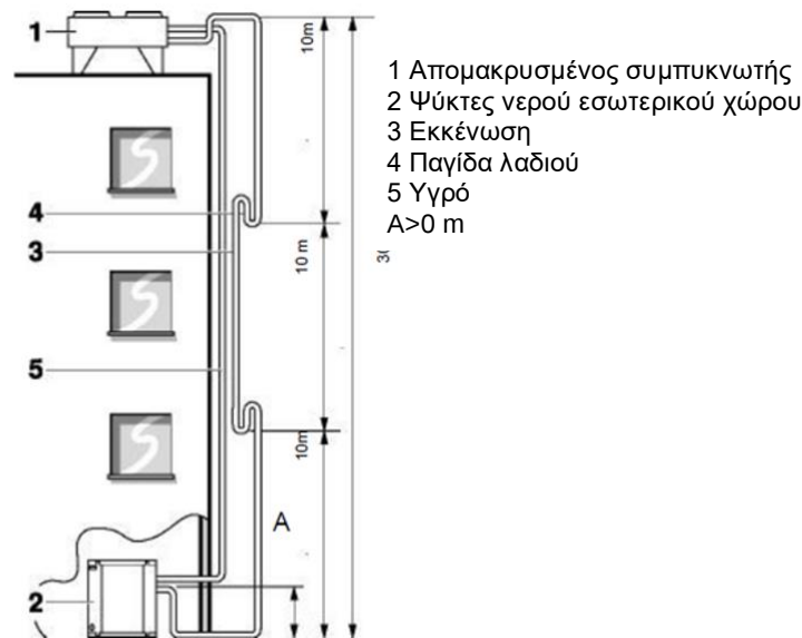
Εικόνα 17 – Σύνδεση του κυκλώματος ψυκτικού (1)
