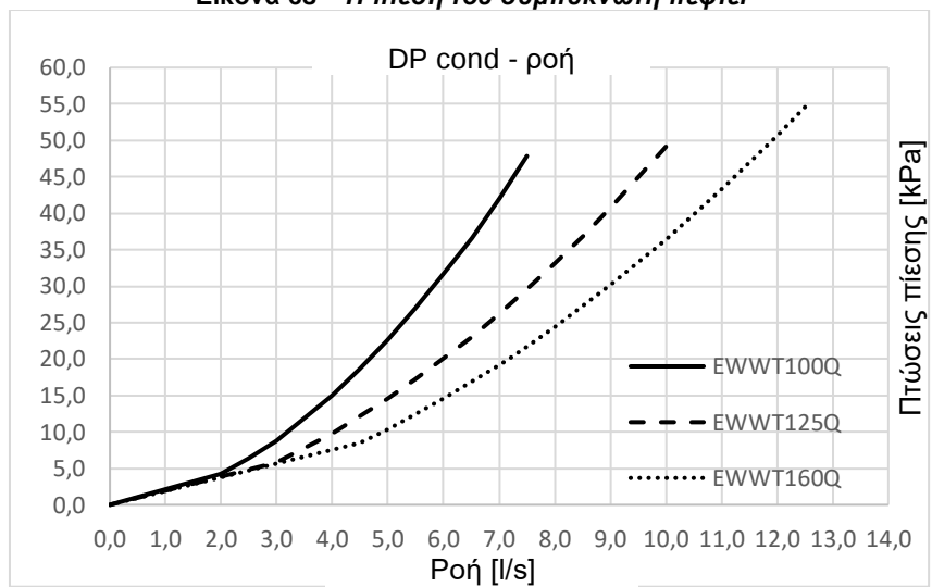
Εικόνα 63 – Η πίεση του συμπυκνωτή πέφτει
