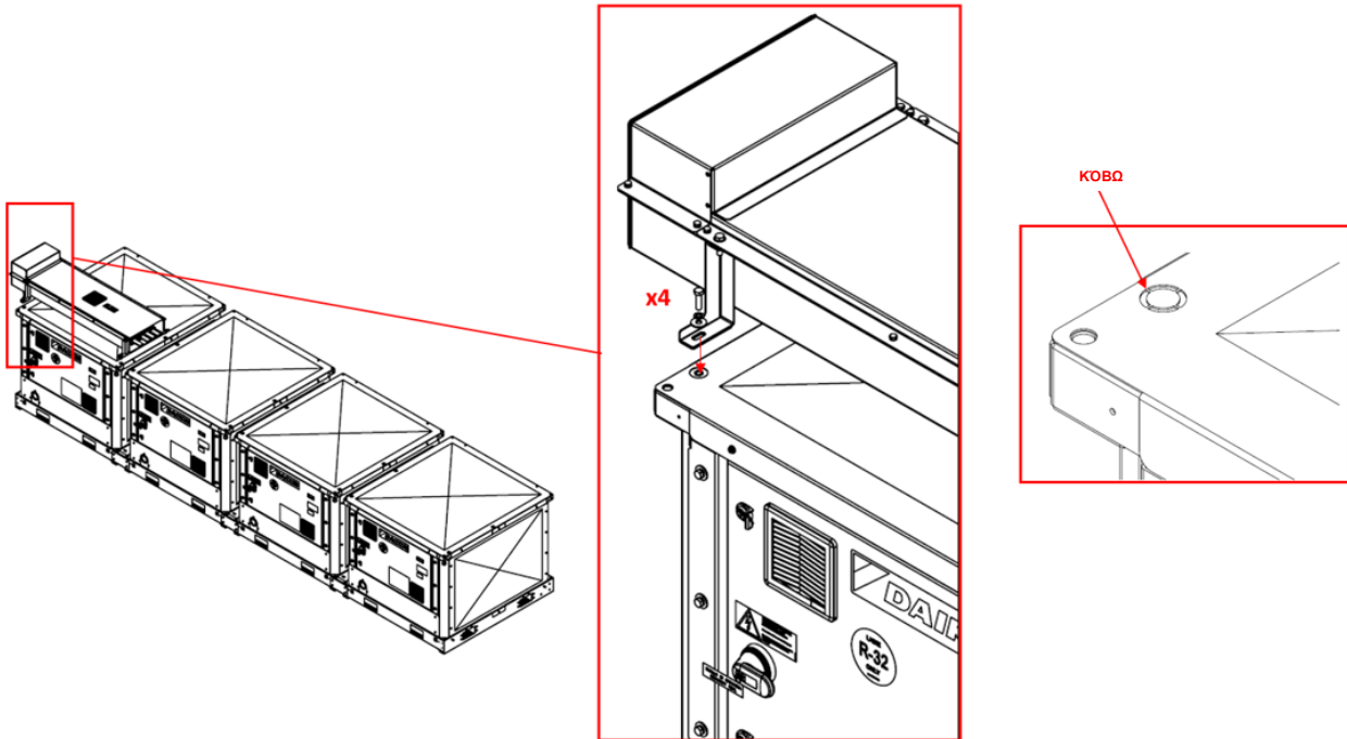
Εικόνα 52 – Στερέωση του συστήματος ράβδου ισχύος στη μονάδα
