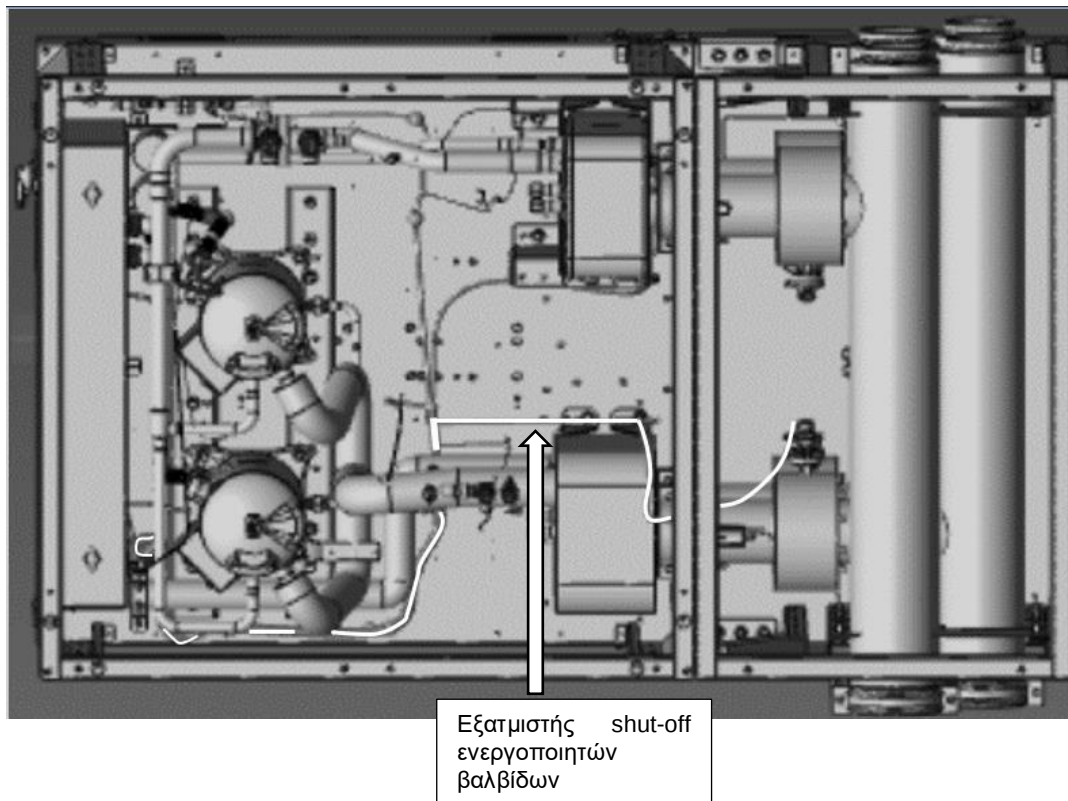
Εικόνα 37 – Δρομολόγηση καλωδίου ενεργοποιητή βαλβίδας διακοπής λειτουργίας συμπυκνωτή
