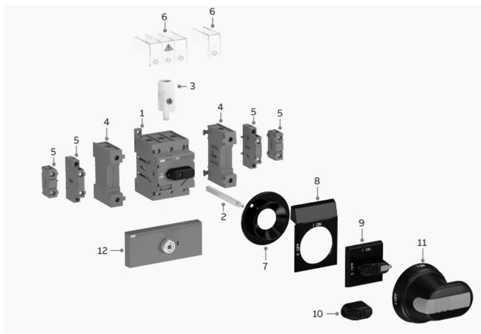
Εικόνα 20 – Οδηγίες συναρμολόγησης λαβής
