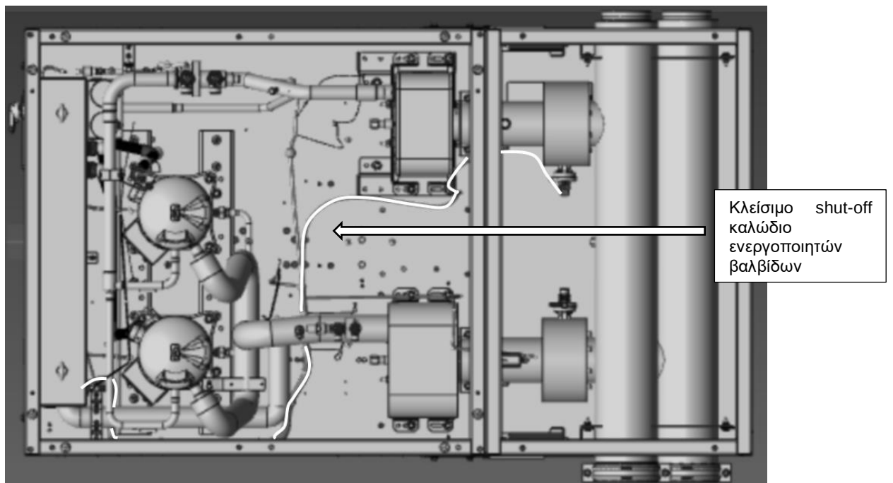
Εικόνα 37 – Δρομολόγηση καλωδίου ενεργοποιητή βαλβίδας διακοπής λειτουργίας συμπυκνωτή
