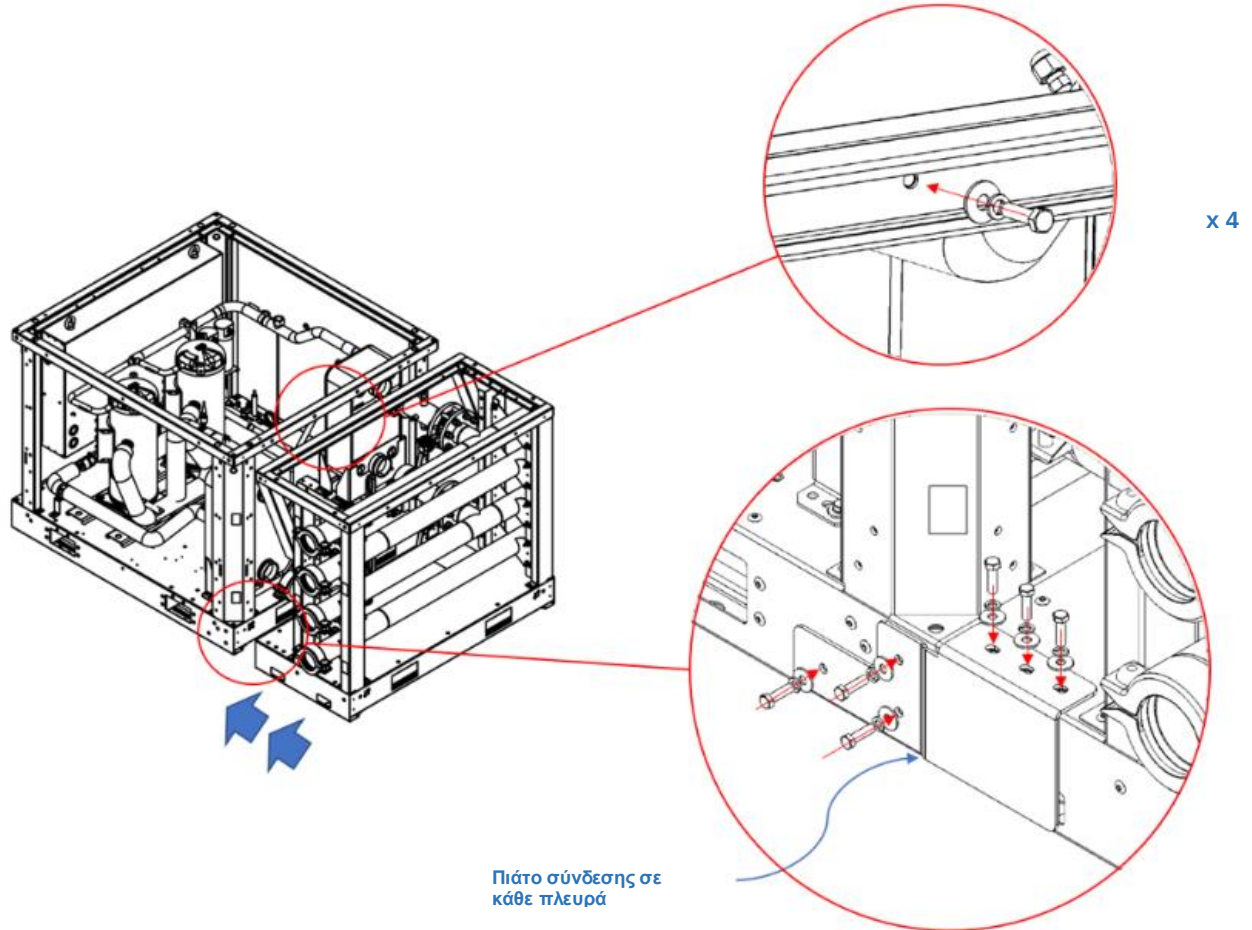
Εικόνα 23 – Οδηγίες σύνδεσης μεταξύ ψύκτη και πολλαπλών μονάδων
