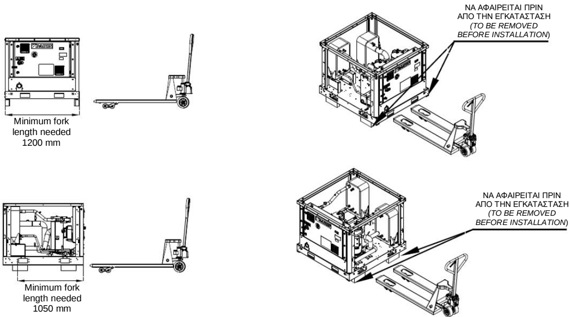
Εικόνα 10 – Εναλλακτική μέθοδος χειρισμού με παλετοφόρο
