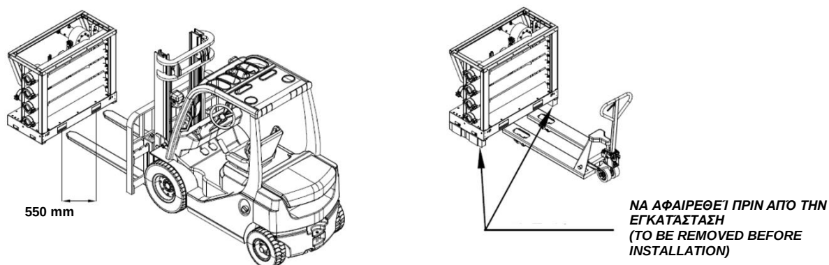
Εικόνα 44 – Χειρισμός πολλαπλής μονάδας
