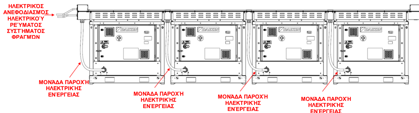
Εικόνα 50 – Δρομολόγηση καλωδίων μεταξύ συστήματος ράβδου και μονάδας
