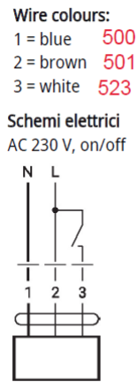
Εικόνα 35 – Διάγραμμα καλωδίωσης ενεργοποιητή βαλβίδας διακοπής λειτουργίας
