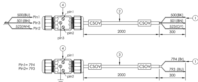
Εικόνα 34 – Προσαρμογείς καλωδίων για ενεργοποιητή βαλβίδας διακοπής λειτουργίας συμπτυκνωτή και διακόπτες ορίου
