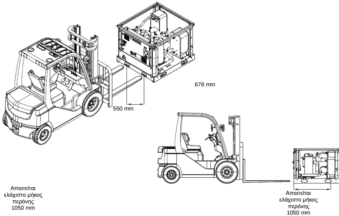
Εικόνα 9 – Εναλλακτική μέθοδος χειρισμού με περνοφόρο ανυψωτικό
