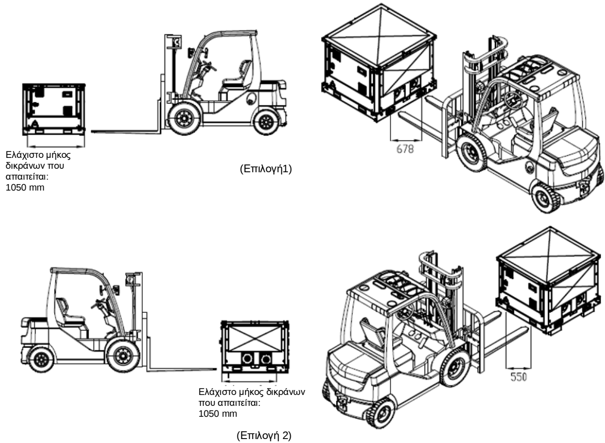
Εικόνα 47 – Χειρισμός μονάδας αντλίας με χρήση περονοφόρου
