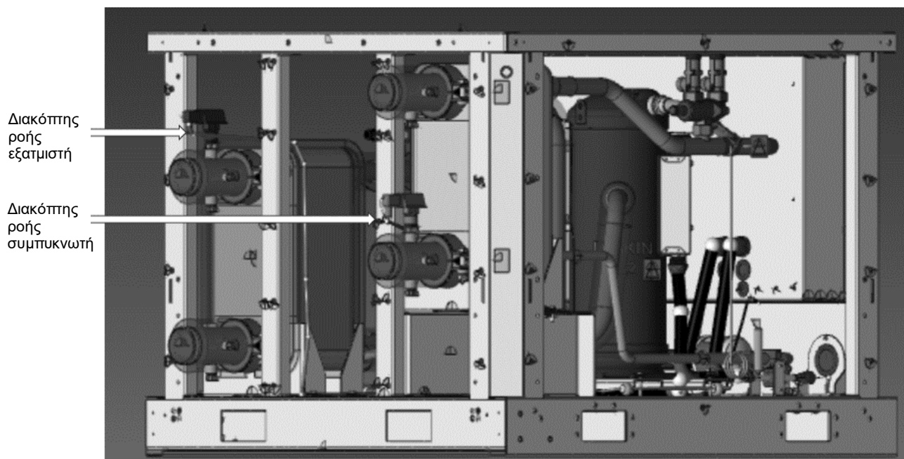
Εικόνα 13 – Δρομολόγηση καλωδίων του διακόπτη ροής εξατμιστή
