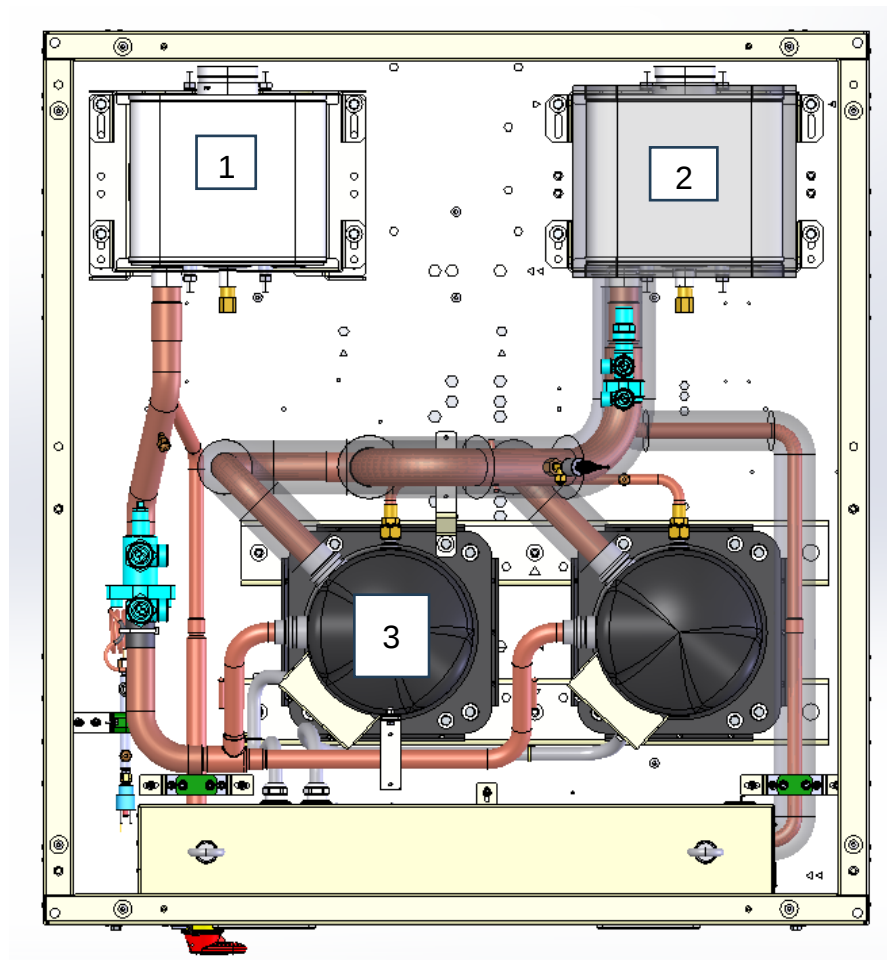
Εικόνα 11 – Σχέδιο αναφοράς για αναγνώριση εξατμιστή και συμπυκνωτή
