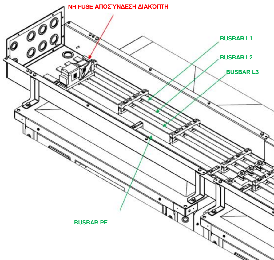
Εικόνα 55 – Λεπτομέρεια των ασφαλειών και του κουτιού για τη δρομολόγηση των καλωδίων της μονάδας της ράβδου ισχύος
