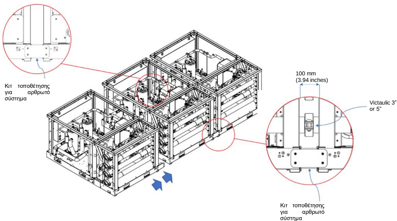
Εικόνα 26 – Σύνδεση αρθρωτών συστημάτων
