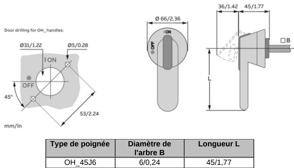
Fig. 23 - Détails de la poignée du pistolet
