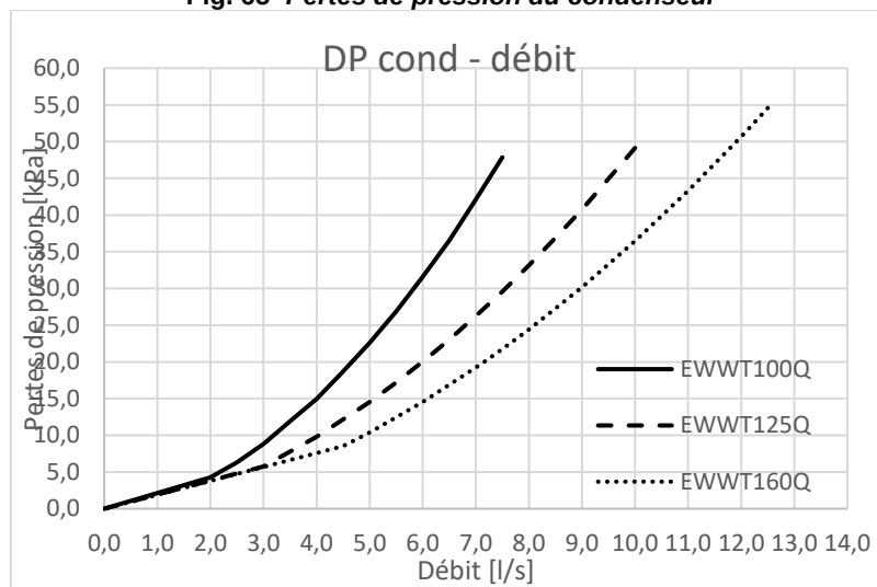
Fig. 65 - Pertes de pression du condenseur
