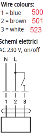
Fig. 37 - Schéma de câblage de l'actionneur de la vanne d'arrêt
