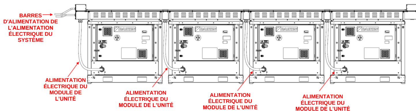
Fig. 52 - Acheminement des câbles entre le système de barres et l'unité
