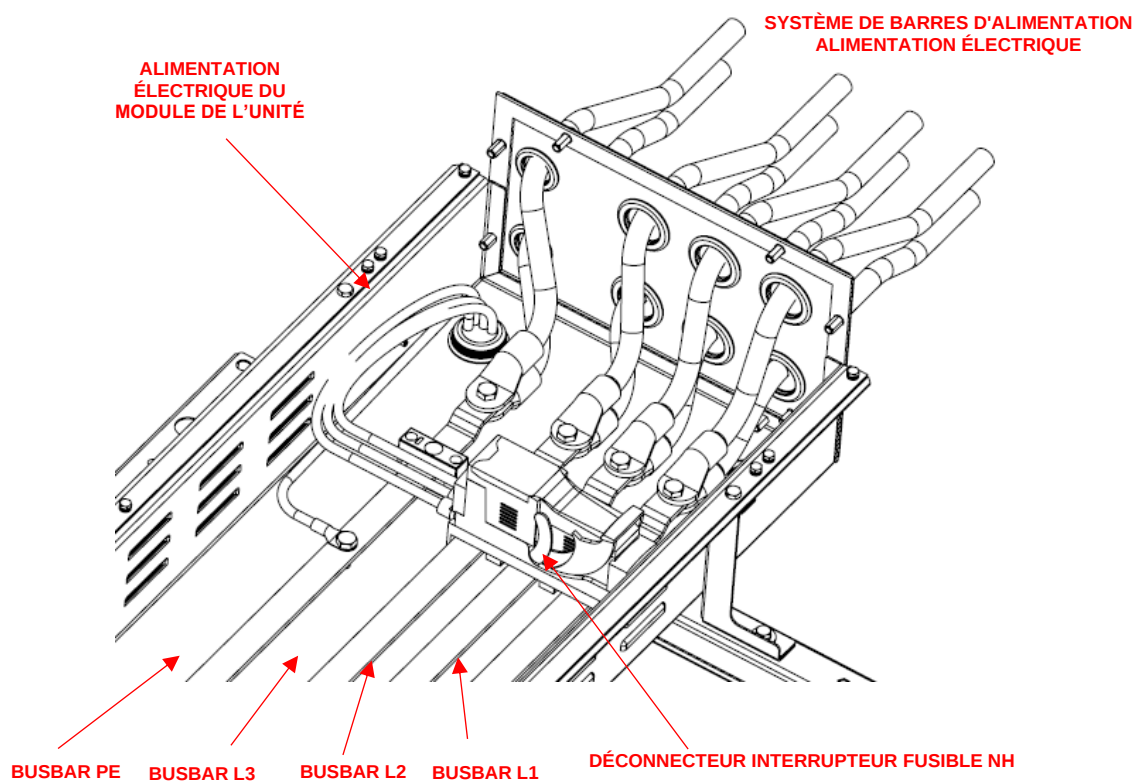
Fig. 58 - Détail de la connexion électrique pour le module de l'unité initiale
