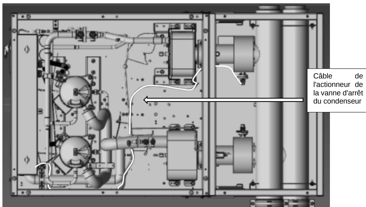
Fig. 39 - Acheminement du câble de l'actionneur de la vanne d'arrêt du condenseur
