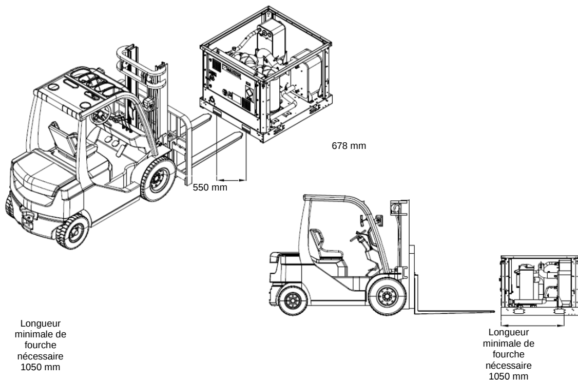
Fig. 9 - Autre méthode de manutention avec chariot élévateur
