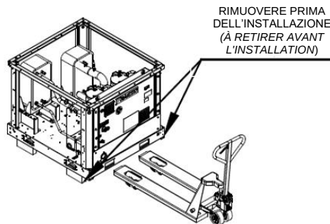
Fig. 10 - Autre méthode de manutention avec un transpalette
