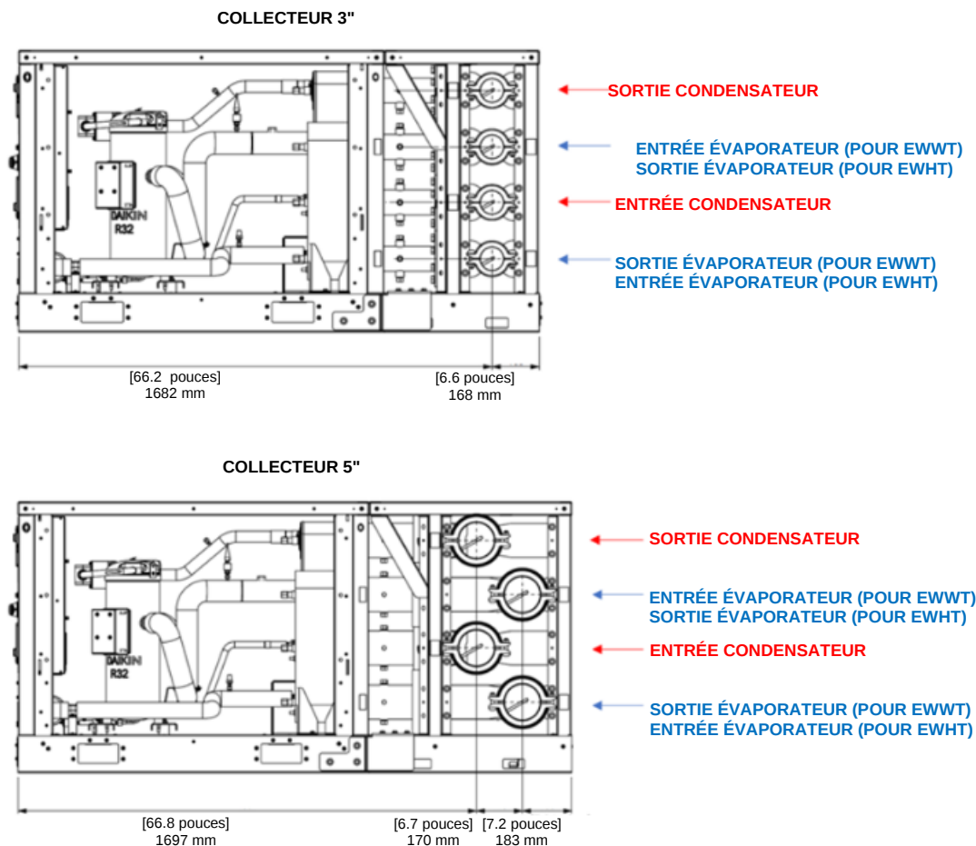
Fig. 29 - Dimensions des collecteurs d'eau
