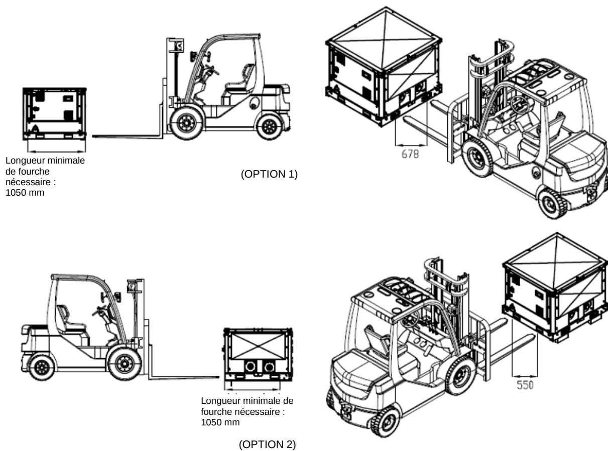
Fig. 49 - Manutention du module de pompe à l'aide d'un chariot élévateur
