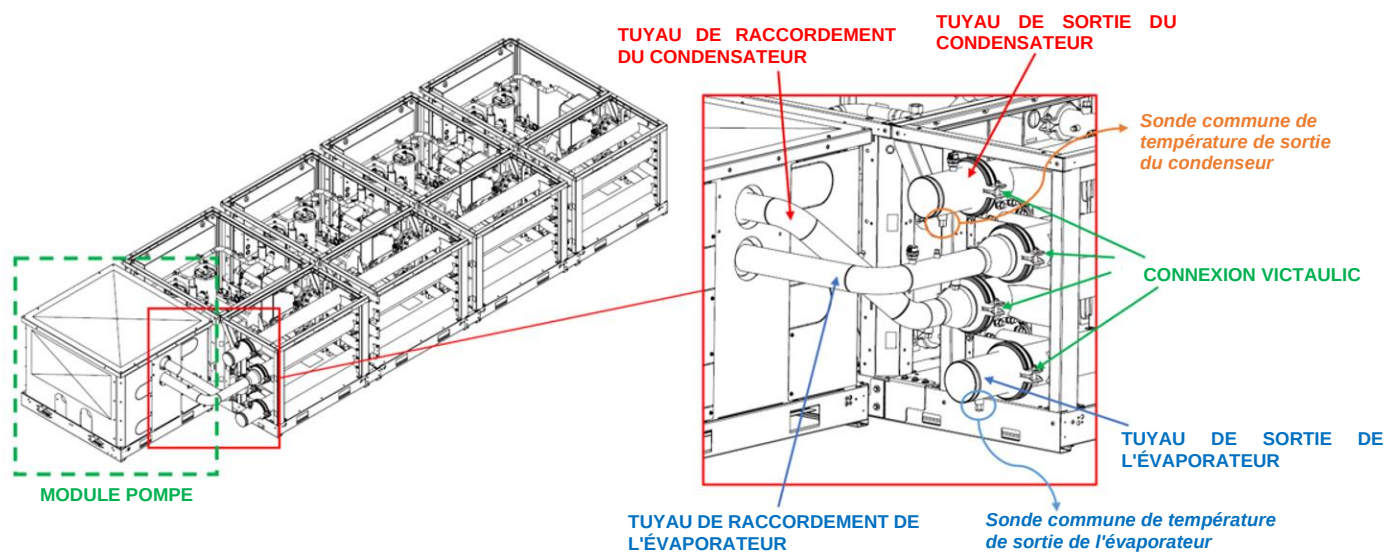
Fig. 62 - Détails du positionnement des sondes sur les tuyaux
