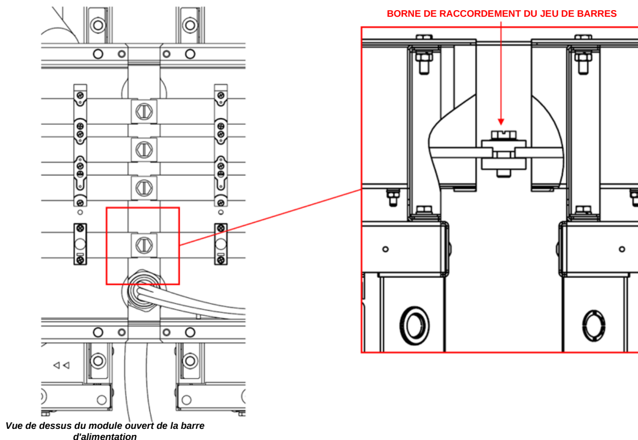
Fig. 56 - Détails de la connexion des modules de la barre d'alimentation
