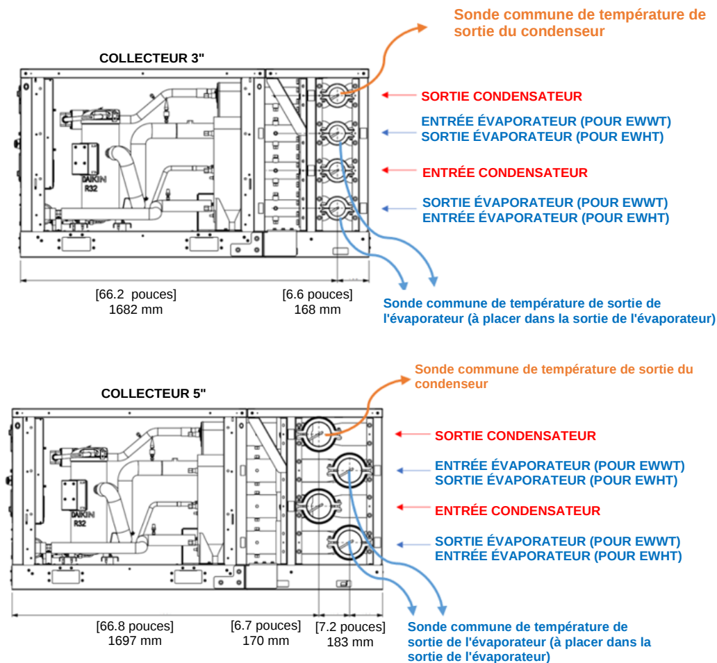
Fig. 61 - Positions des sondes de température pour les collecteurs 3" et 5"
