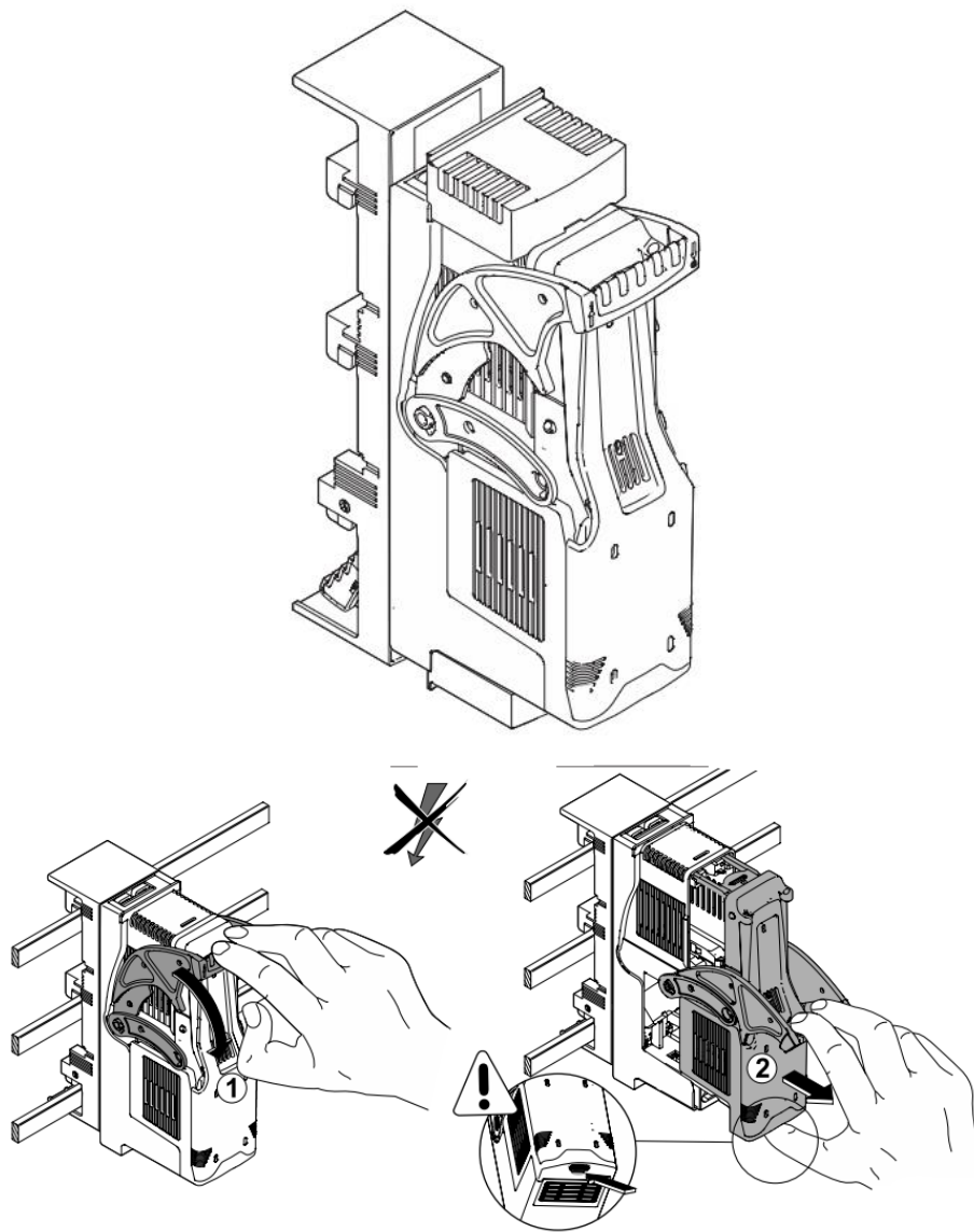
Fig. 60 - Interrupteur-sectionneur à fusible NH
