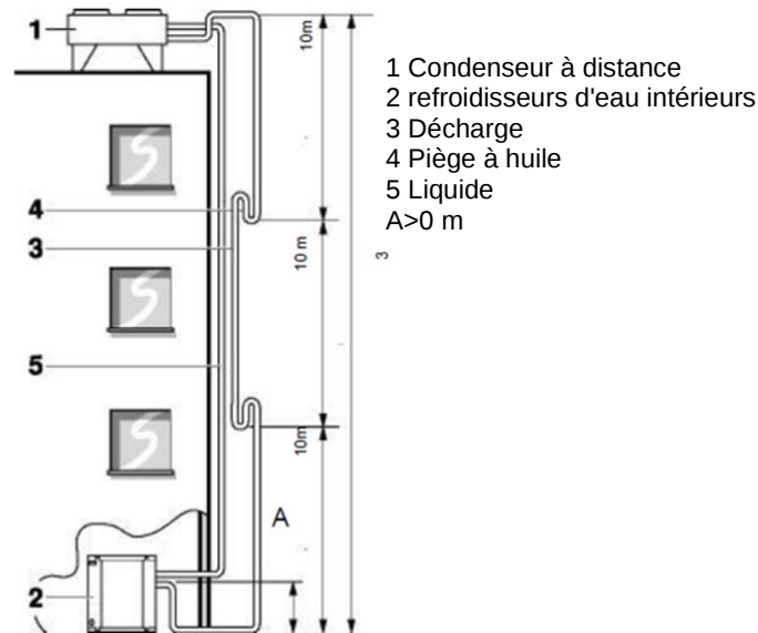
Fig. 19 - Raccordement du circuit du réfrigérant (1)
