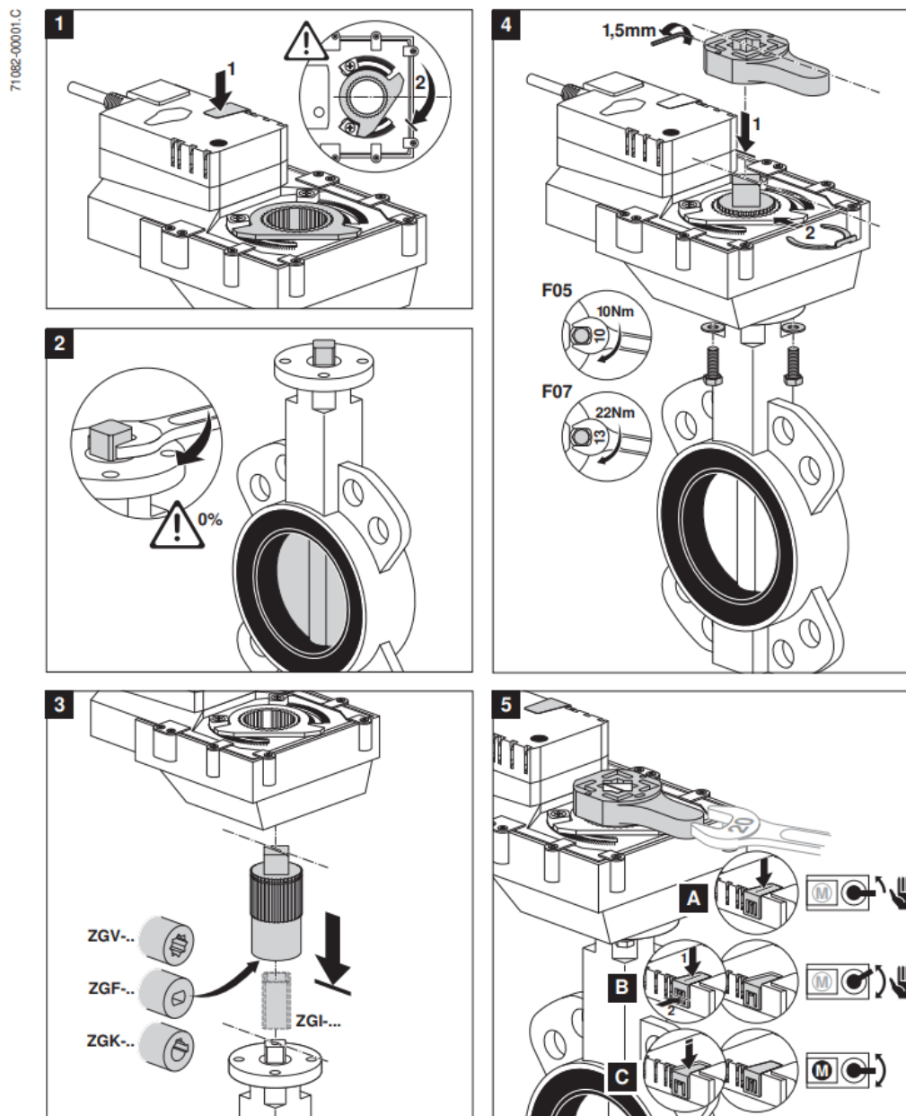
Fig. 31 - Instructions de montage pour l'actionneur de vanne
