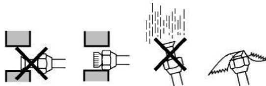
Fig. 20 - Raccordement du circuit de réfrigérant (4)
