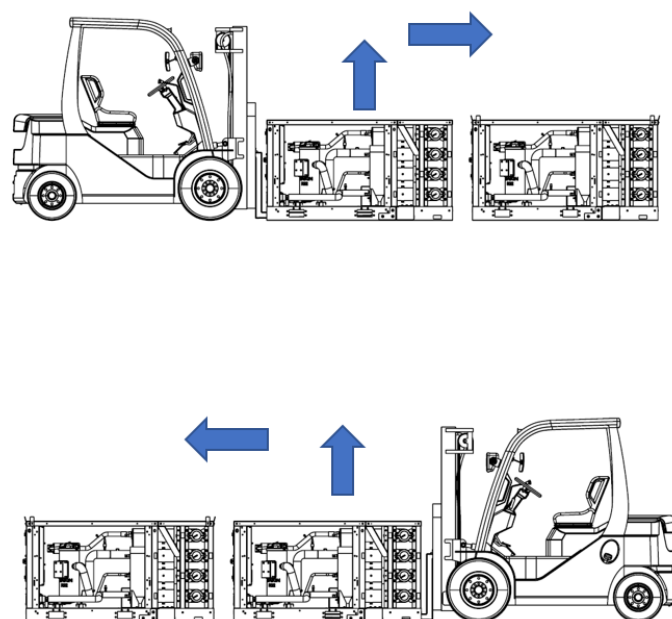
Fig. 49 - Manutention du module de pompe à l'aide d'un chariot élévateur
