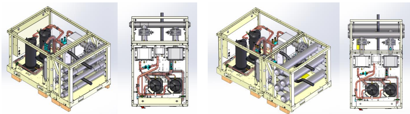
Obr. 26 – Trubky PHR s rozdělovacím modulem (vlevo pro 3palcové - vpravo pro 5palcové rozdělovací trubky)
