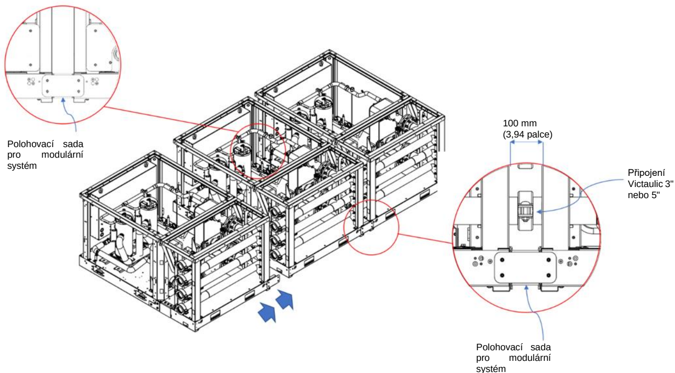
Obr. 28 - Připojení modulárních systémů
