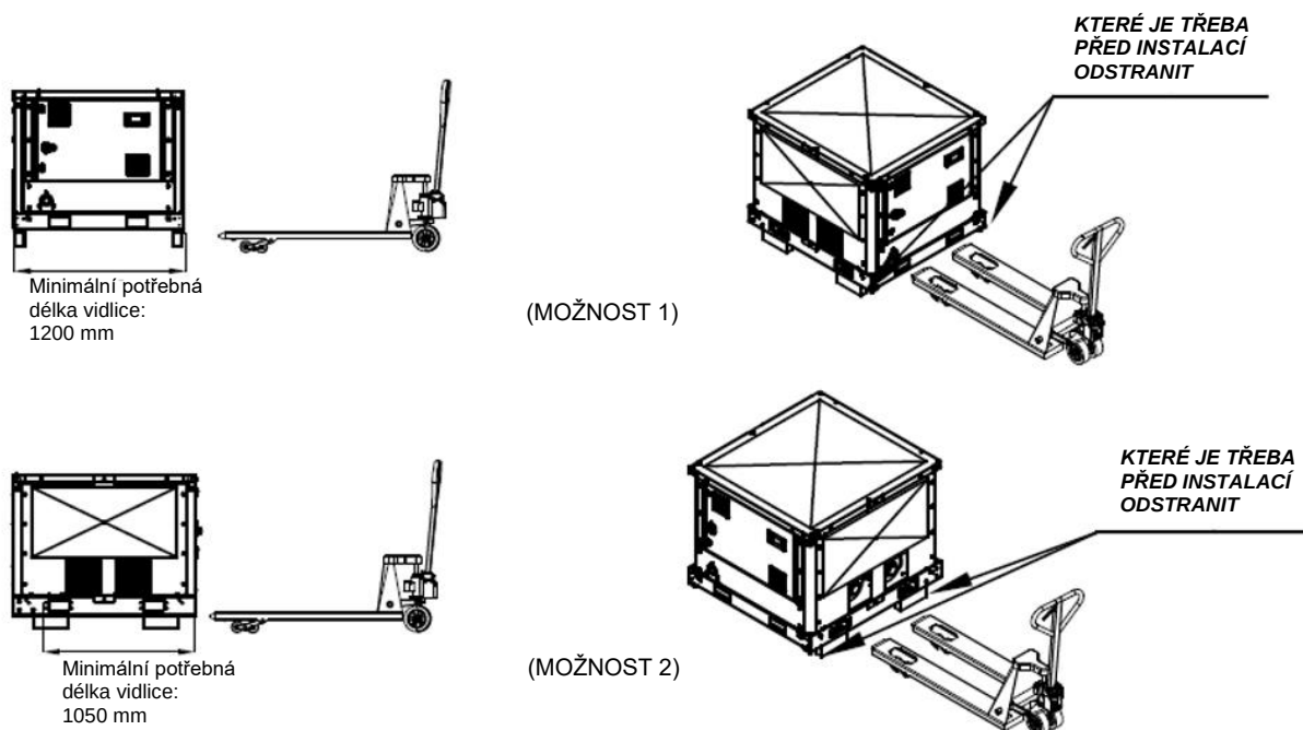
Obr. 50 - Manipulace s modulem čerpadla pomocí paletového vozíku
