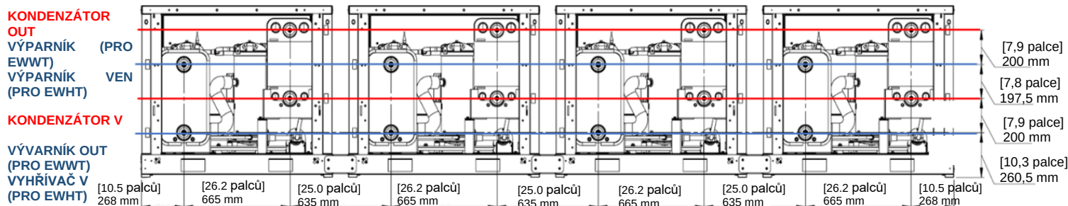
Obr. 27 - Konfigurace vodovodního potrubí
