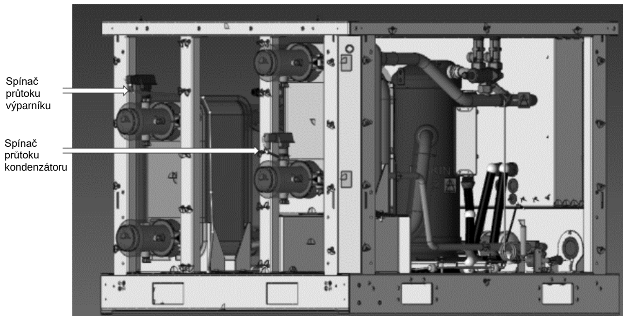
Obr. 15 - Vedení kabelů spínače průtoku výparníku
