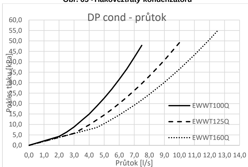
Obr. 65 - Tlakové ztráty kondenzátoru
