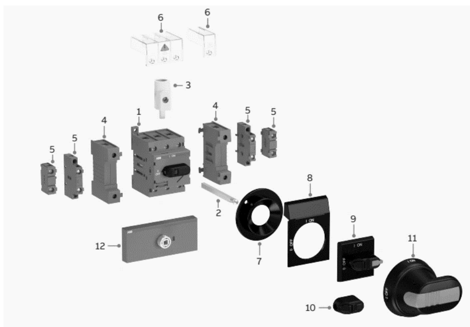
Obr. 22 - Návod k montáži rukojeti
