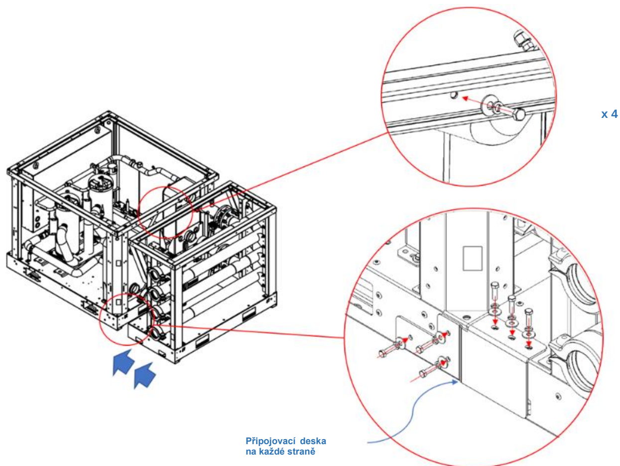
Obr. 25 - Pokyny pro připojení chladicích a rozdělovacích modulů
