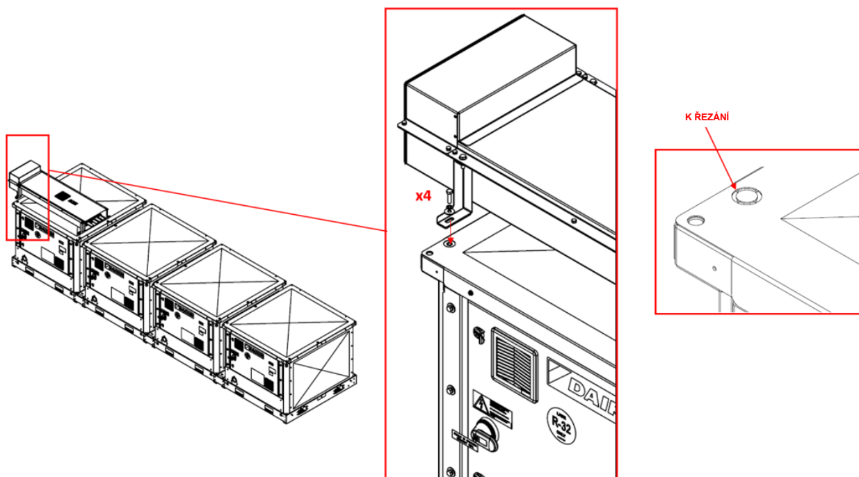
Obr. 54 - Upevnění systému napájecích tyčí k jednotce
