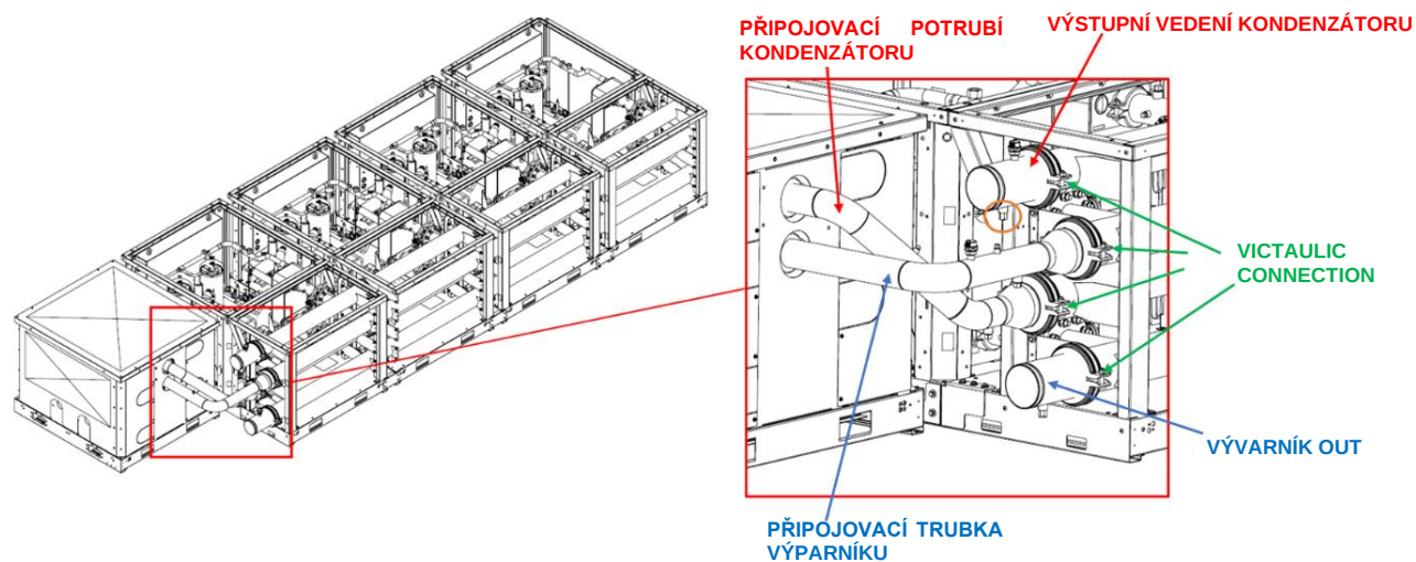
Obr. 45 - Instalace modulu čerpadla - detaily potrubí
