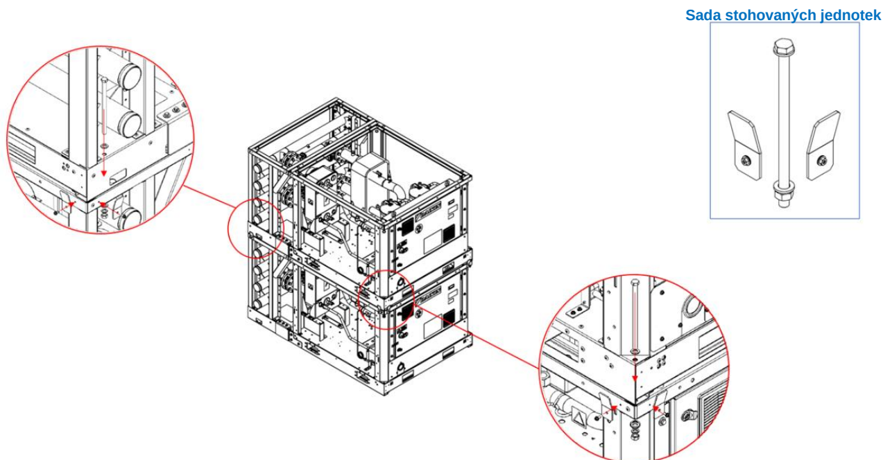
Obr. 42 - Pokyny pro montáž stohovaných jednotek
