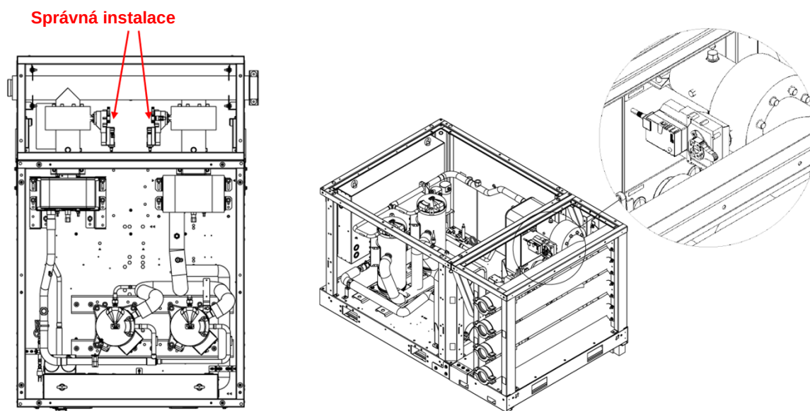
Obr. 33 - Montážní údaje pro pohon ventilu
