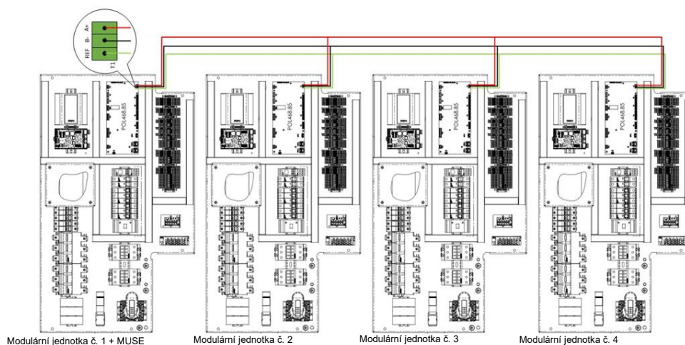
Obr. 63 - Zapojení 4 PLC do stejné sítě Modbus
