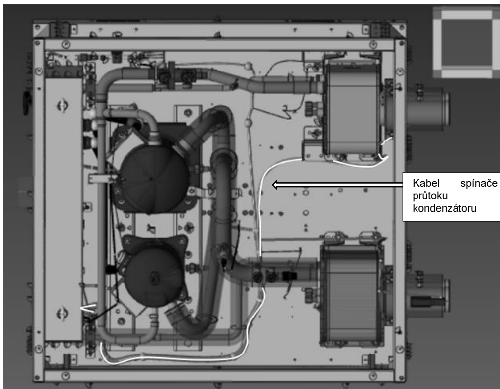
Obr. 17 - Vstupní místo elektrického panelu pro kabely spínače průtoku výparníku a kondenzátoru
