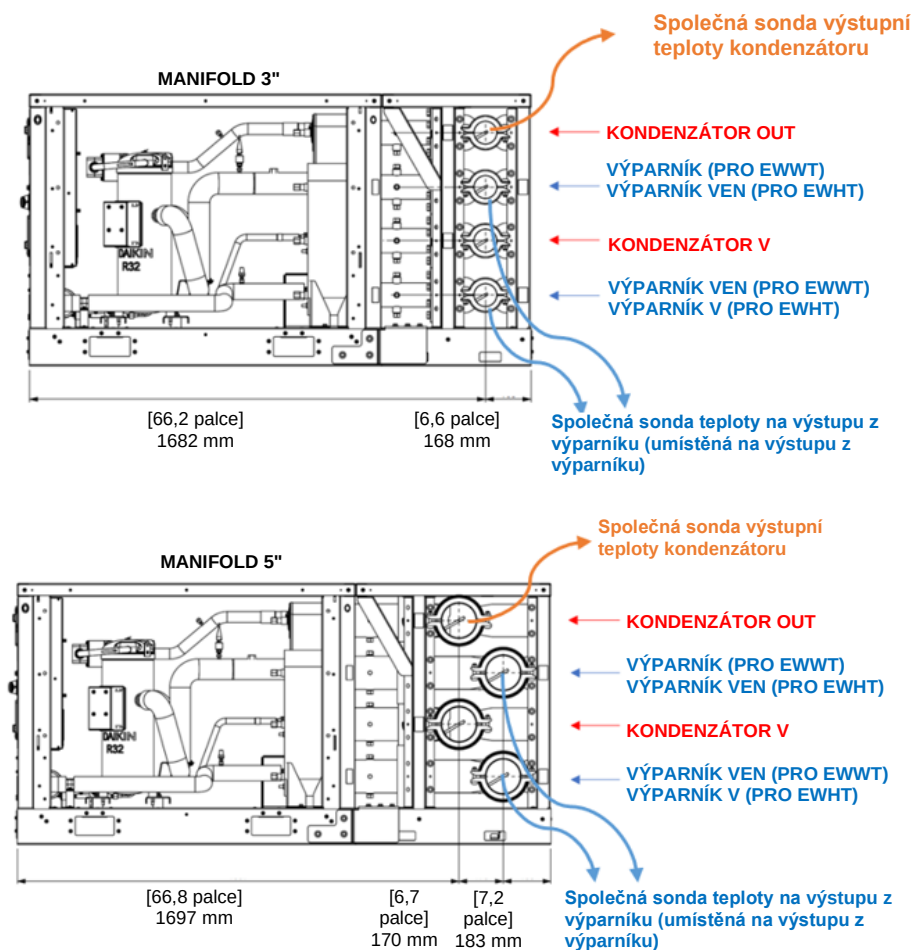
Obr. 61 - Umístění teplotních sond pro 3" a 5" rozdělovač
