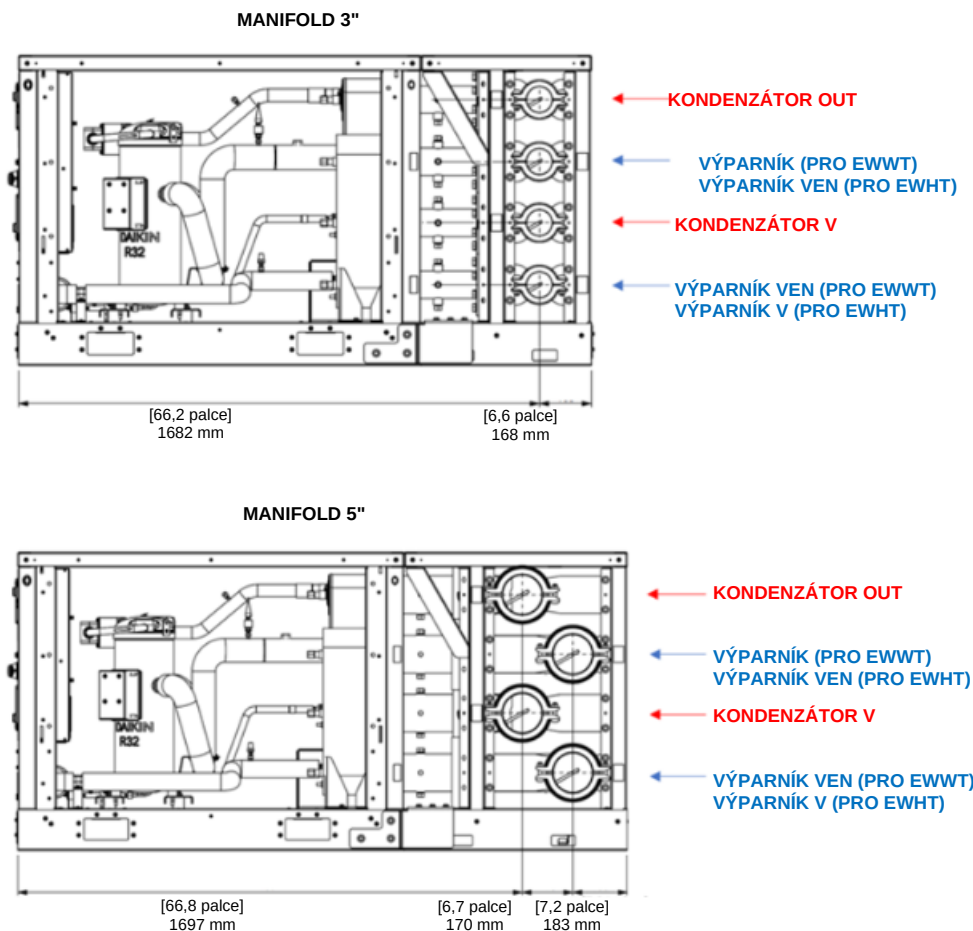
Obr. 29 - Rozměry rozdělovače vody
