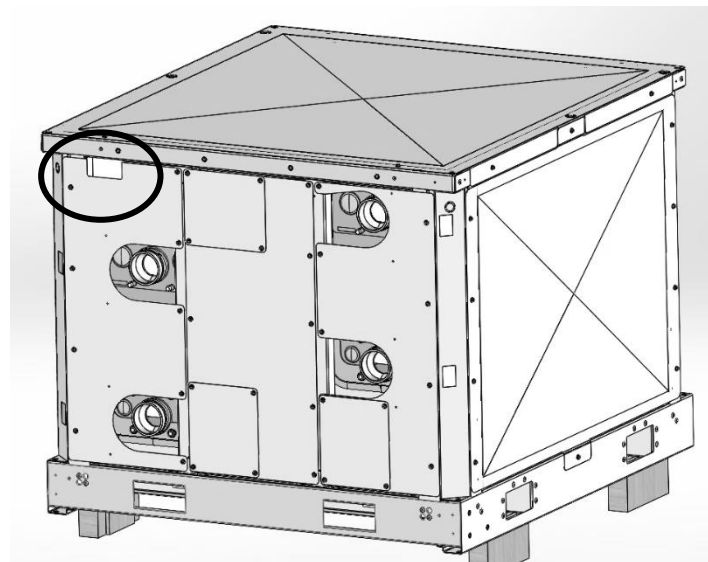
Obr. 12 - Poloha bezpečnostních ventilů jednotky
