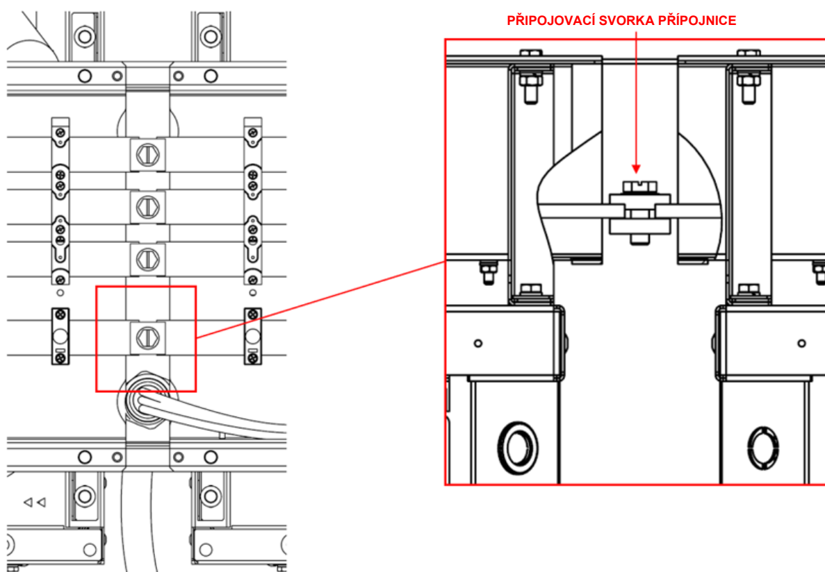
Obr. 56 - Detaily propojení modulů napájecí lišty dohromady
