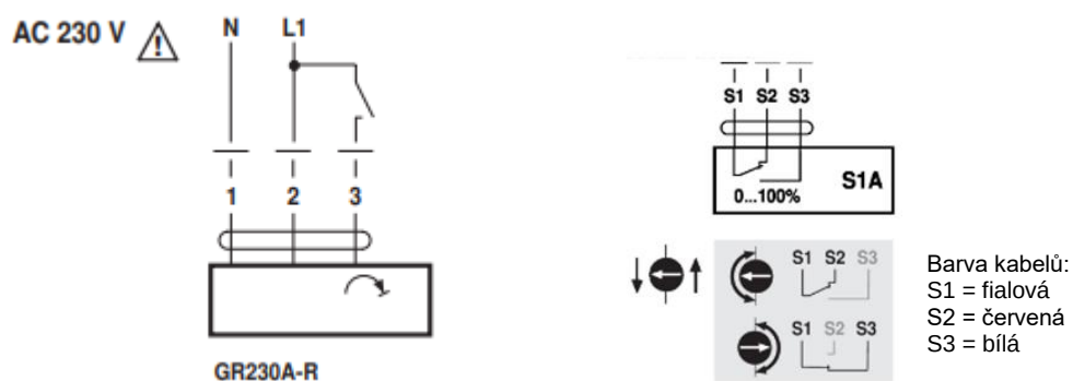
Obr. 34 - Schéma zapojení motoru (levý obrázek) a koncových spínačů (pravý obrázek)
