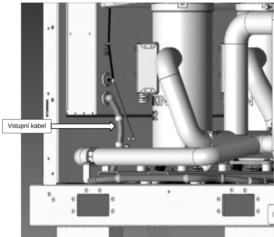
Obr. 40 - Vstup do elektrického panelu pro kabely pohonu uzavíracího ventilu výparníku a kondenzátoru
