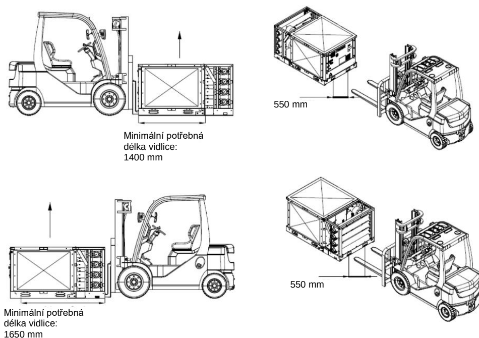
Obr. 47 - Manipulace s jednotkou a rozdělovacími moduly
