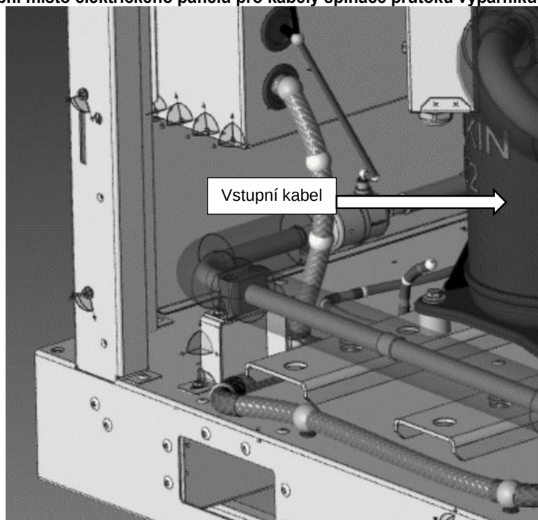
Obr. 17 - Vstupní místo elektrického panelu pro kabely spínače průtoku výparníku a kondenzátoru
