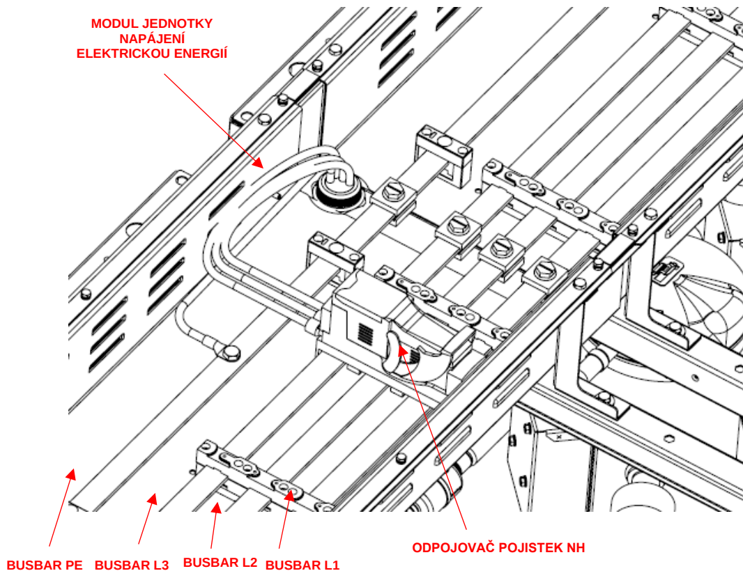
Obr. 59 - Detail elektrického připojení pro jakýkoli jiný modul jednotky
