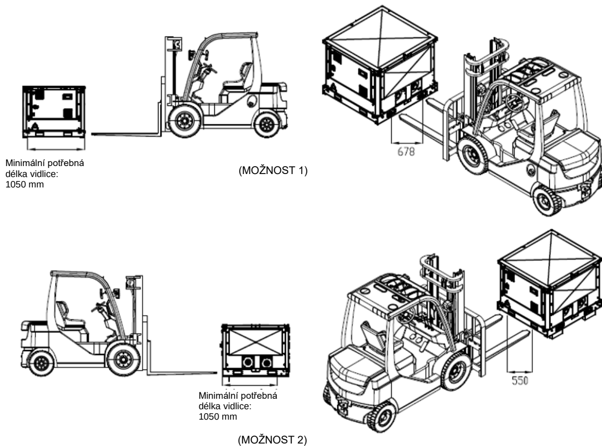
Obr. 49 - Manipulace s modulem čerpadla pomocí vysokozdvížného vozíku
