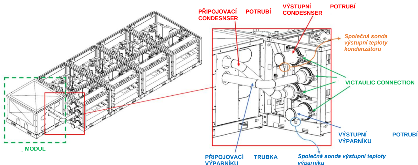
Obr. 62 - Detaily umístění sond na potrubí
