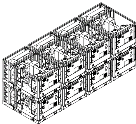
Obr. 43 - Pokyny pro montáž více systémů s jednotkovými rozvaděči dohromady
