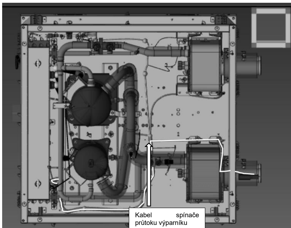
Obr. 15 - Vedení kabelů spínače průtoku výparníku
