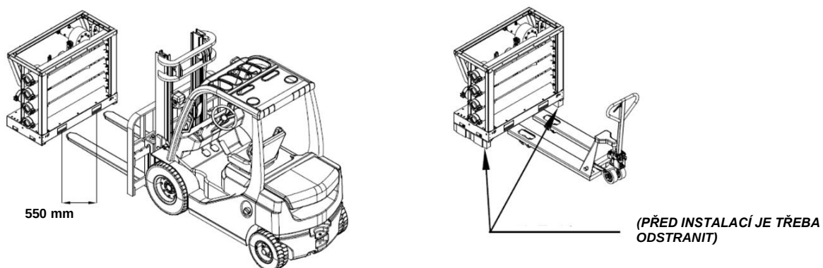
Obr. 46 - Manipulace s rozdělovacím modulem
