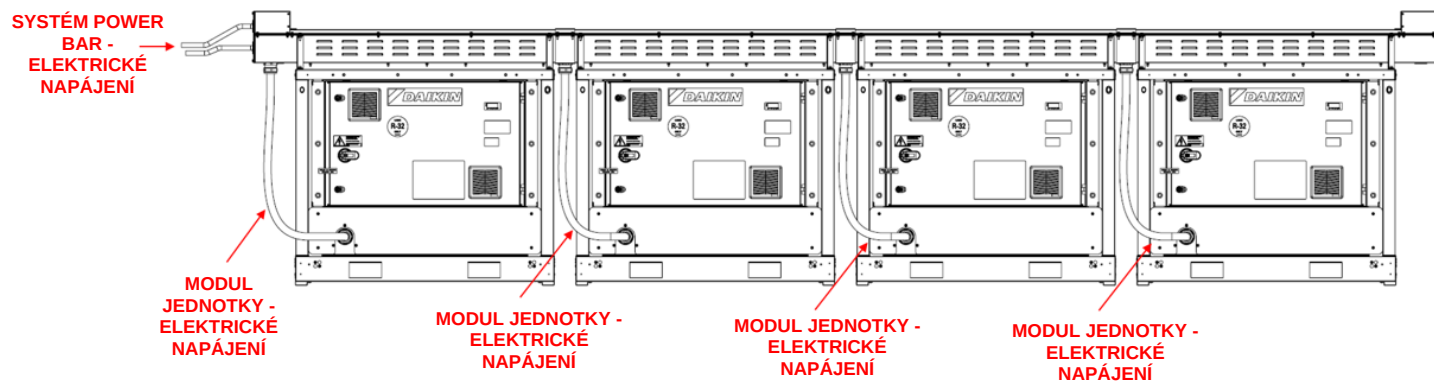
Obr. 52 - Vedení kabelů mezi lištovým systémem a jednotkou
