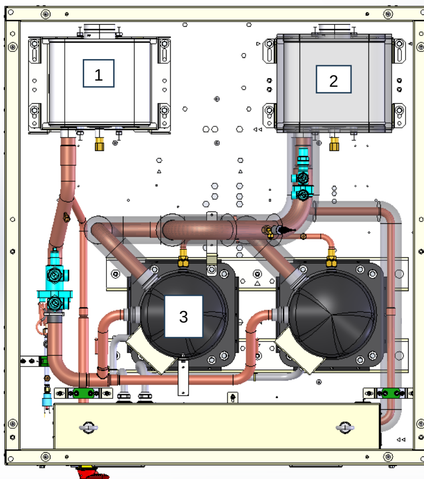
Obr. 13 - Referenční výkres pro identifikaci výparníku a kondenzátoru
