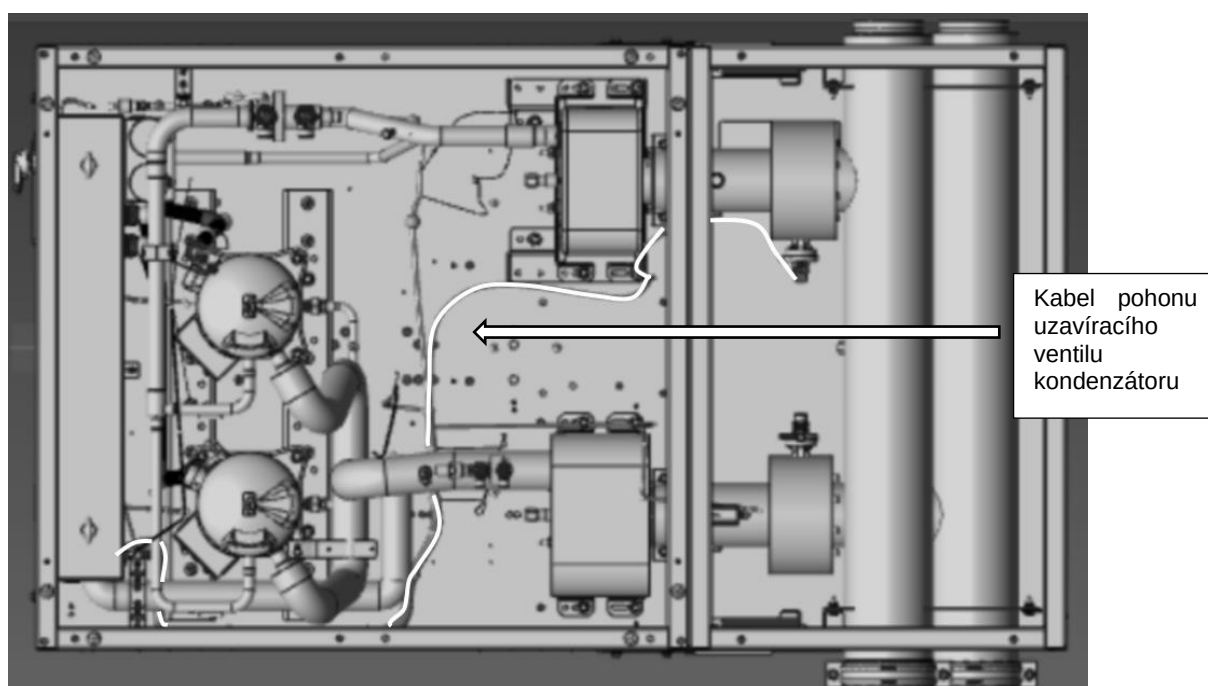
Obr. 39 - Vedení kabelů pohonu uzavíracího ventilu kondenzátoru
