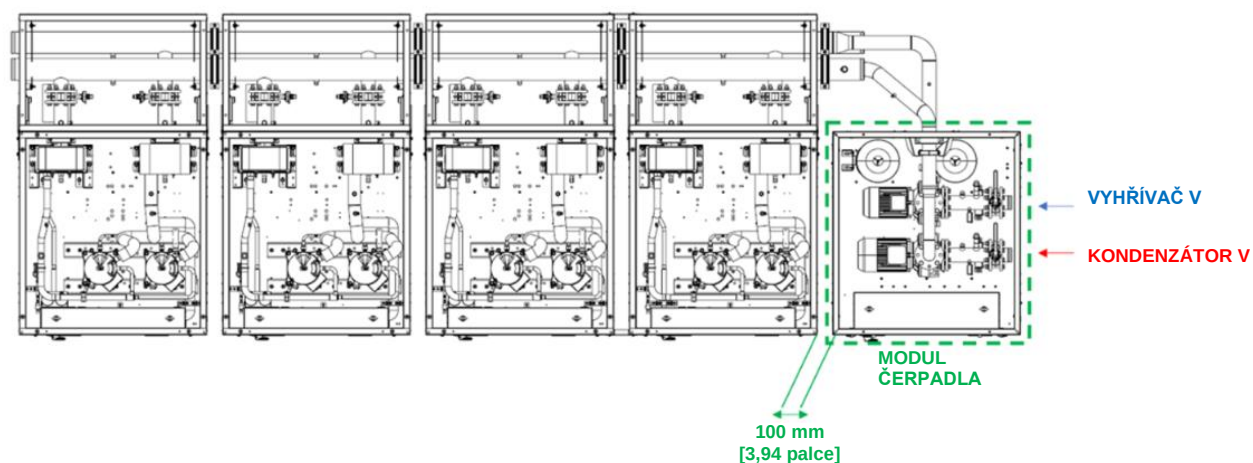
Obr. 45 - Instalace modulu čerpadla - detaily potrubí
