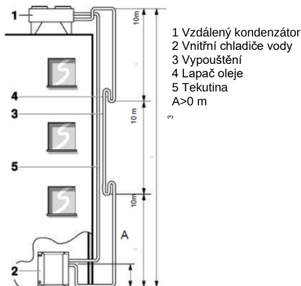
Obr. 19 - Připojení chladicího okruhu (1)
