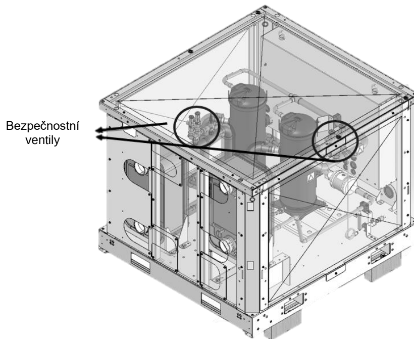
Obr. 11 – Poloha bezpečnostních ventilů jednotky
