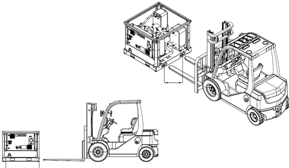
Obr. 8 - Manipulace s jednookruhovou jednotkou
