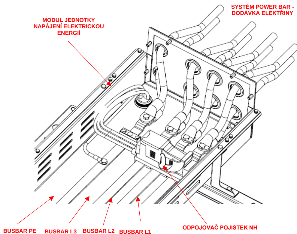
Obr. 58 - Detail elektrického zapojení počátečního modulu jednotky
