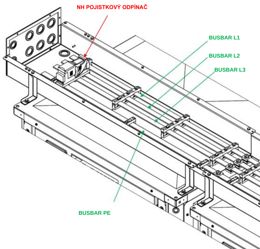
Obr. 57 - Detail pojistek a krabice pro vedení kabelů modulu napájecí lišty
