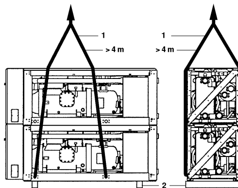
Figura 3- Sollevamento
