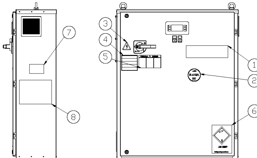
Obrázek 1 – Identifikace štítků aplikovaných na elektrickém panelu (Standardní*) Kompresor s jedním okruhem
