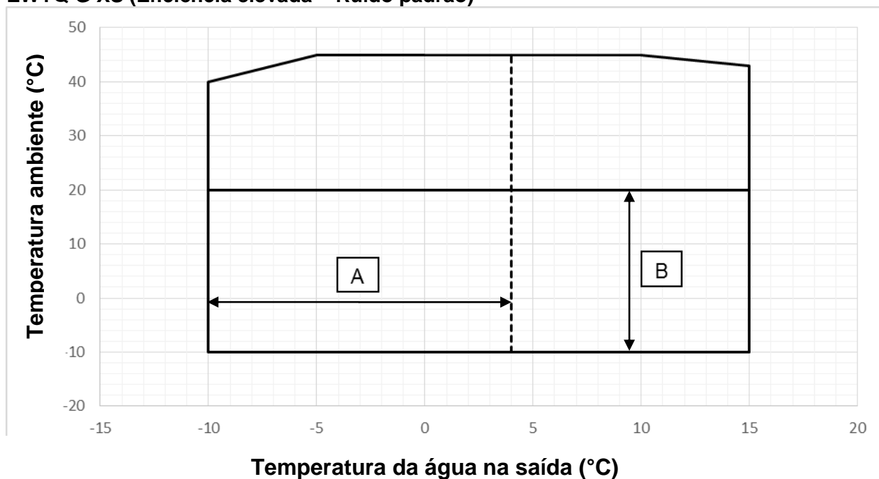
Figura 2 - Limites de funcionamento em modo de refrigeração
