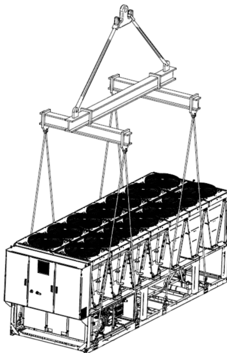
Enhet med åtta lyftpunkter
