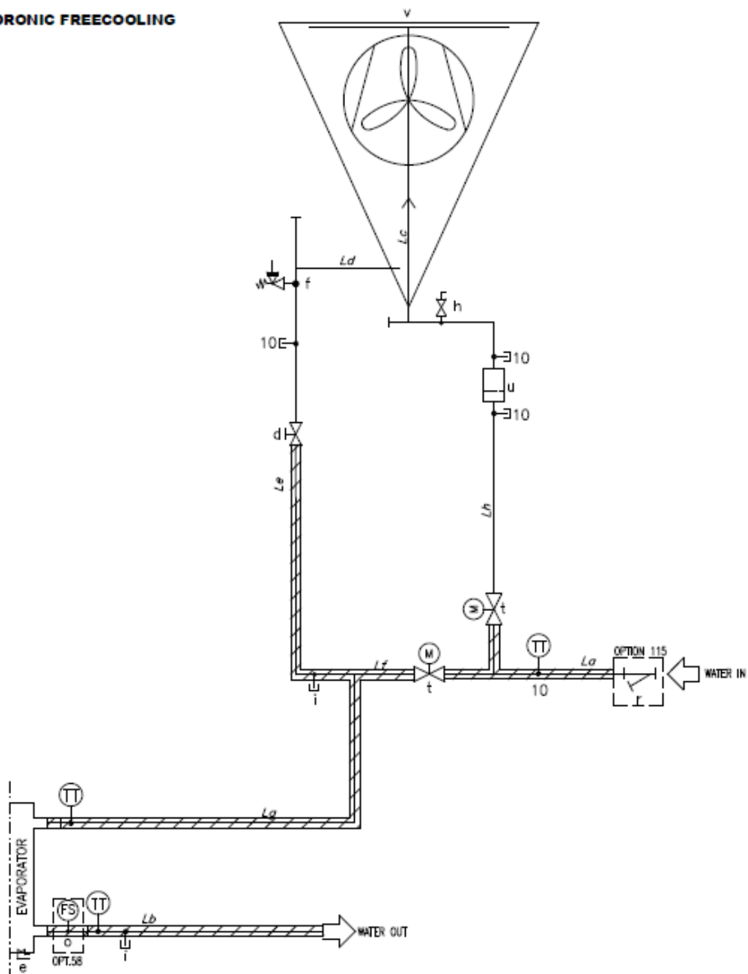
Slika 3– Hidronični sistem za prosto hlajenje (P&ID)
