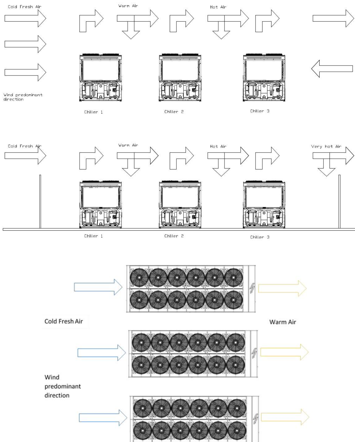
Slika 17– Namestitev več hladilnikov
