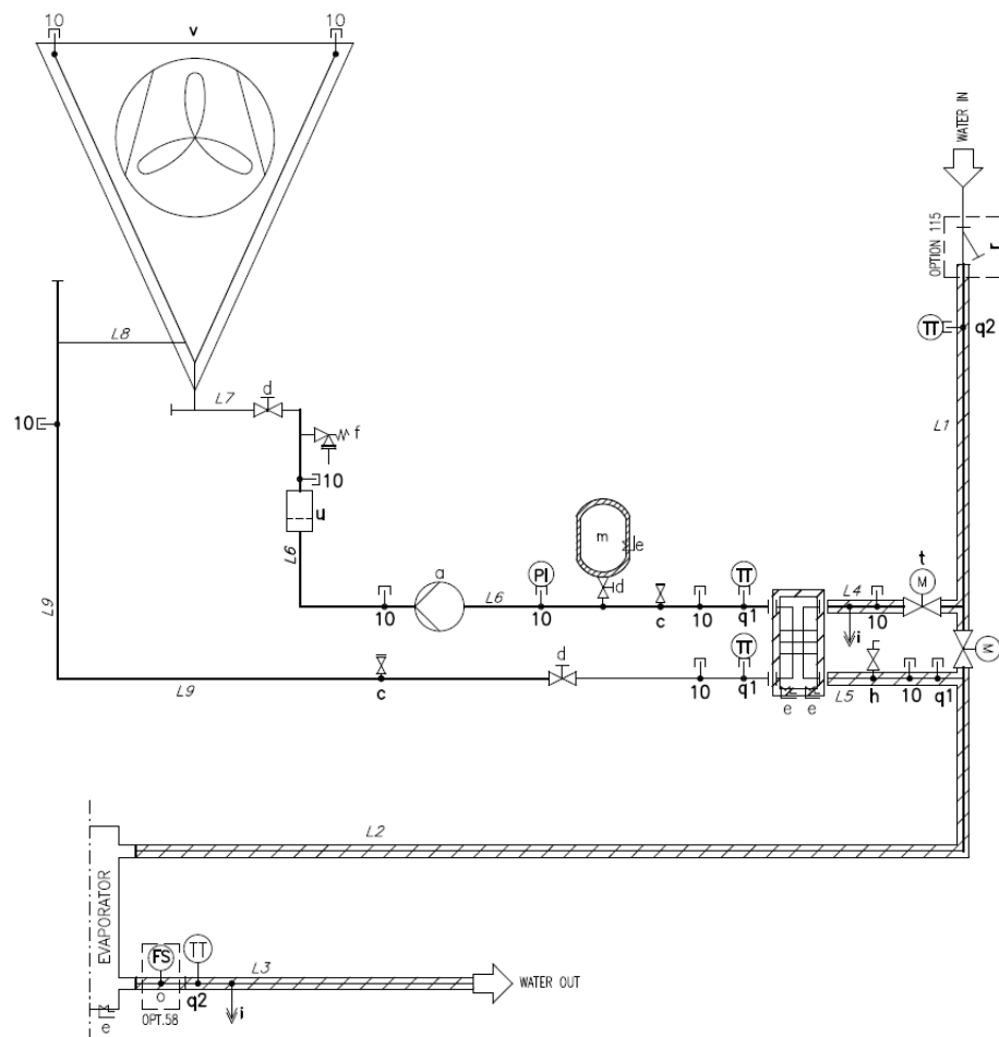
Fig. 21– Circuit fermé Hydronic Free cooling P&ID (Opt. 231)
