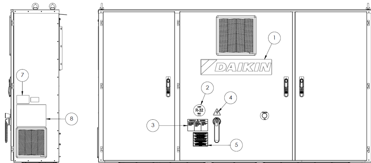
Fig. 22– Description des étiquettes appliquées sur le Table électrique
