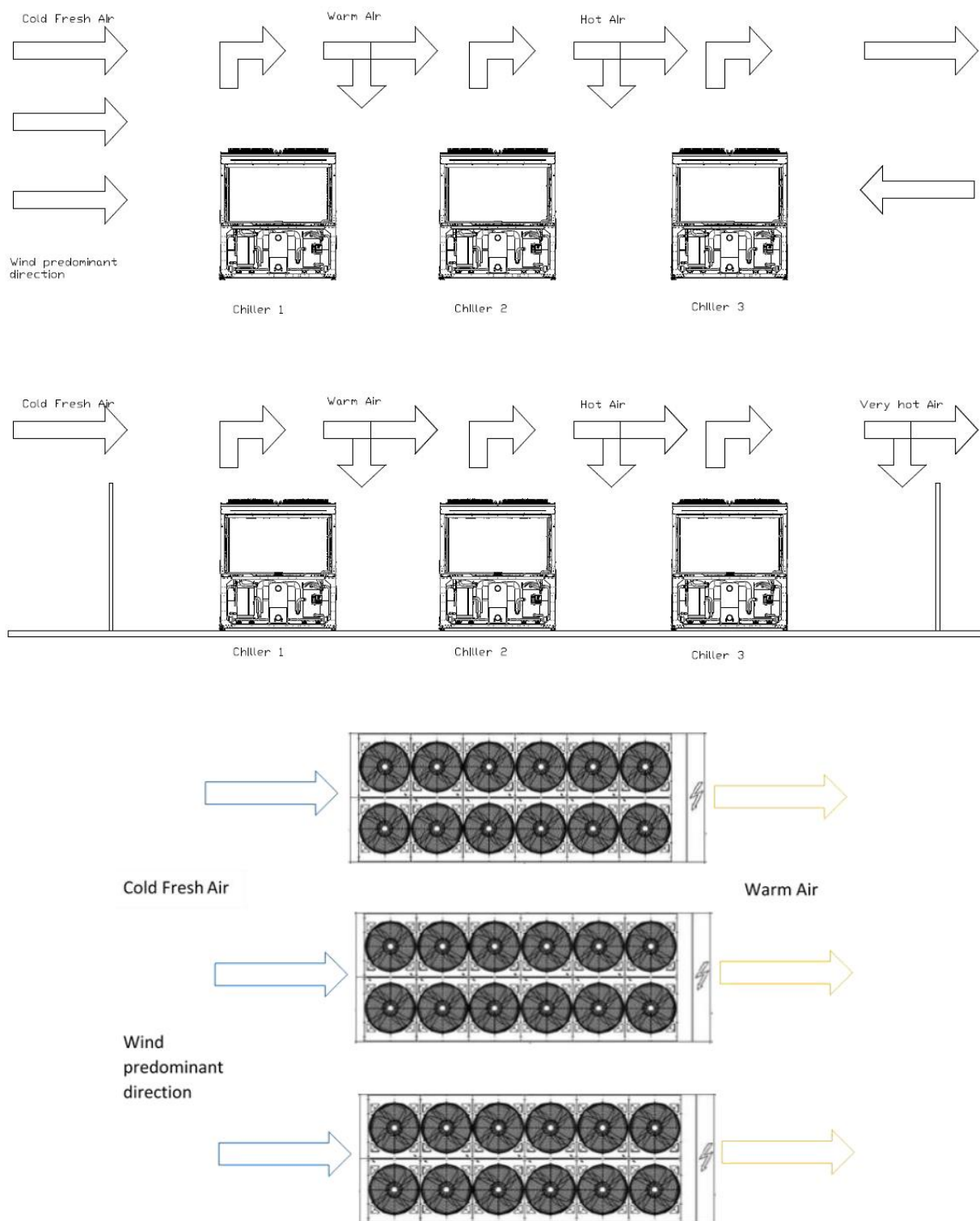
Fig. 15– Installation de refroidisseurs multiples
