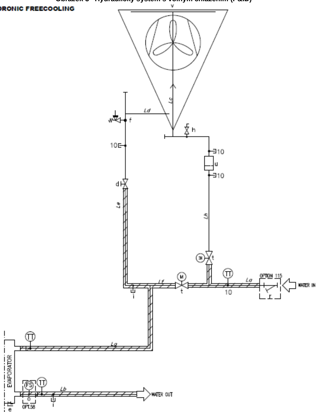
Obrázek 3– Hydraulický systém s volným chlazením (P&ID)
