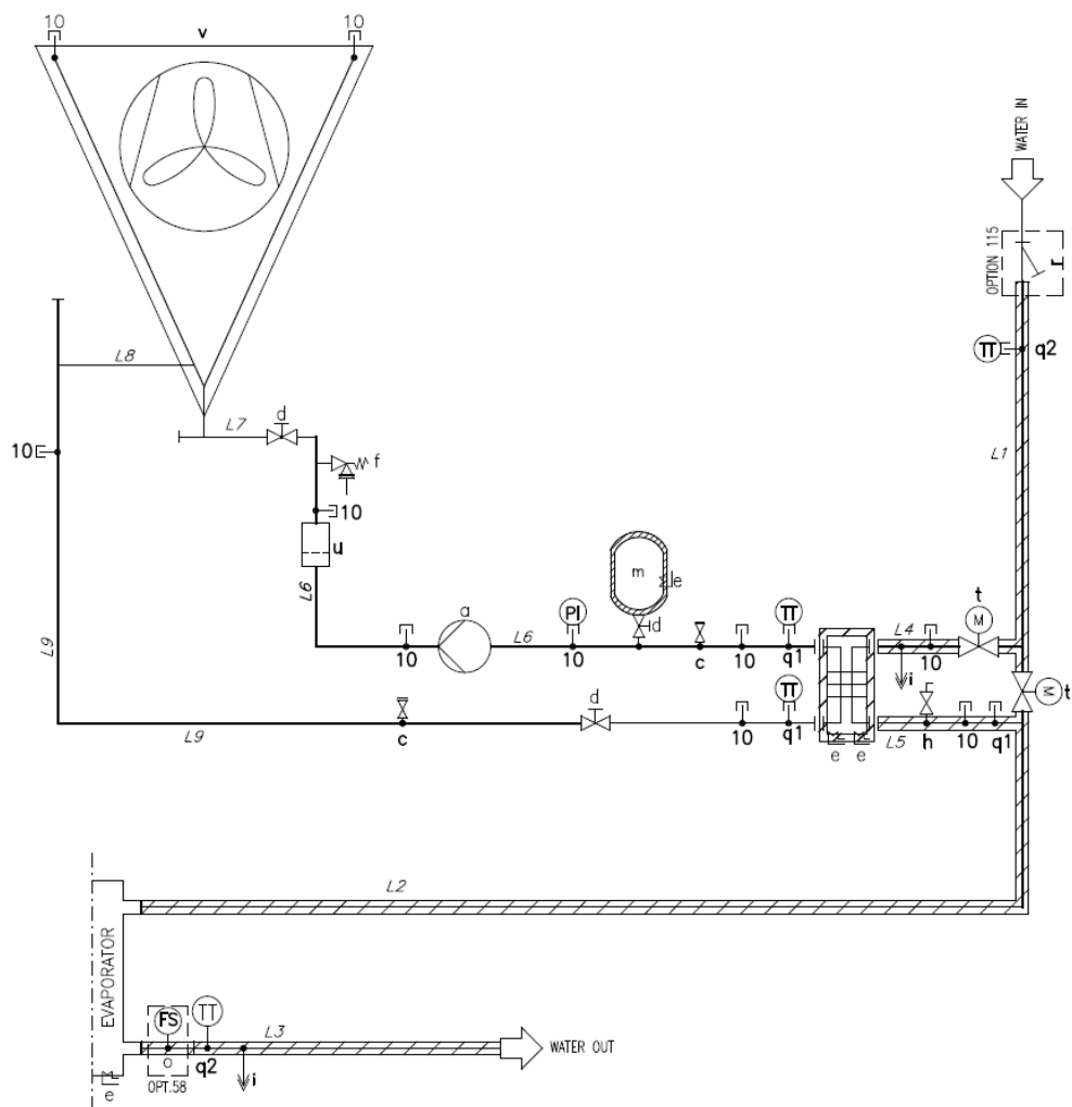
Obrázek 26- Uzavřená smyčka Hydronic Free cooling P&ID (Opt. 231)
