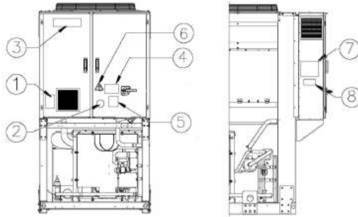
Şekil 1 - Elektrik panoda bulunan işaretlerin açıklaması
