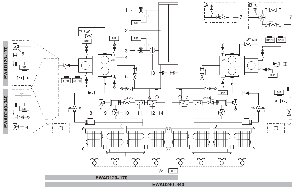
Figur - Funktionsdiagram
