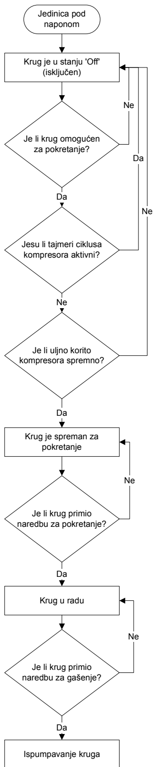
Slika 6, Slijed operacija kruga
