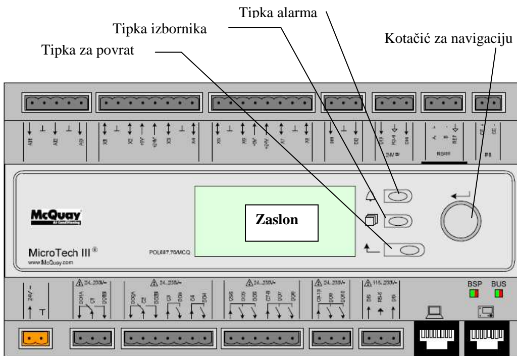
Slika 7, Kontroler jedinice
