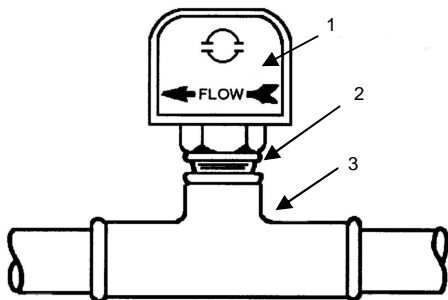
Afbeelding 2 - Installatie stromingsschakelaar
