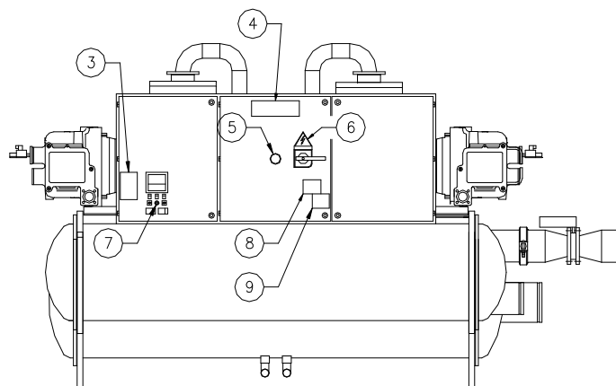
Unit met 2 compressoren
