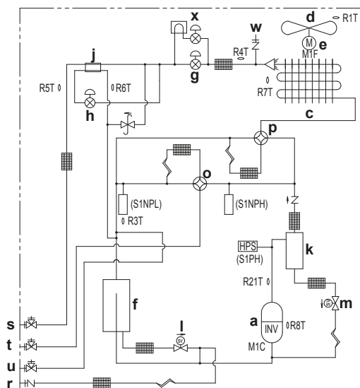
Schema cjevovoda: RYMQ8~12
