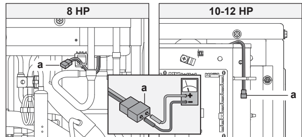
a Конектор за проверка на напрежението на кондензатора
