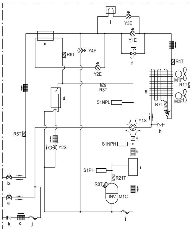
Rördragningsschema: 8 HP
