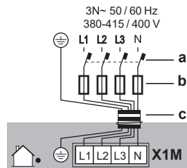
a Jordfelsbrytare b Säkring c Strömförsörjningskabel
