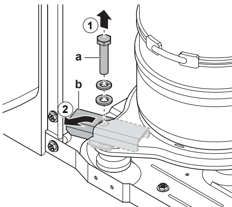
a Bult b Transportstöd
