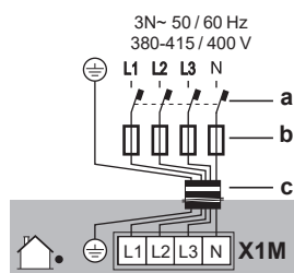
a Disjuntor contra fugas para a terra b Fusível c Cabo da fonte de alimentação
