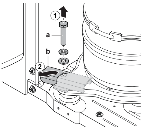
a Csavar b Szállítótámasztékek
