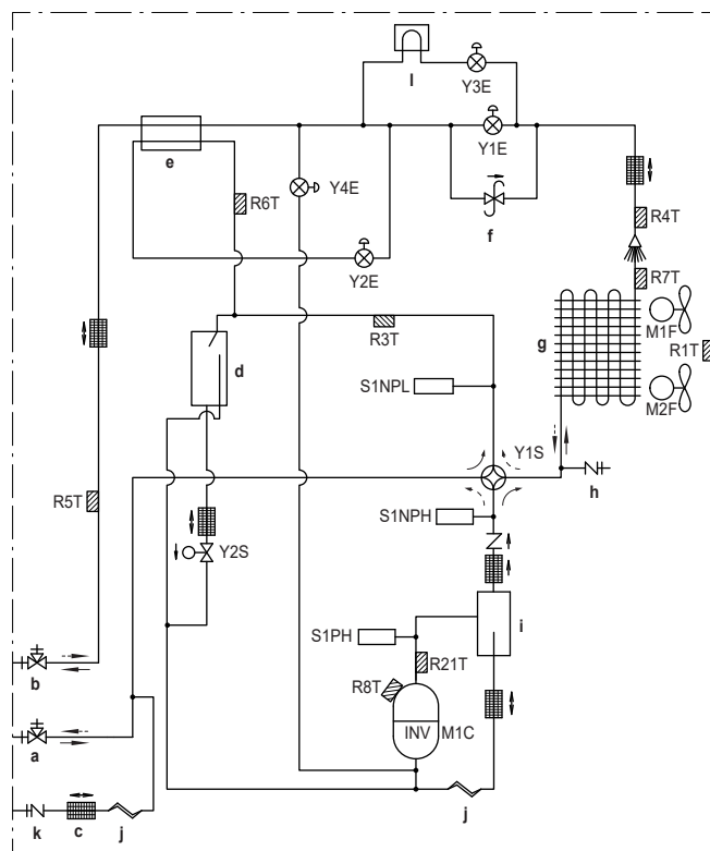
Διάγραμμα σωληνώσεων: 10+12 HP
