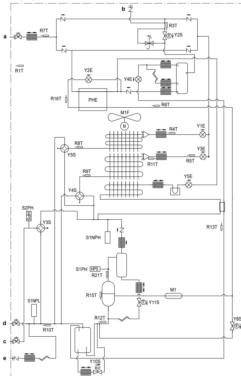
Rördragningschema: 5~12 HP
