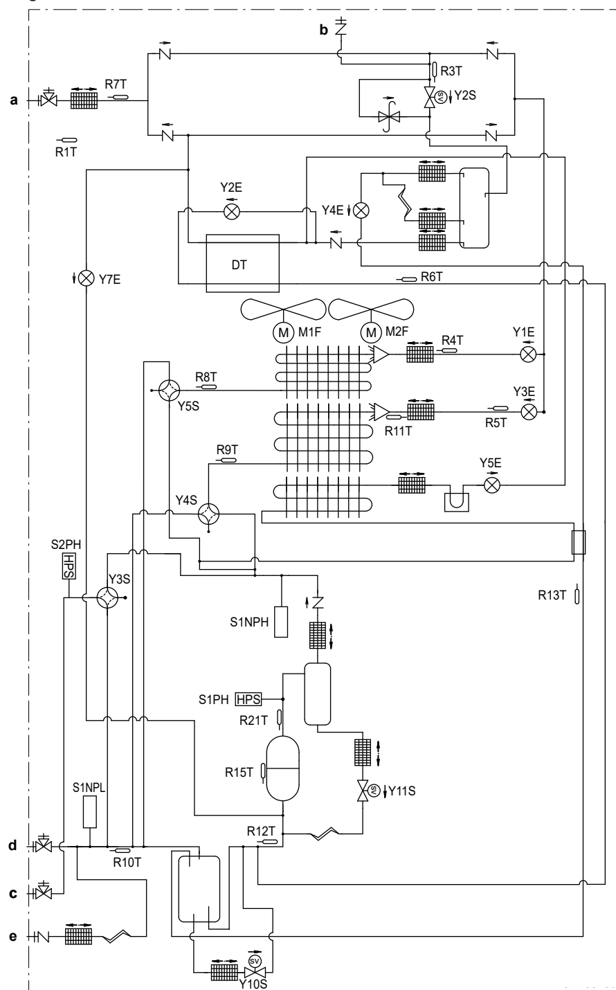
Diagram cevovoda: 14~20 HP
