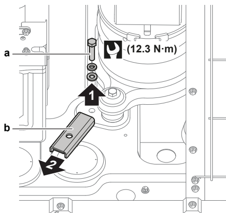
a Csavar b Szállítótámaszték
