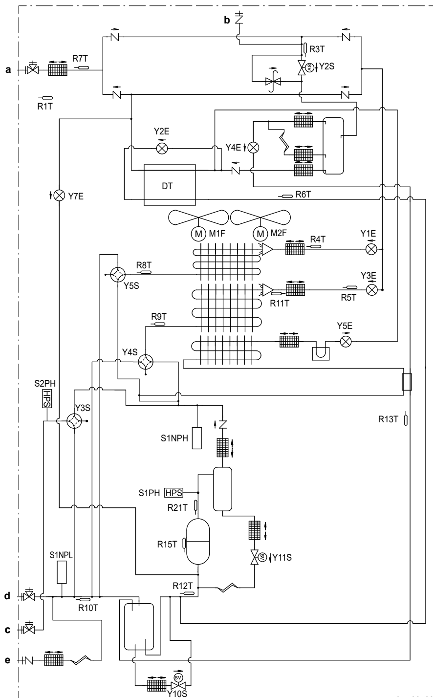
Csőszerelési ábra: 14~20 HP
