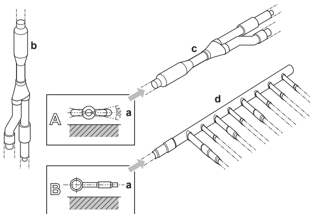
a Superficie horizontal b Junta Refnet montada en vertical c Junta Refnet montada en horizontal d Colector
