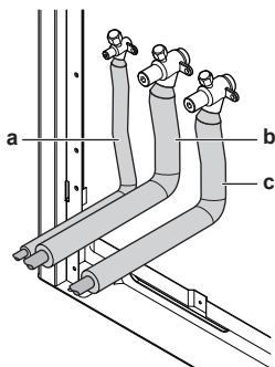
a Potrubí kapaliny b Vyrovnávací potrubí c Potrubí plynu
