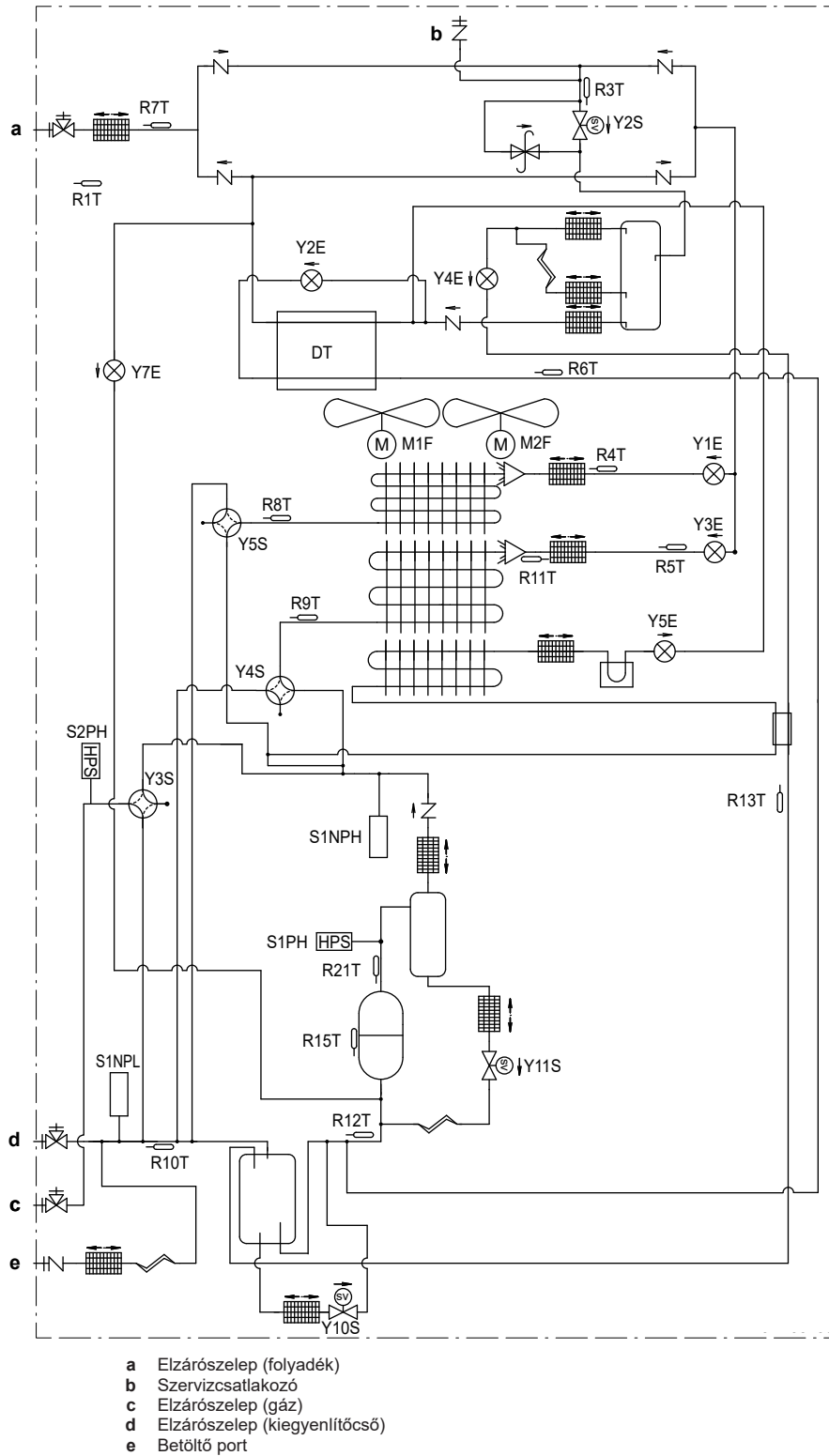
Csőszerelési ábra: 14~20 HP
