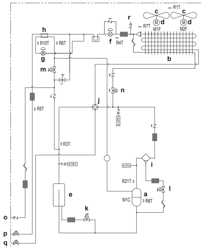
Vamzdžių schema. RXMLQ8 + RXYLQ10~14
