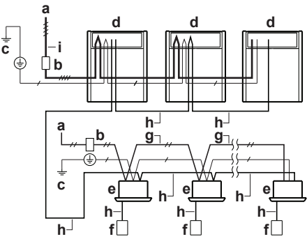
а Праводка, што пракладваецца на месцы ўсталявання (з апаратам засцярогі ад уцечкі ў зямлю)
