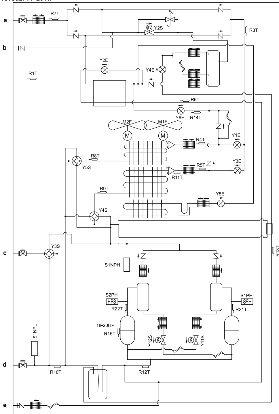
Diagram cevovoda: 14~20 HP
