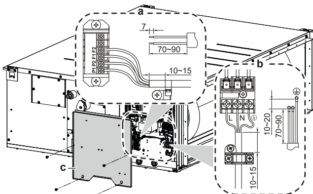
a Кабел за кориснички интерфејс и кабел за меѓусебно поврзување b Кабел за снабдување со електрична енергија c Капак за сервисирање со дијаграм за вжичување
