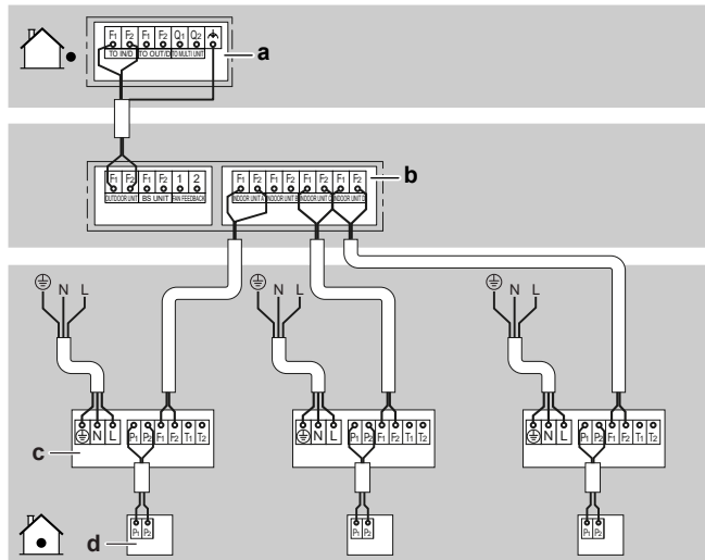
a Надворешна единица b Повеќекратна BS единица c Внатрешна единица d Кориснички интерфејс
