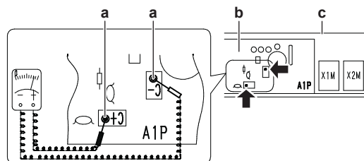
a Точки за измерване на остатъчно напрежение b Печатна платка c Контролна кутия
