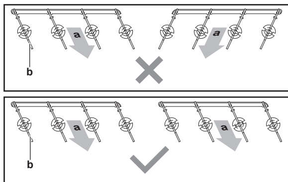
a Въздушна струя b Вертикални ребра
