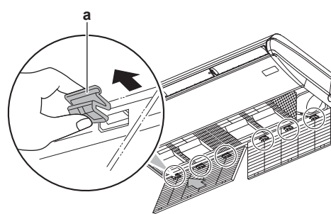
а Скоба
