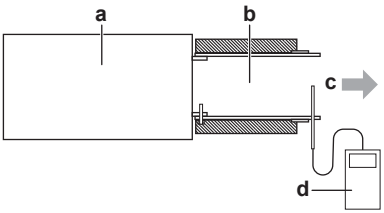
a BS ünitesi b Hava çıkış kanalı c Hava akış yönü d Kızgın telli rüzgar ölçer
