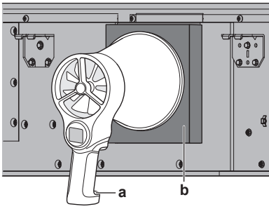
a Pervaneli rüzgar ölçer b Kanal bağlantı kiti (EKBSDCK)
