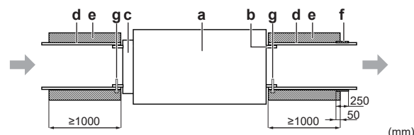
a BS-enhet b Luftkanal (luftutlopp) c Tillvalspaket EKBSDCK (luftintag) d Luftkanal (anskaffas lokalt) e Isolering (anskaffas lokalt) f Tätning (tillbehör) g Skruv (anskaffas separat)
