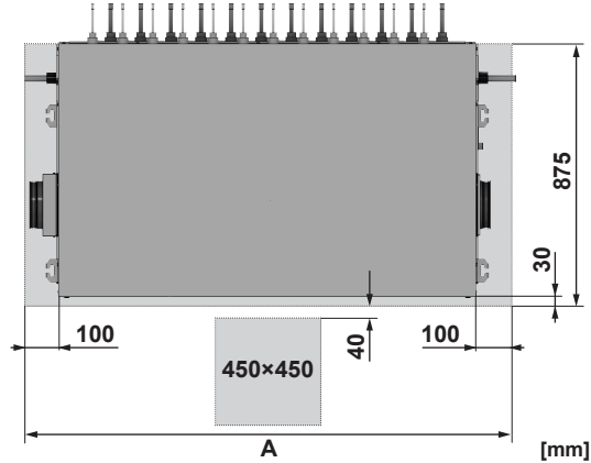
A Mått, öppning i innertak:
