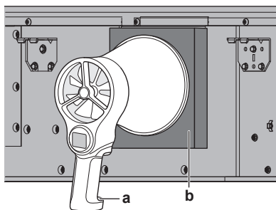
a Anemometer b Luftkanalanslutningspaket (EKBSDCK)
