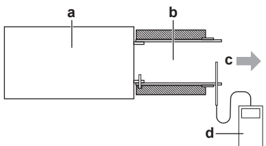
a BS-enhet b Luftutloppskanal c Riktning luftflöde d Anemometer med varm tråd
