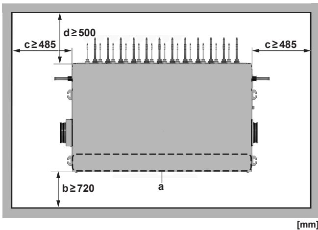
a T-koppling
